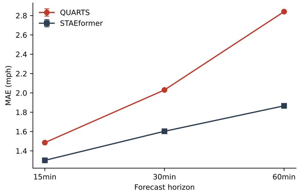
PEMS BAY
