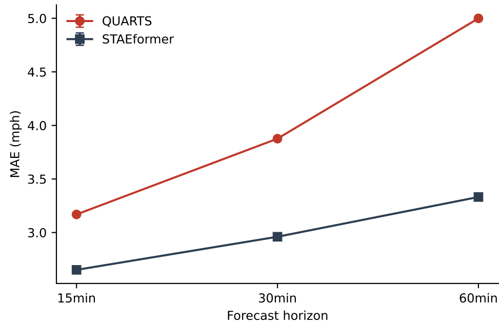
METR LA
