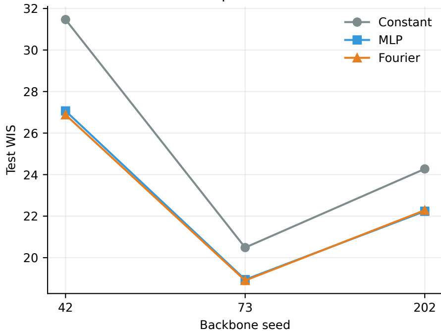
PeMSD4 independent backbones
