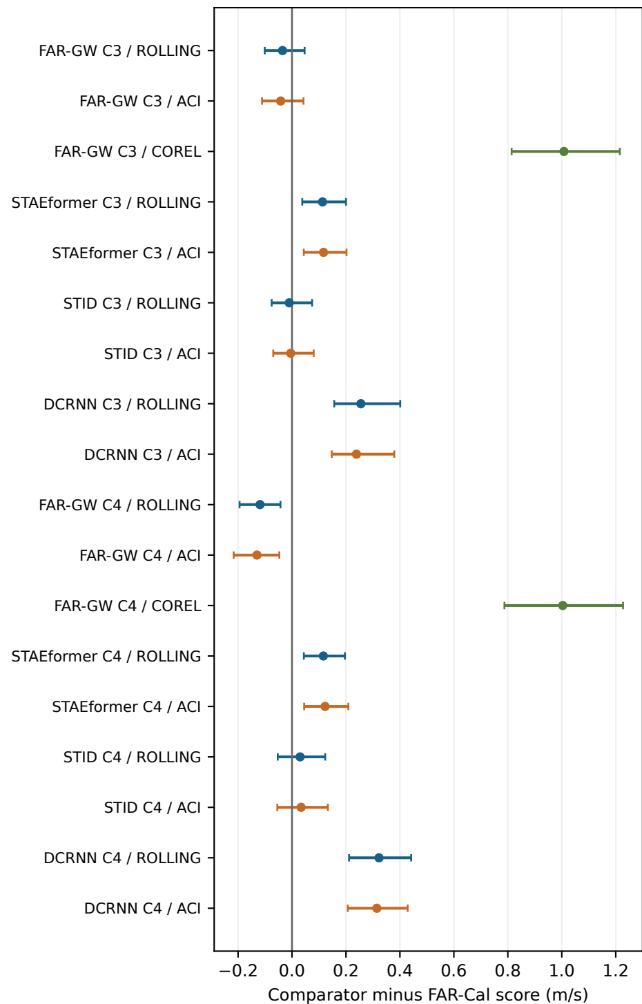
PEMS-BAY
