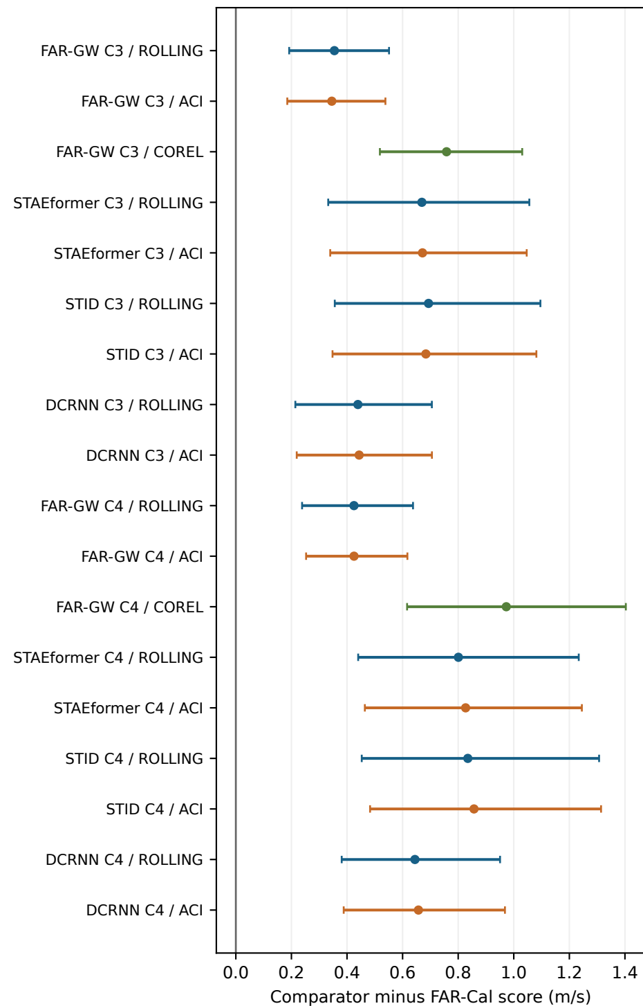
METR-LA
