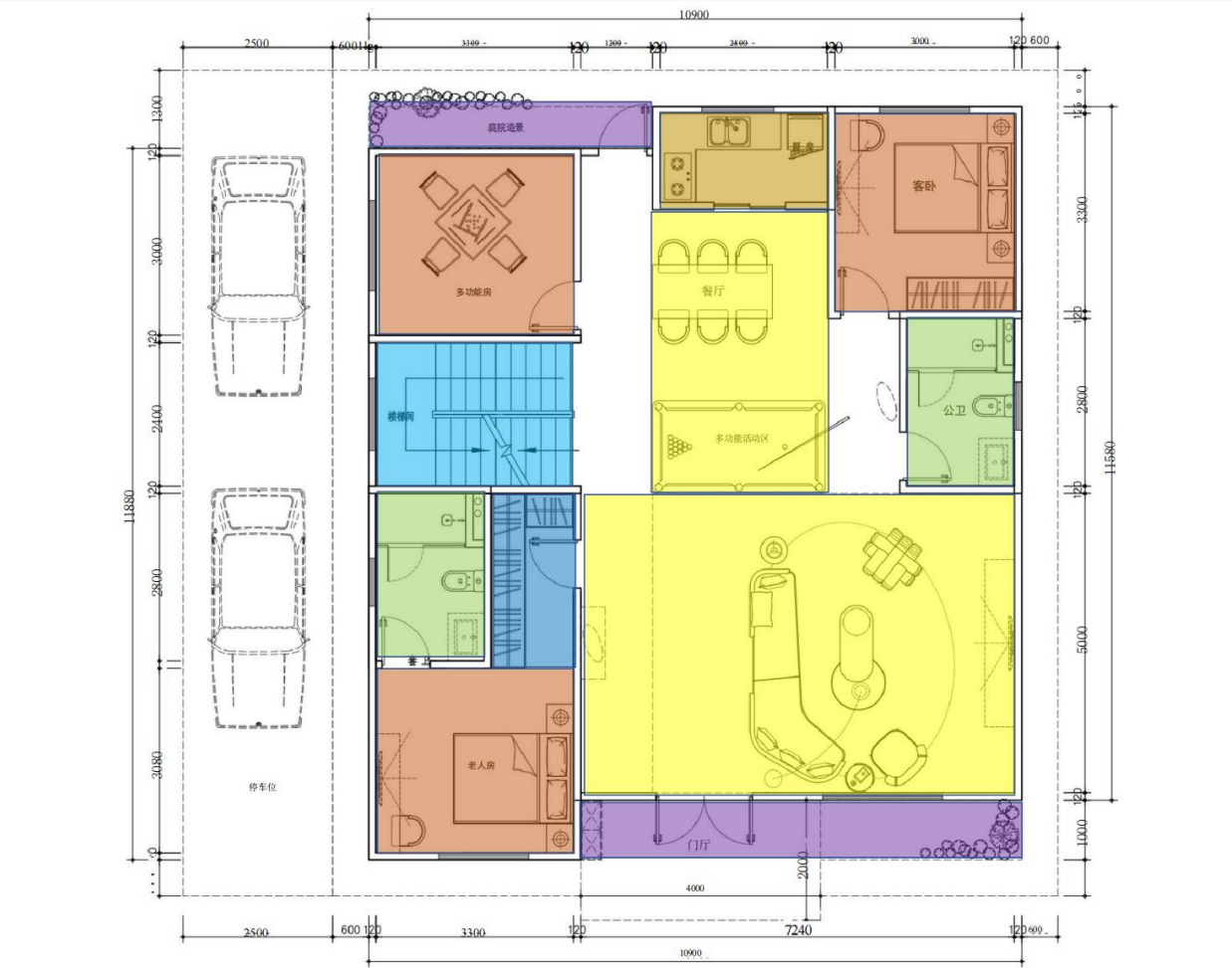
200户型一层平面布置图(套内面积120m²)
