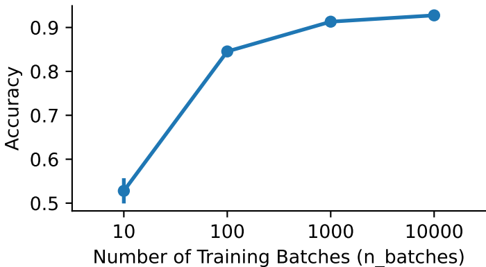
Softmax Regression (n_models=10)
