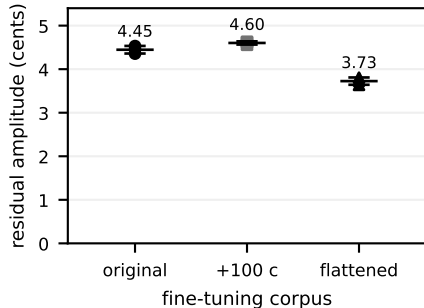
(d) decoder fine-tuning, 3 seeds per arm
