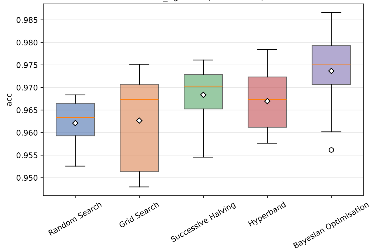
rbv2_xgboost (Dataset 16)
