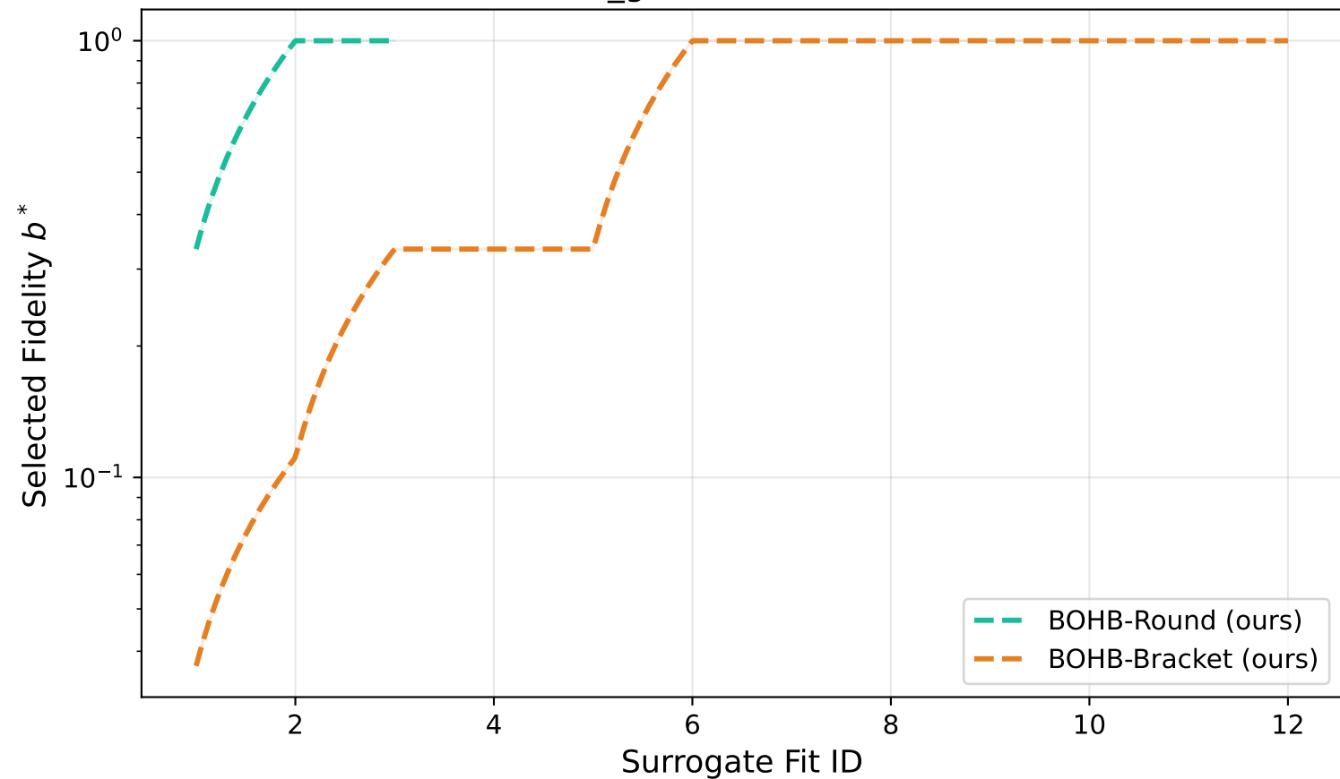
rbv2\_glmnet (Dataset 16)
