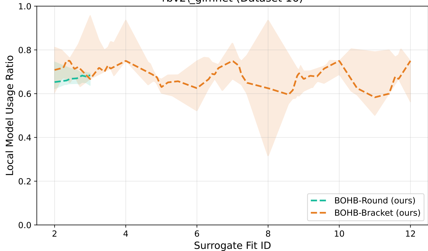
rbv2\_glmnet (Dataset 16)
