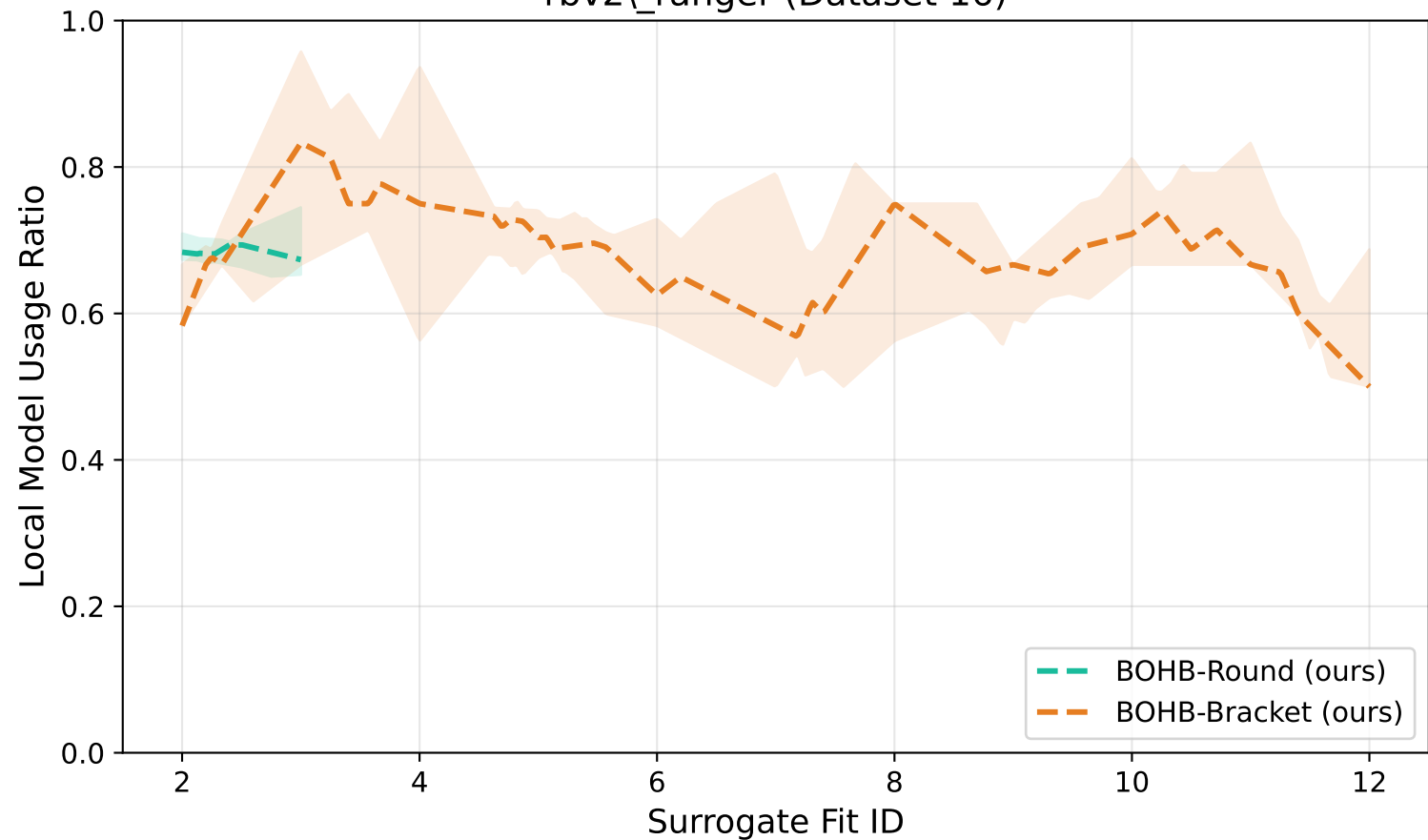
rbv2\_ranger (Dataset 16)
