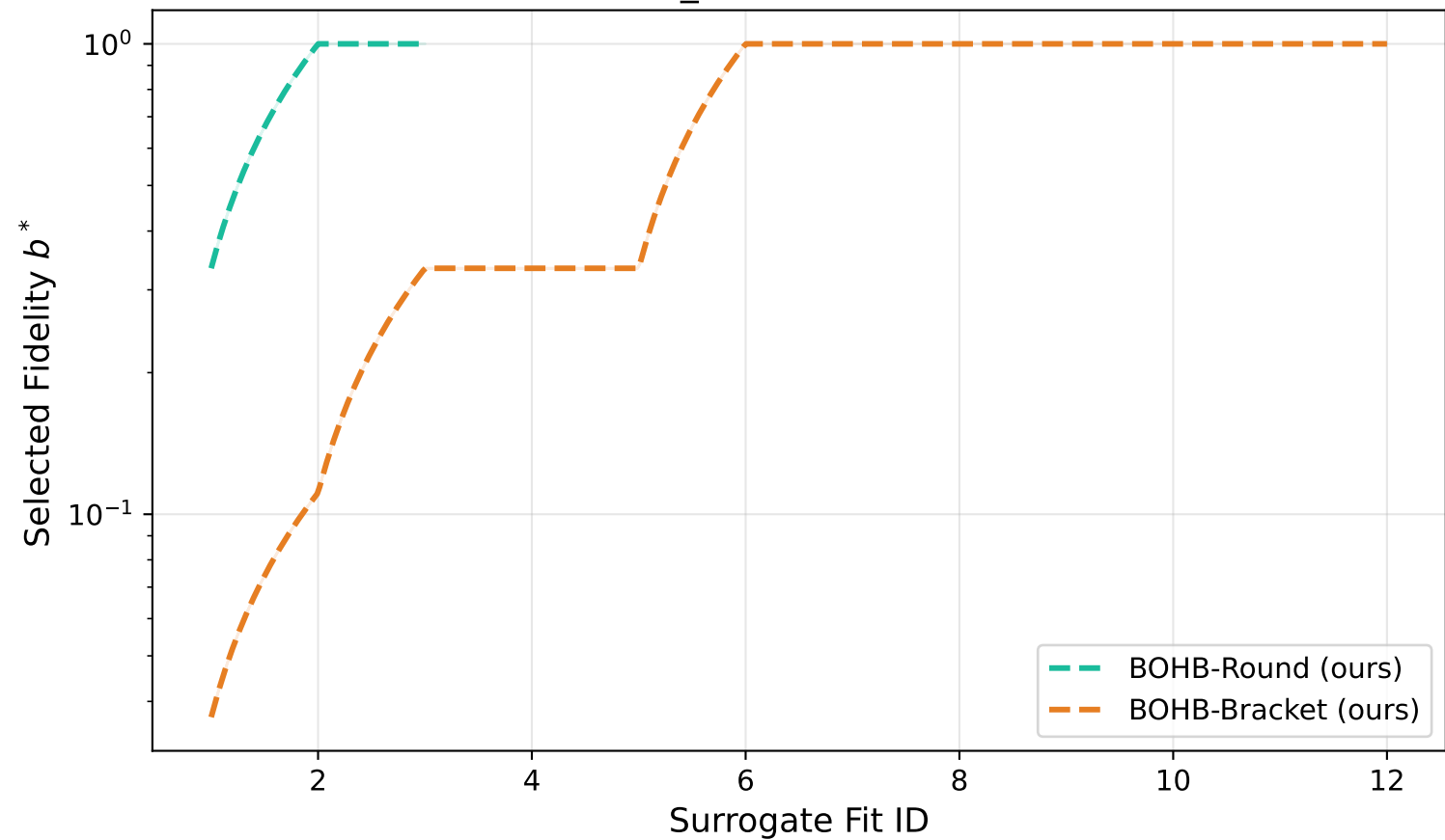
rbv2\_svm (Dataset 16)
