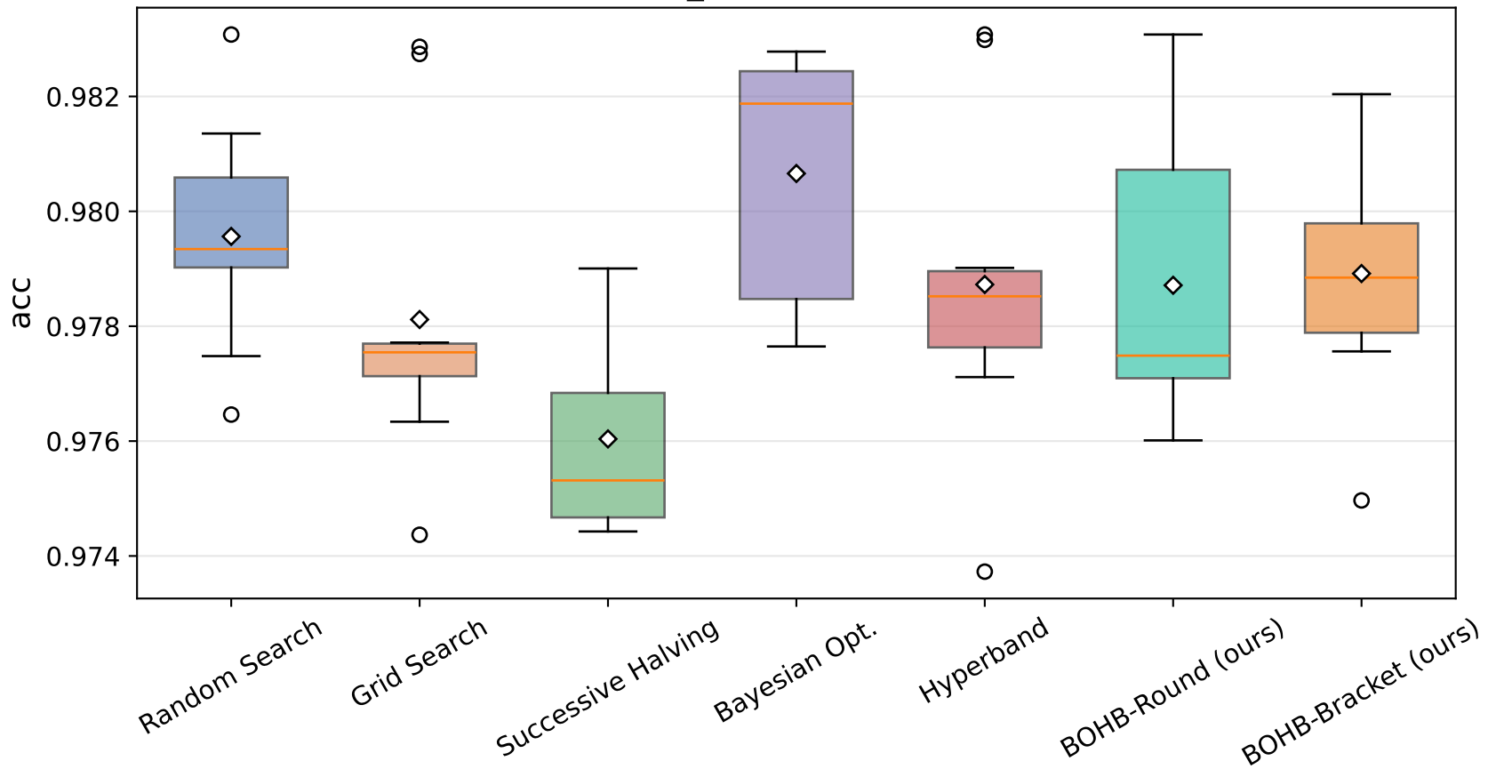
rbv2\_svm (Dataset 16)
