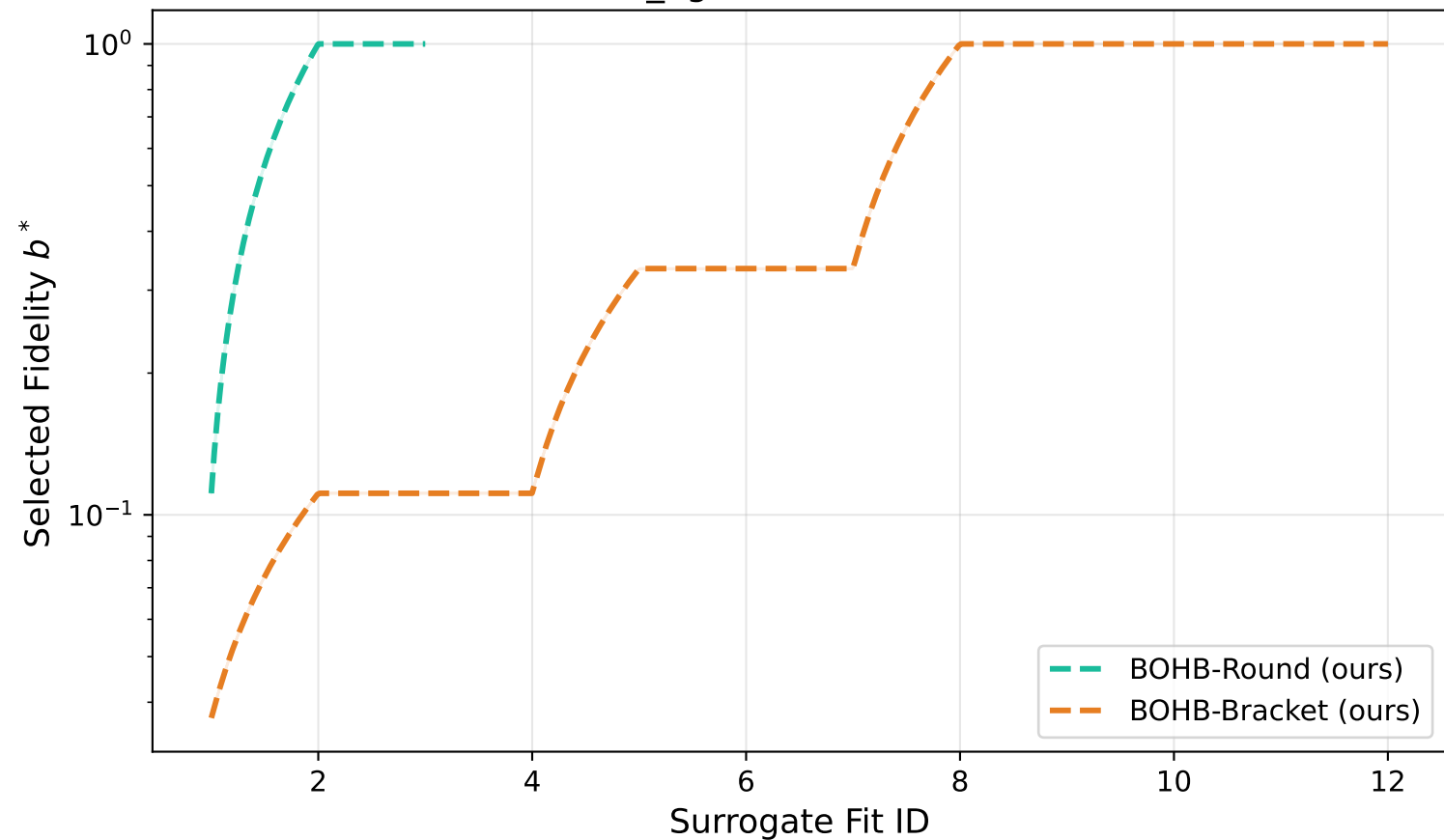
rbv2\_xgboost (Dataset 16)
