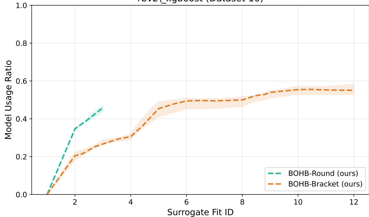
rbv2\_xgboost (Dataset 16)
