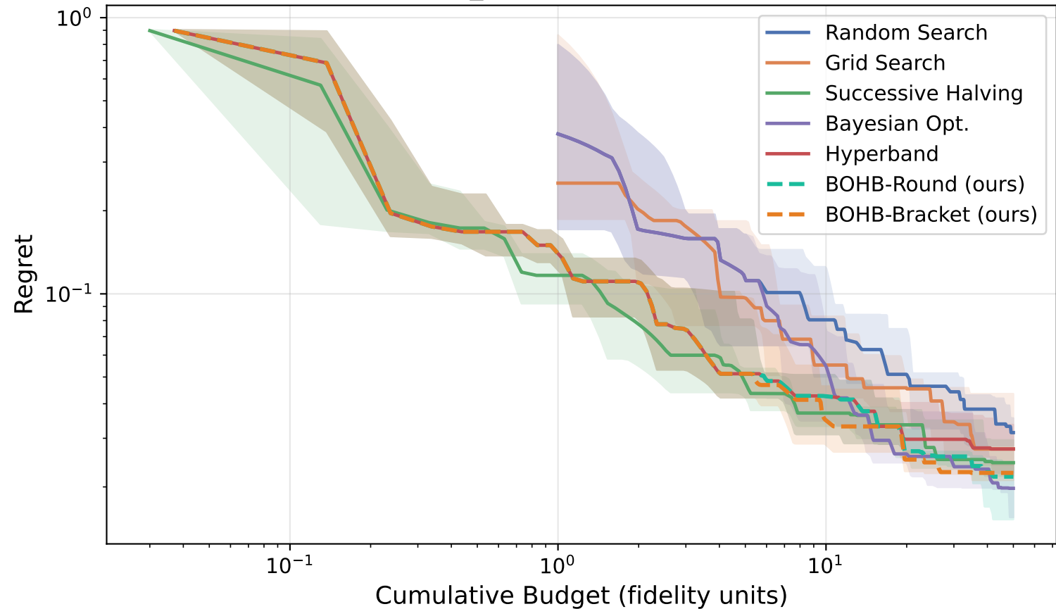
rbv2\_xgboost (Dataset 16)
