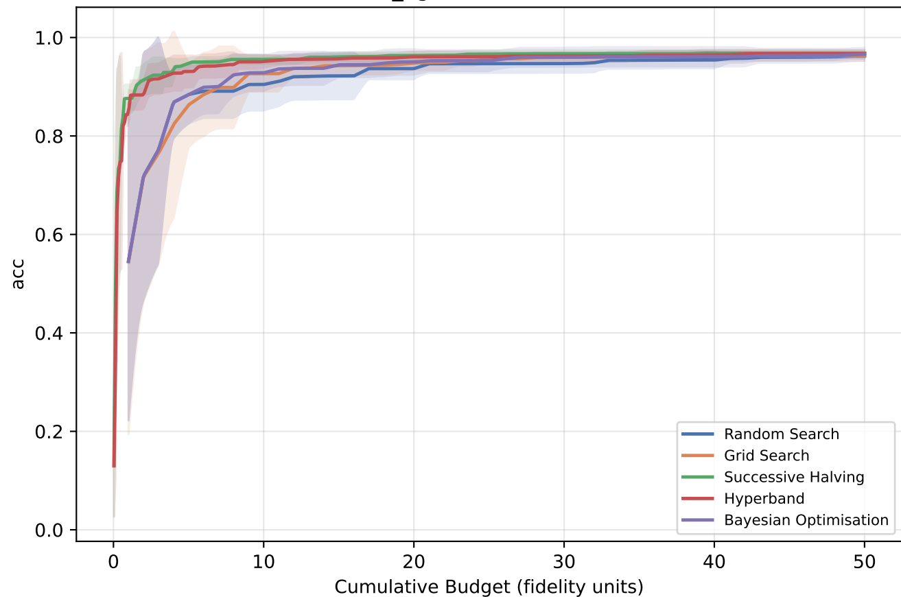
rbv2_xgboost (Dataset 16)
