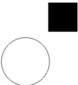
pred IoU=1.00
