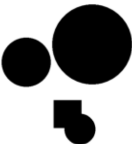
pred IoU=0.98
