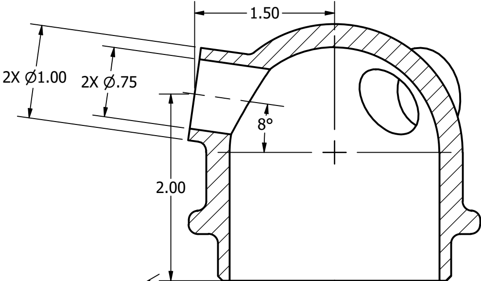
SECTION AB-AB SCALE 1 : 1
