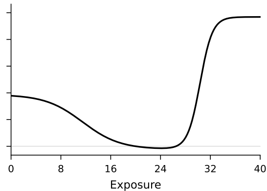
DGP 2
