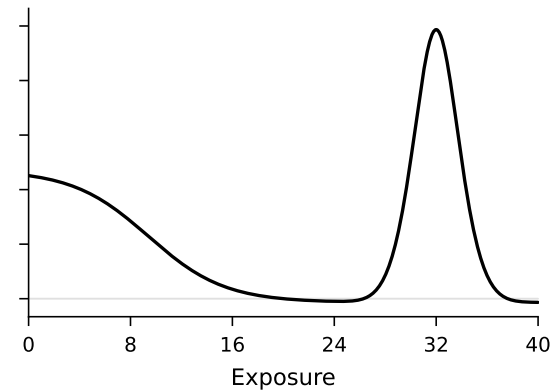
DGP 3
