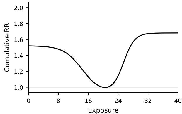
DGP 1
