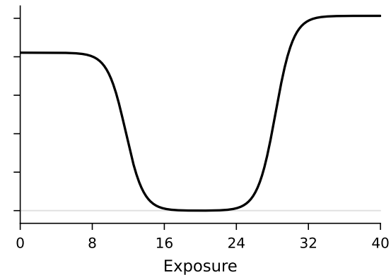
DGP 4
