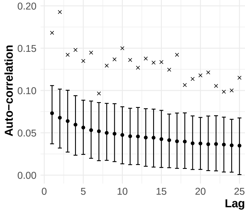
Neg. Bin. DLNM
