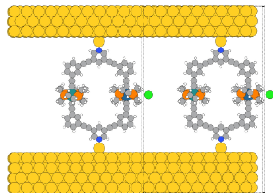
(a) Ru/Os(Cl)
