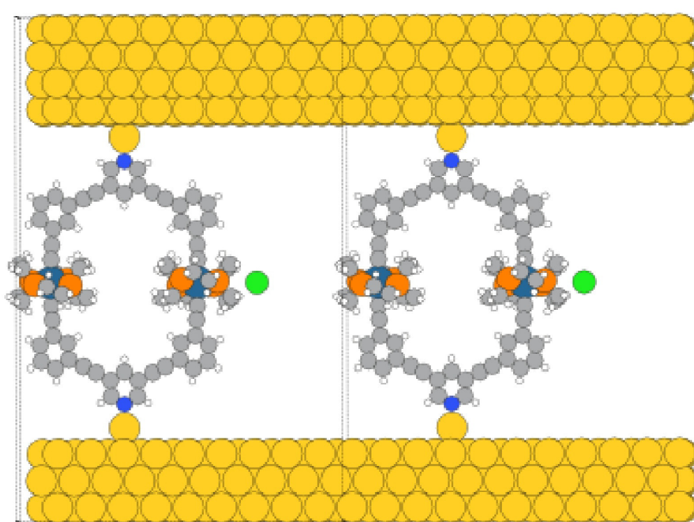
(b) Os/Os(Cl)
