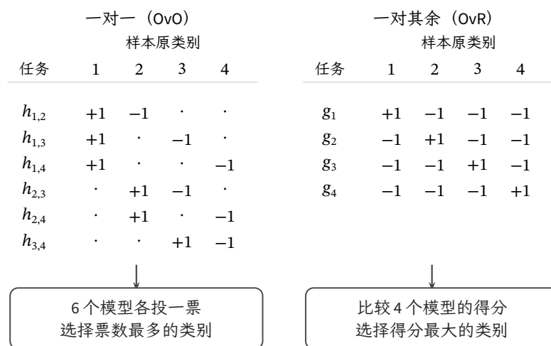
图 3.3 四分类任务中的两种二分类组合方式。各行对应一个待训练模型，各列对应样本的原类别；+1 和 -1 是为该任务重新编码的标签，点号表示该类样本不参与训练。一对一训练 6 个模型并汇总类别选票，一对其余训练 4 个模型并比较实值得分。图中给出训练与预测规则，不预设两种方法会产生相同的分类结果。
