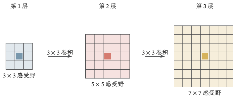
图 9.17 三个步长一、无空洞的 3 \times 3 卷积逐层扩大几何感受野。彩色方格表示一个高层位置在原输入上可能读取的范围，中心实色格只用于对齐位置；跨度依次为 3, 5, 7。图没有计入池化、跨位置归一化或边界填充造成的额外依赖。
