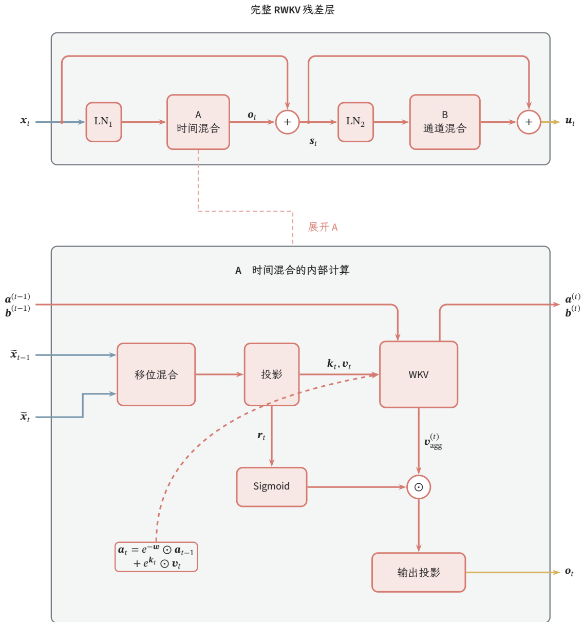
图 10.16 RWKV-4 的完整残差层与时间混合子模块。上方在 A、B 之前分别归一化，并在各子模块之后作残差相加，第一次相加得到 \mathbf{s}_t 。下方只展开 A，无箭头虚线表示对应关系； \tilde{\mathbf{x}}_t = \text{LN}_1(\mathbf{x}_t) 是归一化后的特征。红框给出未作数值重缩放时的简化递推，说明旧状态按 e^{-w} 衰减、当前键值按 e^{k_t} 写入；实际实现还维护分母状态。图中省略稳定化重缩放、移位缓存的保存箭头及 B 的内部计算。
