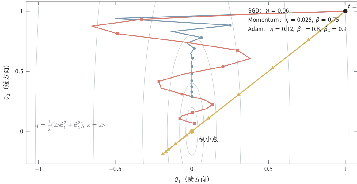
图 14.3 SGD、动量与 Adam 在同一病态二次目标上的前 20 步。目标为 q(\theta) = (25\theta_1^2 + \theta_2^2)/2 ，条件数 \kappa = 25 ，三者均从 (1, 1)^\top 出发并使用完整梯度；灰线为等高线，黄色点为唯一极小点。轨迹由正文定义的递推式直接计算，图例列出步长和矩系数。不同超参数会改变速度与振荡，不能据此推出某方法对一般非凸随机训练恒优。
