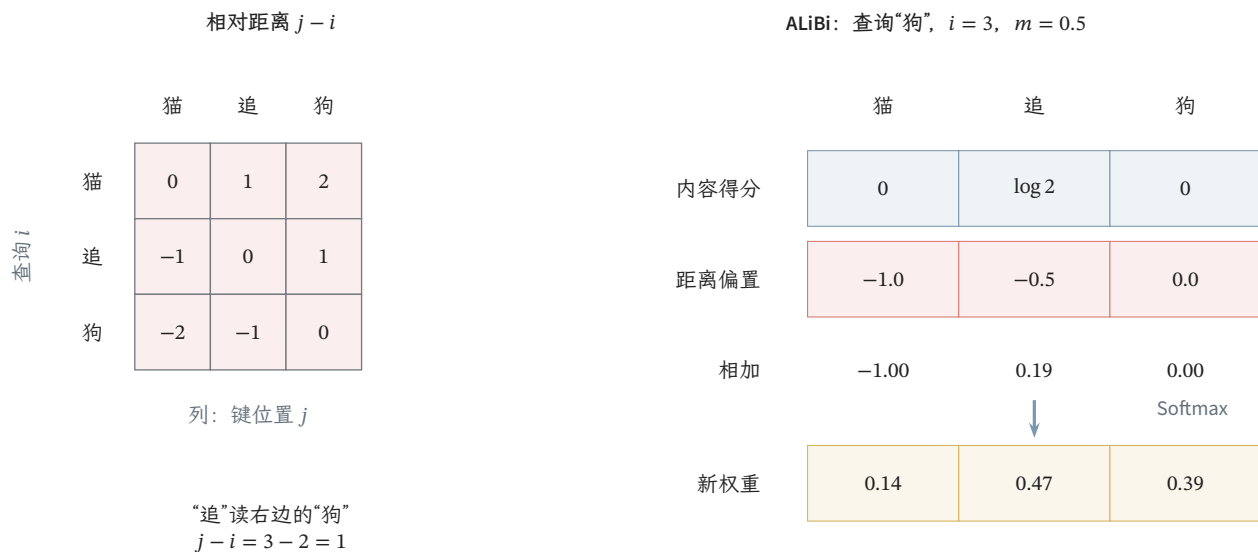
图 12.15 “猫/追/狗”的相对位置。左图行是查询位置 i 、列是键位置 j ，格内为 j - i ，正负号区分左右方向。右图取“狗”为查询、斜率 m = 0.5 ，演示 ALiBi 如何修正教学得分并重新归一化；显示数值保留两位小数，真实计算使用未舍入值。
