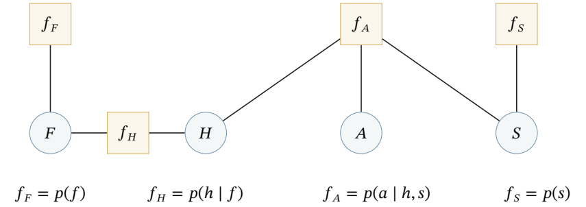
图 19.4 报警模型的因子图。圆形是随机变量，方形是四个局部条件或先验因子。 f_H 连接 F, H ， f_A 连接 H, A, S ；连接线表示函数输入关系，而不是有向生成边。
