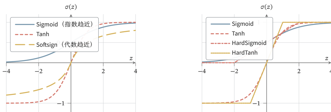
图 8.3 双侧饱和激活函数。左图比较 Logistic / Sigmoid、Tanh 与 Softsign；Softsign 采用长虚线，以便在黑白打印中仍能与 Sigmoid 区分，图例同时指出前者按代数速度、后者按指数速度趋近渐近值。右图将 HardSigmoid 和 HardTanh 与对应平滑函数比较。HardSigmoid 采用式(8.7)中的斜率 1/4 及截断点 \pm 2 。
