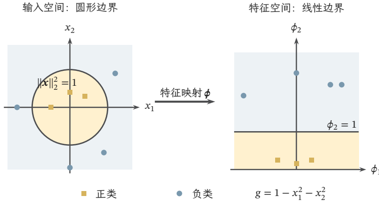
图 1.1 非线性边界在特征映射前后的对应，两个面板的坐标均无量纲。正类方点为 (-0.5, 0) 、 (0, 0.4) 、 (0.4, 0.3) ，负类圆点为 (-1.4, 0) 、 (0, -1.6) 、 (1.2, 0.9) 、 (0.9, -1.2) 。右图逐点使用 \phi_1 = x_1 、 \phi_2 = x_1^2 + x_2^2 ；水平线 \phi_2 = 1 对应左图半径为 1 的圆。数据与边界均为教学构造。
