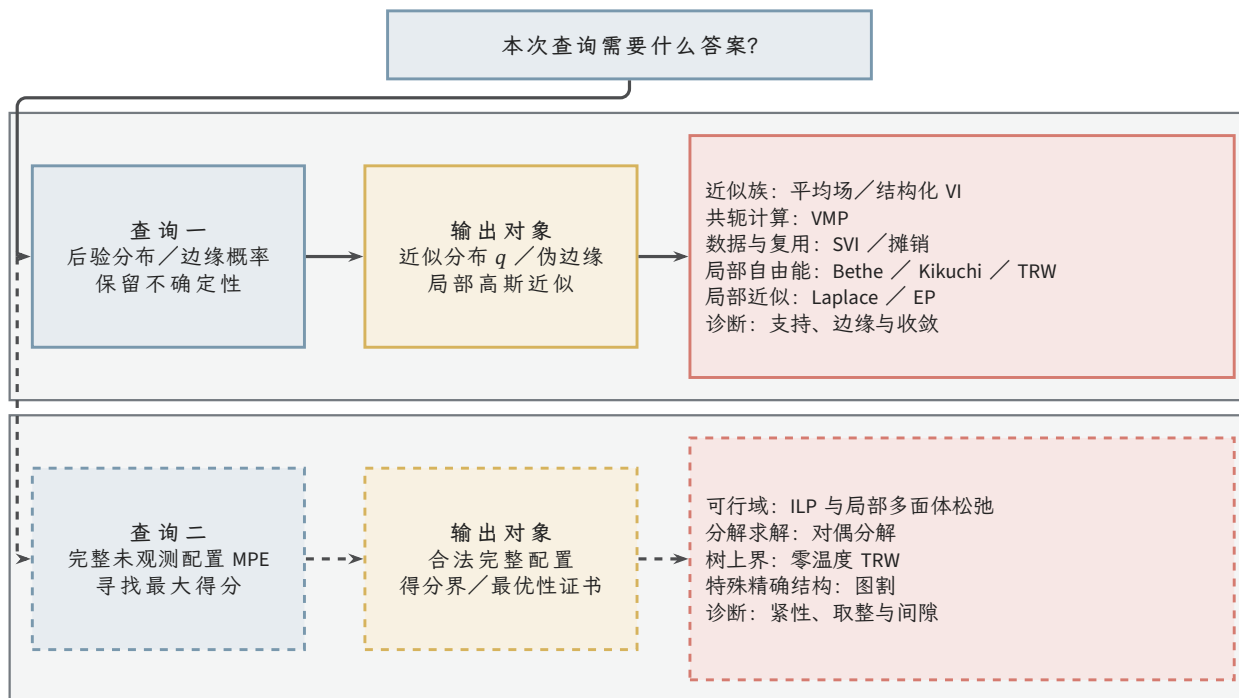
图 22.1 按查询选择阅读路线。上支保留后验或边缘不确定性，下支回答完整配置 MPE；图中的实线与虚线用于区分两支，不表示精确与近似。方法入口按所改变的对象分组，不是互斥算法清单。正温度 TRW 近似分布查询，零温度 TRW 提供 MPE 得分上界；含求和与最大化的边缘 MAP 不在本图范围内。
