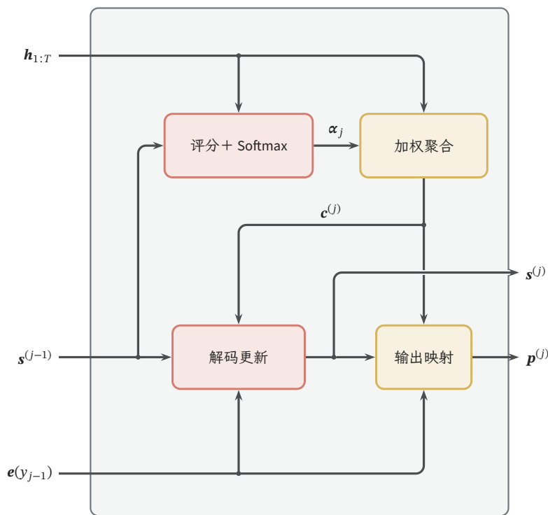
图 10.11 带注意力的一个解码步。左侧为保存的编码状态 h_{1:T} 、旧解码状态和此前目标的嵌入，右侧为新解码状态和输出概率。查询先用旧解码状态产生权重 \alpha_j = (\alpha_{j,1}, \dots, \alpha_{j,T}) ，上下文再进入更新与输出映射；输出映射还可读取目标嵌入。编码状态在各解码步重复读取，图中不重新执行编码器。
