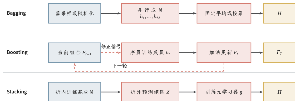
图 6.1 Bagging、Boosting 与 Stacking 的成员生成及组合关系。实线表示训练或预测的主路径，虚线表示由前一轮组合产生的修正信号。三类方法都输出组合预测，但成员间依赖与组合规则不同；图中流程为机制示意，不表示三者必须使用相同成员模型。
