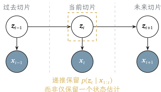
图 28.1 状态空间模型的有限展开。空心节点表示潜状态, 填色节点表示观测; 竖直虚线区分时间切片。消去过去后, 当前潜状态上的后验分布是继续预测所需的信息, 图中箭头表示生成依赖而不是推断只能进行的方向。
