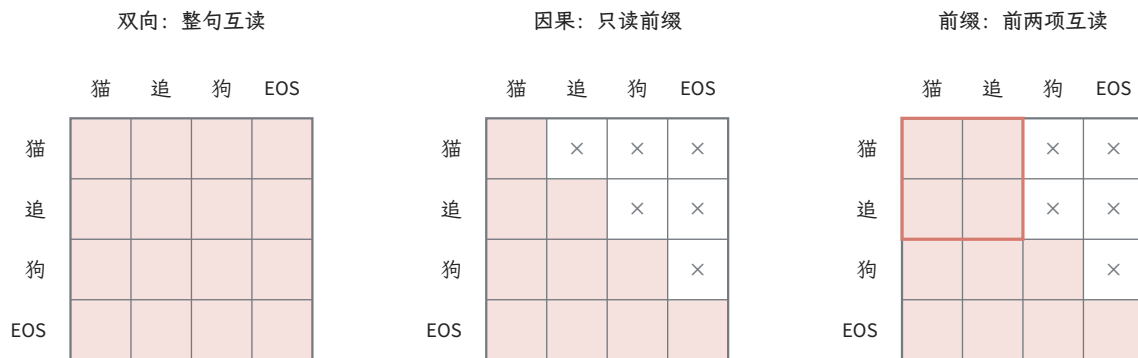
图 12.17 四个位置的读取范围。行表示查询位置 i ，列表示键位置 j ，着色格允许读取，带叉白格禁止读取。左为全部有效输入间的双向读取，中为 j \leq i 的因果读取，右为前两个位置构成条件前缀的读取：前缀内部双向，目标读取全部前缀与截至当前位置的目标输入。目标输入已移位，因此读取当前输入不等于读取当前待预测标签。
