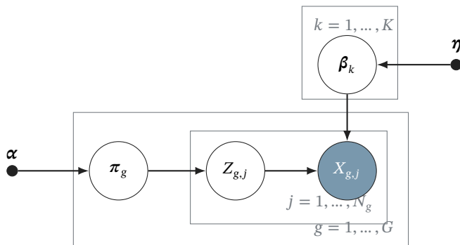
图 26.3 主题词分布也带先验的 LDA 板图。空心圆为随机潜在量，填色圆为观测词，实点为给定超参数。 G 个文档分别有主题比例 \pi_g ，每篇有 N_g 个主题分配和词； K 个主题词分布 \beta_k 在所有文档间共享。指向词的主题参数边表示按 Z_{g,j} 选择对应分布。
