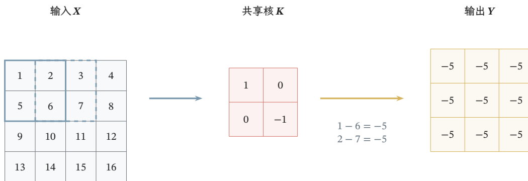
图 9.2 共享核在二维矩阵上滑动的教学例子。蓝色实线和虚线分别框出相邻的两个 2 \times 2 输入窗口，红色矩阵为不翻转的核，黄色矩阵为互相关输出。每个输出计算窗口左上数值减去右下数值，因此均为 -5；两个位置使用同一组权重。
