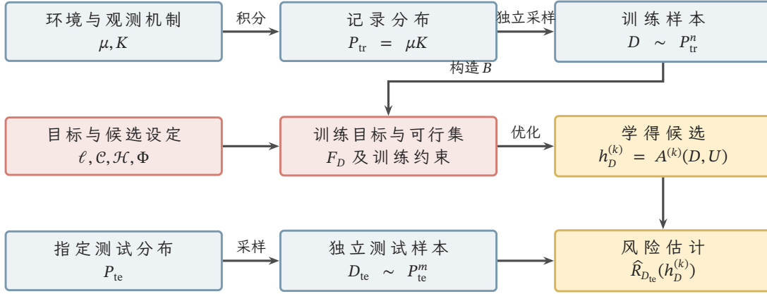
图 17.1 静态学习中的数据、目标与方法。蓝色节点表示数据对象，红色节点表示训练计算，黄色节点表示学得对象与评价结果。图中取独立采样 Q_n = P_{tr}^n ； P = \mu K 是分布运算， D \sim Q_n 是采样。目标构造 B 与优化规则共同组成学习映射 A 。独立测试样本只用于估计指定的评价风险。
