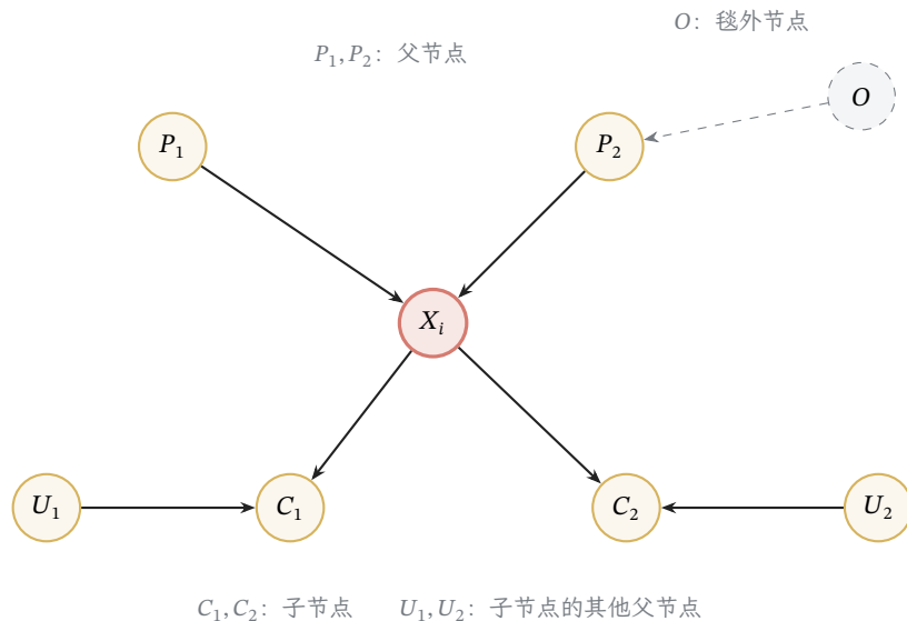
图 17.2 有向图中节点 X_i 的 Markov 毯。黄色节点构成 \text{mb}(i) : P_1, P_2 是父节点， C_1, C_2 是子节点， U_1, U_2 是子节点的其他父节点；虚线节点 O 位于毯外。
