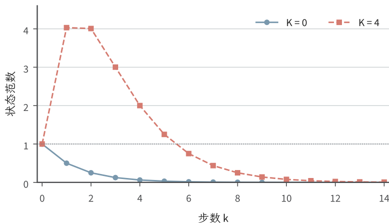
图 16.3 离散教学系统 A = \begin{bmatrix} 1/2 & K \\ 0 & 1/2 \end{bmatrix} 从 x_0 = (0, 1)^T 出发。蓝色圆点取 K = 0 ，红色方点取 K = 4 ；两者谱半径均为 1/2 。后者在前两步的欧氏范数约为 4.03、4.01，然后趋零。灰线标记初始范数 1，图中放大来自状态耦合，未加入输入或数值离散误差。
