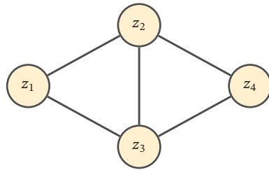
图 14.1 由第 2 章约束作用域导出的变量关系图。每条边表示两个变量共同出现在至少一个约束中；共享边 \{2, 3\} 是左右两个三角形的接口。边权、方向与关系的数值含义需要另行给出。
