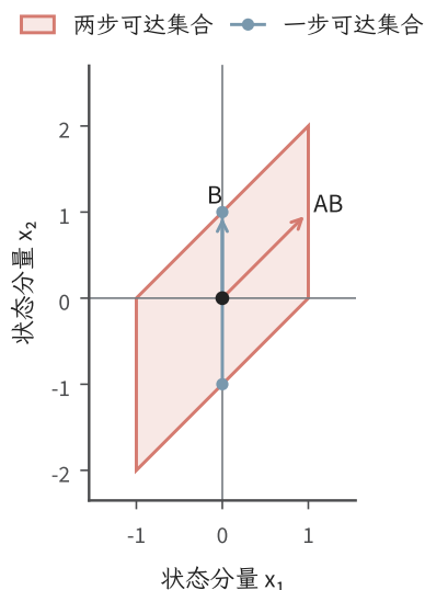
图 18.1 教学系统 A = \begin{bmatrix} 1 & 1 \\ 0 & 1 \end{bmatrix} 、 B = (0, 1)^T 与零初态。蓝色线段为 |u_0| \leq 1 时的一步可达集合, 红色区域为 |u_0|, |u_1| \leq 1 时的两步可达集合; 箭头标出 B 与 AB 。输入先改变第二个坐标, 经一次状态传播后获得新的方向。输入幅值界只服务于有限区域的绘图, 不属于定理 18.3 的无约束假设。
