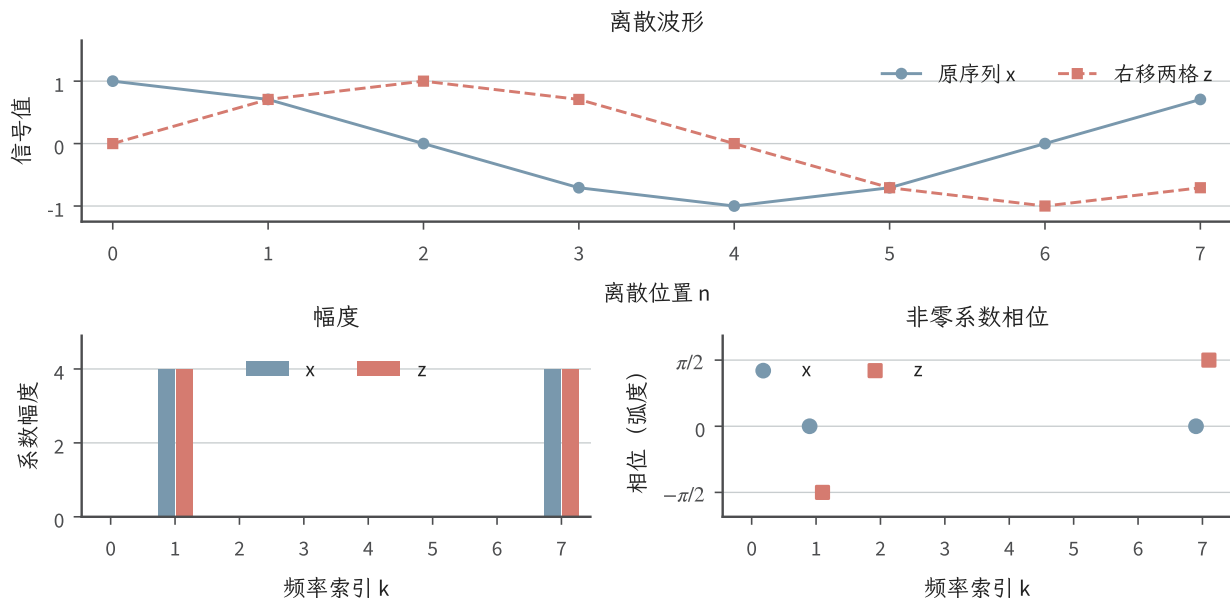
图 15.3 长度 8 的教学信号 x[t] = \cos(2\pi t/8) 与循环平移后的 z[t] = x[(t-2) \bmod 8] 。上图为两条离散波形，下图固定相同频率索引，分别比较 DFT 幅度与非零系数的主值相位。两者只有 k=1, 7 处幅度为 4，位移改变这两个系数的相位而不改变幅度。波形连线帮助观察顺序，不表示已经选定连续时间插值。
