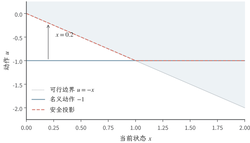
图 18.3 教学积分器 \dot{x} = u 、安全集合 x \geq 0 及 \alpha(h) = h 。灰色虚线是可行域边界 u = -x ，其上方阴影表示允许动作；蓝色实线为名义动作 u = -1 ，红色虚线为投影 u^* = \max\{-1, -x\} 。在 x = 0.2 处，原动作修正为 -0.2 。此图假设无额外执行器约束，不能用来判断有限输入范围下的联合可行性。
