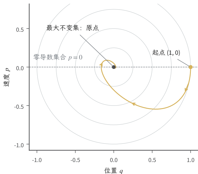
图 16.2 教学阻尼振子 \dot{q} = p 、 \dot{p} = -q - p 的精确轨迹，初态 (1, 0) 。黄色轨迹在 t = 0 至 12 间逐渐靠近原点，箭头表示时间前进；灰色虚线是零导数集合 p = 0 ，浅灰圆是 V = (q^2 + p^2)/2 的参考等值线。整条零导数直线并不不变，原点才是其中最大不变集。
