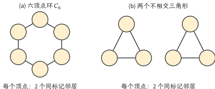
图 14.12 相同局部计数不保证相同整体结构。所有顶点从同一标记开始，每轮都看见两个同标记邻居，因此两张六顶点图的 1-WL 标记计数始终相同。左图只有一个连通分量，右图有两个；这证明该局部细化不能在这个例子中识别连通性的差异，而不是说连通性本身难以计算。浅黄填充只表示同标记，圆内不放唯一编号，以免改变例子的输入。
