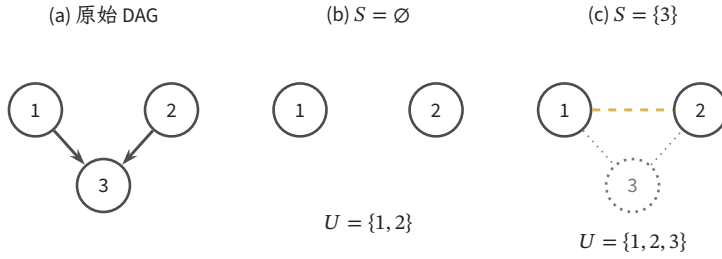
图 14.6 碰撞结构中的查询图取决于条件集。查询端点固定为 1, 2。空条件集的祖先道德图只有两个孤立顶点；给定 3 时，祖先集合 U 扩大，道德化加入黄虚线 1-2。右图灰色顶点及灰点线表示随后删除的条件顶点与关联边，黄虚线表示删除后仍保留的新增边。点线与虚线区分两种操作，灰度阅读也可辨认。
