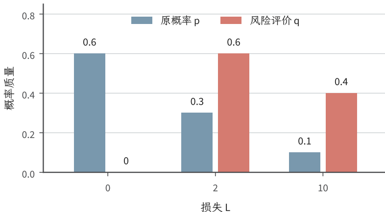
图 17.3 教学损失 0, 2, 10 的名义概率为 (0.6, 0.3, 0.1)。CVaR 0.75 对偶中的约束 q_i \leq 4p_i 与 \sum_i q_i = 1 给出最优重加权 (0, 0.6, 0.4), 其期望为 0.6 \times 2 + 0.4 \times 10 = 5.2 。蓝色为名义质量, 红色为对偶最优质量; 重加权只改变评价权重, 不表示真实损失的发生概率已经改变。
