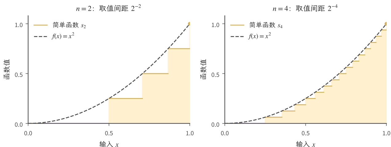
图 3.6 按取值分层的简单函数逼近。两图都使用式 (3.30) 的构造，分别取 n = 2 和 n = 4 ；本例中高度截断不起作用。黄色阶梯下的面积是有限加权和，目标曲线下的面积为 1/3 。两图共用坐标尺度。
