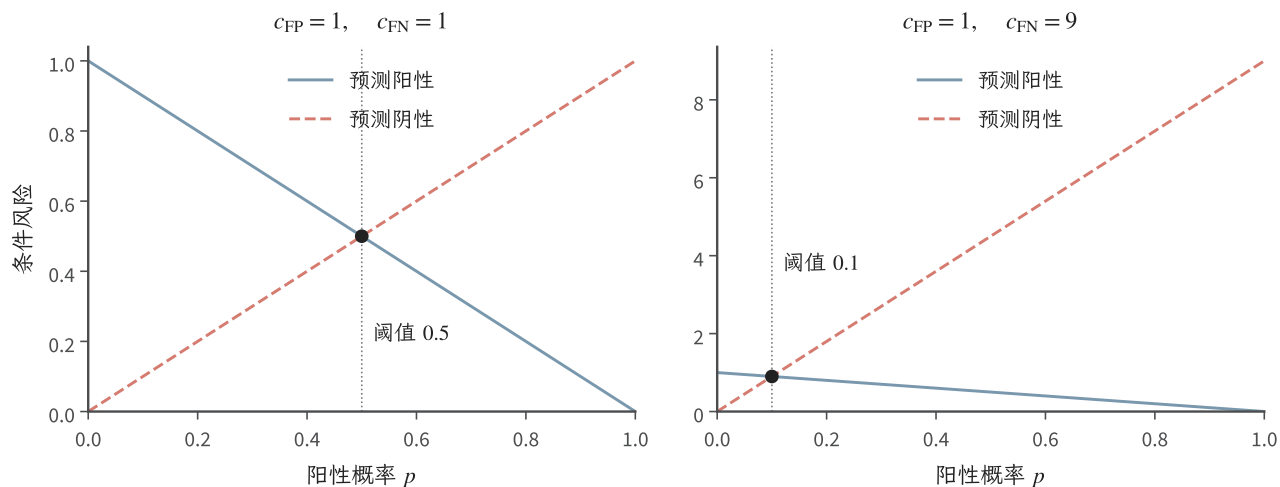
图 17.1 二分类中的条件风险。蓝色实线为预测阳性的风险 c_{FP}(1-p) ，红色虚线为预测阴性的风险 c_{FN}p 。左图两种错误成本均为 1，阈值为 0.5；右图仅将漏诊成本增至 9，阈值降为 0.1。两图使用相同横轴，纵轴明确显示各自的损失范围；教学成本用于说明损失设定如何改变行动。
