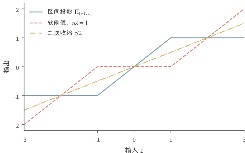
图 4.6 同一输入 z 的三种邻近映射。投影采用 C = [-1, 1] ；软阈值与二次收缩均取 \eta\lambda = 1 ，分别输出 \text{sign}(z)(|z| - 1)_+ 和 z/2 。横轴刻度标出阈值位置，曲线由完整分段解析式生成。
