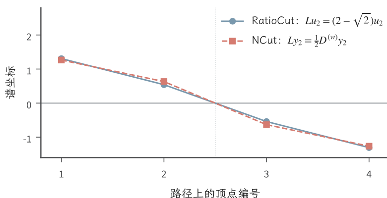
图 14.10 单位边权路径 1-2-3-4 的两个精确谱方向。蓝实线为组合拉普拉斯的第二特征向量, 红虚线为度加权广义特征向量; 点形同时区分两者。为比较形状, 图中两向量均按欧氏范数 2 缩放, 此显示约定不改变各自的特征方程, 也不替代 NCut 推导中的度加权范数。横轴只有四个顶点, 连线仅引导阅读, 竖虚线标出零阈值切分的位置。
