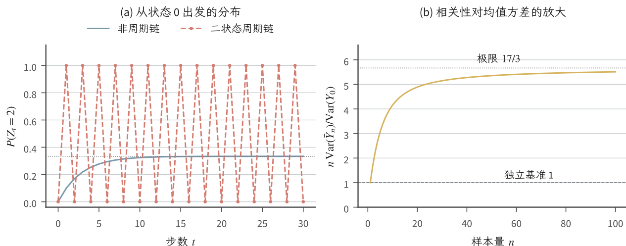
图 10.1 两状态链的解析式教学图。左图蓝线使用例 10.8 的转移矩阵，从 Z_0 = 0 出发绘制 \mathbb{P}(Z_t = 2) = (1 - 0.7^t)/3 ；红线使用确定交替的转移矩阵。右图使用平稳初态和 \rho_k = 0.7^k ，绘制 1 + 2 \sum_{k=1}^{n-1} (1 - k/n) \rho_k ，其极限为 17/3 ，独立观测基准为 1。
