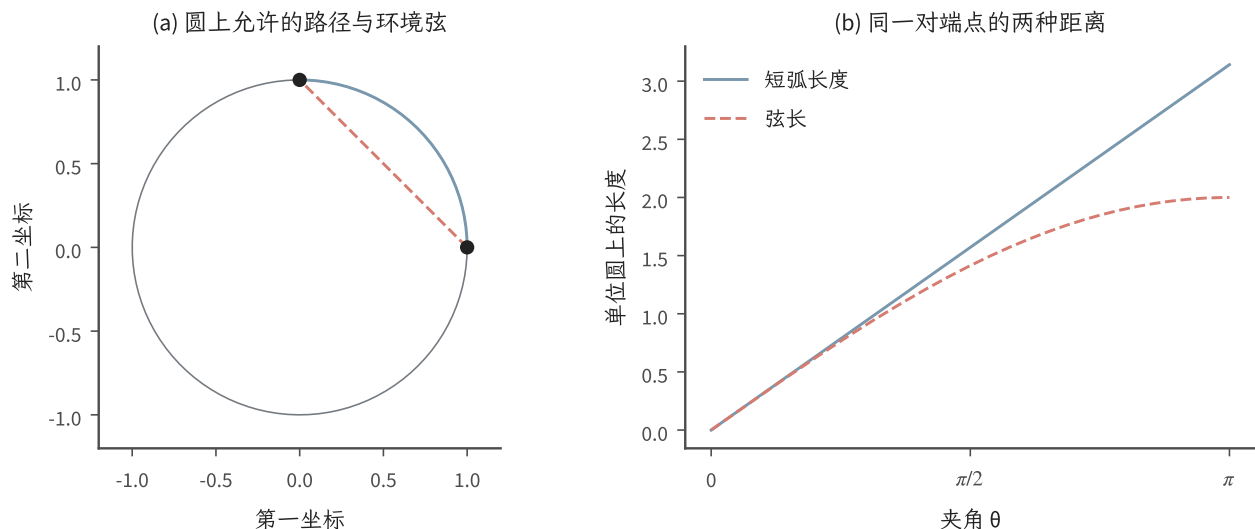
图 8.2 完整单位圆上的短弧与环境弦长。左图取夹角 \pi/2 ，蓝线沿圆移动，红虚线穿过圆内；右图比较全部 \theta \in [0, \pi] 的两种长度。弦在环境平面中可行，在圆上却不是允许路径。图为解析教学示例。
