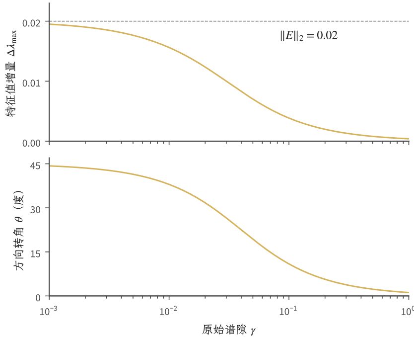
图 7.4 同一对称扰动下的特征值与方向变化。对 \mathbf{A}_r 加入 \mathbf{E}_{0.02} ，上图绘制最大特征值的增量 \sqrt{(\gamma/2)^2 + 0.02^2} - \gamma/2 ，灰虚线为扰动范数 0.02；下图绘制转角 \theta = \frac{1}{2} \arctan(0.04/\gamma) 。两图横轴相同，角度用度表示；数值来自二阶特征方程的解析解。
