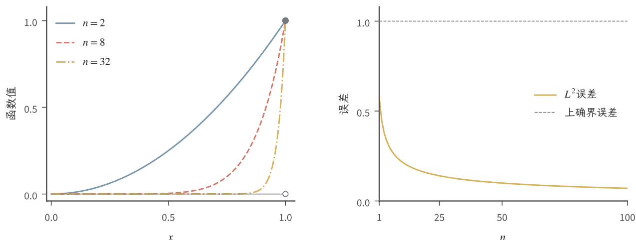
图 3.7 x^n 在 [0, 1] 上的两种整体尺度。左图蓝、红、黄线分别取 n = 2, 8, 32 ；灰线与端点标记表示逐点极限，它在 x < 1 处为零、在 x = 1 处为 1。右图黄色曲线为精确的 L^2 误差 (2n+1)^{-1/2} ，灰虚线为始终等于 1 的普通上确界误差；单点 x = 1 的修改不影响积分。图为解析教学示例。
