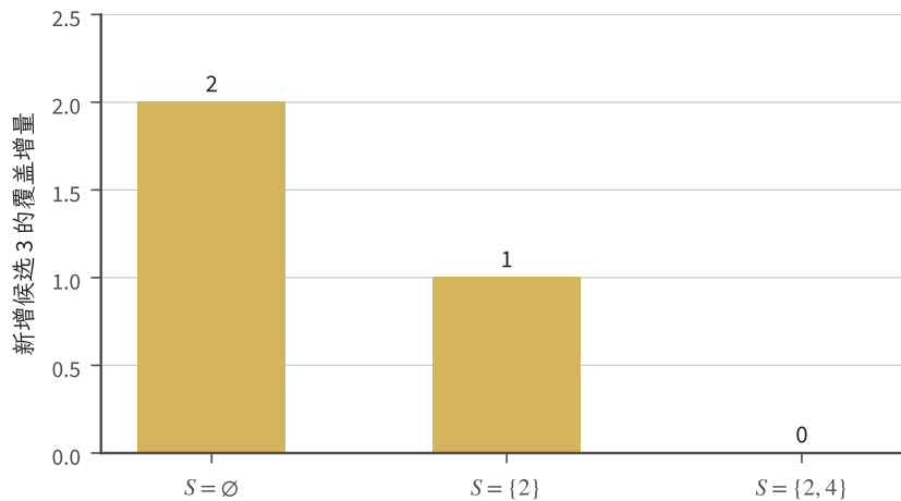
图 2.6 覆盖函数的有限教学构造。使用式 (2.19) 中的 Q_2, Q_3, Q_4 , 向 \emptyset \subset \{2\} \subset \{2, 4\} 分别加入候选 3, 覆盖增量为 2, 1, 0。柱高从零基线起画; 图中只展示一个具体递减链, 完整次模性仍由集合差证明。
