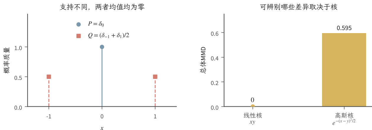
图 12.2 同均值分布在不同核下的 MMD (解析式教学图)。左图蓝圆点为 P = \delta_0 , 红方点为 Q = (\delta_{-1} + \delta_1)/2 ; 两者均值均为零。右图使用精确总体期望, 线性核的 MMD 为零, 高斯核的 MMD 约为 0.595。没有进行有限样本估计。
