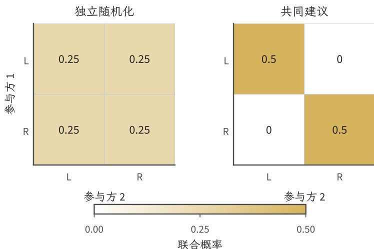
图 19.2 二行动协调博弈的两个教学联合分布，共用 0 至 0.5 的概率色阶。行为参与者 1 的行动，列为参与者 2 的行动。左图为独立均匀策略，四格质量均为 0.25；右图只推荐 (L, L) 与 (R, R) ，各占 0.5。两者边缘概率均为 (0.5, 0.5) ，但每人期望收益分别为 1 和 2；相关分布并非边缘分布的乘积。
