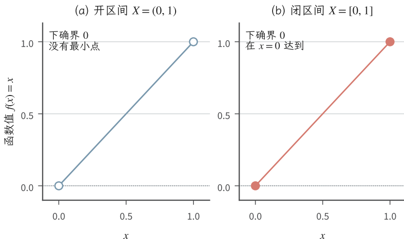
图 1.1 同一函数 f(x) = x 的边界对照。左图定义域为 (0, 1) ，空心端点不属于图像，函数值可任意接近 0，却不能取到；右图定义域为 [0, 1] ，实心端点 (0, 0) 达到下确界。两图的下确界相同，最小点是否存在取决于可行端点是否保留。图为解决析教学示例。
