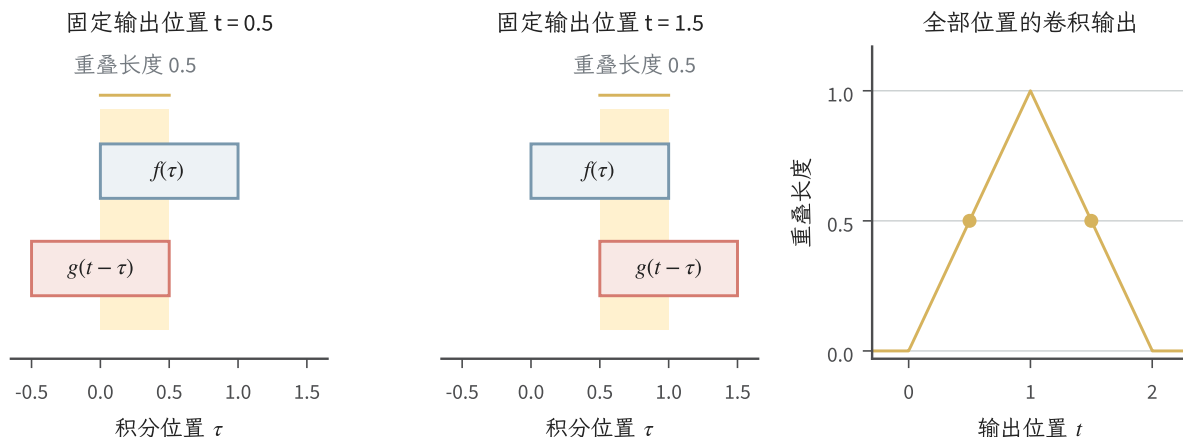
图 15.1 教学函数 f = g = \mathbb{I}_{[0,1]} 的连续卷积。左两图分别固定 t = 0.5 与 t = 1.5 ：蓝色区间是 f(\tau) 的支撑，红色区间是 g(t - \tau) 的支撑，黄色重叠的长度都为 0.5。右图将所有输出位置的重叠长度画成 (f * g)(t) ，在 t = 1 处达到 1。左两图的横轴 \tau 与右图的横轴 t 承担不同角色。
