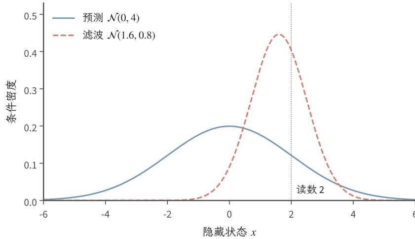
图 16.4 标量 Kalman 更新的教学例。蓝色曲线为预测 \mathcal{N}(0, 4) ，红色曲线为观察 y = 2 后得到的 \mathcal{N}(1.6, 0.8) ，观测噪声方差为 1，虚线标记实际读数。这里 \mathcal{N} 的第二个参数是方差；比较的是同一隐藏状态在新观测前后的条件密度。
