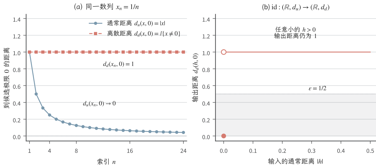
图 3.2 数值相同, 距离不同。(a) 数列 x_n = 1/n 到 0 的通常距离趋于零, 离散距离却恒为 1, 所以收敛要连同度量说明。(b) 恒等映射从通常度量空间映入离散度量空间时, 任意非零且很小的输入位移仍对应输出距离 1, 不能进入 \varepsilon = 1/2 的输出邻域, 故它在 0 处不连续。图为解析教学示例。
