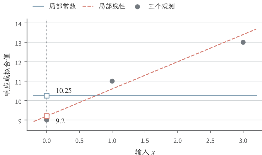
图 11.3 边界处的局部常数与局部线性拟合（教学数据图）。观测为 (0, 9), (1, 11), (3, 13) ，权重为 1, 0.75, 0.25 。蓝实线为加权常数 10.25 ，红虚线为 9.2 + 1.4x ，边界 x_0 = 0 处分别预测 10.25 和 9.2 。
