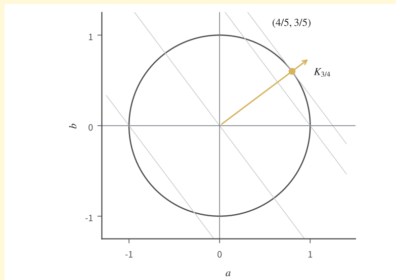
图 5.3 仿射 RKHS 中读取 f(3/4) = a + 3b/4 。灰圆表示 a^2 + b^2 \leq 1 , 黄箭头是核截面 K_{3/4} 对应的系数 (1, 3/4) ; 灰平行线为相同点值。黄圆点 (4/5, 3/5) 达到单位范数球上的最大点值 5/4 。这里坐标是函数系数, 不是输入位置。图为解析教学示例。
