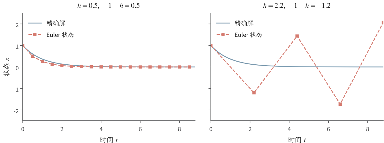
图 16.1 教学方程 \dot{x} = -x 、 x(0) = 1 的精确解与 Euler 近似。蓝色实线是同一精确解，红色方点是各自步长下的数值状态；左图 h = 0.5 衰减，右图 h = 2.2 交替增长。两图使用相同坐标范围，连线仅显示相邻数值状态，不能解释为 Euler 方法在步间的精确解。
