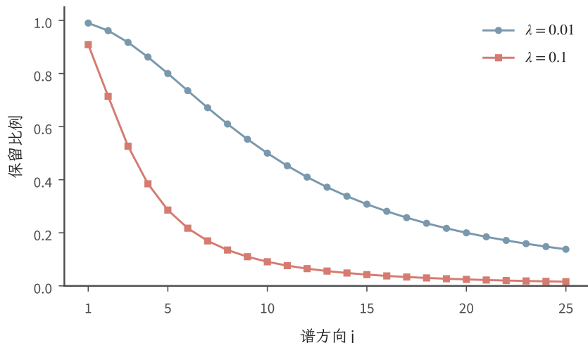
图 5.4 教学谱 \mu_j = j^{-2} 上的收缩比例 \mu_j/(\mu_j + \lambda) 。蓝、红线使用 \lambda = 0.01 和 0.1 ，点标出前 25 个方向；增大正则化后更多方向被抑制。有效维度的定义仍对全部谱方向求和。
