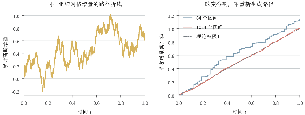
图 16.5 以固定随机种子构造的高斯增量教学例。左图由 4096 个独立增量 \Delta W_i \sim \mathcal{N}(0, 1/4096) 累计成路径折线；右图将同一组增量分别合并为 64 和 1024 个时间区间，再累计各区间增量的平方。蓝、红阶梯线使用不同分割，灰色参考线为理论二次变差 t 。这里只绘制有限网格，不把某一条折线作为连续布朗路径或收敛证明。
