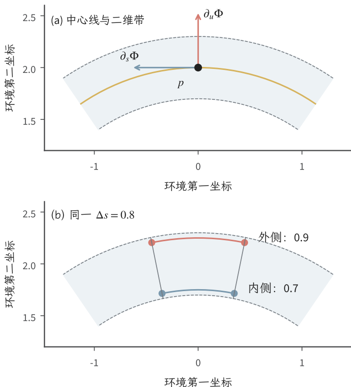
图 8.1 弯曲带的自由度与坐标尺度。取 R = 2 、 w = 0.3 。上图显示二维开带、中心线上的点 p 及两个参数方向 \partial_s \Phi 、 \partial_u \Phi , 箭头仅标方向; 仅把中心线作为对象时, 径向方向不属于其切空间。下图取 u = -0.25 与 u = 0.25 , 同一坐标增量 \Delta s = 0.8 对应弧长 0.7 与 0.9。灰虚线表示不纳入开带的边界, 两图等比例绘制, 均为解析教学示例。
