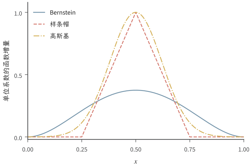
图 5.5 单个系数改变对函数的影响。蓝线为 6x^2(1-x)^2 ，即四阶 Bernstein 多项式的中心基；红线为中心 1/2 、相邻结点 1/4, 3/4 的线性样条帽；黄线为中心 1/2 、宽度 0.12 的高斯基。系数增量均为 1，不另行缩放峰高；图比较作用范围，未比较三种方法的最优逼近误差。
