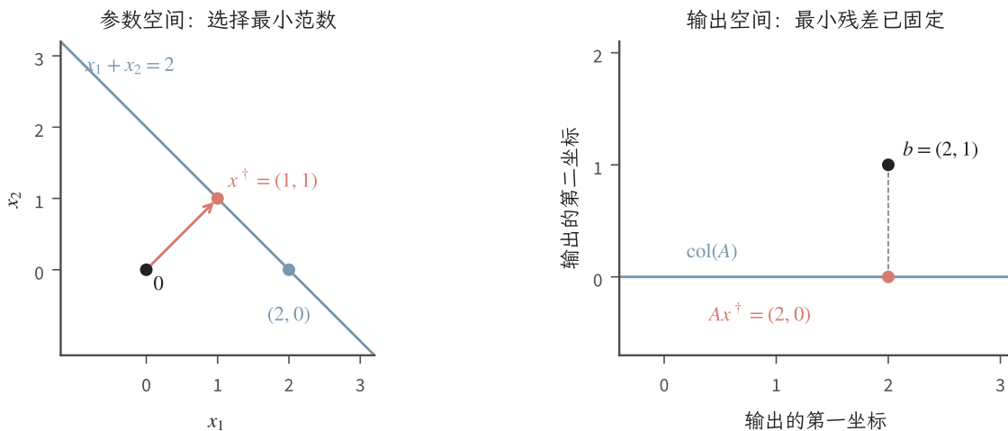
图 7.2 同一秩亏系统中的输出投影与参数选择。取 \mathbf{A} = \begin{bmatrix} 1 & 1 \\ 0 & 0 \end{bmatrix} 、 \mathbf{b} = (2, 1)^T 。右侧的蓝线是可达输出，红点 (2, 0)^T 使残差最小；左侧的蓝线 x_1 + x_2 = 2 是全部最小二乘参数，红点 \mathbf{x}^\dagger = (1, 1)^T 进一步使参数范数最小。两图表示不同空间，各自按比例绘制，均为解析教学构造。
