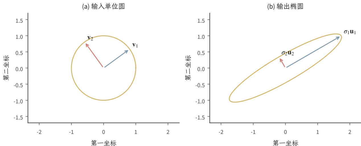
图 7.1 矩阵 \mathbf{A} = \mathbf{R}(\pi/6) \text{diag}(2, 0.4) \mathbf{R}(\pi/5)^\top 将单位圆变为椭圆。蓝、红箭头分别标出两个右奇异方向及其像 \sigma_i \mathbf{u}_i ；奇异值控制伸缩，左右正交矩阵改变方向。两图使用相同坐标比例，图为教学构造。
