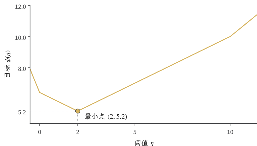
图 17.2 教学损失分布 P(L = 0) = 0.6 、 P(L = 2) = 0.3 、 P(L = 10) = 0.1 在 \alpha = 0.75 下的阈值目标 \phi(\eta) = \eta + 4\mathbb{E}[(L - \eta)_+] 。暖黄色折线的最小点为 (2, 5.2); 阈值 2 是 VaR, 最小目标值 5.2 是 CVaR。二者位于不同坐标轴, 不能把“最优阈值”当作“尾部平均损失”。
