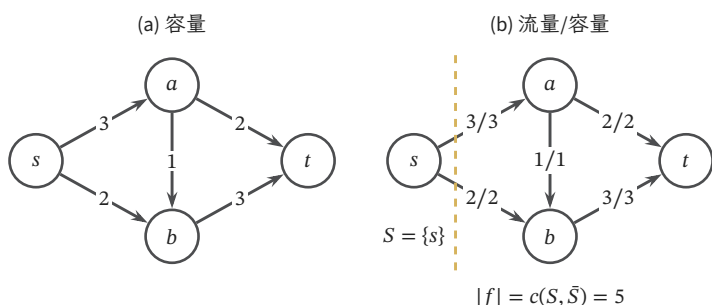
图 14.7 可行流与同值割共同给出最优性证书。左图标容量, 右图标流量/容量, 右侧每个内部顶点均满足流守恒。黄虚线划出 S = \{s\} , 跨出该集合的两条弧容量和为 3 + 2 = 5 , 等于已实现的流值。图中的有向弧都是原网络弧, 残量反向弧未画出。
