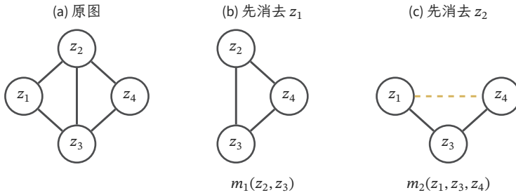
图 14.3 同一图两种首步消元。消去 z_1 时，接口 \{2, 3\} 已有边；消去 z_2 时，接口 \{1, 3, 4\} 必须补成团，黄虚线是新增填充边 \{1, 4\} 。下方列出新消息的自变量；在二值稠密表中，两者分别有 4 和 8 个条目。图记录可能的函数依赖范围，特殊因子还可能进一步分解。
