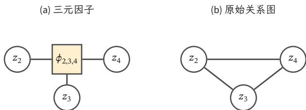
图 14.2 三元因子与原始关系图的区别。左侧方框代表一个依赖 z_2, z_3, z_4 的函数, 连线表示变量属于其作用域; 右侧只保留共同出现关系。右侧三条边不构成把该函数拆成三个二元函数的等价变换。
