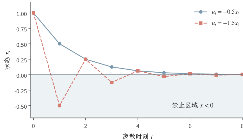
图 18.2 教学系统 x_{t+1} = x_t + u_t 从 x_0 = 1 出发。蓝色圆点采用 u_t = -0.5x_t ，保持 x_t \geq 0 ；红色方点采用 u_t = -1.5x_t ，第一步越过边界后交替衰减。两条轨迹都渐近稳定，只有前者保持安全集合 [0, \infty) 。灰色区域表示禁止的负半轴。
