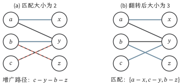
图 14.8 二部匹配的增广。顶点组为 U = \{a, b, c\} 、 W = \{x, y, z\} ，蓝实线是当前匹配，左图红虚线是增广路径中的未匹配边，灰实线是其余候选边。翻转路径 c - y - b - z 上的选边状态后，保留 a - x ，得到三条互不共享端点的边。无向连线表示候选配对，不表示因果或时间方向。
