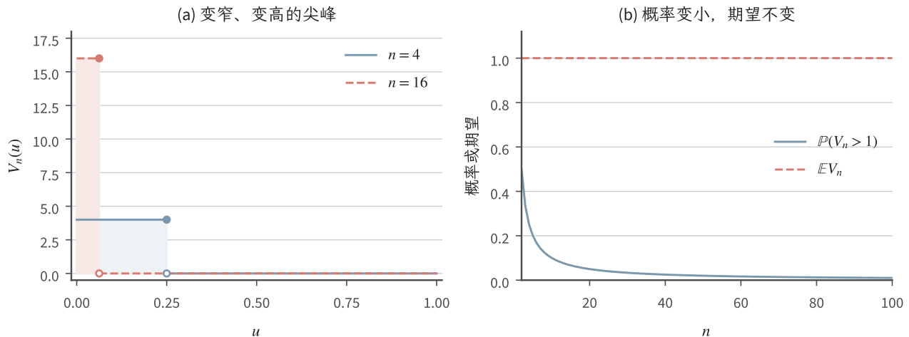
图 9.3 小概率尖峰与期望质量（解析式教学图）。左图为 V_n(u) = n\mathbb{I}\{u \leq 1/n\} 在 n = 4, 16 时的取值，均以面积 1 贡献期望；右图对 n \geq 2 显示 \mathbb{P}(V_n > 1) = 1/n 趋于零，而 \mathbb{E}V_n = 1 不变。基础变量为 U \sim \text{Unif}(0, 1) 。
