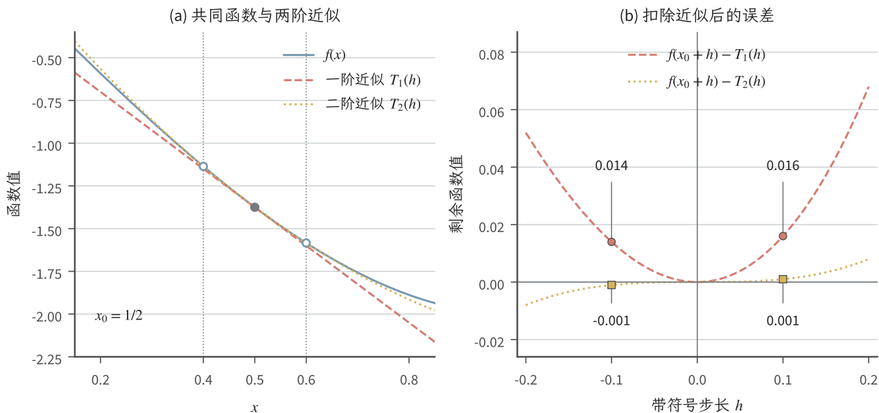
图 3.4 统一函数 f(x) = x^3 - 3x 在 x_0 = 1/2 处的两阶近似，记 h = x - x_0 。(a) 蓝线为真函数，红虚线为切线近似 T_1 = f(x_0) + f'(x_0)h ，黄点线加入二次项 f''(x_0)h^2/2 ，得到 T_2 。(b) 扣除各近似后的带符号余项分别为 3h^2/2 + h^3 与 h^3 ，标出 h = \pm 0.1 的精确结果。一阶导数确定切线，二阶导数补充局部曲率；余项的正负表示真值位于近似值的哪一侧。图为解析教学示例。
