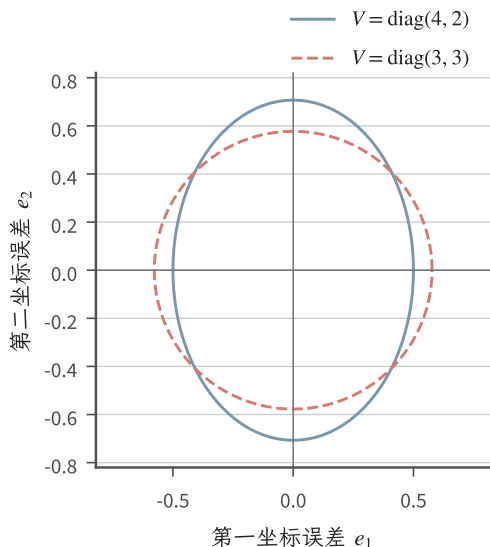
图 10.2 二维设计的归一化误差几何(解析式教学图)。蓝实线为 \mathbf{e}^T \text{diag}(4, 2)\mathbf{e} = 1 , 红虚线为 \mathbf{e}^T \text{diag}(3, 3)\mathbf{e} = 1 。它们不是已经具有相同覆盖概率的数值置信区间; 真实置信半径由式 (10.21) 另行确定。
