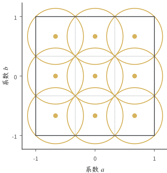
图 5.7 仿射函数族的有限覆盖。方形表示 a, b \in [-1, 1] ，九个实心点是类内代表，圆的半径为 \sqrt{2}/3 。每个小方格都被对应格心的闭球覆盖；圆的重叠与越出方形的部分均不影响覆盖要求。
