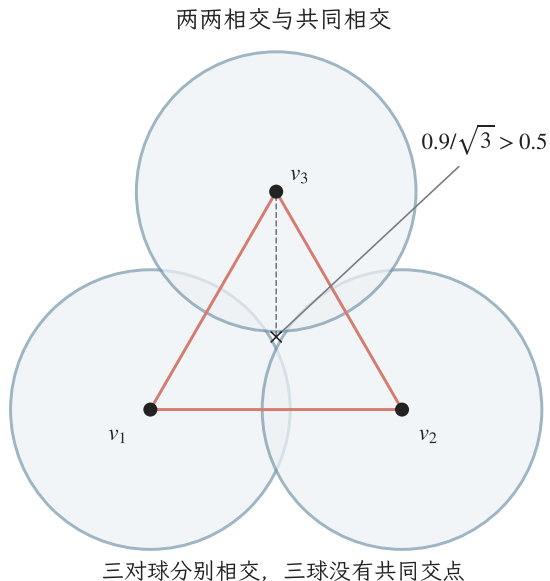
图 8.3 两两距离不能替代共同交集。正三角形边长为 0.9，阈值 \varepsilon = 1 ，每个蓝色开球的半径为 0.5。红色三条边均符合两种复形的连边条件；Čech 构造不纳入二维面，Rips 构造纳入二维面。中心叉号到三顶点的距离均为 0.9/\sqrt{3} > 0.5 ，它给出最小覆盖半径，说明三球没有共同交点。圆周仅标出不属于开球的边界；图为解析教学构造。
