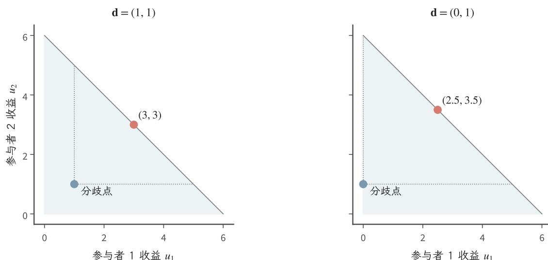
图 19.3 两方协商的教学可行域 u_1, u_2 \geq 0, u_1 + u_2 \leq 6 ，两图坐标一致。蓝点为分歧收益，红点为相对该分歧点的 Nash 乘积最优解。左图 \mathbf{d} = (1, 1) 得到 (3, 3) ，右图 \mathbf{d} = (0, 1) 得到 (2.5, 3.5) ；灰色虚线给出个体可接受的下界。可行总收益没有变化，变化的是退出时可得到的收益。
