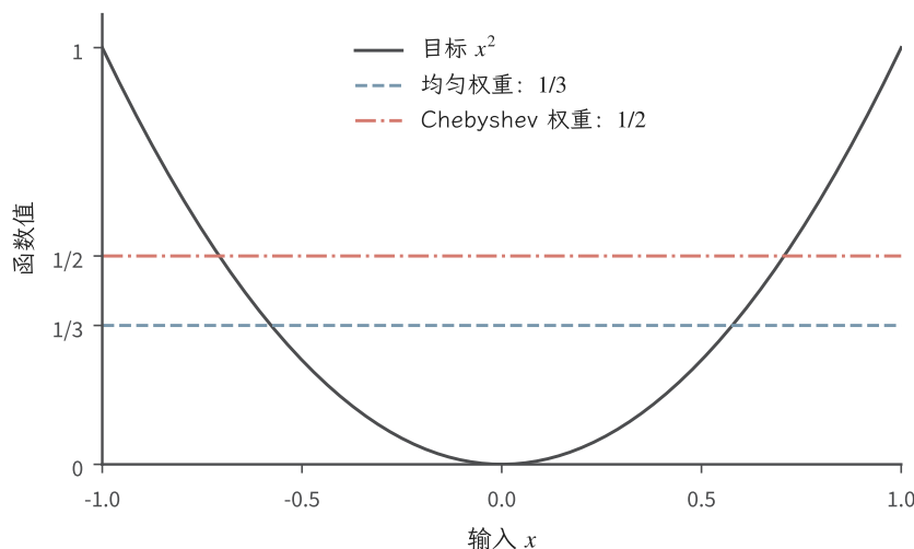
图 5.2 对 x^2 使用同一候选空间 \text{span}\{1, x\} ，均匀权重的最佳常数为 1/3 ，Chebyshev 权重的最佳常数为 1/2 。目标、区间和候选空间保持相同，只改变误差积分的权重。曲线由解析式生成。
