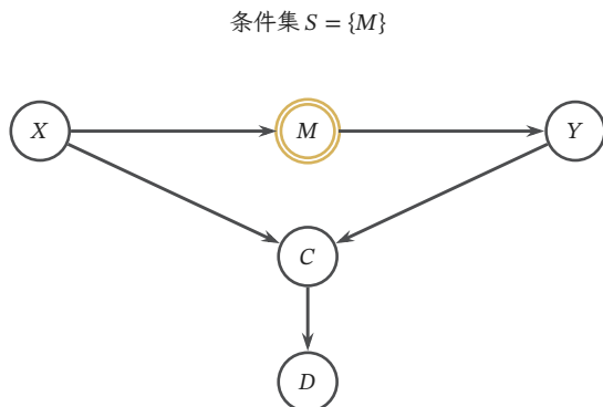
图 13.2 多条路径下的 d-分离。双边框节点 M 属于条件集，因而上方链式路径关闭；碰撞点 C 及其后代 D 均未给定，所以下方路径也关闭。若把 C 或 D 加入条件集，下方路径会重新打开。
