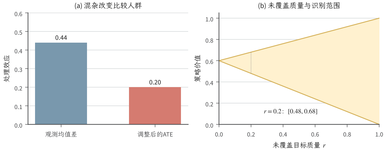
图 13.3 两个独立的因果教学构造。左图复用混杂算例，比较观测均值差 0.44 与调整后的 ATE 0.20。右图假定结果范围为 [0, 1] 、已覆盖部分平均收益为 0.6，绘制式 (13.23) 的范围 [0.6(1 - r), 0.6(1 - r) + r] 。阴影是总体识别范围，不是抽样置信带；两面板也不表示同一数据集。
