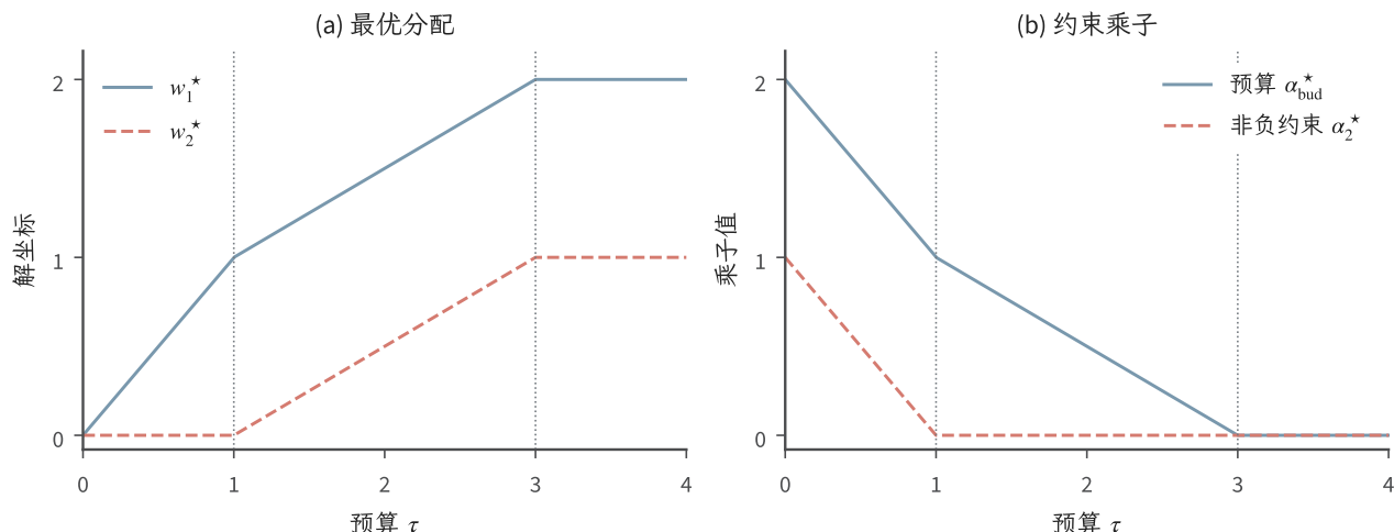
图 4.2 例 4.18 的解析解。左图为两个最优分配坐标，右图为预算乘子与第二个非负约束的乘子。竖参考线标出 \tau = 1, 3 ；在切换点约束可以取等号而乘子为零，说明活跃性与正价格并不等价。
