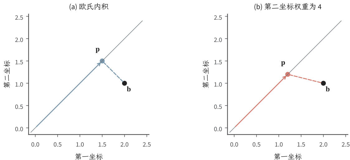
图 6.2 例 6.7 的两个最近点。灰直线是同一个子空间, 黑点是同一目标向量, 实箭头指向投影, 虚线连接残差。右图中的欧氏角度不必为直角, 正交性由加权内积判断。两图坐标比例相同。
