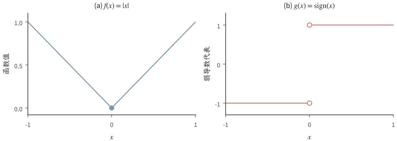
图 5.6 f(x) = |x| 与其一阶弱导数 g(x) = \text{sign}(x) 。左图原点为连续尖点; 右图两段分别为 -1 与 1 , 空心端点表示经典导数在原点未定义。
