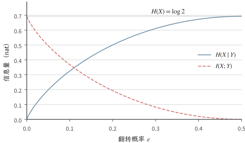
图 12.1 公平二元输入通过独立翻转通道后的信息分配（解析式教学图）。蓝实线为剩余条件熵 H(X|Y) = H_b(\epsilon) ，红虚线为互信息 I(X;Y) = \log 2 - H_b(\epsilon) ，对数取自然底。输入熵 H(X) = \log 2 保持不变。
