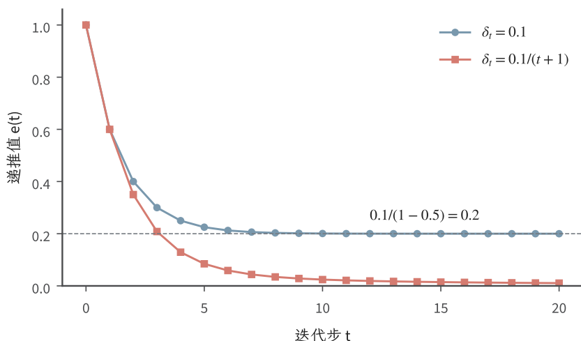
图 3.1 相同初值与收缩系数下的两种递推。蓝线使用持续扰动，红线使用衰减扰动；每个点都是整数步上的精确递推值，灰虚线是持续扰动留下的极限 0.2。图为教学构造。
