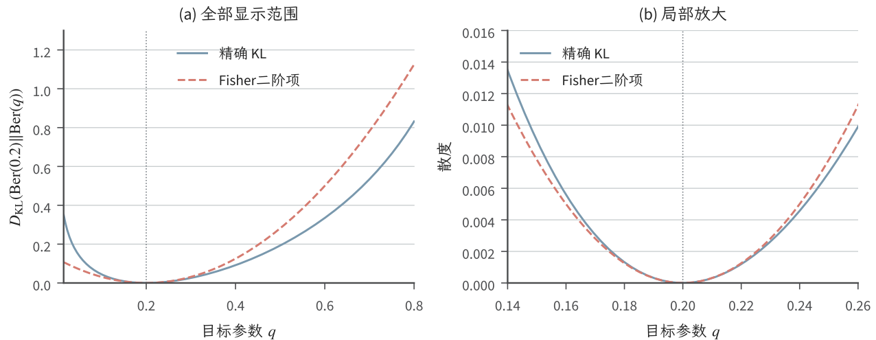
图 12.4 Bernoulli 族在 p = 0.2 处的 Fisher 局部近似（解析式教学图）。蓝实线为 D_{\text{KL}}(P_{0.2}||P_q) ，红虚线为 (q - 0.2)^2/[2(0.2)(0.8)] ；右图放大邻域，显示二阶近似只约束小位移。图中始终满足 0 < q < 1 。
