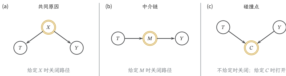
图 13.1 共同原因、中介与碰撞点的局部路径。双边框节点表示已加入条件集，因而图形不只依赖颜色传达条件化。面板 (a)、(b) 中的中间节点是非碰撞点，给定后关闭路径；面板 (c) 中的中间节点是碰撞点，给定后反而打开路径。
