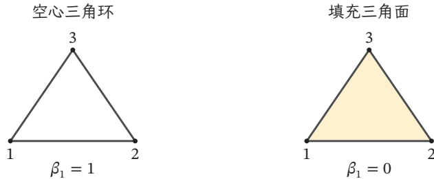
图 8.4 同一圈边在两个复形中的不同含义。左侧没有二维面，闭链 c = [1, 2] + [2, 3] - [1, 3] 不是边界；右侧纳入 [1, 2, 3] ，于是 c = \partial_2[1, 2, 3] 。填充只改变高阶面集合，顶点与边保持相同。图为组合教学示例，不表示观测点云的真实拓扑。
