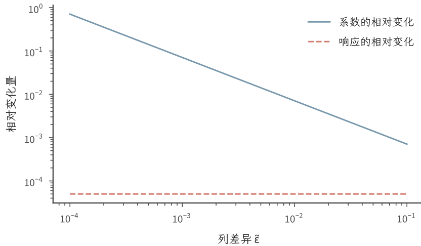
图 7.3 近共线矩阵 \mathbf{X}_\varepsilon 的精确敏感性。取响应 \mathbf{y} = (2, 0)^\top 和扰动 \delta\mathbf{y} = (0, 10^{-4})^\top ；红线是固定的响应相对扰动 5 \times 10^{-5} ，蓝线是解系数相对变化 10^{-4}/(\sqrt{2}\varepsilon) 。双对数坐标显示列越接近，系数变化越大；没有混入数值求解误差。
