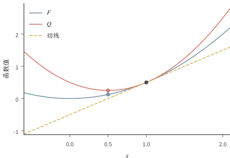
图 4.4 代理上界与切线的区别。蓝线为 F(x) = x^2/2 ，红线为当前点 1 处的主化代理 Q ，黄虚线为同点切线 x - 1/2 。三者在当前点同值同斜率，但切线位于目标下方，最小化它不能使用 MM 的上界链；红点标出代理最小点对应的值。图为解析教学示例。
