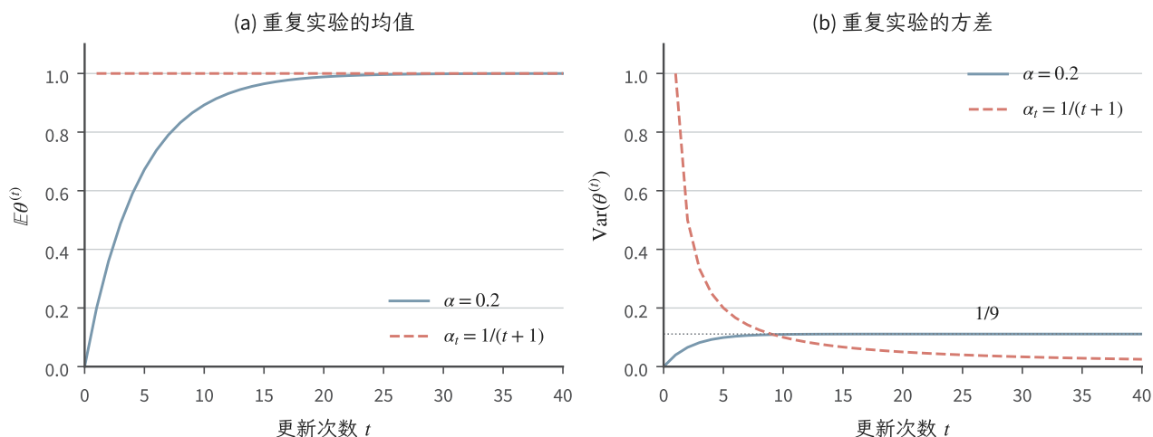
图 10.3 固定步长与样本平均的偏差、方差 (解析式教学图). 取 \theta^{(0)} = 0 , \mu = 1 , \sigma^2 = 1 , 观测独立同分布. 蓝实线对应 \alpha = 0.2 , 红虚线对应 \alpha_t = 1/(t+1) . 右图中固定步长方差趋于 1/9 , 样本平均方差为 1/t .
