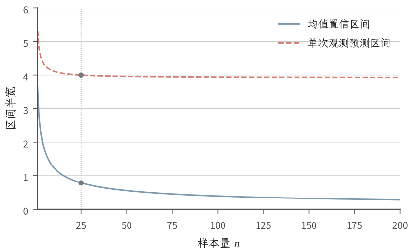
图 11.2 已知 \sigma = 2 的独立高斯位置模型中，两类区间半宽随样本量变化（解析式教学图）。使用四舍五入分位数 1.96，蓝实线为 1.96\sigma/\sqrt{n} ，红虚线为 1.96\sigma\sqrt{1 + 1/n} 。灰竖线标出例 11.17 的 n = 25 ，没有对任何实测数据重复抽样。
