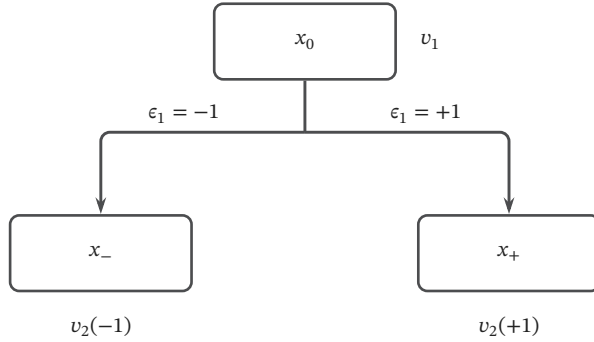
图 5.8 深度为 2 的固定查询树。根查询 x_0 ，左右分支对应 \epsilon_1 = -1 与 +1 ；下方的 v_1, v_2(\pm 1) 是一棵覆盖中心在三个节点预先指定的值，表示近似值而非真实反馈。固定两点输入只观察其中一条路径。
