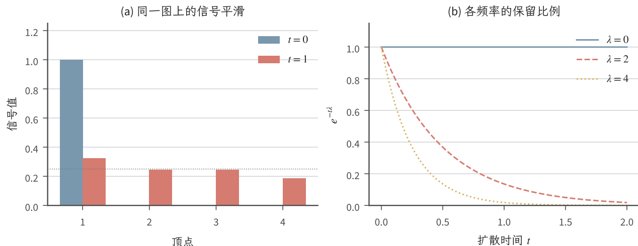
图 14.11 贯穿四顶点图的解析式扩散。左图比较 f(0) = (1, 0, 0, 0)^T 与 f(1) = e^{-L}f(0) ，灰虚线为最终均值 1/4 ；右图绘制三个不同特征值 0, 2, 4 的保留比例，特征值 4 实际具有重数 2 。柱与曲线由该图的拉普拉斯直接计算，不是仿真实验的均值或误差条。
