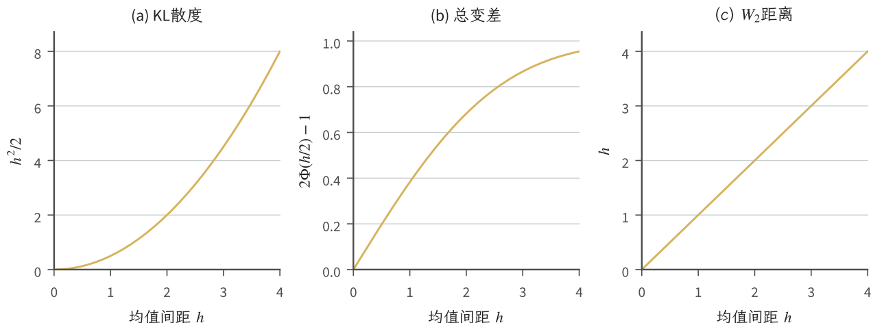
图 12.3 同方差高斯位置族的解析式比较。令 P = \mathcal{N}(0, 1) 、 Q = \mathcal{N}(h, 1) ，分别绘制 D_{\text{KL}} = h^2/2 、 d_{\text{TV}} = 2\Phi(h/2) - 1 与 W_2 = h 。三种量比较的对象和单位不同，面板纵轴也不同。
