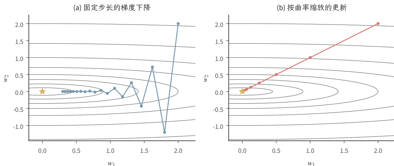
图 4.5 例 4.30 中的精确更新路径。灰线是同一二次目标的等值线，蓝、红圆点分别表示普通更新与预条件更新，黄色星号是最小点。预条件使用了已知曲率，获得和应用这一矩阵的成本仍属于算法代价。
