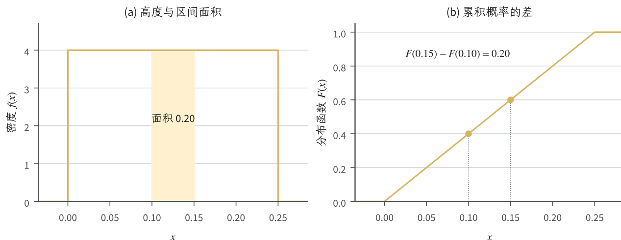
图 9.1 区间 [0, 1/4] 上的均匀分布（解析式教学图）。左图阴影为 [0.10, 0.15] 的概率 0.20，密度高度为 4；右图的概率是 F(0.15) - F(0.10) ，两个端点本身均没有正概率质量。
