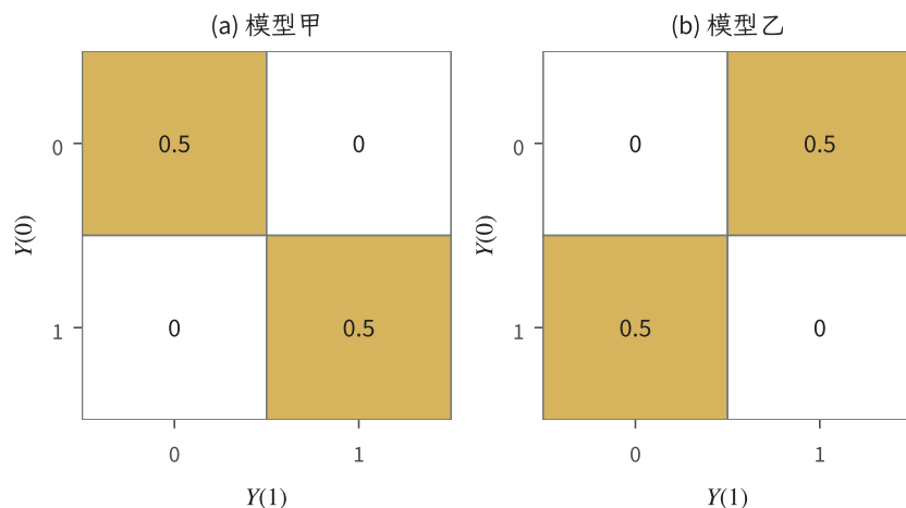
图 13.4 相同干预边缘的两种跨世界配对（教学构造的联合概率图）。行对应 Y(0) ，列对应 Y(1) ，格内数字为联合概率；两图的每个行和、列和均为 1/2 。模型甲个体效应恒为零，模型乙个体效应等概率取 1, -1 ，而两者 ATE 均为零。这些联合表是相容机制的构造，并非从随机试验中直接观测到的数据。
