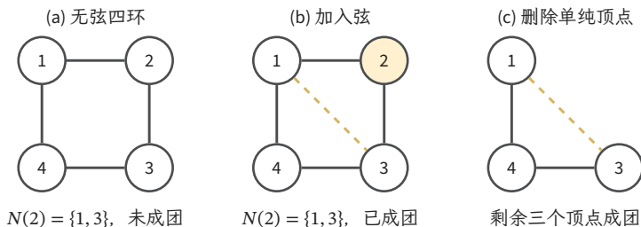
图 14.4 从无弦四环到弦图。黄虚线连接环上的非相邻顶点 1, 3, 把四环分成两个三角形。补边后顶点 2 成为单纯顶点, 删除它留下团 \{1, 3, 4\} , 所以 (2, 1, 3, 4) 是一条完美消元序。树没有长环, 也满足弦图定义; 弦图不要求每个顶点都位于三角形中。
