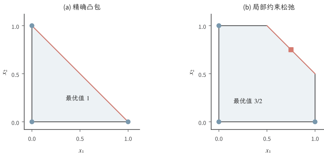
图 4.3 最大化 x_1 + x_2 的两种放宽。左图精确凸包满足 x_1 + x_2 \leq 1 ；右图局部松弛满足 0 \leq x_i \leq 1 与 x_1 + x_2 \leq 3/2 。实心圆为整数可行点，方形为右图的分最优值点 (3/4, 3/4) ，粗边标出各自最优面。两图采用相同坐标尺度。
