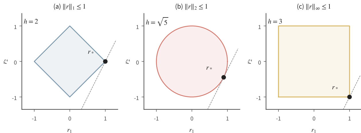
图 6.1 同一线性量 2r_1 - r_2 在三种单位球上的最大值。实线是可行边界，灰虚线是达到最大值时的支撑直线，实心点给出一个最大化扰动。依次得到 2、 \sqrt{5} 和 3；由于单位球关于原点对称，最大绝对值相同，反方向也能达到。三个面板使用相同坐标尺度，图解析教学示例。
