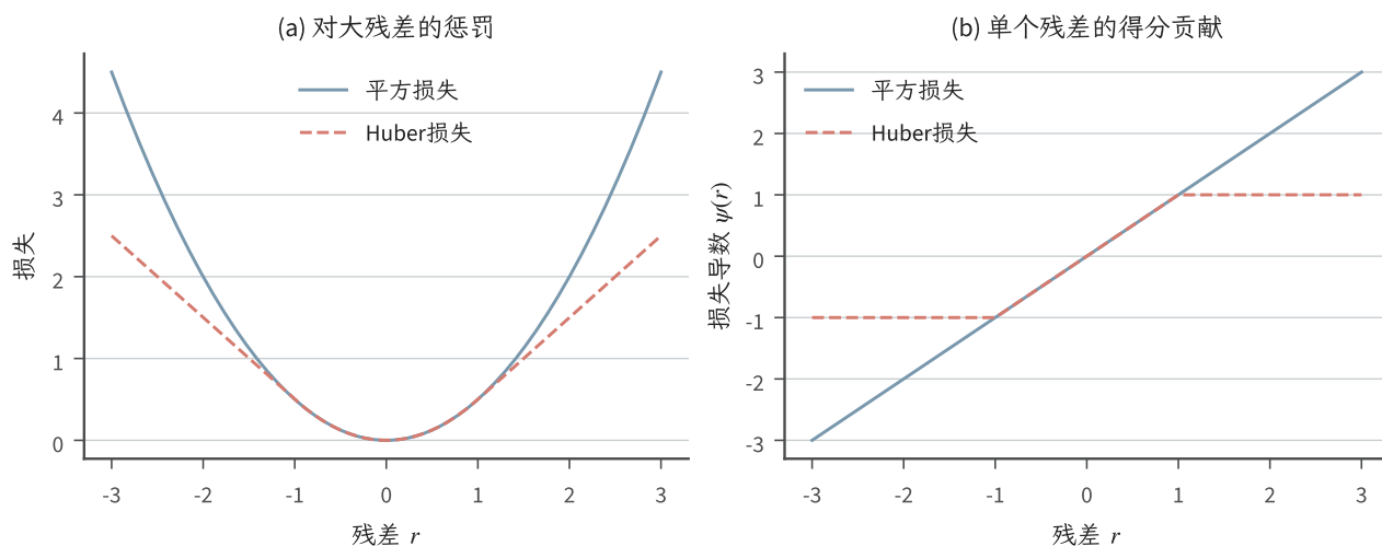
图 11.1 平方损失与阈值 c = 1 的 Huber 损失 (解析式教学图)。左图比较惩罚值, 右图比较对残差的导数; Huber 得分在 [-1, 1] 内截断。横轴是构造残差, 不代表实测异常值分布。
