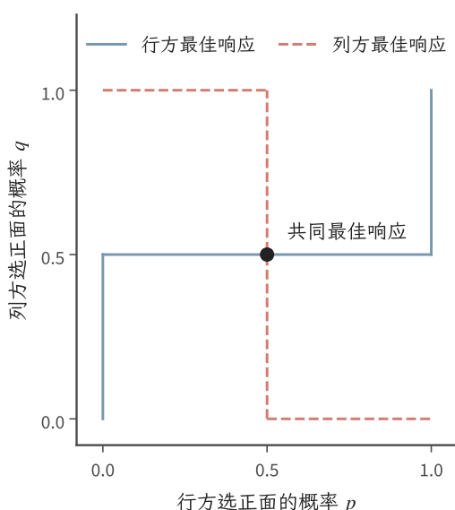
图 19.1 匹配硬币中的最佳响应对应。横轴 p 是行方选 H 的概率，纵轴 q 是列方选 H 的概率；蓝色实线表示行方最大化收益的最佳响应，红色虚线表示列方最小化行方收益的最佳响应。蓝线在 q = 1/2 包含全部 p ，红线在 p = 1/2 包含全部 q ，唯一交点为 (1/2, 1/2) 。线段是最佳响应集合，不是随时间运行的学习轨迹。
