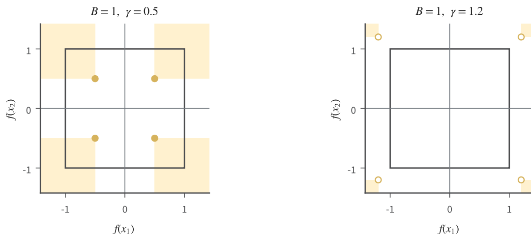
图 2.5 两个分块、 B = 1 与固定阈值 r_1 = r_2 = 0 的输出几何。灰框是函数类允许的 (f(x_1), f(x_2)) \in [-1, 1]^2 ; 浅黄区域要求两坐标分别离阈值至少 \gamma 。左图 \gamma = 0.5 的四种符号可由实心点实现; 右图 \gamma = 1.2 的空心点只标出要求的边界, 全部落在允许框之外, 因而不是类中的函数输出。图为解析教学构造。
