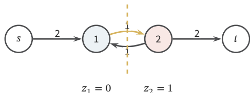
图 14.9 把二值配置读作一个割。图使用正文的两变量数值例子，零容量弧省略。割将 s, 1 与 2, t 分开，因此 z_1 = 0, z_2 = 1 。割容量只计算从源侧指向汇侧的弧：两条容量为 1 的反向弧中，仅黄弧 1 \rightarrow 2 计入，故成本为 1，而不是 2。终端弧 s \rightarrow 1 的容量 2 = D_1(1) 仅在顶点 1 进入汇侧时支付。
