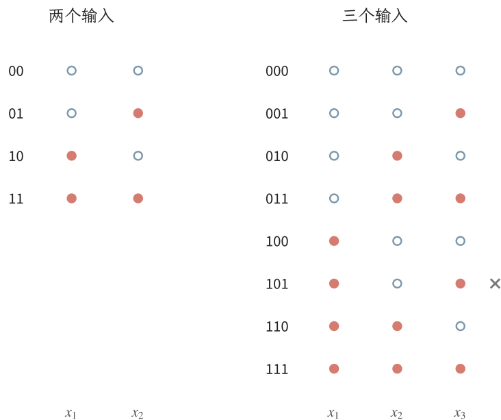
图 2.2 区间分类器在互异有序输入上的全部二值模式。红实心点表示标记 1，蓝空心点表示标记 0；每行是一种模式。左侧两个输入的四行全部可实现，右侧三个输入仅 101 不可实现，灰色叉号标出缺失行。这是精确的有限模式构造，不是抽样统计。
