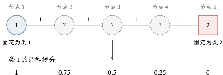
图 3.9 五节点等权无向路径上的硬钳制标签传播。每条边权为 1，左端圆形节点固定为类 1，右端方形节点固定为类 2，问号表示未知标签。下方列出精确调和的类 1 得分，类 2 得分为其补数；内点得分等于两侧邻居的平均。中间节点两类并列，按最小类别编号规则判为类 1。这是教学构造，不是实测结果。
