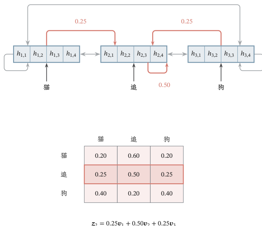
图 12.3 同一序列“猫／追／狗”上的自注意力。每个词元上方的四格条直接表示输入向量的特征坐标；这一组表示分别投影为查询、键和值。灰色双向线表示两个位置可以互相读取，自环表示读取自身，两个方向的权重不必相等。红色箭头从值的来源指向“追”的查询位置，对应下方权重矩阵框出的第 2 行。三个查询各自归一化，图中未另画输出序列；数值为教学设定。
