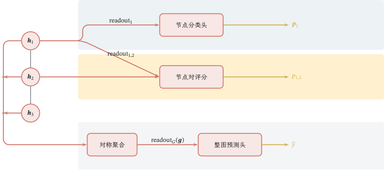
图 11.3 同一组节点表示的三种任务读出。蓝、黄、灰三个底色带分别承载节点、节点对和整图任务，分叉处直接标出 readout_1 、 readout_{1,2} 与 readout_G 。节点预测读取一个节点，边或连接预测读取两个端点及可用的关系属性，整图预测先对全部节点作对称聚合；三个分支不要求在同一模型中同时启用。
