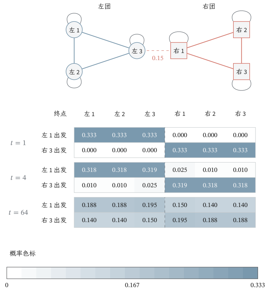
图 5.8 扩散时间与跨团瓶颈。每团三个节点，团内边及所有自环权重为 1，唯一跨团边权重为 0.15。令 \alpha = 0 并按行归一化，热图两行分别表示从左 1、右 3 出发的 \mathbf{P}^t 对应行，六列为固定节点顺序；各时刻共用同一连续概率色标。数值由有理数矩阵乘法计算，显示三位小数，舍入后行和可能略偏离 1。64 步仍未充分混合；因图连通且有自环，极限分布均为 \pi^T = (20, 20, 21, 21, 20, 20)/122 。
