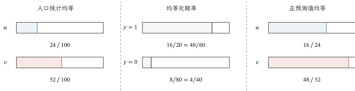
图 13.2 同一批申请者上的三种公平准则。沿用示例 13.1 的计数，两组各 100 人，合格者分别 20 人与 60 人。每条比例条以该项分母为全长，依次比较全体申请者、按资格细分的人、已获选者。共同的真正例率 t = 0.8 与假正例率 f = 0.1 满足均等化赔率，却使另外两项比例不同。此冲突依赖不同基准比例与 0 < f < t < 1 ； f = 0 等边界情形需另行分析。
