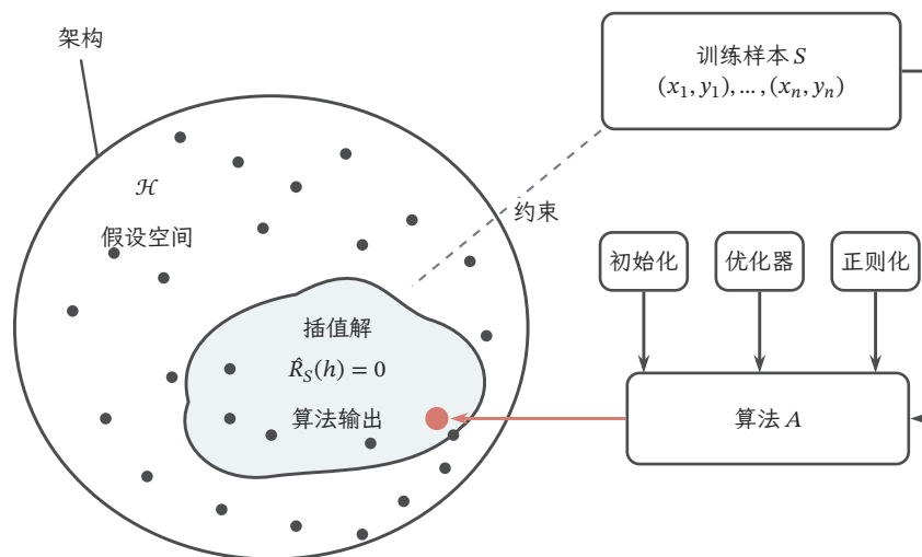
图 8.1 架构、样本和算法分别限定不同对象。外层是假设空间，内层是当前样本上经验风险为零的插值解集合；虚线表示样本施加的约束，实线表示算法的输入与输出。初始化、优化器和正则化参与选解。强调点仅示意算法选出一个插值解，不保证任意算法都实现插值；集合的形状和大小没有数值含义，插值也不保证期望风险小。
