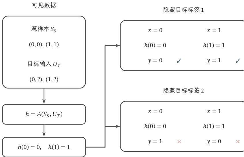
图 9.3 相同可观察数据不能区分两种目标规律。两域都以概率 1/2 产生输入 0 或 1，源标签为 y = x 。算法只收到左侧带标签源样本和无标签目标输入，目标标签并未提供；右侧两种可能分别取 y = x 与 y = 1 - x 。固定算法内部随机数后，两种情形必得到同一输出。图中以 h(x) = x 为例，勾、叉逐点对照同一预测与隐藏标签：零一损失下，源风险为 0，两种目标风险分别为 0、1。任意二分类输出在这两种目标规律下的风险之和为 1。输入完全对齐仍未提供选择目标规律的证据，还需目标标签或连接两域标签规律的额外条件。
