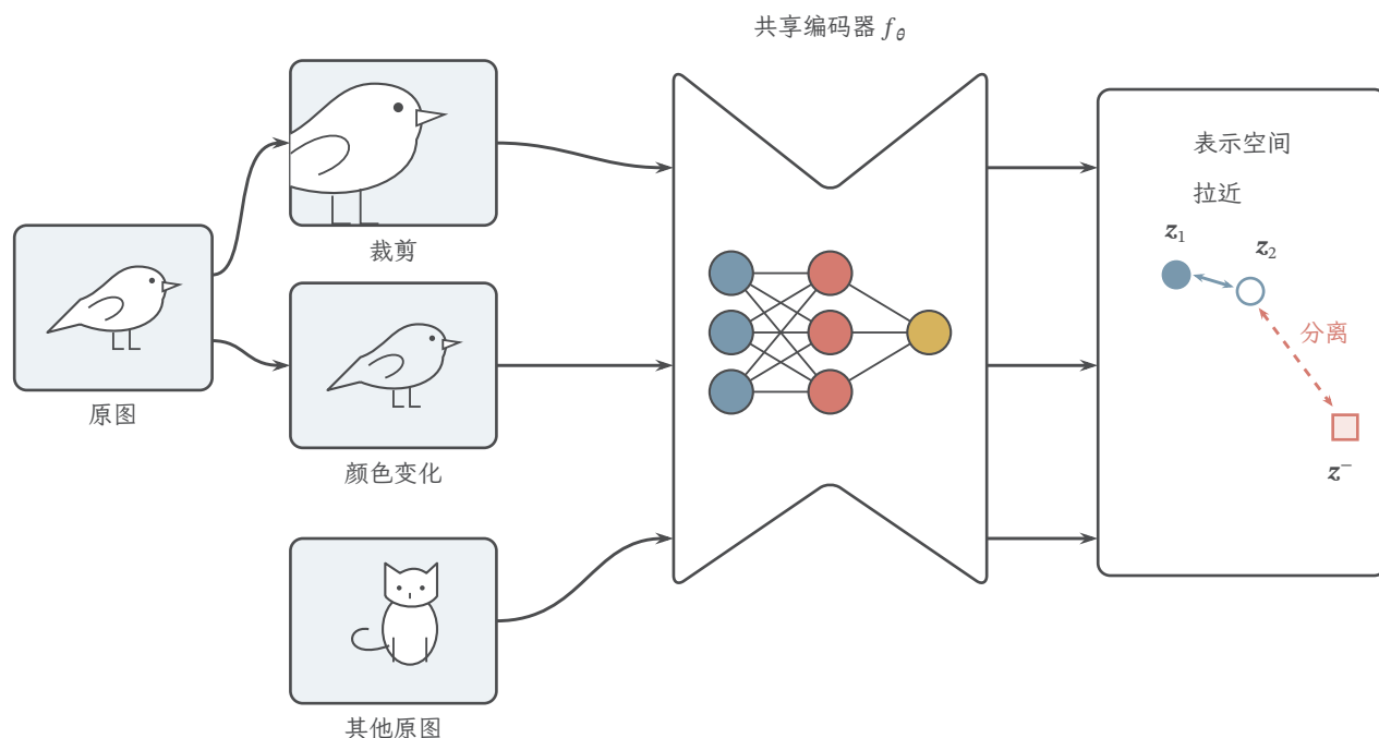
图 3.7 自监督对比学习的教学示意。同一幅鸟的原图经过保留动物可识别性的裁剪与颜色变化，形成两个视图；它们与另一幅猫图的视图经共享参数的编码器得到表示。实心点与空心圆表示同源匹配，方点表示其他原图的对照；箭头只示意同源拉近与对照相对分离的训练目标。动物图元和表示位置均为教学构造，不是实测影像或表示分布。
