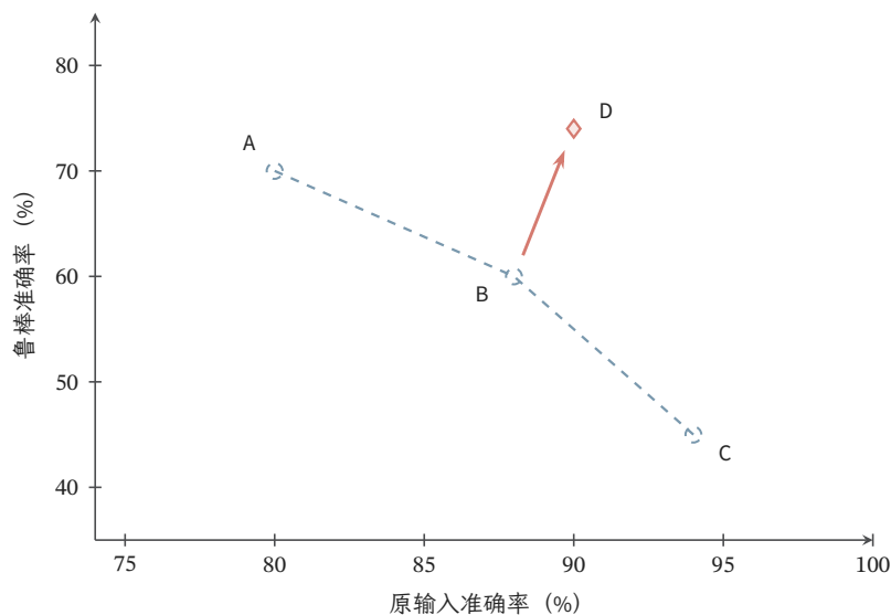
图 12.4 原输入准确率与鲁棒准确率的一种可能取舍。固定 100 个构造样本及同一标签保持扰动范围，A、B、C 的两项正确数分别为 80/70、88/60、94/45；D 为 90/74，同时优于 B。每个候选的鲁棒正确样本都是原输入正确样本的子集。虚线只连接三个教学候选，不是实测曲线或普遍最优边界；评价仍需固定扰动定义与搜索条件。
