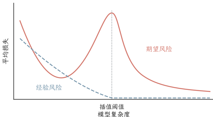
图 8.2 双重下降的定性示意。虚线表示经验风险，实线表示一种可能出现的期望风险变化。插值后的期望风险还取决于算法如何选择。图中曲线用于说明概念，不是实验数据，也不表示所有网络都出现第二次下降。
