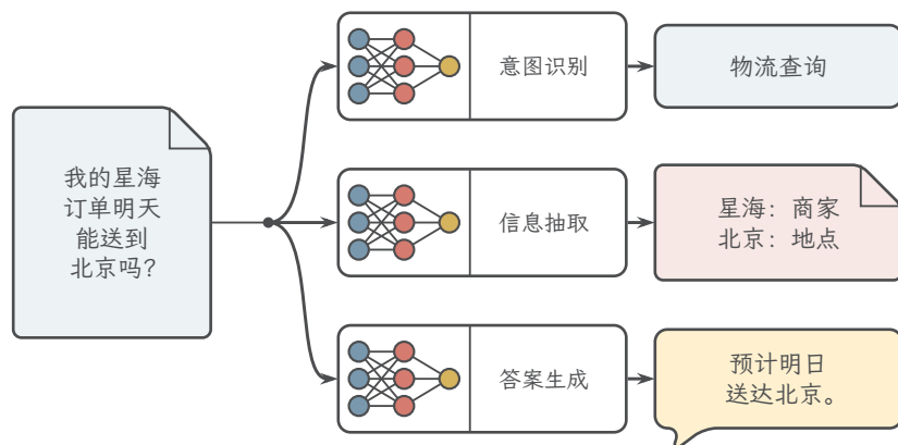
图 1.2 同一句文本的三种输出要求。意图识别输出整句类别，信息抽取识别原文中的实体并给出类型，答案生成产生新的文本。答案句仅为输出形式示意，不声称输入已提供配送承诺。
