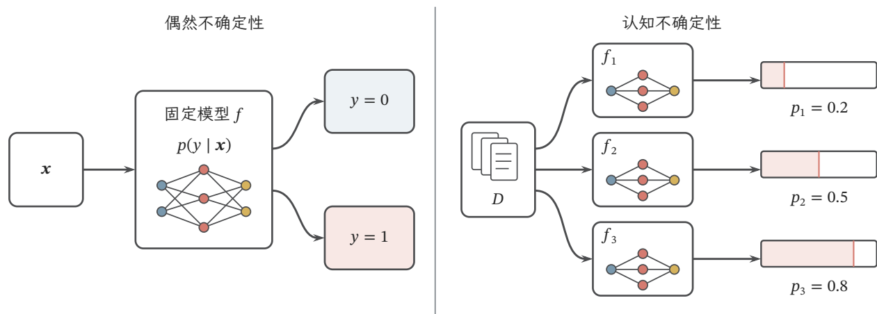
图 11.2 偶然不确定性与认知不确定性的区别。左侧同一可见特征可能对应正常通知或诈骗意图，固定模型也需表达结果分布；右侧相关样本不足，三个候选模型给出不同预测， p_m 简写 p_m(y = 1 | x) 。概率 0.2、0.5、0.8 为教学构造，条长示意预测分歧，不是实测值或后验抽样。两种来源均相对于当前观测与模型假设而言。
