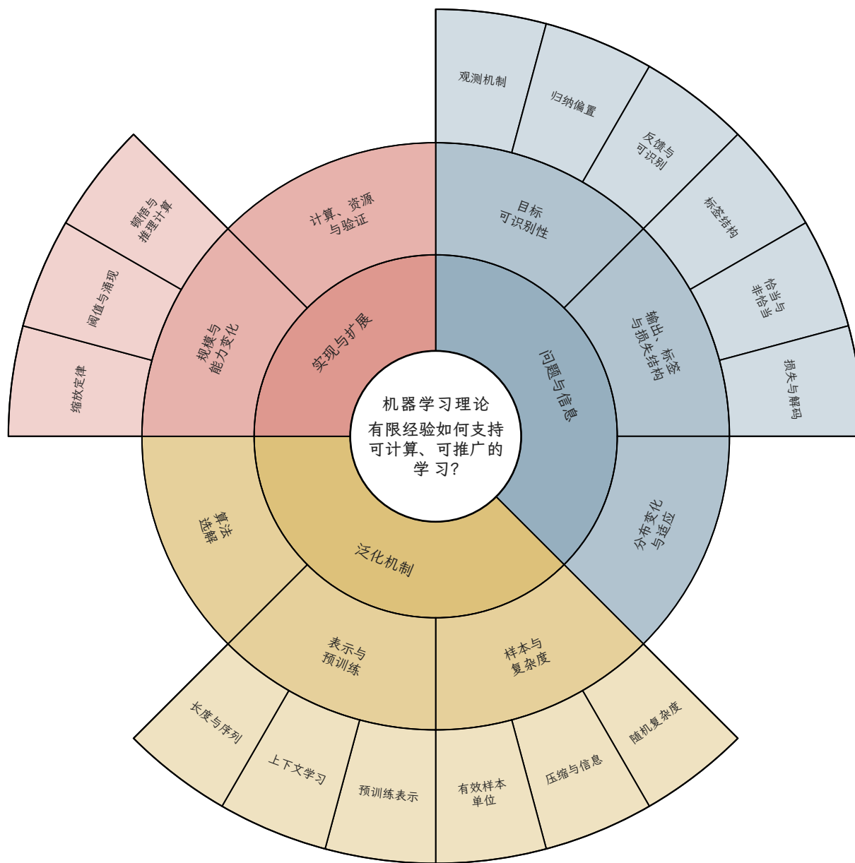
图 4.5 机器学习理论分层研究地图。
