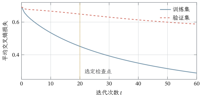
图 1.1 训练集和验证集上的平均交叉熵损失。蓝色实线表示训练曲线，红色虚线表示验证曲线，黄色竖线标出按验证准确率选定的第 20 次迭代；模型选择并非直接读取训练损失的最低点。
