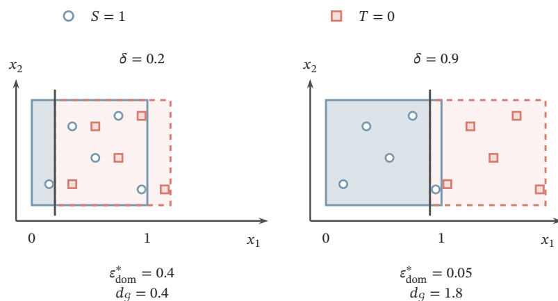
图 9.4 域分类器的错误只对应输入散度项。源输入均匀分布于 [0, 1]^2 , 目标支持沿 x_1 平移 \delta ; 圆点、方块的位置为教学构造, 错误率由区域概率计算。 \mathcal{H} 含双向阈值与常值假设, 域分类器类取 \mathcal{G} = \mathcal{H} \triangle \mathcal{H} 。其中 g = h_0 \oplus h_\delta 在左侧浅色带预测源域, h_a(x) = \mathbb{I}\{x_1 \geq a\} ; 两域均等先验时, 最小域错误为 (1 - \delta)/2 , d_g = 2\delta 。任务风险界还包含源风险及 \lambda = \inf_{h \in \mathcal{H}} (R_S(h) + R_T(h)) , 不能只由域错误决定。
