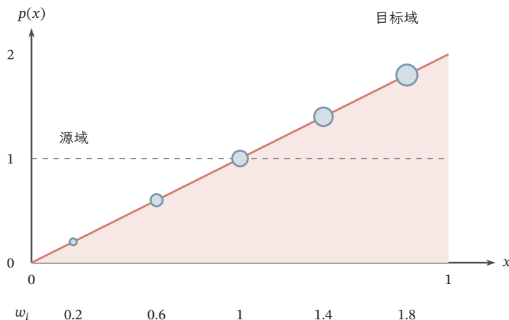
图 9.5 重要性权重重新分配源样本的贡献。在 [0, 1] 上构造源密度 p_S(x) = 1 、目标密度 p_T(x) = 2x ，二者均积分为 1，因此 w(x) = 2x 。五个源样本位置人为取为 0.1、0.3、0.5、0.7、0.9，权重依次为 0.2、0.6、1、1.4、1.8。圆点叠在目标密度上，面积与权重成正比，面积不表示局部样本数量。目标输入必须受到源输入覆盖；要使用风险恒等式，还需保持相同的条件标签分布。
