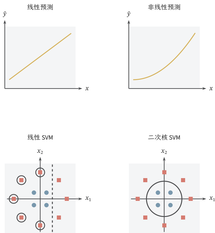
图 2.4 线性与非线性关系的几何示意。上排依次为线性预测与非线性预测，下排用同一组环形样本对照线性 SVM 的限制与二次核 SVM 的表达能力；圆点和方点代表两类。左图虚线只展示一条候选直线，空心圈标出按其左右类别分配时的错分点，不代表最优 SVM 解。外圈方点的凸包包含内圈圆点，故任何直线都不能完全分离这组样本。右图以圆心为坐标原点，半径 8 的边界可由二次核 \kappa(\mathbf{u}, \mathbf{v}) = (\mathbf{u}^\top \mathbf{v})^2 与偏置表示。图为几何构造，非训练结果。
