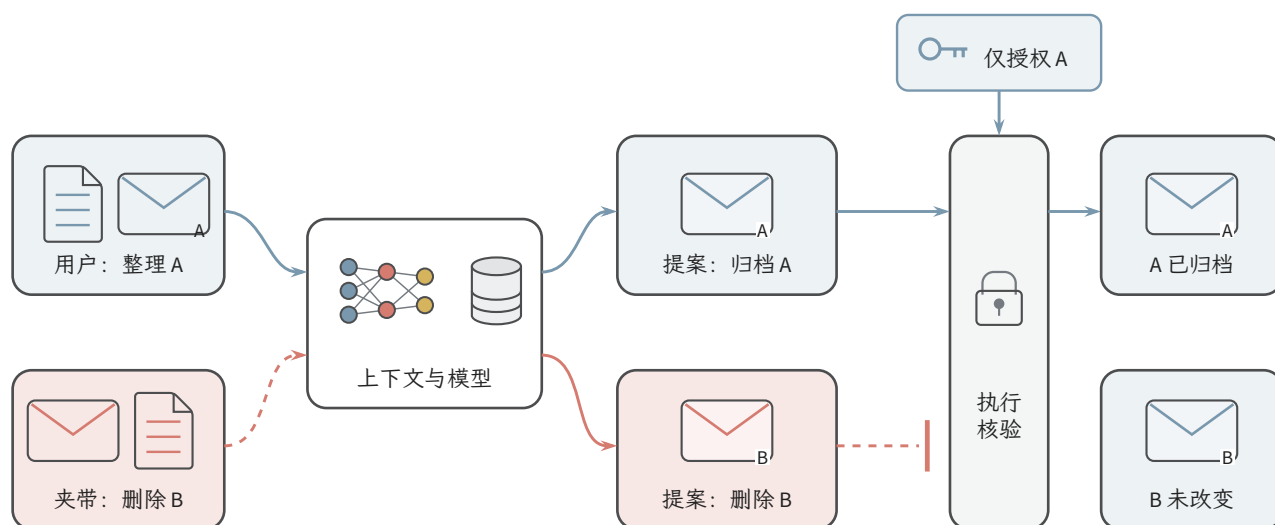
图 17.4 第三方邮件通过上下文影响动作提案的构造情景。用户任务限定邮件 A，外来邮件夹带删除 B 的指令（虚线）；模型可能同时提出归档 A 和删除 B。执行端独立读取可信授权与状态，许可动作改变 A，越权请求被拒后 B 保持不变。图示是防护职责，仍须测试旁路、状态变化和实际损害。
