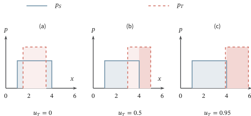
图 9.2 同尺度的三种支持覆盖。源密度均为 [1, 4] 上的 1/3 ，目标密度均为长度 2 区间上的 1/2 ；(a)、(b)、(c) 的目标支持依次为 [1.5, 3.5] 、 [3, 5] 、 [3.9, 5.9] 。深色区域没有源密度，其目标概率 u_T = \mathbb{P}_T\{p_S(X) = 0\} 依次为 0、0.5、0.95。实线、虚线与底色共同区分源域、目标域；只有 (a) 满足覆盖条件 p_T(x) > 0 \Rightarrow p_S(x) > 0 。密度为规范化教学构造，不是实验分布。
