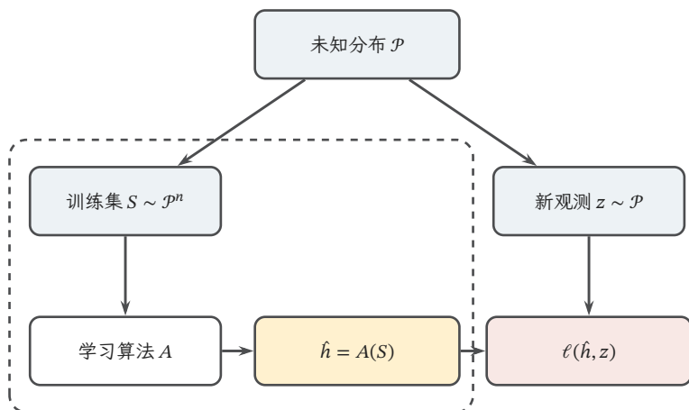
图 4.1 评价分类器与评价学习算法所涉及的两层随机性。固定一次训练的结果后，期望风险对右侧的新观测取平均；重新抽取左侧训练集则可能得到另一个分类器。学习保证还要控制后一种随机性导致训练失败的概率。
