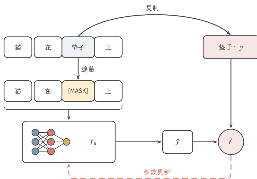
图 3.5 掩码预测以“猫在垫子上”为教学例子。输入将“垫子”替换为 [MASK]，原词单独保留为比较目标；模型只能读可见上下文，不能读被保留的答案。括线汇合全部可见词元，珊瑚红虚线将损失反馈到参数；内部网络只作模型图元。
