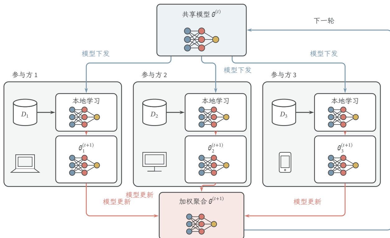
图 3.13 中心协调式联邦学习的一轮通信。协调方向三个示意参与方下发同一组共享参数 \theta^{(t)} ；各方使用边界内的本地记录 D_i 学习，上传本地模型更新。加权聚合形成下一版本 \theta^{(t+1)} ，再统一下发。记录图元与参与方数量为教学示意；原始记录留在本地，但模型更新仍可能泄露信息，联邦组织方式本身不提供隐私保证。
