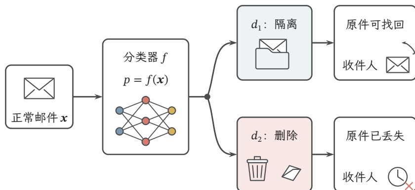
图 10.3 同一封正常邮件被误拦后的两种处置。预测 p = f(\mathbf{x}) 保持不变，上方隔离保留原件并允许找回，下方永久删除原件。末端收件人承担找回成本或错过期限的风险；真实状态 y 、发现延误与恢复成本仍须纳入 L(a, y) 。图示为构造情景，不保证隔离后的邮件会及时找回。
