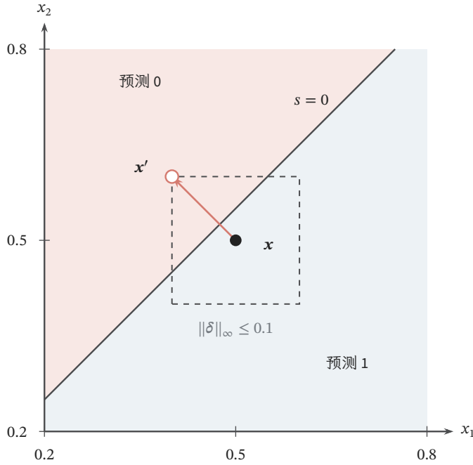
图 17.3 正文二维线性评分器中的预算内扰动。原输入是 (0.5, 0.5) ，分数 0.05；候选 (0.4, 0.6) 的扰动为 (-0.1, 0.1) ，无穷范数 0.1，分数变为 -0.15 。浅色区域区分模型预测，实线为 s = 0 ，虚线方形为允许的扰动集合。模型翻转与真实标签改变是不同事件：只有确认邻域真实标签仍为 1 时，该候选才是有效攻击反例。几何与分数均为教学构造，单步搜索不保证任意模型上的攻击成功。
