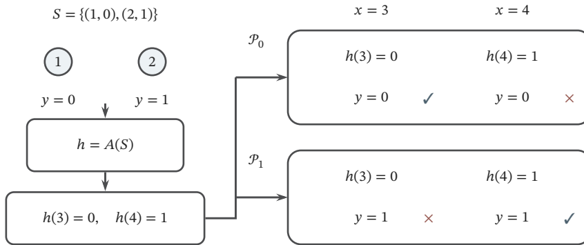
图 4.2 同一训练样本不能排除两种相反的隐藏真值。四个输入各以 1/4 的概率出现；两种来源在已见的编号 1、2 上分别标为 0、1，在未见编号 3、4 上分别全标为 0 或全标为 1。图中固定输出取 h(3)=0, h(4)=1 ，勾、叉直接标出它在两个来源中各错一个未见输入。给定一样本和算法内部随机数，两种来源中必有同一输出；对任意二分类预测，每个未见输入的两份零一损失之和都是 1，故风险之和至少为 1/2 。此图展示固定样本的信息缺口；下文定理再处理随机训练样本。
