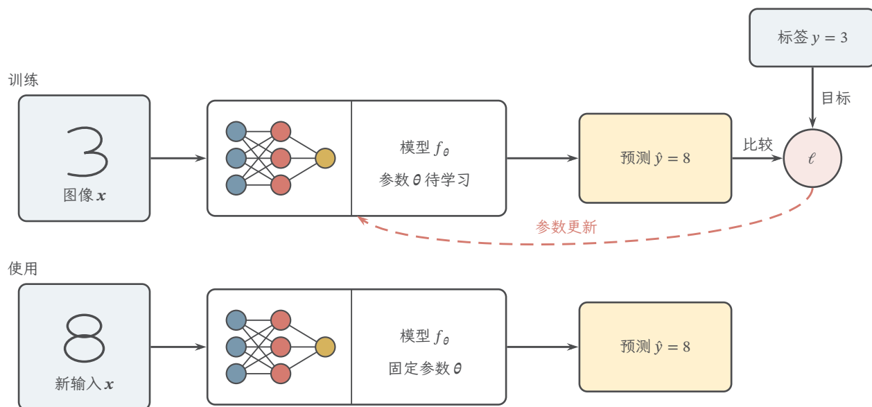
图 3.1 监督学习中的训练与使用。训练时图像进入模型，目标标签单独进入损失比较，虚线反馈用于更新参数；使用时只提供新图像。训练行中，数字 3 被暂时预测为 8，原标签 3 只进入比较；使用行没有提供目标。图像卡与内部网络为教学示意，不指定模型架构。
