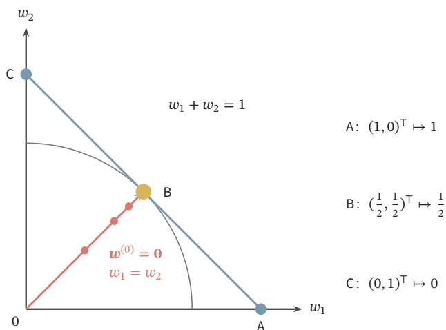
图 8.6 一个训练观测对应多个插值参数。直线上的 A、B、C 都使输入 (1, 1)^T 的预测为 1，右侧列出它们对同一新输入 \mathbf{x}_{\text{new}} = (1, 0)^T 的预测。对半平方损失从零初始化，图中以步长 1/4 画出前三次更新，轨迹趋向 B；细弧表示经过 B 的欧氏范数等值线，说明 B 是插值直线上距离原点最近的点。这个教学例子解释选解规则，不给出新输入的真实标签或泛化保证。
