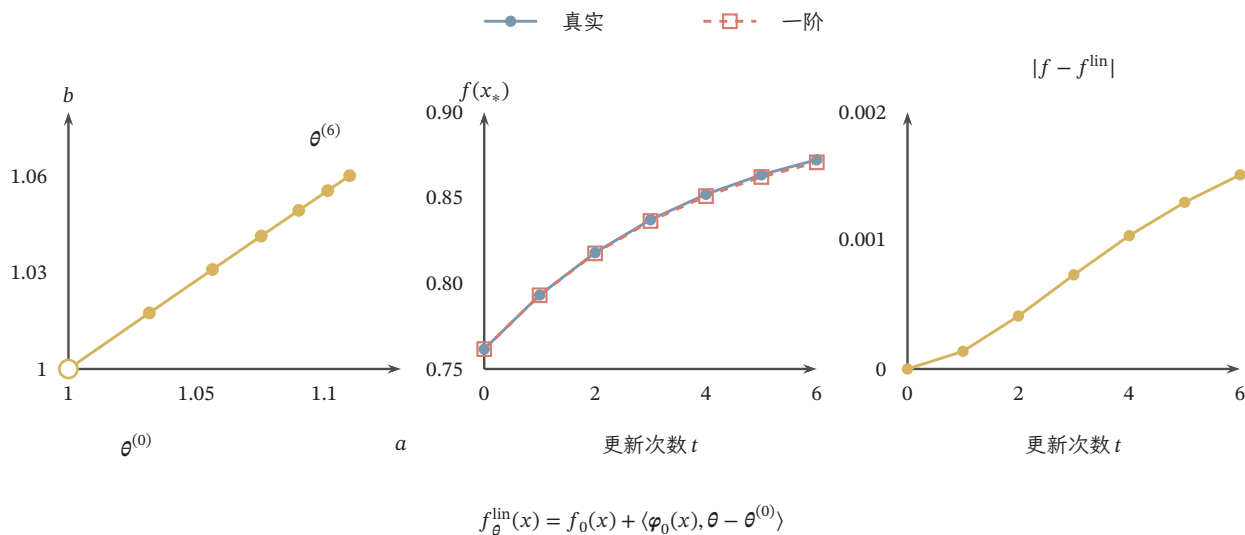
图 8.4 初始化附近的参数轨迹与输出线性化。教学网络为 f_{(a,b)}(x) = a \tanh(bx) ，初值为 (1, 1)^T ；用单个样本 (x, y) = (1, 0.9) 的半平方损失、步长 0.3 执行六次梯度下降，连同初值共七个检查点。中间的真实输出和一阶输出均在左侧同一参数轨迹上计算；三面板绘图区大小相同，参数、输出和绝对余项各用所标坐标范围，不能按纸面高度直接比较数值。右侧余项末次约为 0.00152。近初始化时二者接近，但余项并非零。参数增量经初始雅可比映射到输出/函数空间的切空间；NTK 是初始梯度在不同输入上的内积。此有限网络示例展示近似对象，不证明训练中核恒定或新输入上的误差受控。
