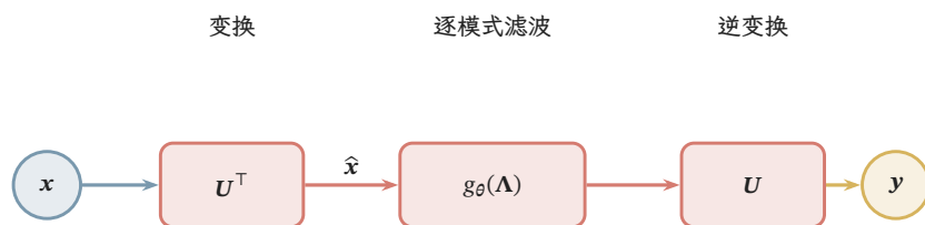
图 11.5 谱滤波的计算路径。节点信号 \mathbf{x} 经 \mathbf{U}^\top 分解为图傅里叶系数, 每个模式由 g_\theta(\lambda_k) 调整, 再经 \mathbf{U} 还原为节点信号。左、右两端使用同一张图和同一节点顺序; 中间向量的下标表示频率模式。
