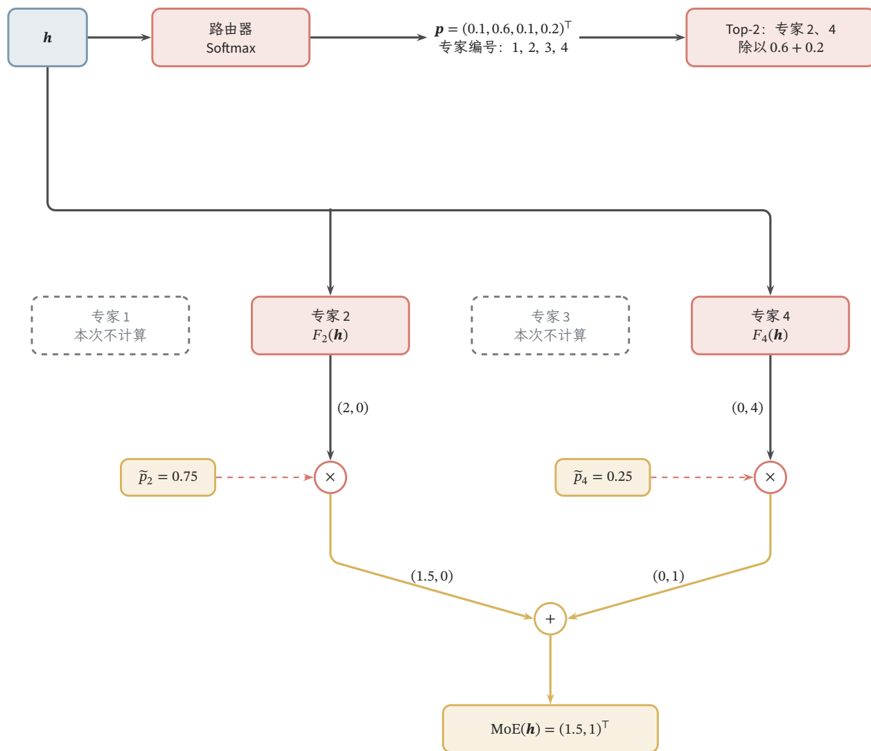
图 12.25 Top-2 混合专家的一次完整计算，概率与二维专家输出均为教学设定。上方路由器选出专家 2、4 并给出重新归一化的权重；下方实线传递隐藏表示及专家结果，虚线向乘法节点提供标量权重。专家输入始终是同一个 h ，加权发生在专家输出之后，最终 0.75(2, 0)^T + 0.25(0, 4)^T = (1.5, 1)^T 。灰色专家 1、3 本次不计算；图省略容量限制、辅助训练目标及块外残差。
