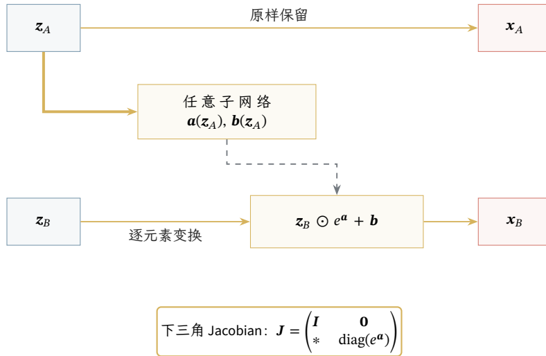
图 29.2 仿射耦合层的计算依赖。粗线把 \mathbf{z}_A 送入任意子网络, 该子网络只产生缩放和平移参数; 下方逐元素仿射变换才真正改变 \mathbf{z}_B 。Jacobian 为下三角结构, 因此子网络不必可逆, 整层的对数行列式只需对缩放对数求和。逆向计算先恢复原样保留的 \mathbf{z}_A , 再撤销缩放和平移。
