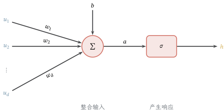
图 7.6 人工神经元的计算示意。标有 w_j 的输入边表示乘以权重，求和节点再加入偏置 b ，激活函数产生输出 h 。接收输入、整合影响与产生输出，是它与生物神经元之间的功能对应；图中的数学运算不完整复现细胞机制。
