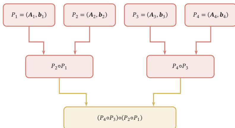
图 10.12 仿射状态更新的有序组合。四个单步变换先组成两个连续片段，再组成整段； Q \circ P 表示先执行 P 再执行 Q 。平衡组合树展示的是扫描中的汇总阶段，完整前缀扫描还要把此前片段的结果传给各位置，才能得到每步状态。树形计算可缩短依赖深度，但不改变输入顺序。
