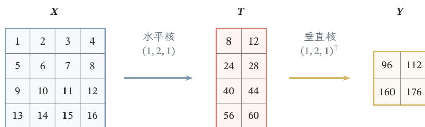
图 9.12 秩一空间核的两阶段计算。水平核与垂直核均为 (1, 2, 1) ，组成 3 \times 3 核 \mathbf{u}\mathbf{v}^\top 。在步长一、无填充条件下，原 4 \times 4 输入先变为 4 \times 2 中间结果，再变为 2 \times 2 输出。该小例子的两阶段核心乘法量仍为三十六次，图示验证的是结果等价，而非每种输入尺寸都能节省计算。
