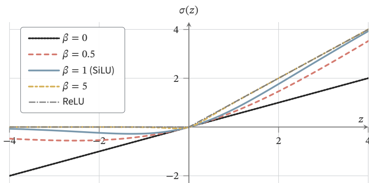
图 8.6 Swish 在不同 \beta 下的函数图像。 \beta = 0 给出线性函数 z/2 ， \beta = 1 就是 SiLU，较大的 \beta 逐渐形成接近 ReLU 的响应。图中参数固定为 0, 0.5, 1, 5，ReLU 用作极限参照；它不展示可学习 \beta 在某次训练中的实际轨迹。
