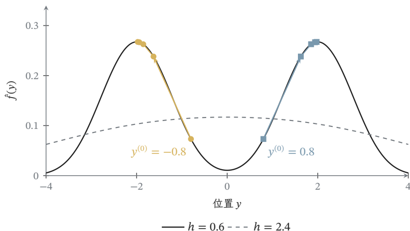
图 4.5 Mean Shift 的密度爬升与带宽效应。左右各有三个样本，位置为 -2.5, -2, -1.5 和 1.5, 2, 2.5 ，均采用高斯核。彩色标记给出带宽 h = 0.6 时从 \pm 0.8 出发的初始位置和四次更新，箭头指示第一次移动；灰色虚线对应 h = 2.4 ，轨迹在黑色实线上计算。
