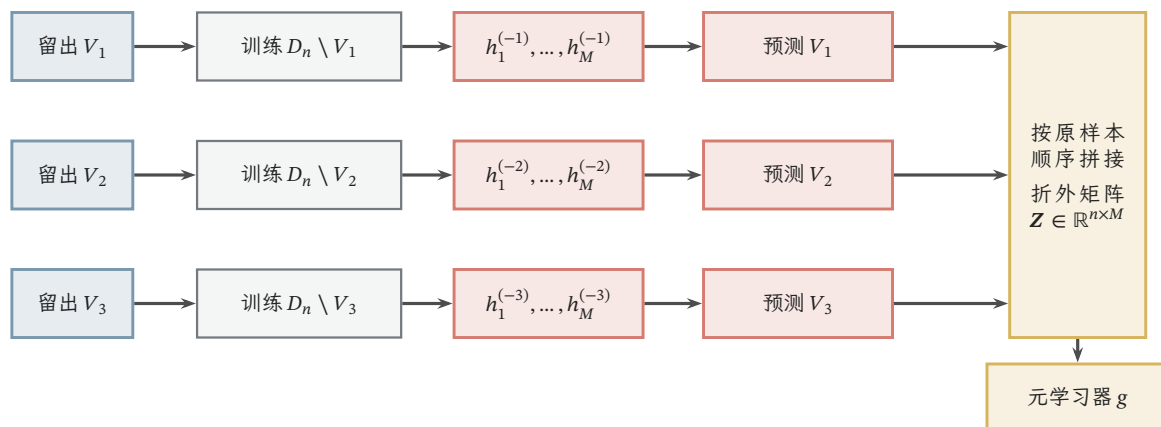
图 6.9 三折 Stacking 的折外特征构造。每一折轮流作为留出折, 临时成员只在其余两折训练, 并为留出折产生预测; 拼接三次预测得到完整折外矩阵 \mathbf{Z} , 元学习器以 \mathbf{Z} 为输入并使用对应标签拟合。部署阶段的基成员还需按预先规定的方式重训或保留。
