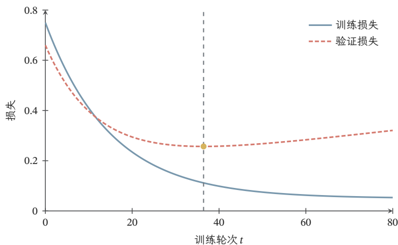
图 15.2 提前终止的示意曲线。训练损失取 0.05 + 0.7 \exp(-t/15) ，验证损失取 0.16 + 0.5 \exp(-t/12) + 0.002t ， t 为训练轮次。虚线标出该构造验证函数的极小点附近，说明继续拟合与验证表现可能分离；这些函数仅用于讲解，不是实验记录。
