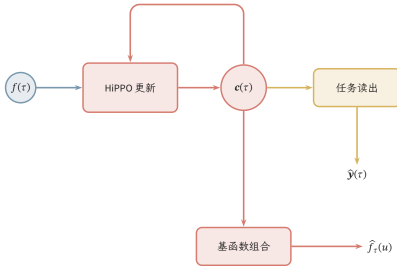
图 10.13 HiPPO 投影记忆与任务网络的一种组合。红色反馈维护系数状态，黄色读出产生任务预测；下方将同一系数与基函数组合，近似重构历史信号。HiPPO 本身规定记忆表示及更新，图中的任务读出与输入特征映射可另行学习，并非唯一的 HiPPO 网络架构。
