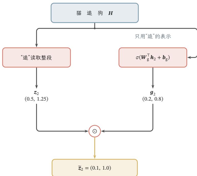
图 12.18 以“追”为查询的聚合后门控。左支路从整段序列读取内容，右支路仅由当前词元表示产生 Sigmoid 门。教学数值中，聚合结果 (0.5, 1.25) 与门 (0.2, 0.8) 逐坐标相乘，得到 (0.1, 1.0) 。门控制的是输出特征，而不是三个来源位置的概率；图中固定一个头并省略头索引、多头拼接和输出投影，数值并非训练测量。
