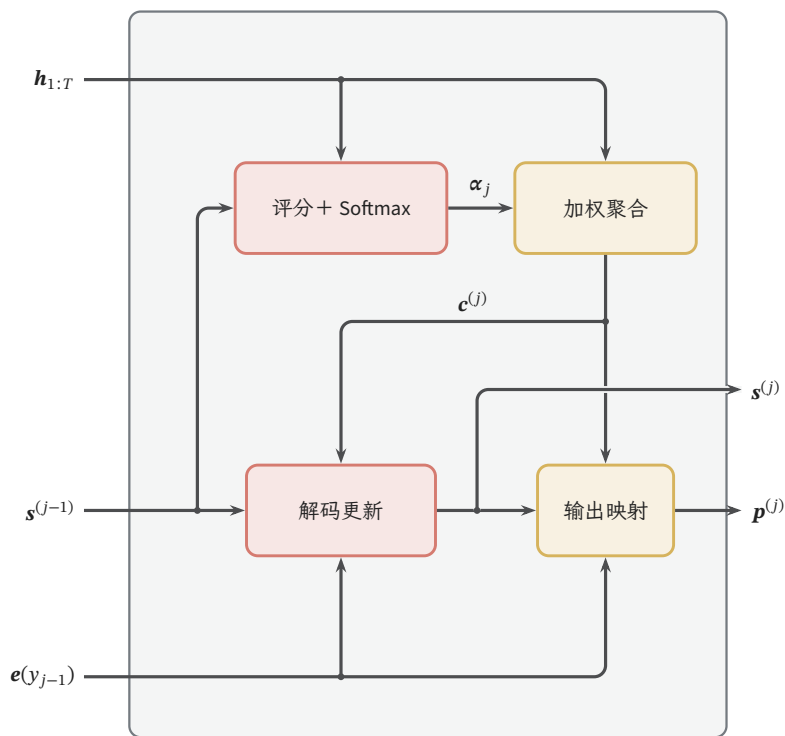
图 10.11 带注意力的一个解码步。左侧为保存的编码状态 \mathbf{h}_{1:T} 、旧解码状态和此前目标的嵌入，右侧为新解码状态和输出概率。查询先用旧解码状态产生权重 \alpha_j = (\alpha_{j,1}, \dots, \alpha_{j,T}) ，上下文再进入更新与输出映射；输出映射还可读取目标嵌入。编码状态在各解码步重复读取，图中不重新执行编码器。
