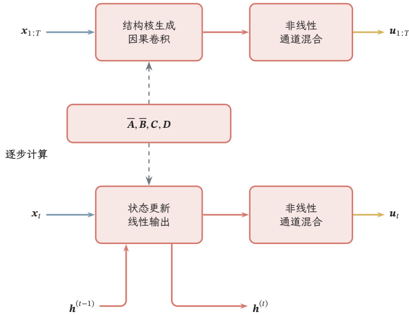
图 10.14 S4 层的整段与逐步计算。两个路径共享同一组离散状态参数及后续通道映射，虚线表示参数供给。零初态时，因果卷积与递推得到相同线性序列输出；非零初态需要补上对应初态响应。图中 \mathbf{u} 是层输出特征，任务预测还需相应读出。
