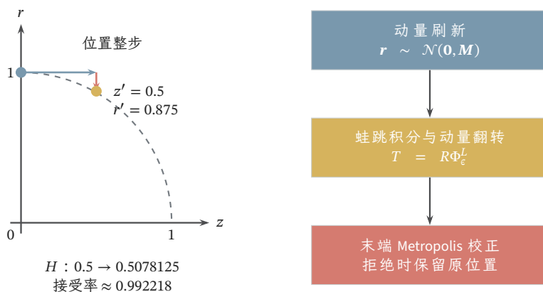
图 23.2 标准正态目标的一步 HMC 计算。左图中虚线圆弧属于 H = 1/2 的精确轨迹, 折线表示 \epsilon = 0.5 的蛙跳位置整步与末端动量半步; 初始动量半步因 z = 0 而不移动。右图区分保持扩展分布的动量刷新与校正更新; 末端动量翻转未画在相图上。
