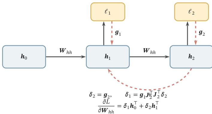
图 10.5 两时间步 BPTT 的显式展开。蓝色实线是共享 \mathbf{W}_{hh} 的前向调用, 红色虚线从 \ell_2 与 \ell_1 回传并在 \delta_1 处汇合; 同一循环矩阵的梯度等于两个调用位置的外积贡献之和。底部指出长序列中状态 Jacobian 连乘是梯度消失或爆炸的直接来源。
