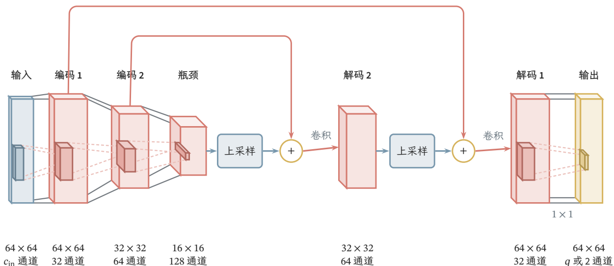
图 9.23 用于分割或着色的三尺度编码器—解码器。长方体表示特征张量，标签给出空间尺寸和通道数。每级解码先上采样到下一尺度，再由圆形 + 沿通道拼接同尺度的编码特征，随后卷积融合；上方旁路均接入拼接节点。图中上采样保持通道数，因此两次拼接分别得到 128 + 64 = 192 和 64 + 32 = 96 个通道，卷积后变为 64 和 32 个。输出头产生 q 个类别得分或两个颜色通道；采用 same 卷积，省略原始 U-Net 的裁剪。
