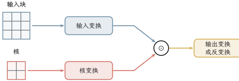
图 9.10 变换类卷积的共同流程与不同目标。Toom-Cook 通过多项式求值及插值恢复完整乘积系数；Winograd 通过固定小矩阵恢复所需输出块；FFT 在补零后的频域相乘并反变换。输入和核可以分别变换，变换结果按输入通道相乘并求和；能复用多少次，决定变换开销能否被摊薄。
