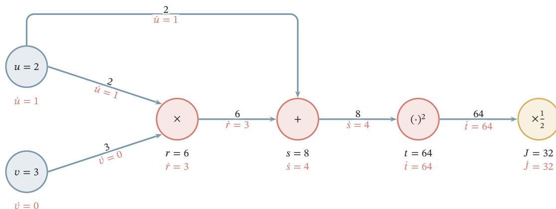
图 8.11 具体算子图上的前向模式。圆形节点表示乘法、加法、平方和缩放; 实线上方的黑色数字是传入算子的值, 下方红色数字是同一路径上的方向导数。每个算子下方再用两行列出其输出值和输出方向导数。输入方向 (1, 0) 给出 \partial J / \partial u = 32 ; 加法处的 \dot{s} = 3 + 1 包含了 u 的两条路径。
