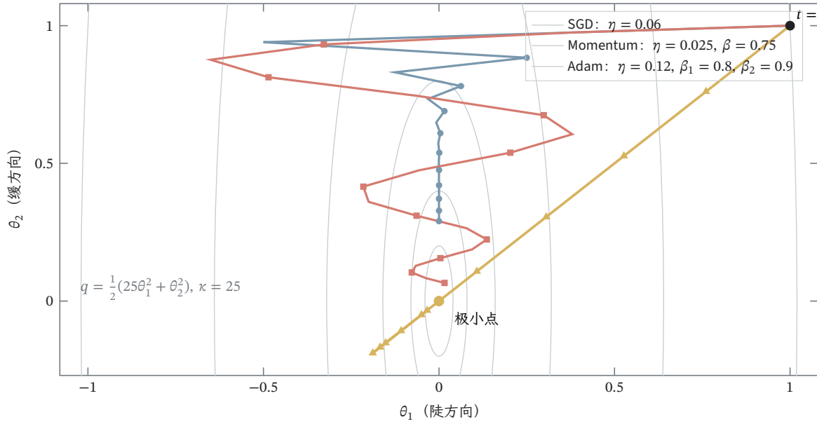
图 14.3 SGD、动量与 Adam 在同一病态二次目标上的前 20 步。目标为 q(\theta) = (25\theta_1^2 + \theta_2^2)/2 ，条件数 \kappa = 25 ，三者均从 (1, 1)^T 出发并使用完整梯度；灰线为等高线，黄色点为唯一极小点。轨迹由正文定义的递推式直接计算，图例列出步长和矩系数。不同超参数会改变速度与振荡，不能据此推出某方法对一般非凸随机训练恒优。
