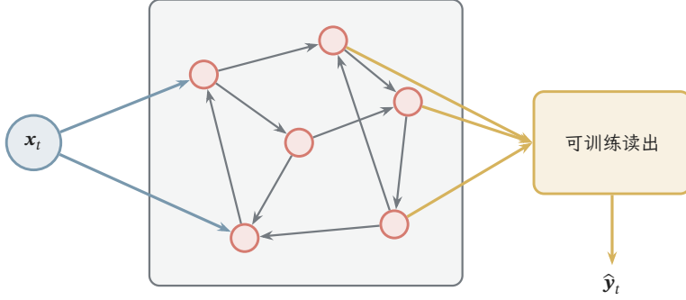
图 10.6 储备池计算的参数分工。输入进入固定的循环动态，多个内部单元共同形成随历史变化的状态，可训练读出将状态映射到目标。灰色连线表示固定连接，黄色箭头表示参与拟合的读出；内部连接只示意结构，不表示某个随机生成样本。ESN 使用连续值激活，LSM 可由脉冲活动及其滤波响应形成读出特征。
