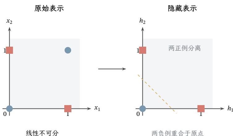
图 7.2 异或任务在变换前后的表示。圆点是标签为 0 的负例，方点是标签为 1 的正例。左侧两类点交错，无法用一条直线分开；右侧按式(7.4)变换后，两个负例重合，虚线 h_1 + h_2 = 1/2 将两类分开。坐标和变换均为教学构造。
