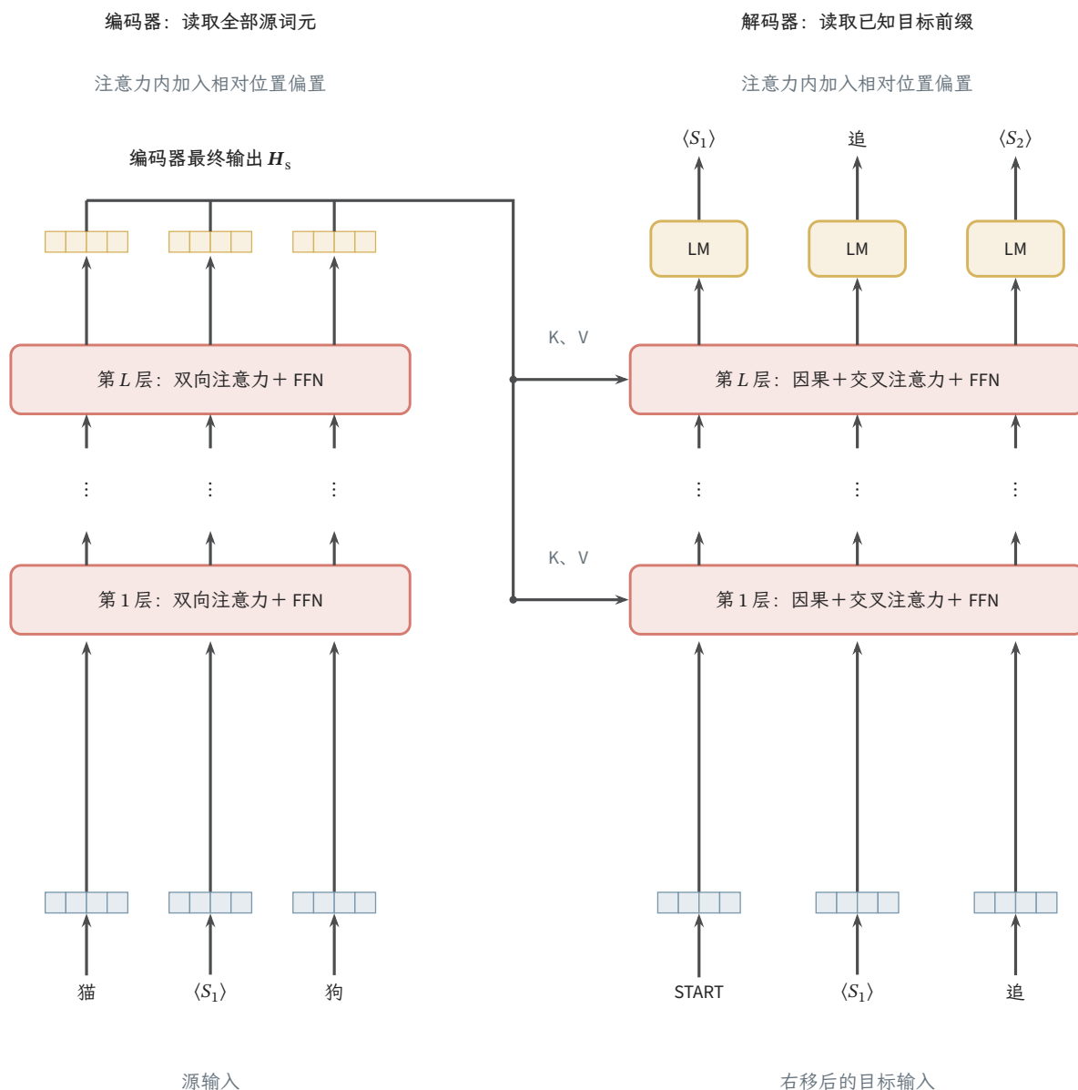
图 12.13 T5 的片段恢复任务与整网结构。 \langle S_1 \rangle 替代源句中被删去的片段，目标中的同名标记引出该片段， \langle S_2 \rangle 标记恢复序列的结束；右侧输入已右移，START 表示解码起始符。每个长条是一整层，编码器最终输出供各解码层的交叉注意力生成 K、V。注意力内部使用相对位置偏置，输入不叠加绝对位置向量。省略层内残差、Pre-LN、Dropout 与末尾 EOS。参考 Bishop 与 Bishop (2024) 图 12.20 的布局重绘，结构与任务依据 Raffel 等 (2020)。
