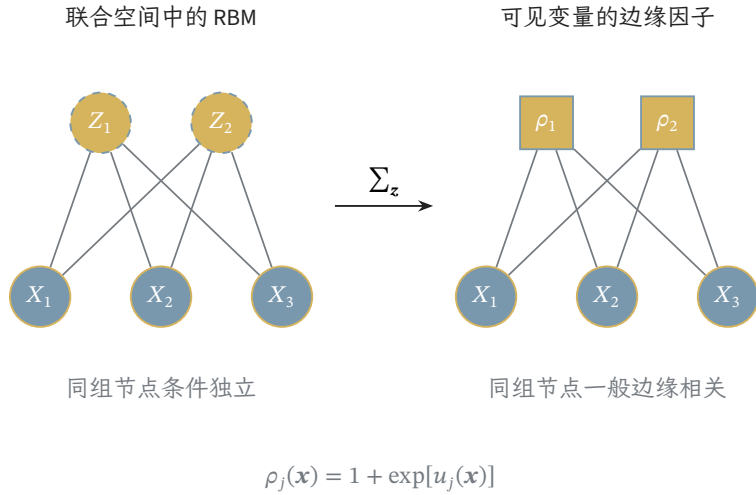
图 27.2 左侧 RBM 只有可见组与隐藏组之间的边；固定任一组，另一组条件独立。右侧消去两个隐藏节点，每个方形因子代表 1 + \exp[u_j(\mathbf{x})] ，均作用于三个可见变量。两侧均省略可见偏置对应的一元势。二部条件独立不等于可见变量边缘独立。
