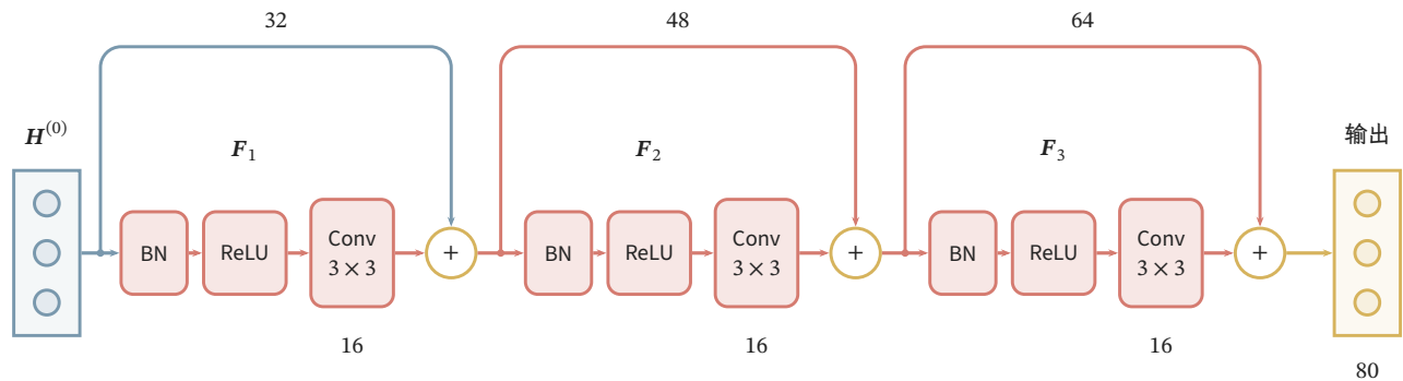
图 9.22 DenseNet 的三层教学密集块。各 F_\ell 依次执行 BN、ReLU 和 3 \times 3 卷积，保持 32 \times 32 空间网格并新增 16 个通道。三次变换分别读取 32、48、64 个通道；上方旁路保留变换前的全部特征，标出的 32、48、64 为累计通道数；卷积下方的 16 为新增通道数。圆形 + 将新旧特征沿通道拼接，最终得到 80 个通道。逐次累积拼接等价于保留并向后传递全部先前层的输出，不作逐元素相加。
