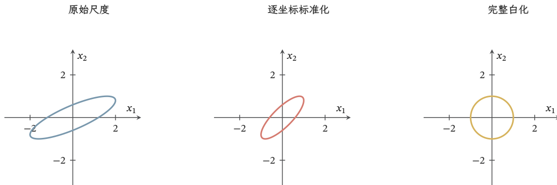
图 14.4 以 \mathbf{C} = \begin{pmatrix} 4 & 1.6 \\ 1.6 & 1 \end{pmatrix} 构造二维协方差椭圆。左图为原尺度，中图分别除以各坐标标准差，边际尺度相同但相关系数仍为 0.8；右图用精确逆平方根白化后成为圆。曲线是解析示意，不是抽样散点或实验结果；忽略稳定项且不加入可学习仿射。
