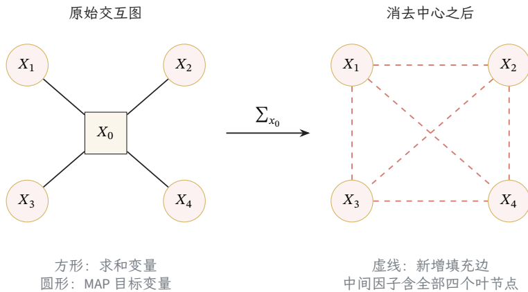
图 20.3 边缘 MAP 引起的填充，图中 k=4 。左侧中心 X_0 要求和，四个叶节点要共同最大化；右侧消去中心后，叶节点由虚线填充边连成团。若是 MPE，则可以先消叶节点，此时不产生这些填充边。
