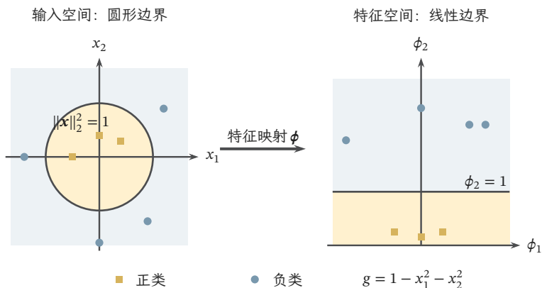
图 1.1 非线性边界在特征映射前后的对应，两个面板的坐标均无量纲。正类方点为 (-0.5, 0) 、 (0, 0.4) 、 (0.4, 0.3) ，负类圆点为 (-1.4, 0) 、 (0, -1.6) 、 (1.2, 0.9) 、 (0.9, -1.2) 。右图逐点使用 \phi_1 = x_1 、 \phi_2 = x_1^2 + x_2^2 ；水平线 \phi_2 = 1 对应左图半径为 1 的圆。数据与边界均为教学构造。
