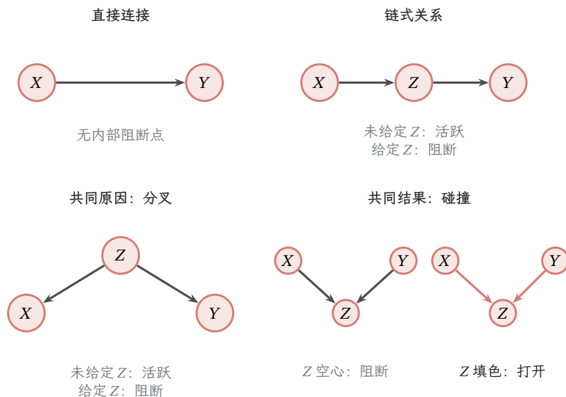
图 17.3 四种基本关系及给定中间节点前后的变化。链和分叉在同一小图中对照状态；碰撞关系拆成两列，空心 Z 表示未观测时阻断，红色填充 Z 表示给定后打开。活跃表示这条路径不再保证两端独立，并不保证任意参数下都实际相关。在更大的图中，碰撞节点的后代被给定也能打开该位置；直接连接则没有内部阻断点。
