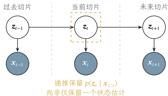
图 28.1 状态空间模型的有限展开。空心节点表示潜状态, 填充节点表示观测; 竖直虚线区分时间切片。消去过去后, 当前潜状态上的后验分布是继续预测所需的信息, 图中箭头表示生成依赖而不是推断只能进行的方向。
