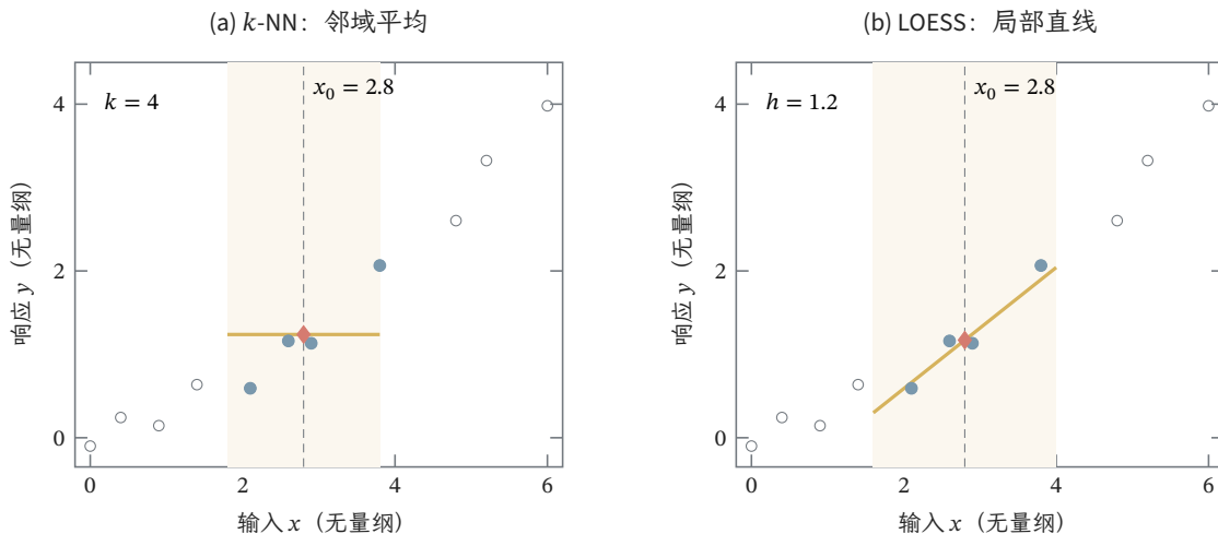
图 2.4 同一查询点上的邻域平均与局部线性拟合。横、纵轴均无量纲，所有点均为构造样本；空心点为未使用样本，蓝色实心点为本次使用的四个样本，菱形为 x_0 = 2.8 处的预测。左图取 k = 4 、等权平均，预测约为 1.238；右图取 h = 1.2 与三立方距离权重，不做残差重加权，局部线性预测约为 1.171。浅色带标出各自的邻域，两图同时改变了局部函数形式和权重，不据此断言某种方法总是更准。
