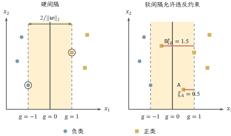
图 3.2 硬间隔与软间隔的教学示意，坐标无量纲。蓝圆为负类，赭方为正类；两个面板都给定 \mathbf{w} = (1, 0)^\top 、 b = -2 ，黑色实线为决策边界 g = 0 ，蓝色虚线为间隔边界 g = \pm 1 。单侧规范间隔为 1/\|\mathbf{w}\|_2 = 1 ，两虚线总宽为 2/\|\mathbf{w}\|_2 = 2 ；左图圈出间隔上的样本。右图红色线段直接标出松弛量：A 位于 x_1 = 2.5 ，正确分类但在间隔内， \xi_A = 0.5 ；B 位于 x_1 = 1.5 ，已被错分， \xi_B = 1.5 。右图仅说明给定分界面下的最小松弛量，并非优化后的 SVM 最优解。
