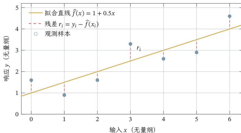
图 2.1 一维 OLS 与响应残差。七个构造样本的最小二乘直线为 \hat{f}(x) = 1 + 0.5x ；蓝色实心点表示观测，黄色实线表示预测，红色竖虚线表示 r_i = y_i - \hat{f}(x_i) 。横、纵轴均为无量纲教学变量。
