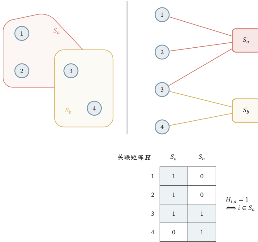
图 11.8 超边及其关联表示。左侧一条超边 S_a 连接节点 1、2、3，另一条超边 S_b 连接节点 3、4。右侧将超边画成方框，以连线表示参与关系；下方 4 \times 2 关联矩阵 H 用同一组 0/1 关系把“集合、二部图、矩阵”对应起来。方框是关系状态，不是新增的原始参与者。
