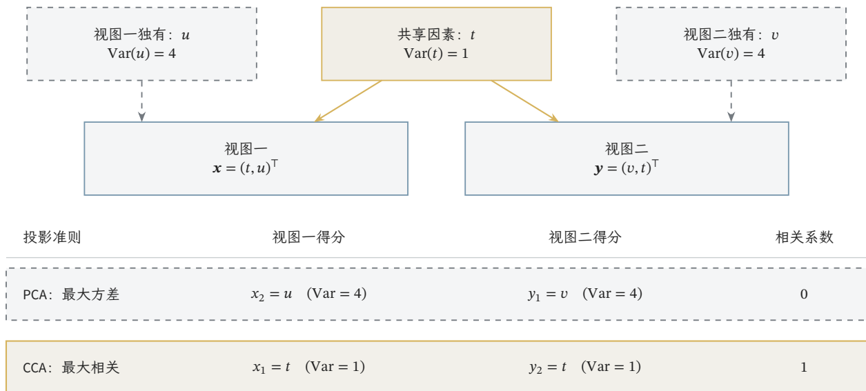
图 5.2 CCA 提取共有变化的构造例子。设 t, u, v 相互独立且均值为零，方差依次为 1, 4, 4；两视图为 \mathbf{x} = (t, u)^\top 和 \mathbf{y} = (v, t)^\top 。实线连接共享因素，虚线连接各视图独有因素。各保留一维时，PCA 选择 u, v ，CCA 选择 t, t ，对应相关系数分别为 0 和 1。箭头表示坐标构造关系，图中结论针对给定总体，不是样本拟合结果。
