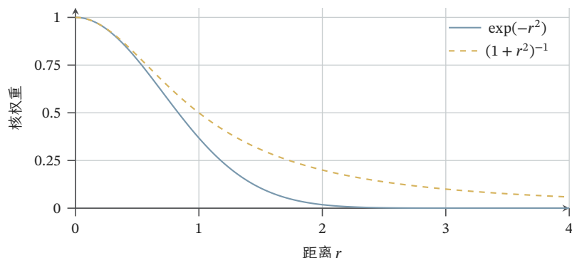
图 5.9 高斯核 \exp(-r^2) 与 Cauchy 形核 1/(1+r^2) 的尾部。横轴 r 为无量纲距离, 纵轴为未归一化核值, 非概率密度、非实验结果; 尾部形状本身不保证嵌入保真。
