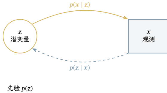
图 5.10 概率生成与后验推断的结构示意。实线表示 \mathbf{z} \rightarrow \mathbf{x} 的生成方向; 虚线表示 \mathbf{x} \rightarrow \mathbf{z} 的后验推断, 不是额外的生成依赖。图中节点与箭头只说明变量角色和条件关系, 不表示实测数据、网络层数或计算流程; 噪声描述观测对信号的偏离, 不是新增的潜变量维数。
