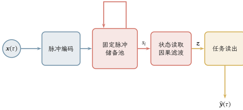
图 10.7 LSM 的输入、动态与读出。输入编码驱动固定的循环脉冲储备池，回路活动形成脉冲列 s_i(\tau) ；因果滤波将这些活动变成当前可读特征 \mathbf{z}(\tau) ，任务读出再映射为预测。红色反馈表示回路动态，黄色表示特征到预测的映射。此处只训练任务读出，脉冲编码、回路参数与滤波核按约定固定。
