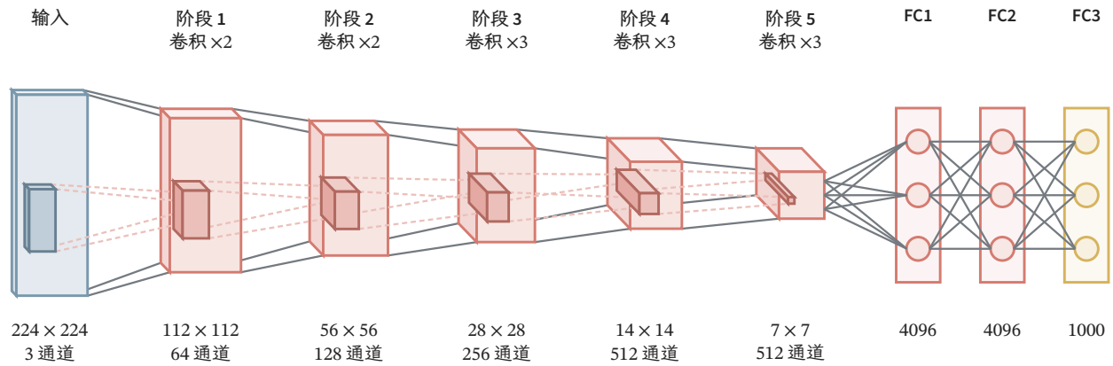
图 9.16 VGG-16 的五阶段卷积主体与全连接尾部。每个阶段内的 3 \times 3 卷积保持空间尺寸，阶段末池化减半；图中主体特征标注为池化后的形状。13 个卷积层与三个全连接层组成 16 个带权重的层。每个卷积阶段合并展示其中的卷积堆叠与末端池化，平面神经元框表示全连接层；层下方分别标出空间尺寸与通道数。
