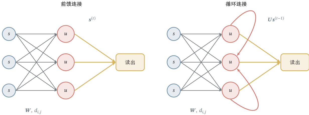
图 13.4 脉冲前馈网络与循环网络的构造性比较。圆内 u 表示各单元保存膜电位，箭头传递离散发放，黄色方框为输出读出。左图只保留层间前馈连接；右图增加使用上一时间步脉冲的循环边 U 。边还可带权重与传播延迟，图中只标出一条代表连接。神经元数和连边用于说明结构，不对应训练模型。
