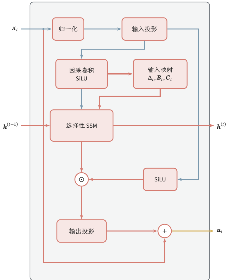
图 10.15 原始 Mamba 模块的主要计算路径。红色粗分支强调选择性的来源：短卷积后的输入特征生成 \Delta_t, B_t, C_t ，并据此调节 SSM 更新；另一路特征调制 SSM 输出，底部直达线完成跨层残差。 u_t 是模块输出，任务预测由后续网络读出。图中省略短卷积缓存、批次维和跨通道广播细节。
