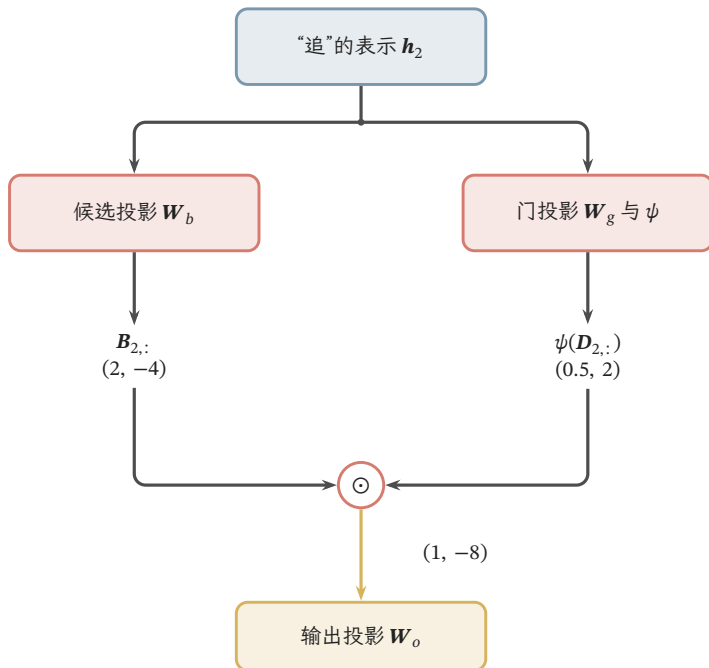
图 12.24 门控前馈层对“追”的一次逐位置计算。候选特征 (2, -4) 与激活后的调制量 (0.5, 2) 相乘为 (1, -8)，再经输出投影恢复隐藏宽度。数值是教学假设；大于 1 的调制量适用于 GEGLU 或 SwiGLU 的解释，GLU 的 Sigmoid 门则限制在 0 与 1 之间。猫、追、狗使用同一套参数分别计算，不发生跨位置读取。
