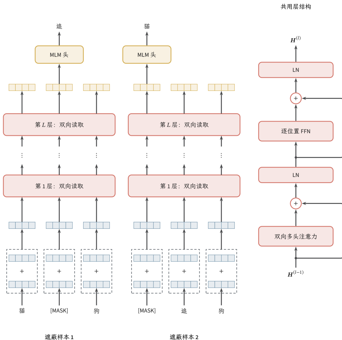
图 12.11 RoBERTa 对“猫追狗”的两次动态遮蔽。两组输入分别前向，使用同一套骨干参数，各长条只在所属样本内部进行双向读取；两次 MLM 监督分别恢复“追”和“猫”。词元与位置嵌入相加，中间层省略，右侧展开共用的 Post-LN 层。格条只示意特征维；[MASK] 采用教学记号，省略实际特殊词元、输入归一化与 Dropout。训练不使用 NSP。参考 Bishop 与 Bishop (2024) 图 12.18 的布局重绘，训练差异依据 Liu 等 (2019)。
