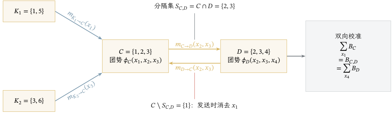
图 21.4 团间消息的组成与双向校准。蓝色箭头是 C 收到的入站消息，团势与这些消息相乘后，对 C \setminus S_{C,D} = \{1\} 中的 x_1 求和，得到定义在分隔集 \{2, 3\} 上的 m_{C \rightarrow D} ；发送时排除接收方 D 的入站消息。黄色双向箭头分别汇总树边两侧的贡献，收集与分发都完成后，两个团消去非共享变量所得的表均等于分隔集势 B_{C,D} 。
