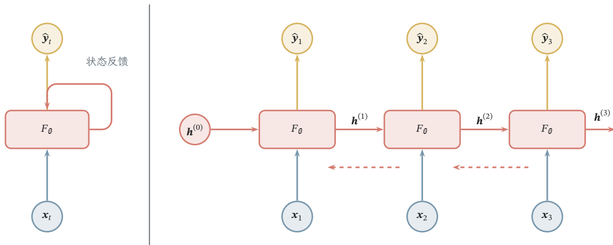
图 10.1 状态递推的紧凑表示与时间展开。蓝色节点提供当前输入，红色方框计算隐状态，黄色节点读出预测。展开图中的 F_\theta 是同一个更新函数的多次调用，参数共享而状态值不同。红色虚线示意较晚损失沿状态依赖回传梯度；图中只画三个更新步。
