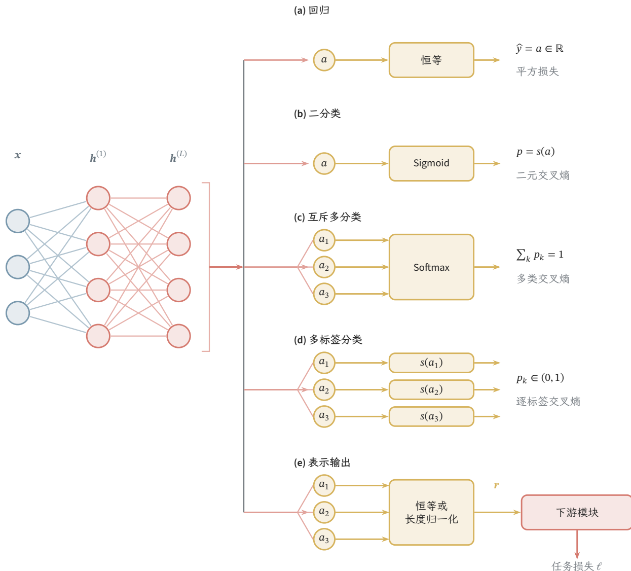
图 8.9 共同的前馈结构与五种可替换的输出头。左侧蓝色输入单元经红色隐藏单元形成 \mathbf{h}^{(L)} ；汇合线传递整组隐藏坐标，不执行求和。右侧黄色单元产生各任务自己的原始得分，每个单元都读取全部隐藏坐标，并具有独立的输出权重与偏置。(a)、(b) 只需一个得分；(c) 联合归一化，(d) 逐坐标变换；(e) 产生由下游任务约束的表示。向量头仅画三个坐标示意，实际维度由任务决定。右侧文字区分预测量与训练目标，隐藏激活无需与输出变换相同。
