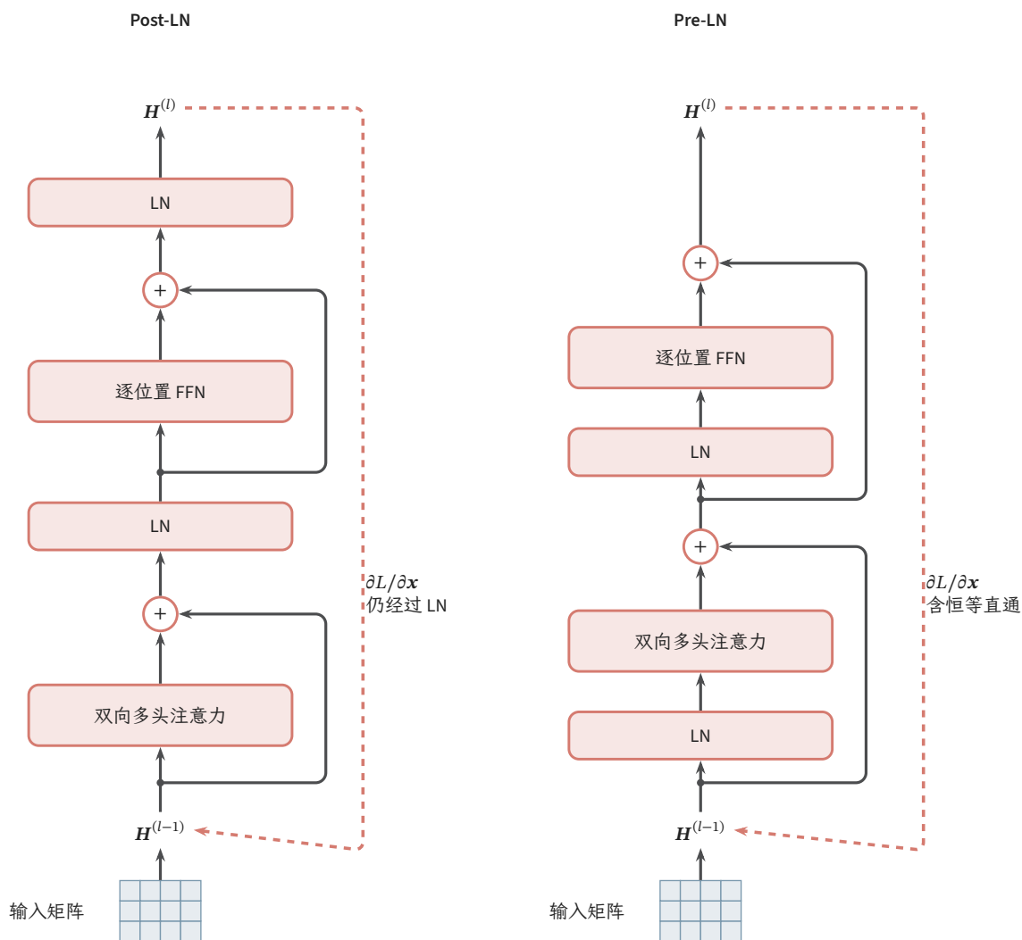
图 12.7 Post-LN 与 Pre-LN 编码器块的计算次序。底部矩阵的三行对应“猫/追/狗”，列示意特征维度，格子数不代表实际宽度。自注意力在行间交换信息，FFN 分别变换各行；圆形 + 表示逐元素残差相加。红色虚线概括反向梯度路径：Post-LN 的层间路径仍经过 LN，Pre-LN 则包含沿残差支路的恒等直通。省略 Dropout 与 Pre-LN 堆叠末尾的归一化。
