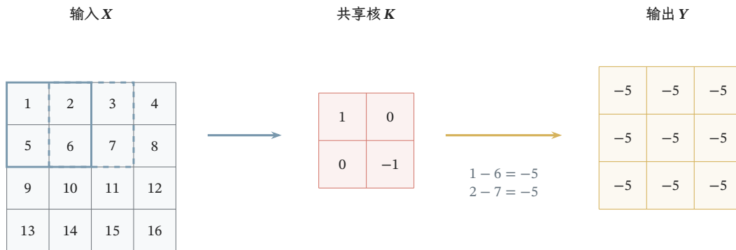
图 9.2 共享核在二维矩阵上滑动的教学例子。蓝色实线和虚线分别框出相邻的两个 2 \times 2 输入窗口，红色矩阵为不翻转的核，黄色矩阵为互相关输出。每个输出计算窗口左上数值减去右下数值，因此均为 -5；两个位置使用同一组权重。
