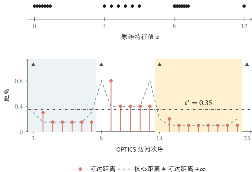
图 4.4 固定一维教学数据上的 OPTICS 排序，取 \text{MinPts} = 3 (含自身)、 \varepsilon_{\max} = 1.1 。三组样本的间距分别为 0.15、0.4、0.1，另有 x = 12 的孤立点。红色竖棒为可达距离，蓝色虚线为核心距离；蓝、黄底色标出两个低谷。无穷可达距离用顶部三角形表示，不能按其显示高度作数值比较；水平点划线展示阈值切割在本例中提取哪些低谷。
