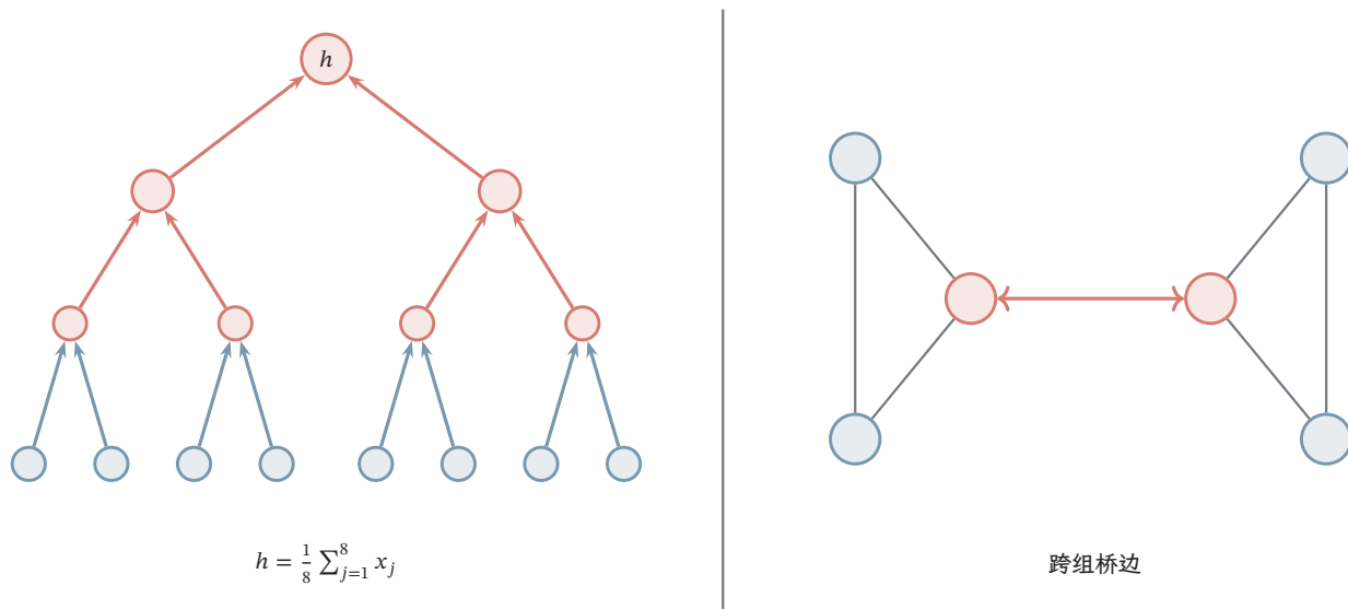
图 11.10 两种信息汇聚瓶颈。左侧八个叶子经三层平均进入一个根状态，每个叶子的影响系数为 1/8 ；右侧两组节点的跨组信息必须经过一条桥边。红色表示承担汇聚或跨组传递的状态，蓝色表示外围输入。图不要求所有状态相同，强调的是大量信息必须经过较少的表示通路。
