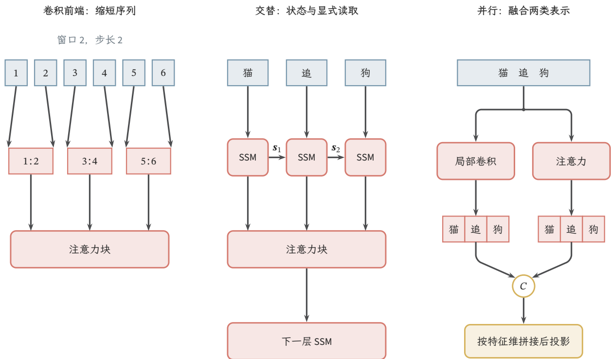
图 12.27 三种混合结构改变的是不同环节。左图以窗口 2、步长 2 的卷积前端将 6 个输入位置变成 3 个特征位置，再交给注意力；中图对猫、追、狗递推状态，并将各位置输出交给注意力层，随后继续交替；右图对同一序列并行计算局部卷积和注意力， C 表示按特征维拼接，再经投影融合。并行分支采用保持长度的位置对齐设置，所有分支还需满足任务的因果约束。
