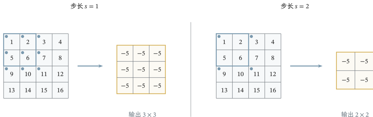
图 9.4 跨步改变输出位置的密度。输入、 2 \times 2 核和无填充设置保持不变，只将高、宽步长从一改为二。每个蓝色圆点标记一个窗口的左上起点，起点分别形成 3 \times 3 和 2 \times 2 的网格；实线框只画出第一个窗口。该教学矩阵的所有窗口都得到 -5 ，输出值相同不表示读取的位置相同。
