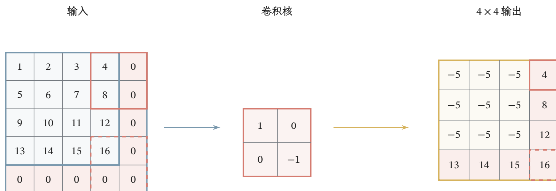
图 9.3 不对称零填充与边界输出。蓝色框内是原 4 \times 4 输入，浅红色区域是右侧、下侧各新增的一列、一行零。红色实线窗口产生右上输出 4，虚线窗口产生右下输出 16，输出矩阵中用相同线型标记对应位置。核为 (1, 0; 0, -1) ，步长一、空洞率一，计算采用互相关。
