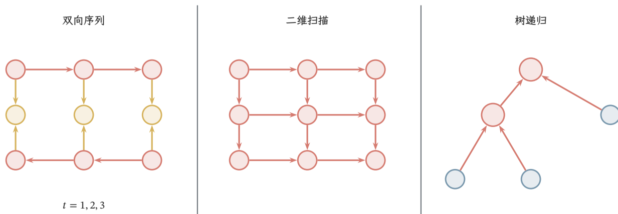
图 10.17 状态依赖拓扑。左图在同一输入位置组合正向与反向状态；中图由上方、左方前驱形成二维状态，箭头给出一个扫描方向；右图由叶节点向父节点组合子结构。红色表示隐藏计算，黄色节点表示组合读出。图中只表达依赖关系；不同方向、位置或孩子组合是否共享参数，需要由具体模型说明。
