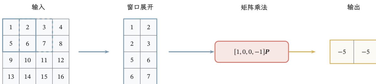
图 9.8 局部点积如何成为矩阵乘法。图中只取两个相邻窗口，按核行、核列的顺序展平成 \mathbf{P} 的两列；核按相同顺序展平成一行。矩阵乘法同时得到这两个窗口的输出，完整计算包含九列。这里画的是代数上的窗口矩阵，是否实际复制全部数值由工程实现决定。
