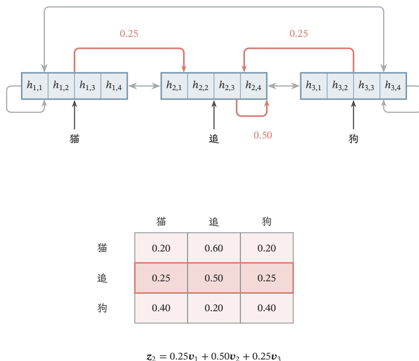
图 12.3 同一序列“猫/追/狗”上的自注意力。每个词元上方的四格条直接表示输入向量的特征坐标；这同一组表示分别投影为查询、键和值。灰色双向线表示两个位置可以互相读取，自环表示读取自身，两个方向的权重不必相等。红色箭头从值的来源指向“追”的查询位置，对应下方权重矩阵框出的第2行。三个查询各自归一化，图中未另画输出序列；数值为教学设定。
