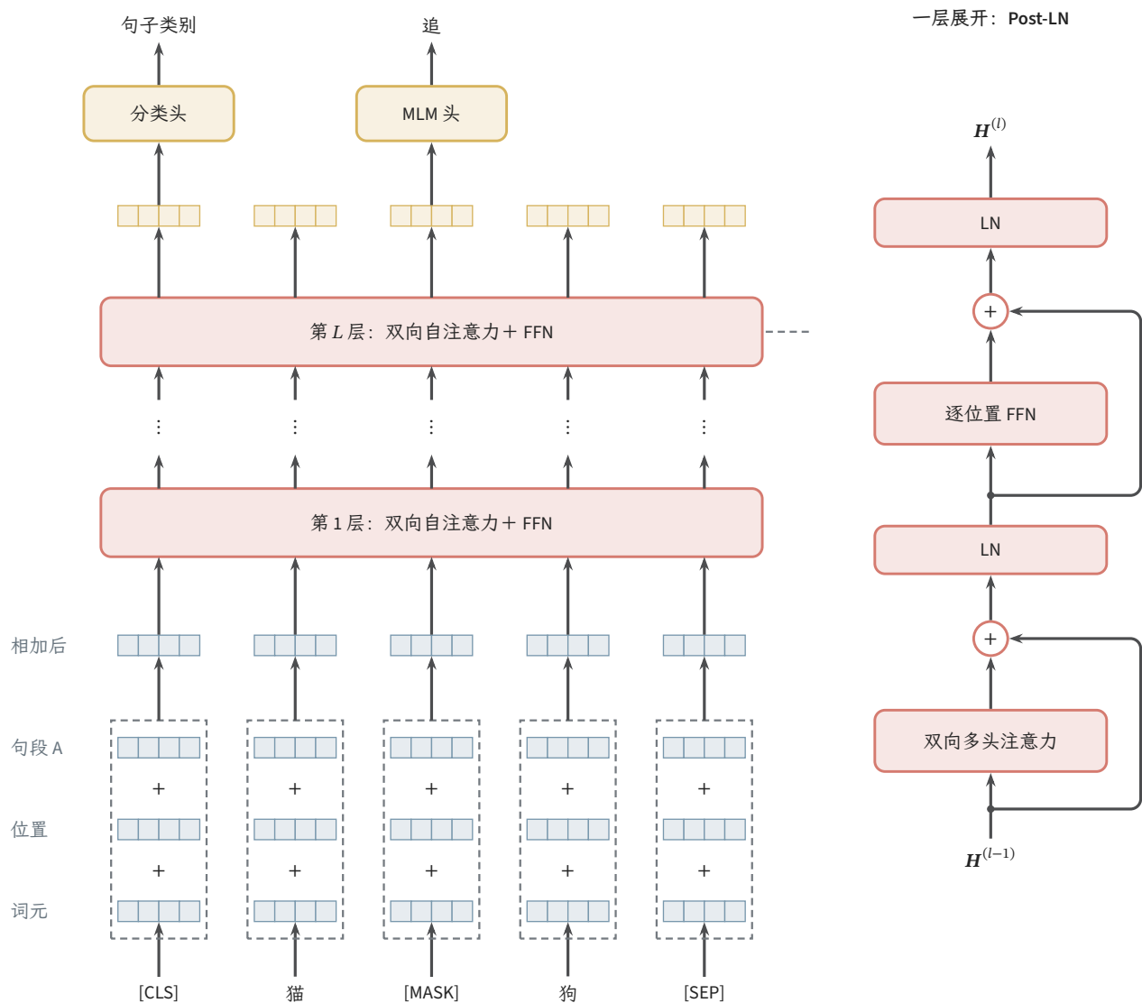
图 12.10 BERT 的双向编码器与预测位置。每列的词元、位置、句段嵌入逐元素相加，本例同属句段 A；向量格条只示意特征维。每个长条是一整层双向自注意力与 FFN 计算，能够在所有有效词元之间交换信息，中间层省略。MLM 头在遮蔽位置恢复“追”，CLS 分类头用于任务适配；两者不要求同时使用。右侧展开一层的 Post-LN 与残差，省略输入归一化、Dropout 与 NSP 头。参考 Bishop 与 Bishop (2024) 图 12.18 的整序列布局重绘，输入与训练目标依据 Devlin 等 (2019)。
