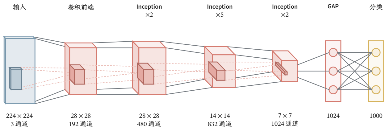
图 9.19 经典 GoogLeNet 的主分类路径。卷积前端把 224 \times 224 输入变成 28 \times 28 \times 192 ；两个、五个、两个 Inception 模块组成三个阶段，阶段间池化改变空间尺度。各阶段末的通道数为 480、832 和 1024，全局平均池化后接 1000 类分类器。辅助分类分支及模块内部细节省略，模块内部结构见图 9.18。
