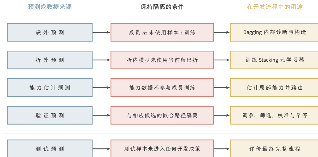
图 6.11 集成学习中的数据隔离与预测职责。每一行从预测或数据来源出发，经由相应隔离条件到达允许的用途；水平分隔线表示训练、调参、筛选、校准和部署规则已经冻结。测试数据位于分隔线之后，不能沿开发路径回流。
