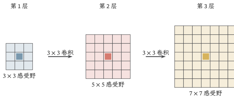
图 9.17 三个步长一、无空洞的 3 \times 3 卷积逐层扩大几何感受野。彩色方格表示一个高层位置在原输入上可能读取的范围，中心实色格只用于对齐位置；跨度依次为 3, 5, 7。图没有计入池化、跨位置归一化或边界填充造成的额外依赖。
