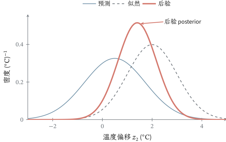
图 28.3 标量 Kalman 更新的可复算密度。蓝色实线为预测 \mathcal{N}(0.5, 1.5) ，灰色虚线为对状态归一化后的似然 \mathcal{N}(2, 1) ，红色粗线为后验 \mathcal{N}(1.4, 0.6) ，并由曲线旁的引线直接标出。横轴是温度偏移，纵轴是密度；本例观测矩阵为 1，似然才可直接画成同一坐标下的归一化密度。
