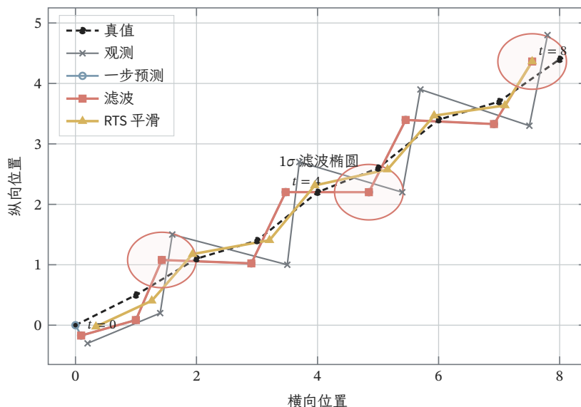
图 28.2 二维 Kalman 滤波与 RTS 平滑的可复算轨迹。黑色虚线是人工真值，灰叉是固定观测，蓝色空心点为观测前的一步预测，红色方点为在线滤波均值，黄色三角为使用全部九次观测的平滑均值。红色半透明椭圆分别给出 t = 2, 5, 8 处滤波后验的逐坐标 1 倍标准差区域；末时刻没有未来观测，滤波与平滑重合。模型参数和全部坐标固定写在图源中，不表示任意运动都适合随机游走模型。
