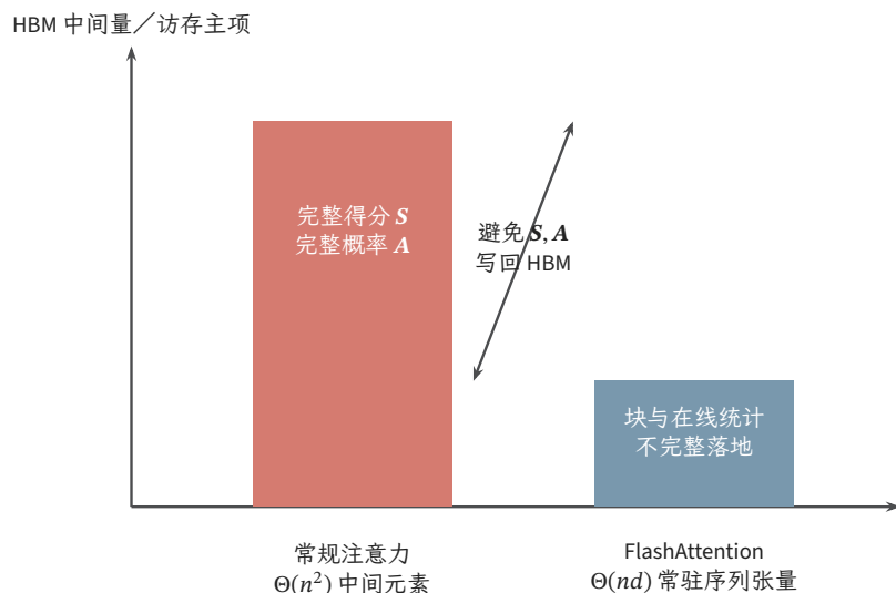
图 12.21 常规实现与 FlashAttention 的 HBM 中间量对比。柱高只表示量级差异，不是硬件实测：常规路径显式保存两个 n \times n 矩阵，FlashAttention 避免它们完整落地，只保留 \Theta(nd) 规模的序列张量及分块统计。它仍计算稠密位置对，算术量没有因此从平方降为线性；真实 I/O 还依赖片上容量和块大小。
