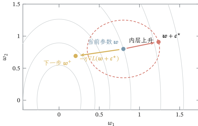
图 15.3 SAM 一次近似更新的几何过程。灰线为教学目标 L(\mathbf{w}) = (4w_1^2 + w_2^2)/2 的等高线，红色虚线是以当前参数为中心、半径 \rho = 0.45 的扰动邻域。红箭头沿当前梯度的一阶近似到达边界高损失点，黄色箭头使用该扰动点的梯度更新原参数。图示解释两次梯度读取的位置，不表示 SAM 必然找到内层精确最大值或必然改善泛化。
