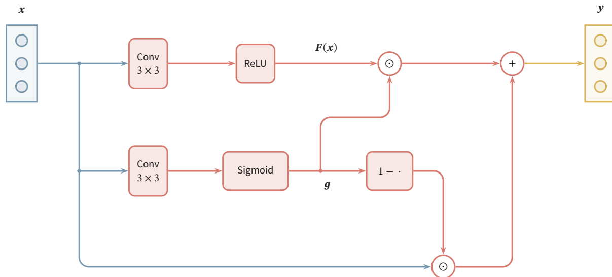
图 9.21 同形状卷积 Highway 模块。上方卷积与 ReLU 产生 F(x) ，门路径经卷积与 Sigmoid 产生 g ，蓝色保留路径传递原输入；两个 \odot 节点分别计算 g \odot F(x) 和 (1-g) \odot x ，再由 + 节点相加。所有特征与门具有同一空间、通道形状，圆角方框表示各条路径的处理算子。
