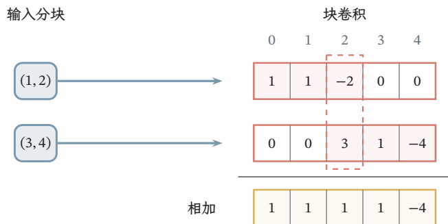
图 9.11 重叠相加的数值例子。输入在原位置零和二分别开始两个长度二的块，块内补零后计算与 (1, -1) 的完整卷积，恢复到图上的五个全局输出位置。红色区域表示该块可能产生贡献的位置，区域外记为零。虚线框内的两项贡献相加为一，最终结果与不分块的线性卷积相同。
