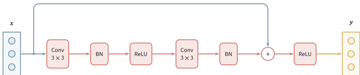
图 9.20 残差基本模块中的逐层变换与恒等旁路。主分支依次经过 3 \times 3 卷积、BN、ReLU 及第二个 3 \times 3 卷积、BN，再与直接传来的输入逐元素相加并激活。两次卷积均保持 32 \times 32 \times 64 形状，上方蓝色旁路跳过主分支的变换。圆角方框表示算子，圆形加号节点表示逐元素相加；改变尺度或通道时，旁路需要投影。
