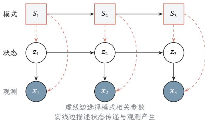
图 28.4 切换线性动态系统的三层展开。方形节点为离散模式，空心圆为连续状态，填充圆为观测。给定完整模式路径后，连续部分可用 Kalman 递推；只给定当前模式不足以合并具有不同历史的所有高斯分量。
