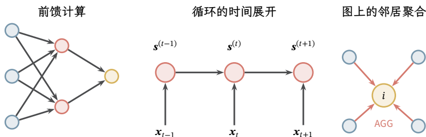
图 7.8 三种不同对象的结构示意。左侧是前馈计算中的单元依赖；中间是循环更新的时间展开，三个更新位置共享同一组状态更新参数；右侧显式画出图神经网络的一次邻居聚合，蓝色邻居沿箭头向中心节点 i 提供消息。输入关系可以有环，但一次同步更新的计算依赖仍按层推进。
