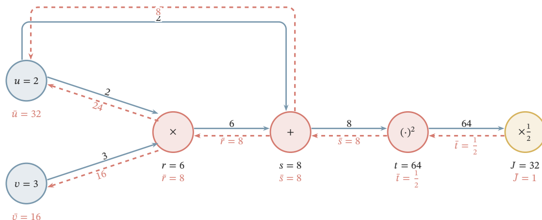
图 8.12 同一算子图上的后向模式。节点位置与前向模式相同，实线及其黑色标注保留前向传递值，红色虚线及其标注从 J = 1 开始回传导数贡献；每个算子下方两行分别给出输出值和伴随值。输入 u 收到经乘法传来的 24 和直接经加法传来的 8，累加为 32；输入 v 得到 16。一次后向遍历同时得到两个偏导。
