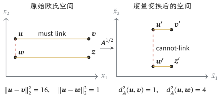
图 4.10 度量如何改变成对关系的几何表达。四点为 \mathbf{u} = (-2, 0.5) 、 \mathbf{v} = (2, 0.5) 、 \mathbf{w} = (-2, -0.5) 、 \mathbf{z} = (2, -0.5) 。实线连接 must-link 对，虚线连接 cannot-link 对。这里人为设定 \mathbf{A} = \text{diag}(1/16, 4) ；右图的距离等于左图的 Mahalanobis 距离，不表示一次真实训练的结果。
