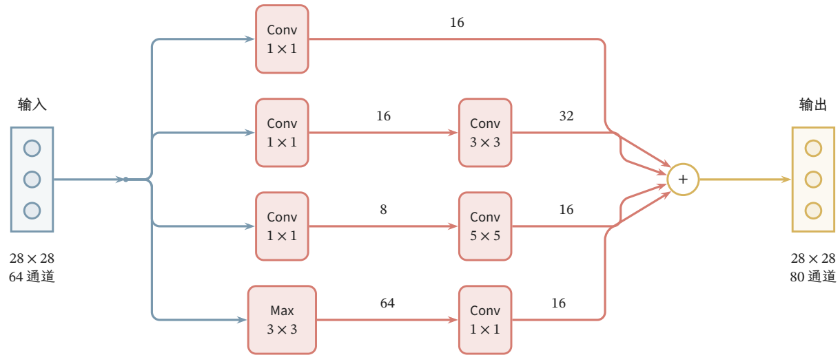
图 9.18 一个 Inception 模块的四分支教学配置。输入为 28 \times 28 \times 64 ；四条分支分别输出 16、32、16、16 个通道，保持同一空间尺度，拼接得到 28 \times 28 \times 80 。中间的逐点卷积先压缩通道，最大池化采用步长一及 same 填充。圆角方框表示处理算子，Max 为最大池化，线路上的数字为通道数；圆形 + 表示沿通道拼接，四条路径实际并行，激活省略。
