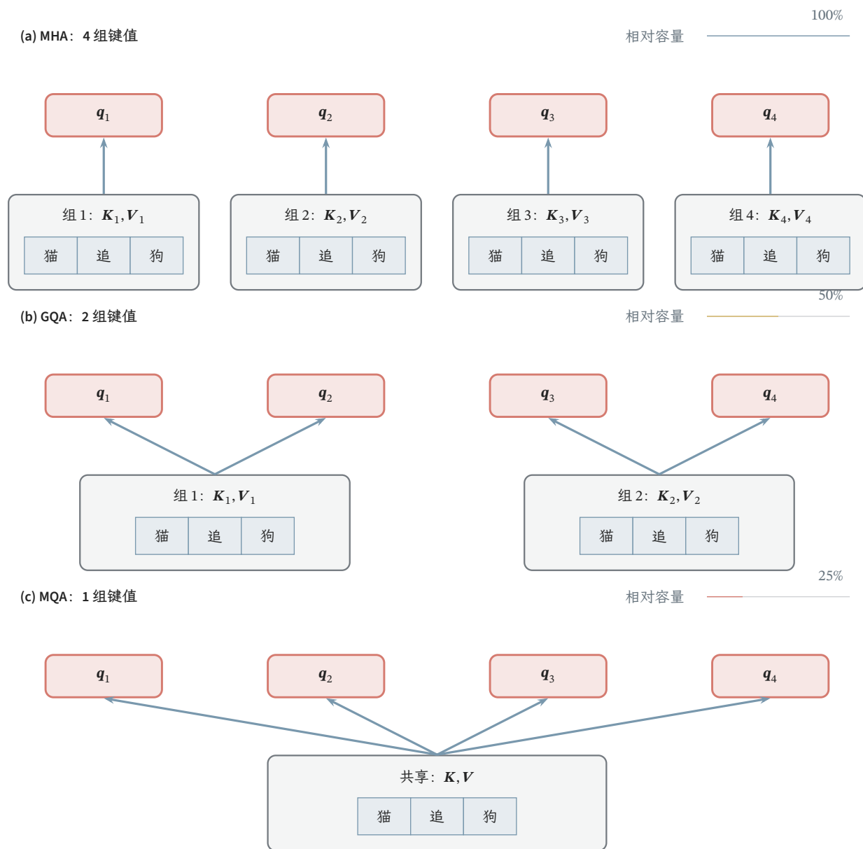
图 12.22 相同历史序列在 MHA、GQA 和 MQA 中的缓存布局。每个带词元名的小格代表该位置在一组投影下的一对键和值；大框是一整组历史缓存，箭头指向读取它的查询头。4 个查询头分别使用 4 组、2 组或 1 组键值时，缓存为 12、6 或 3 对，右上容量条相对于 MHA 依次为 100%、50% 和 25%。共享发生在键值表示及其存储上，各查询头仍独立计算注意力权重。图只计一层的一条序列，不含当前新位置追加的缓存。
