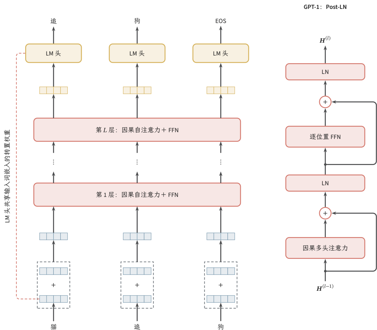
图 12.12 GPT 的因果网络与下一词元监督。每列的词元与位置嵌入相加后，经过整序列网络层，再由 LM 头预测下一词元；“追”所在列只能读取“猫、追”，对应标签为“狗”。左侧红色虚线表示 LM 词表投影与输入词嵌入共享转置权重。右侧展开 GPT-1 的 Post-LN 层；GPT-2 与 GPT-3 改用 Pre-LN 并在堆叠末尾归一化。格条只示意特征维，省略 Dropout 与 KV 缓存。
