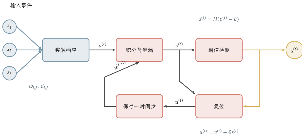
图13.2 离散脉冲神经元的计算结构。蓝色输入事件经带权突触形成输入增量 a^{(t)} ，红色模块完成积分、泄漏、阈值检测和复位，黄色路径输出 s^{(t)} 。下方反馈保存复位后电位 u^{(t)} ，供下一步使用； v^{(t)} 为复位前电位。图表示本章的更新次序，不表示细胞的解剖结构；突触自身也可保存状态，见式(13.8)。
