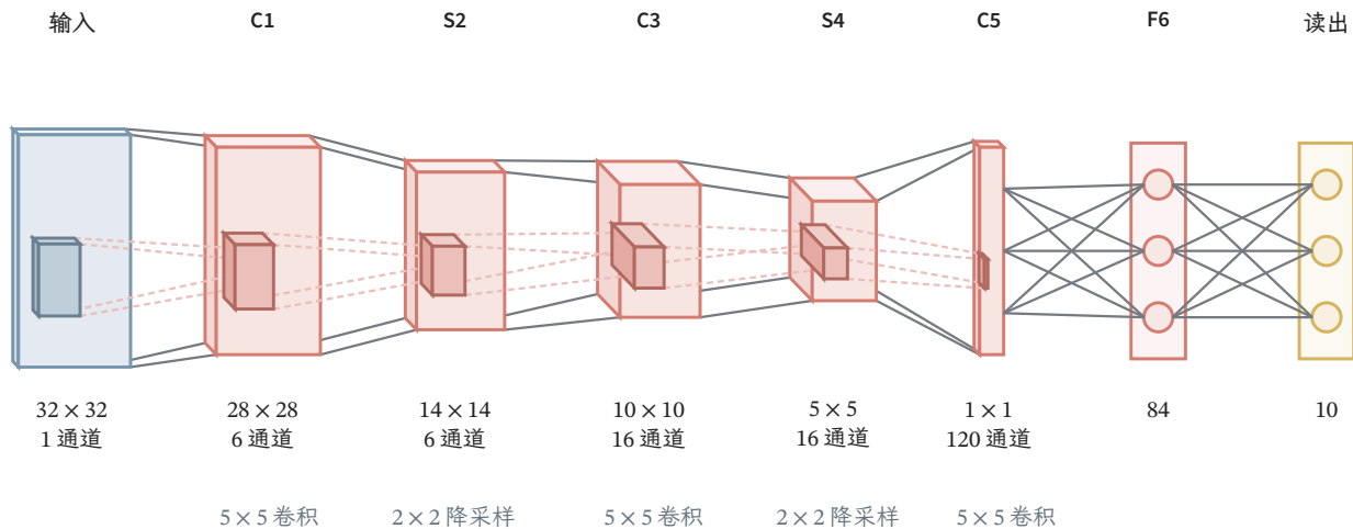
图 9.14 LeNet-5 的层次结构。C1、C3 和 C5 为卷积层，S2、S4 为原网络可学习的降采样层，F6 为全连接层；原始十类读出采用欧氏径向基函数单元。长方体和局部映射均为示意，标签给出实际形状。C3 的部分通道连接与降采样层的可学习参数未在图中逐条展开。
