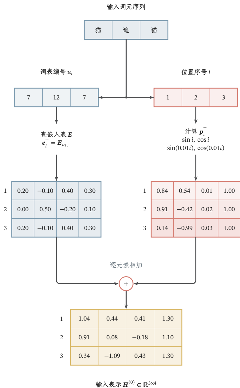
图 12.1 序列“猫／追／猫”的输入构造。左路用词元编号查嵌入表，右路把位置序号代入正弦、余弦函数，两组 3 \times 4 表示再逐元素相加。三个矩阵的行均按输入位置排列，每格是一个特征值。两个“猫”的内容相同、位置不同，输出的第 1 行与第 3 行因而不同。词元编号和嵌入为教学设定；位置向量按弧度计算，数值保留两位小数，最后一列看似相同是舍入所致。
