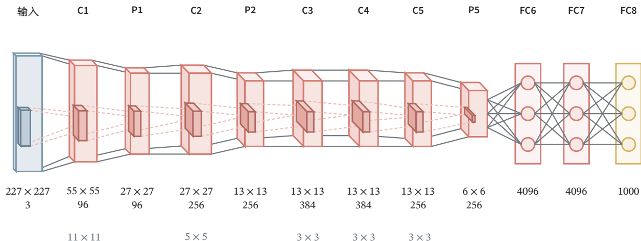
图 9.15 AlexNet 的五个卷积层与三个全连接层。全部主路径在一行展开，卷积层、最大池化层与全连接层分别绘出；最后一次池化的输出展平为 9216 维。各层下方给出空间尺寸和通道数，C 表示卷积，P 表示池化。此图采用 227 输入及正文给定的填充约定，省略局部响应归一化、Dropout 和原始双 GPU 的分组细节。
