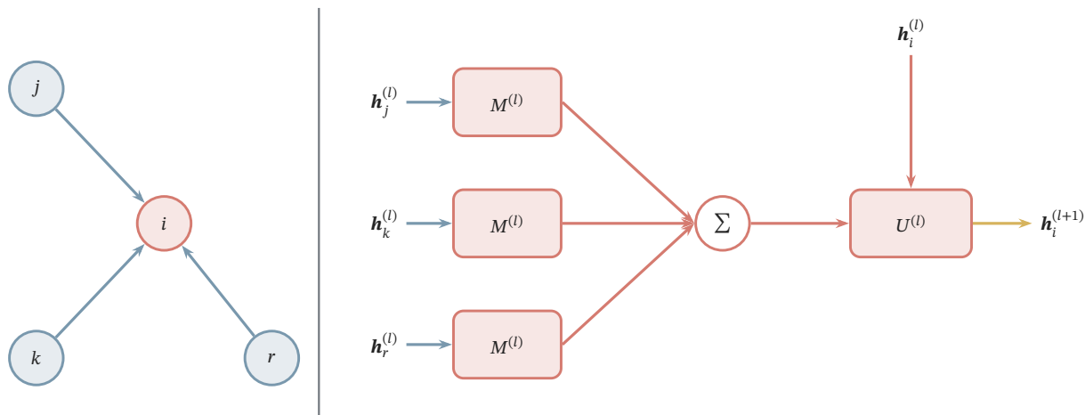
图 11.1 节点 i 的一轮消息传递。左侧蓝色节点 j, k, r 与红色节点 i 相连, 右侧分别计算三条消息, 再求和并更新 i 。上方路径把 i 的旧表示送入更新函数。图中省略消息函数对接收节点和边属性的额外输入, 所有节点使用相同的消息与更新规则。
