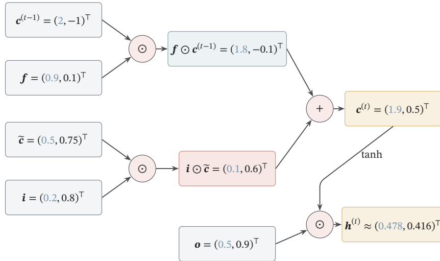
图 10.9 二维 LSTM 的一步数值走查。蓝色与深灰数字分别表示两个通道；保留分支计算 f \odot c^{(t-1)} ，写入分支计算 i \odot \tilde{c} ，二者相加得到新记忆，再经 o \odot \tanh(c^{(t)}) 得到隐藏状态。所有数值均由图内向量逐坐标计算，第二通道结果为 0.9 \tanh(0.5) \approx 0.416 。图中暂把门值和候选值视为已知，不展开它们的仿射计算。
