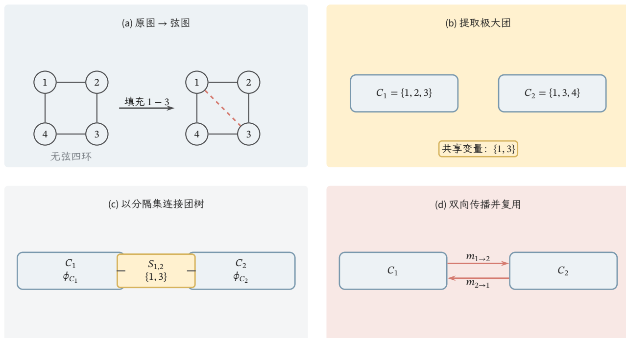
图 21.2 团树编译与传播总览。四个面板按两行两列展开：四环先通过填充边 1-3 变为弦图，再提取极大团 C_1 = \{1, 2, 3\} 与 C_2 = \{1, 3, 4\} ；金色分隔集 S_{1,2} = \{1, 3\} 明确标出两团共享状态，最后用双向消息汇总树边两侧的贡献。团树的节点和边属于计算结构，不是把原变量图改画成树。
