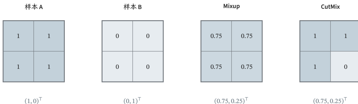
图 15.1 构造的两类 2 \times 2 输入及其混合。样本 A 各位置为 1，目标为 (1, 0)^T ；样本 B 各位置为 0，目标为 (0, 1)^T 。Mixup 取 \lambda = 0.75 ，各位置变为 0.75；CutMix 替换右下位置，保留面积也为 0.75。二者目标均为 (0.75, 0.25)^T ，但空间组织不同。这是机制示例，不代表真实图像类别。
