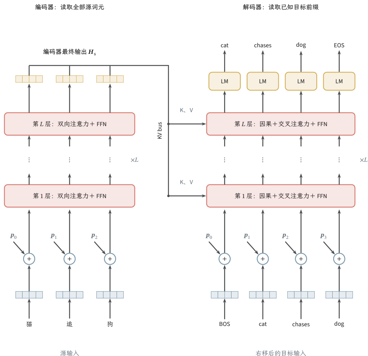
图 12.8 将“猫／追／狗”翻译为“cat / chases / dog”的整网结构。每个长条表示作用于整段序列的一层， \times L 表示重复堆叠；词元列保持位置对应。训练时右移的目标输入分别预测 cat、chases、dog、EOS。左侧最终源表示沿标出的 KV bus 供每个解码器层生成 K、V，Q 来自该层目标路径；不会把某个中间编码层与同编号解码层一一配对。省略层内残差、归一化与 Dropout。
