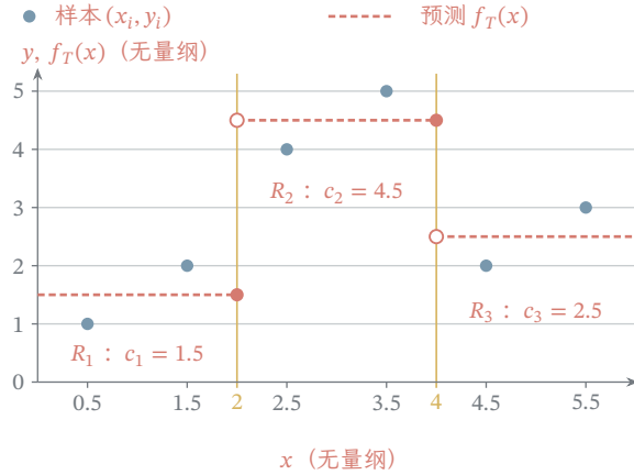
图 2.5 给定阈值树与分段常数预测。六个无量纲教学样本按 x 递增排列；按 x \leq 2 及右分支上的 x \leq 4 划分后，三组响应分别为 (1, 2) 、 (4, 5) 、 (2, 3) ，叶均值为 1.5、4.5、2.5。蓝色点表示样本，红色虚线表示预测，黄色竖线表示阈值；阈值处实心、空心端点区分取与不取该值。右图只显示 0 \leq x \leq 6 ，树结构预先给定。
