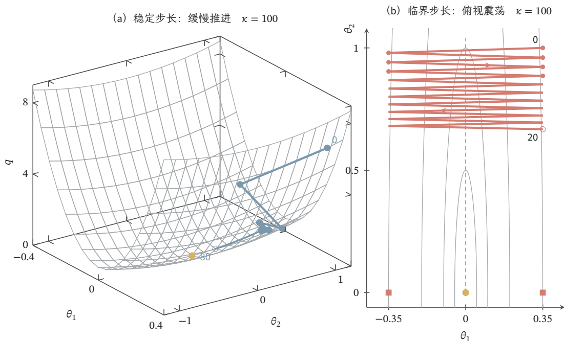
图 14.2 同一病态二次目标在两种步长下的轨迹，标题直接标出条件数 \kappa = a/b = 100 ，黄色点为极小点。(a) 三维图采用稳定步长 0.015，蓝色实心圆标出第 0–8 步，空心圆标出第 80 步；陡方向收缩快，谷底推进慢。(b) 俯视投影采用临界步长 0.02，深红线连接第 0–20 步，实心圆标出第 0–6 步，空心圆为第 20 步；灰线为等高线，竖虚线为谷底。左右摆幅保持 0.35，损失趋向 6.125 而无法达到原点处的 0。
