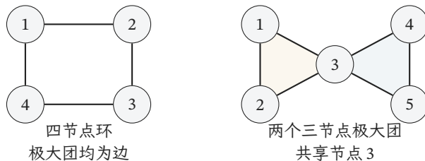
图 18.1 两种无向连接。左图的极大团是四条边，四节点形成环不等于形成团；右图的两个三角形分别是极大团，共享节点 3。线段没有方向，节点编号对应随机变量下标。
