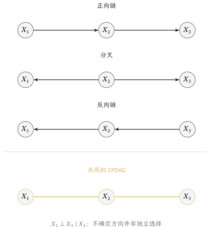
图 25.1 三个无碰撞有向图共享骨架和条件独立关系，以底部的 CPDAG 统一表示。无向边表示方向在类内可变，不表示两个方向同时存在；把两条边同时指向 X_2 会产生新碰撞结构，不是合法补全。
