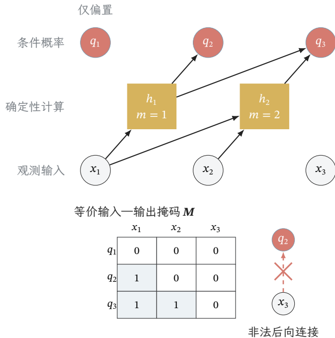
图 26.2 MADE 的合法计算路径。方框表示确定性隐藏计算，圆框表示输入或条件分布输出；输出 q_i 代表 p(X_i = 1 | \mathbf{x}_{<i}) 。下方 3 \times 3 输入—输出掩码直接列出可读关系，蓝格中的 1 表示允许依赖；右侧以 x_3 \rightarrow q_2 为非法后向连接反例。隐藏单元的次序号限定可读前缀，任何 q_i 都不能访问 x_i 或更后的输入。
