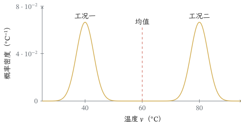
图 16.1 同一个双峰预测分布可以产生均值为 60°C 的点预测。实线为两个等权高斯密度的混合，每个分量的标准差为 3°C；虚线标出均值。点预测没有保留两个高概率区域的位置。
