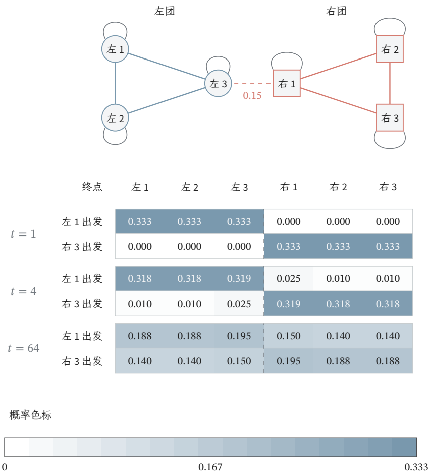
图 5.8 扩散时间与跨团瓶颈。每团三个节点，团内边及所有自环权重为 1，唯一跨团边权重为 0.15。令 \alpha = 0 并按行归一化，热图两行分别表示从左 1、右 3 出发的 P^t 对应行，六列为固定节点顺序；各时刻共用同一连续概率色标。数值由有理数矩阵乘法计算，显示三位小数，舍入后行和可能略偏离 1。64 步仍未充分混合；因图连通且有自环，极限分布均为 \pi^T = (20, 20, 21, 21, 20, 20)/122 。
