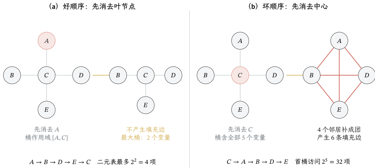
图 20.2 同一因子图上的好、坏消元顺序。所有变量均为二元，原始交互图是五节点星形图。(a) 先消去叶节点时，每个桶最多只含叶与中心两个变量，不产生填充边；(b) 先消去中心时，四个剩余邻居被补成团，第一桶必须枚举五个变量的 2^5 = 32 种配置。红色节点表示当前先消去的变量，红边表示由该步新增的填充边。这里比较的是稠密表格实现的结构代价，不是两种顺序的数值答案。
