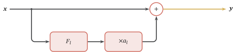
缩放残差
