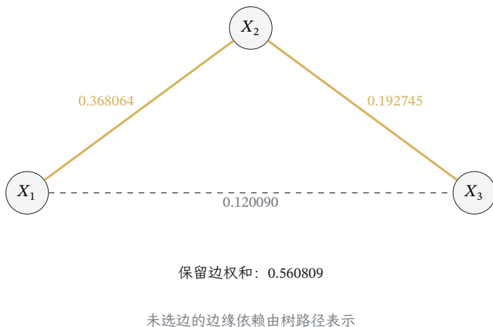
图 25.2 同一计数表产生的三个互信息边权, 单位为 nat。实线为最大权生成树保留的边, 虚线为未选边。树分布在此例恰好复原经验分布, 但算法一般只能给出最佳树近似。
