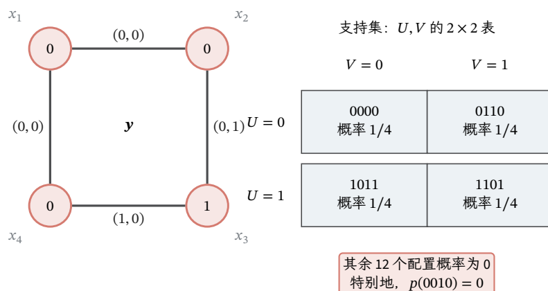
图 18.6 零概率破坏逆向分解的反例。左侧节点给出被禁止配置 \mathbf{y} = (0, 0, 1, 0) , 边旁的每个局部取值对都曾在正概率配置中出现。右侧 2 \times 2 支持表按 (U, V) 列出四个正概率配置, 并直接标出其余 12 个配置概率为 0。若存在非负边势分解, \mathbf{y} 对应的四个边势值就必须都为正, 其乘积也为正, 与 p(\mathbf{y}) = 0 矛盾。
