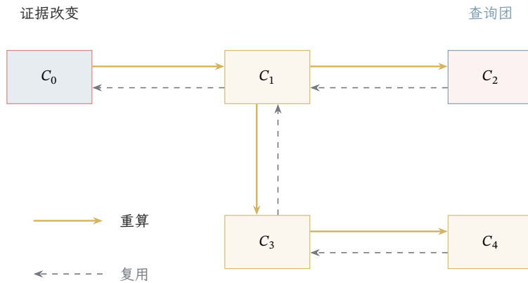
图 21.5 仅 C_0 的局部势改变时的更新方向。实线箭头沿远离 C_0 的方向传播新贡献，反向虚线箭头表示仍可复用的消息；团节点只画名称，具体变量集合须满足运行交集。查询 C_2 时只需更新路径 C_0 - C_1 - C_2 ，其他团的旧边缘不因路径更新而自动全部有效。
