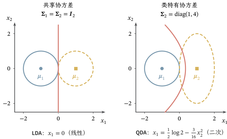
图 3.7 两图均取 \pi_1 = \pi_2 = 1/2 、 \mu_1 = (-1, 0)^T 、 \mu_2 = (1, 0)^T 和 \Sigma_1 = I_2 ，仅第 2 类协方差变化。蓝色圆点和黄色方点为均值，蓝色实线与黄色虚线分别为 \Delta_1 = 1 和 \Delta_2 = 1 的等密度轮廓；不同类的这些轮廓不保证密度值相同。红色粗线按 g_1 = g_2 的解析式绘制，底部公式分别给出 LDA 的线性边界与 QDA 的二次边界。参数均为教学构造，不是采样或拟合结果。
