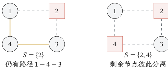
图 18.4 删除条件节点以检测分离。方形节点属于 S ，虚线边随节点一同删除，实线边保留。左侧删除 2 后仍有路径 1-4-3 ；右侧同时删除 2, 4 后，1 与 3 处于不同连通分量。
