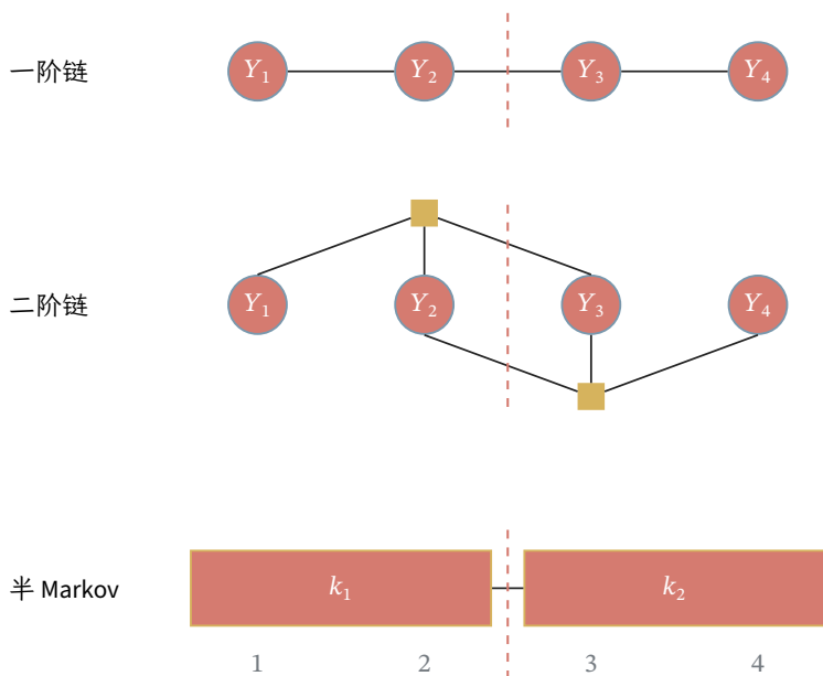
图 27.3 输出作用域的三种选择。一阶链的切分处只需保留一个标签; 二阶链中, 跨切分处的三元势需要保留两个标签。半 Markov 模型按片段边界递推, 图中展示一种 [1, 2] 与 [3, 4] 的分段, 推断时还须对其他合法边界求和。
