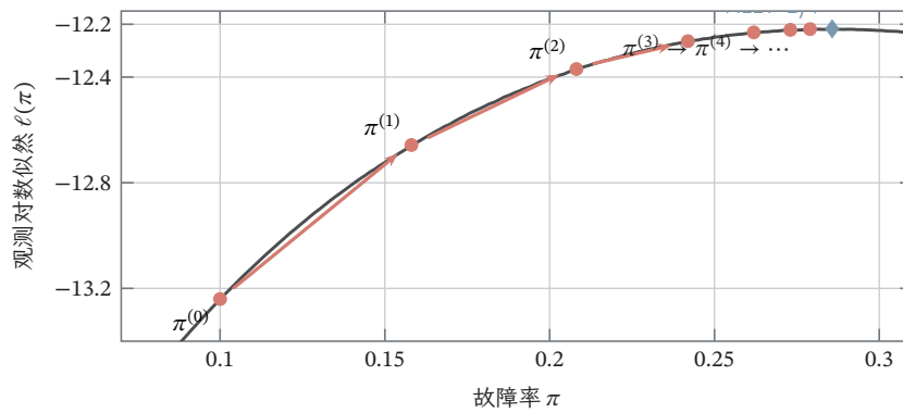
图 24.2 同一标量例子的多轮 EM 轨迹。红点依次为 \pi^{(0)}, \dots, \pi^{(6)} ，纵坐标均使用观测对数似然而非各轮不同的下界；蓝色菱形是解析 MLE 2/7 。轨迹展示似然逐轮上升并逐渐靠近驻点，但不把这一维构造推广为一般 EM 的全局最优保证。
