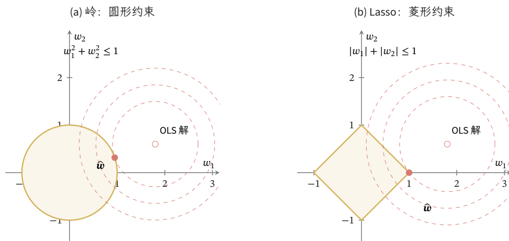
图 2.2 岭与 Lasso 的约束几何。构造损失为 J(\mathbf{w}) = \|\mathbf{w} - (1.8, 0.6)^T\|_2^2/2 , 虚线为等损失线, 浅色区域为可行域, 空心点为 OLS 解, 实心点为约束最优解。左图解为 (1.8, 0.6)^T/\sqrt{3.6} , 右图解为 (1, 0)^T 。两图都取单位约束半径以比较形状, 不表示相同的惩罚强度; Lasso 也并非总在尖点取到最优解。
