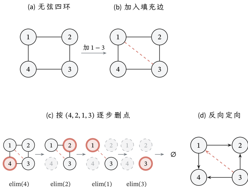
图 19.2 从无弦四环到完美有向图。先加入虚线填充边 1-3 完成弦化，再按完美消除序 (4, 2, 1, 3) 逐步删点；红色双圈标出当前消去节点，已消去节点保留为灰色虚线轮廓，便于跨快照对照。序列上方给出通用规则：elim( X_k ) 时补齐其未消去邻居为团。最终从序中较晚节点指向较早节点；实线箭头来自原四环，虚线箭头来自填充边。
