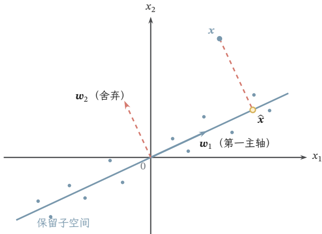
图 5.1 二维到一维的正交投影示意。蓝色实线方向 w_1 是保留的第一主轴，红色虚线方向 w_2 是被舍弃的正交主轴。点 x 投到 \hat{x} ，重构残差沿 w_2 方向。图中散点为示意位置，未表示真实实验。
