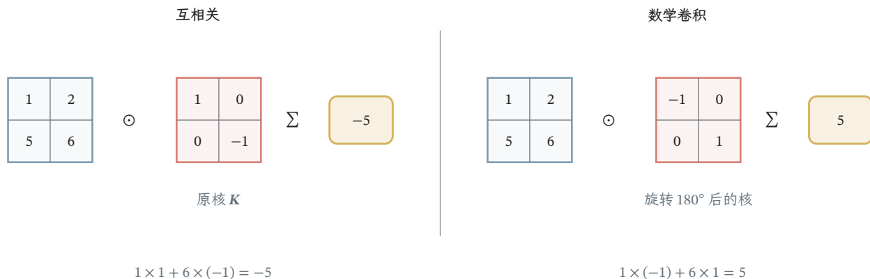
图 9.1 核的方向改变输出。输入窗口固定为 \begin{bmatrix} 1 & 2 \\ 5 & 6 \end{bmatrix} ，核固定为 \begin{bmatrix} 1 & 0 \\ 0 & -1 \end{bmatrix} 。左侧直接逐元素相乘后求和，得到互相关输出 -5；右侧先把核旋转 180 度，再求和，得到数学卷积输出 5。 \odot 表示逐元素乘法， \Sigma 表示把四个乘积相加。
