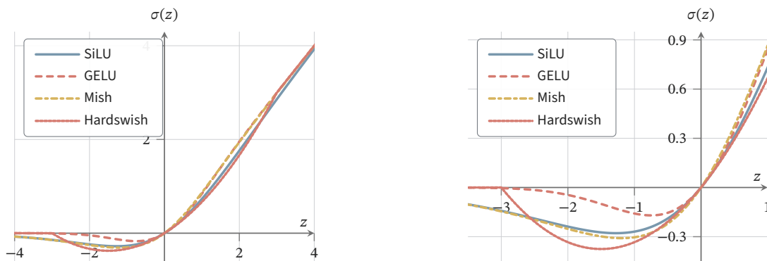
图 8.7 SiLU、GELU、Mish 与 Hardswish。左图展示整体响应, 右图放大原点附近的负值和过渡区域; GELU 按标准正态累积分布函数采样。它们在正端接近线性, 但负区间的形状和拐点不同。SiLU、GELU 与 Mish 平滑, Hardswish 含有分段边界; 两图使用不同坐标范围以显示细节。
