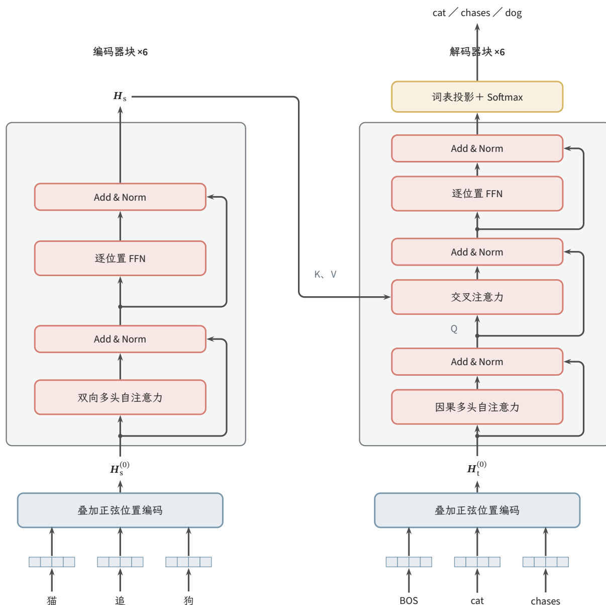
图 12.9 原始 Transformer 基础模型的层内计算与条件生成。浅色框内的编码器块和解码器块各堆叠 6 次；图展开一个块，Add & Norm 表示残差相加后逐位置 LN。源端最终输出供每个解码器块的交叉注意力生成 K、V，目标路径提供 Q。三个目标输出是对应右移输入的监督标签，推理时逐步生成。省略 Dropout、嵌入缩放和各头内部投影。参考 Bishop 与 Bishop (2024) 图 12.9、12.19 与 12.20 的布局重绘，结构依据 Vaswani 等 (2017)。
