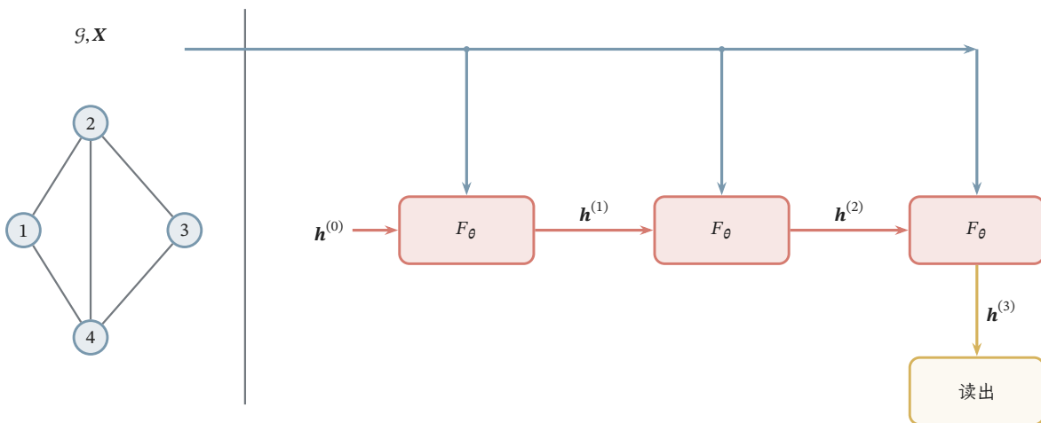
图 11.7 固定图上的循环更新。左侧表示邻接关系，右侧展开三轮共享更新 F_{\theta} ，每个状态向量包含整张图的节点状态。蓝色路径提供固定的图与输入特征，红色路径传递状态，黄色路径读出任务结果。轮次是内部计算步，不表示图已经发生三个时间点的变化。
