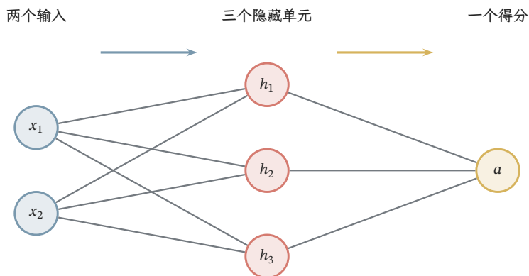
图 7.1 一个 2-3-1 多层感知机。两项输入先变成三个隐藏数值，再组合成一个分类得分。细线表示带权连接，箭头标出从左到右的计算方向；三个隐藏单元各作一次非线性变换，所有计算单元的偏置均省略。图只规定结构，权重尚未指定，也不要求某个隐藏单元预先代表某一种邮件特征。
