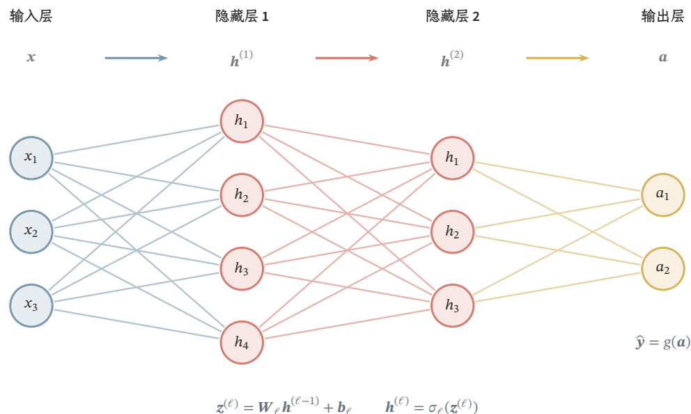
图 8.1 两个隐藏层的全连接前馈神经网络。蓝色圆点提供输入 \mathbf{x} ，红色圆点计算隐藏表示，黄色圆点产生原始得分 \mathbf{a} ，之后再使用任务规定的输出变换 g 。细线表示可学习的连接，层间箭头标明前向计算方向；每个目标单元还具有一个未画出的偏置。图中层宽依次为 3, 4, 3, 2，只是结构示例。
