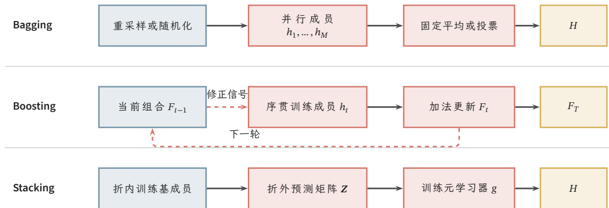
图 6.1 Bagging、Boosting 与 Stacking 的成员生成及组合关系。实线表示训练或预测的主路径，虚线表示由前一轮组合产生的修正信号。三类方法都输出组合预测，但成员间依赖与组合规则不同；图中流程为机制示意，不表示三者必须使用相同成员模型。
