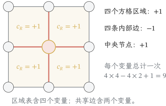
图 22.3 方格区域近似的计数。浅色块表示四个四变量区域，粗线标出需减去的内部边，中央节点需再加一次。每条区域一致性约束都要求大表格向交集边缘化后与小表格相同；颜色之外还用区域面积、线条和节点区分三个层次。
