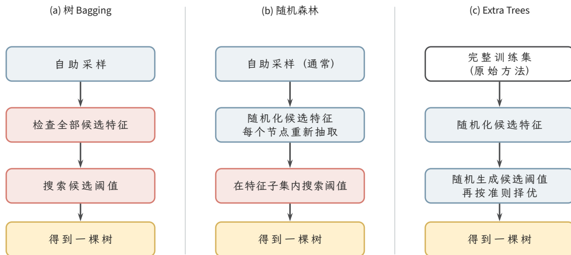
图 6.4 树 Bagging、随机森林与 Extra Trees 的随机化位置。蓝色节点表示引入随机性的环节，红色节点表示仍按任务准则执行的搜索，黄色节点表示得到的成员树。每栏首框直接标出训练样本来源：前两栏采用自助采样，Extra Trees 栏采用原始方法的完整训练集设定；具体实现也可能额外启用自助采样。
