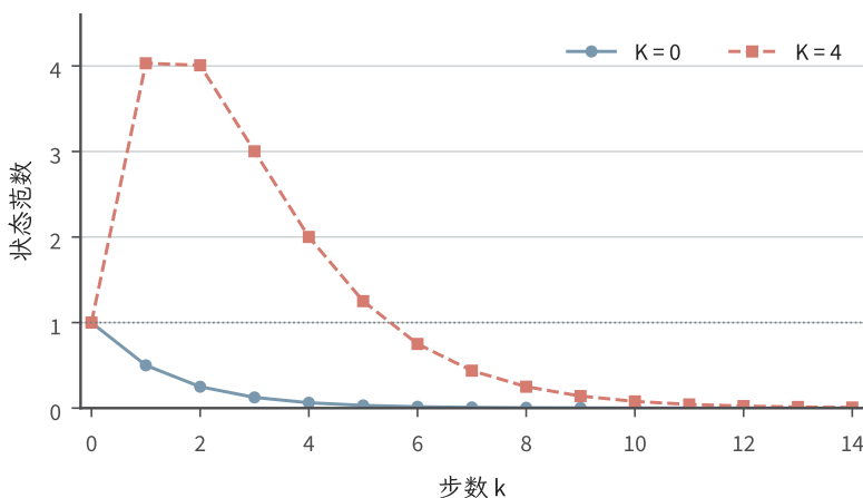
图 13.2 同谱系统的不同瞬态。初值均为 (0, 1)^\top , 蓝色圆点取 K = 0 , 红色方点取 K = 4 , 谱半径均为 1/2 。后者前两步范数约为 4.03、4.01, 随后才趋零; 灰线为初始范数 1。长期衰减不等于每一步都收缩。
