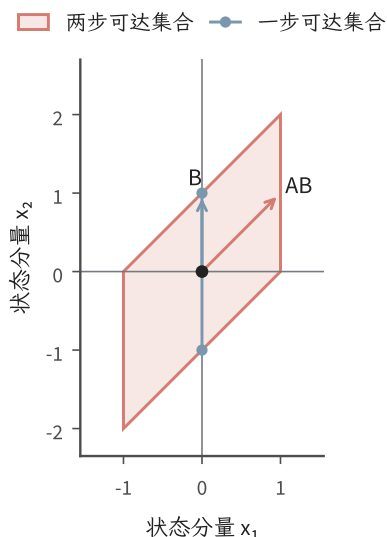
图 14.1 教学系统 \mathbf{A} = \begin{bmatrix} 1 & 1 \\ 0 & 1 \end{bmatrix} 、 \mathbf{B} = (0, 1)^\top 从零出发。蓝色线段为 |u_0| \leq 1 的一步可达集合，红色区域为 |u_0|, |u_1| \leq 1 的两步可达集合；箭头为 \mathbf{B} 与 \mathbf{A}\mathbf{B} 。幅值限制用于显示可达区域，不属于无约束可控性秩判据的假设。
