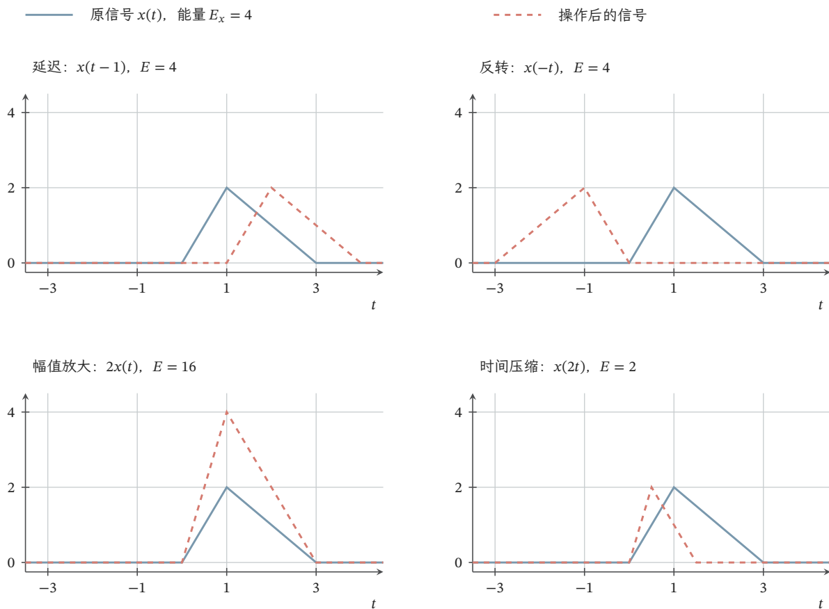
图 12.2 对同一非对称三角脉冲分别延迟、反转、放大幅值和压缩时间。每幅图的蓝线均为式(12.14)的原信号，红线为指定操作结果，横轴为时间、纵轴为幅值，坐标尺度一致。平移和反转保持整轴能量 4，幅值乘 2 使能量变为 16，时间压缩为一半使能量变为 2；各图均在整轴零值背景下观察，不作窗口裁剪。
