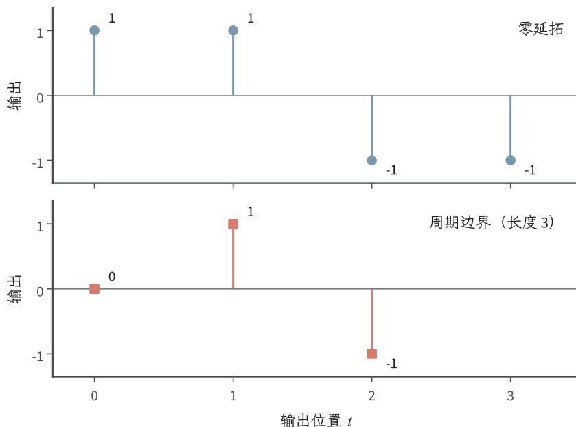
图 12.4 输入 (1, 2, 1) 与核 (1, -1) 的边界比较。蓝色圆点采用零延拓，给出四项线性卷积；红色方点采用长度 3 的循环边界，末项 -1 回到首项并与 1 抵消。连线只指示离散数值的顺序，不定义整数之间的信号值。
