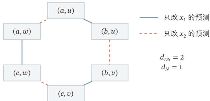
图 2.7 六模式族 V 的逐坐标邻接。每个顶点是一种两输入预测; 蓝实线只改变第一坐标, 红虚线只改变第二坐标。每个顶点在两个方向上都有邻居, 所以它构成二维伪立方体; 图中没有固定两标签对形成的四角矩形, 故其 DS 维为 2 而 Natarajan 维为 1。
