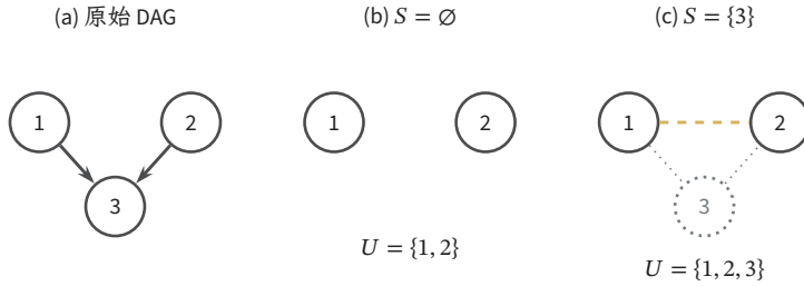
图 11.4 祖先道德图随查询条件改变。端点固定为 1, 2 ；空条件集时，查询图只有两个孤立顶点。给定 3 时，先扩大的祖先集合使道德化加入黄虚线 1-2 ，随后删除灰色条件点及灰点线，却不删除这条新增边。不能先道德化整图再取查询顶点。
