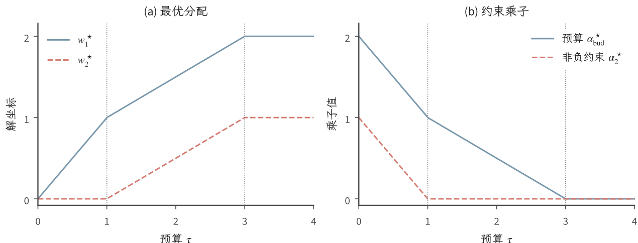
图 4.4 例 4.19 的解析解。左图为两个最优分配坐标，右图为预算乘子与第二个非负约束的乘子。竖参考线标出 \tau = 1, 3 ；在切换点约束可以取等号而乘子为零，说明活跃性与正价格并不等价。
