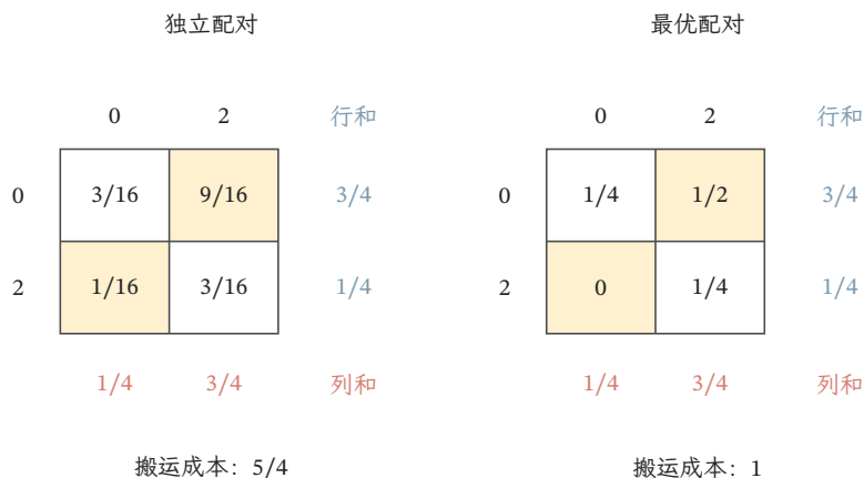
图 9.5 同一边缘约束下的两张搬运表。来源和目标都位于 0, 2 ，蓝色行和为 \mathbf{p} = (3/4, 1/4) ，红色列和为 \mathbf{q} = (1/4, 3/4) 。黄色单元格承担非零距离成本。独立表的成本为 5/4 ，最优表为 1；正文的势函数给出与最优表相等的对偶值。
