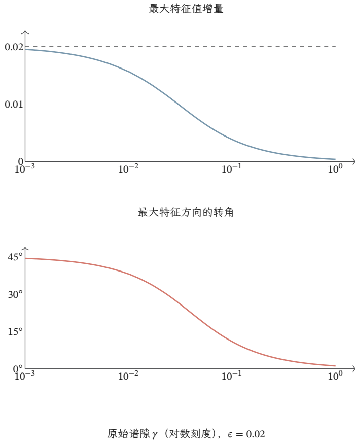
图 6.9 同一对称扰动下，谱值稳定不等于方向稳定。上图为 \sqrt{(\gamma/2)^2 + 0.02^2} - \gamma/2 ，灰虚线为扰动范数 0.02；下图为 \theta = \frac{1}{2} \arctan(0.04/\gamma) ，角度用度表示。两图共用谱隙横轴，所有数值均来自二阶特征方程的解析解。
