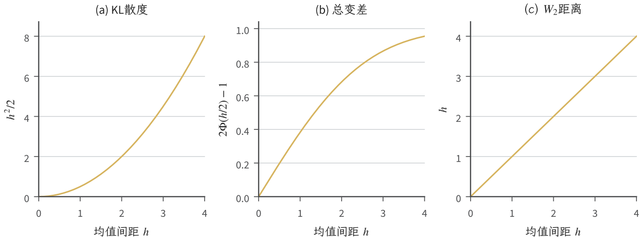
图 9.3 同方差高斯位置族的解析式比较。固定 P = \mathcal{N}(0, 1) 、 Q = \mathcal{N}(h, 1) ，三图分别为 D_{\text{KL}} = h^2/2 、 d_{\text{TV}} = 2\Phi(h/2) - 1 与 W_2 = h ，图中 h \geq 0 。纵轴分别表达对数代价、事件概率差与搬运位移。
