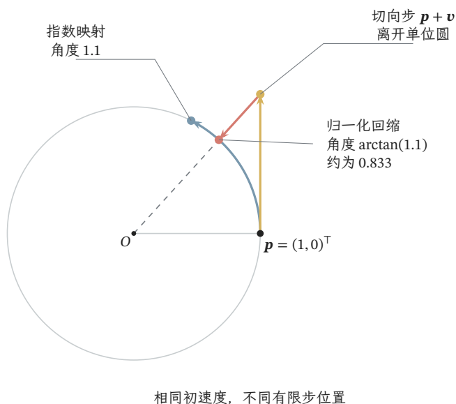
图 7.6 单位圆截面中的切向步、指数映射与归一化回缩。从 \mathbf{p} = (1, 0)^\top 沿 \mathbf{v} = (0, 1.1)^\top 直接相加得到圆外点；蓝色指数更新转过 1.1 弧度，红色归一化更新转过 \arctan(1.1) 弧度。两条曲线在零步长处有相同初速度，但有限步位置不同。图为解析教学示例。
