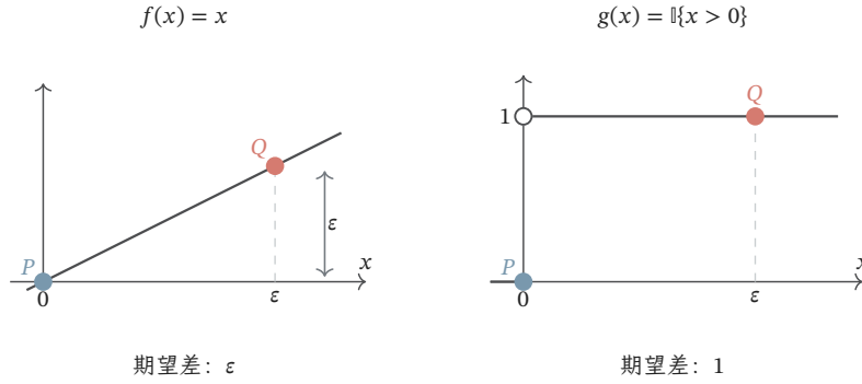
图 9.4 同一小位移对两种固定评价的影响。取 P = \delta_0 、 Q = \delta_\varepsilon 、 \varepsilon > 0 ，底层距离为绝对值。左图的 1-Lipschitz 函数 f(x) = x 变化 \varepsilon ；右图的事件函数 \mathbb{1}\{x > 0\} 变化 1。横向位置仅作示意，结论对任意正的 \varepsilon 成立。
