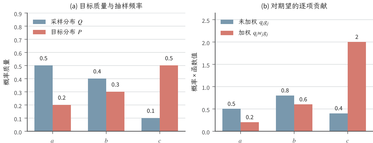
图 8.4 三结果换测度的有限构造。左图比较采样分布 Q 与目标分布 P ，右图比较 q_j g_j 与 q_j w_j g_j = p_j g_j 。各柱从零起画；右图柱高之和分别为 1.7 和 2.8，并非单点概率。
