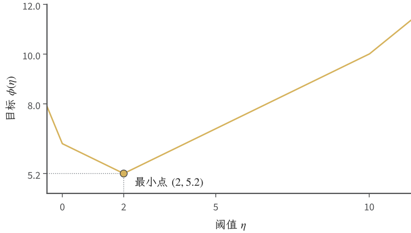
图 15.1 教学分布 P(L=0)=0.6 、 P(L=2)=0.3 、 P(L=10)=0.1 在 \alpha=0.75 下的阈值目标 \phi(\eta) = \eta + 4E[(L - \eta)_+] 。暖黄色折线的最小点为 (2, 5.2) ；阈值 2 与尾部平均 5.2 不能混用。
