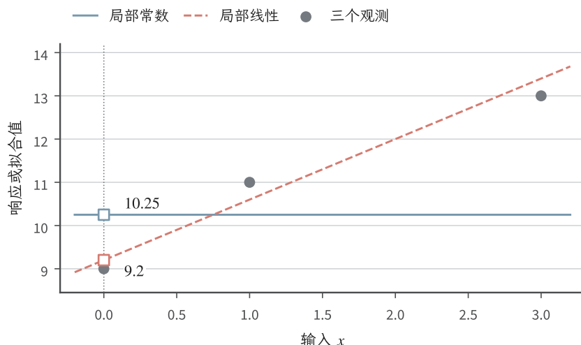
图 8.11 边界处的局部常数与局部线性拟合（教学数据图）。观测为 (0, 9), (1, 11), (3, 13) ，权重为 1, 0.75, 0.25 。蓝实线为加权常数 10.25，红虚线为 9.2 + 1.4x ，边界 x_0 = 0 处分别预测 10.25 和 9.2。
