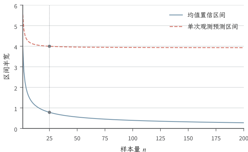
图 8.12 已知 \sigma = 2 的独立高斯位置模型中，两类区间半宽随样本量变化（解析式教学图）。使用四舍五入分位数 1.96，蓝实线为 1.96\sigma/\sqrt{n} ，红虚线为 1.96\sigma\sqrt{1 + 1/n} 。灰竖线标出例 8.95 的 n = 25 ，没有对任何实测数据重复抽样。
