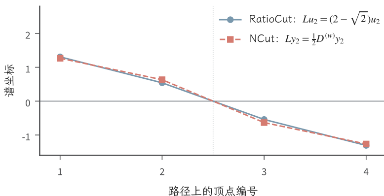
图 11.11 单位权四顶点路径的两种谱方向。蓝实线为组合拉普拉斯第二特征向量，红虚线为度加权广义特征向量，点形也作区分。显示时均按欧氏范数 2 缩放，不替代 NCut 的度加权范数。横轴为四个离散顶点，连线仅引导阅读；竖虚线标出零阈值分割，两种方向虽同号分组，相对幅度并不相同。
