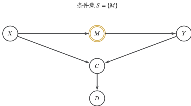
图 10.4 多条路径下的 d-分离。双边框节点 M 属于条件集，上方链式路径关闭；碰撞点 C 及其后代 D 都未给定，下方路径也关闭。若再把 C 或 D 加入条件集，下方路径就会打开，说明增加条件可能破坏原有的分离。
