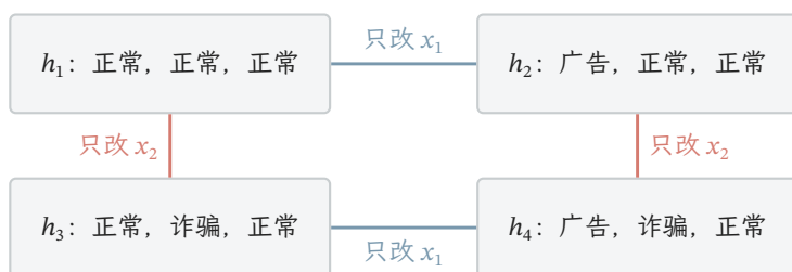
图 2.6 Natarajan 打散的四中预测。每个框中的三项依次对应 x_1, x_2, x_3 ；横向只改变 x_1 ，纵向只改变 x_2 ，而 x_3 始终预测为正常。每个输入处的两个标签预先固定，四个函数实现全部二选一组合。
