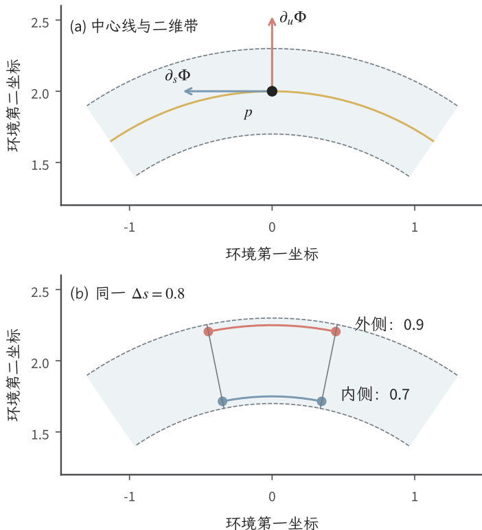
图 7.3 开带与中心线的局部方向不同。取 R = 2 、 w = 0.3 。上图的两个参数方向属于二维开带，仅以中心线为对象时，径向方向不属于其切空间；箭头平移到 p 只是画法。下图取 u = -0.25, 0.25 ，同一 \Delta s = 0.8 对应圆弧长度 0.7, 0.9。灰虚线为不纳入开带的边界，两图等比例绘制，均为解析教学示例。
