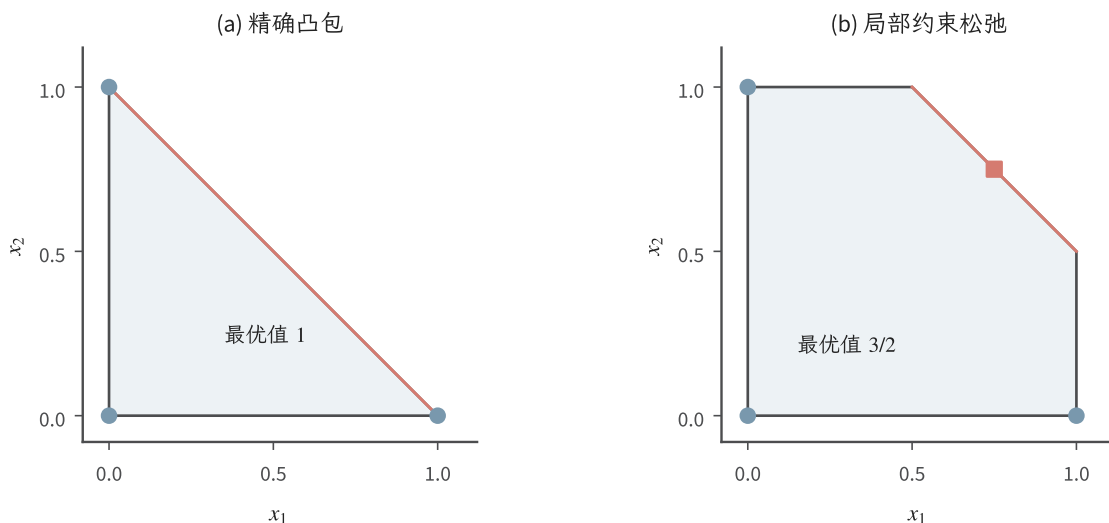
图 4.5 最大化 x_1 + x_2 的两种放宽。左图精确凸包满足 x_1 + x_2 \leq 1 ；右图局部松弛满足 0 \leq x_i \leq 1 与 x_1 + x_2 \leq 3/2 。实心圆为整数可行点，方形为右图的分数最优点 (3/4, 3/4) ，粗边标出各自最优面。两图采用相同坐标尺度。
