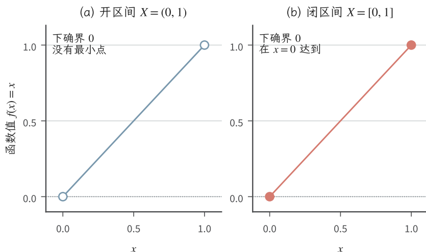
图 1.2 同一函数 f(x) = x 的边界对照。左图定义域为 (0, 1) ，空心端点不属于图像，函数值可任意接近 0，却不能取到；右图定义域为 [0, 1] ，实心端点 (0, 0) 达到下确界。两图的下确界相同，最小点是否存在取决于可行端点是否保留。图为解决教学示例。
