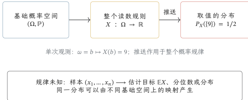
图 8.1 基础结果经随机变量映射成为读数；把事件概率推送到取值空间得到分布。分布未知时，样本用于估计指定目标，并不能唯一还原基础空间上的映射。
