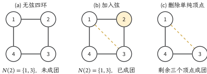
图 11.7 四环补入弦 1-3 后, 顶点 2 的两个邻居已经相邻。删除 2 不需填充, 余图 \{1, 3, 4\} 是团, 因此 (2, 1, 3, 4) 是补弦图的完美消元序。补边改变了原图的路径与分离关系, 不能把右图当作左图所有查询的等价表示。
