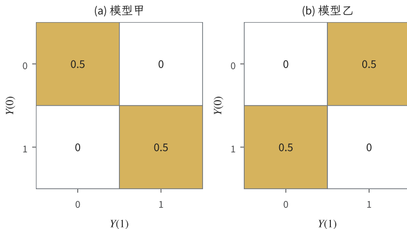
图 10.1 相同干预边缘的两种跨世界配对。行对应 Y(0) ，列对应 Y(1) ，格内数字为联合概率；每张表的行和、列和均为 1/2 。甲的个体效应恒为零，乙的个体效应等概率取 1, -1 ，两者 ATE 均为零。这是相容机制的教学构造，不是随机试验直接观察到的潜在结果联合表。
