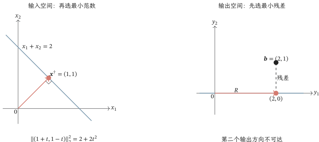
图 6.4 伪逆的两次选择。右图先在可达输出中选择离 \mathbf{b} = (2, 1)^T 最近的 (2, 0)^T ；左图再在整条原像直线 x_1 + x_2 = 2 上选择最靠近原点的 (1, 1)^T 。两图属于不同空间，各自等比例绘制。
