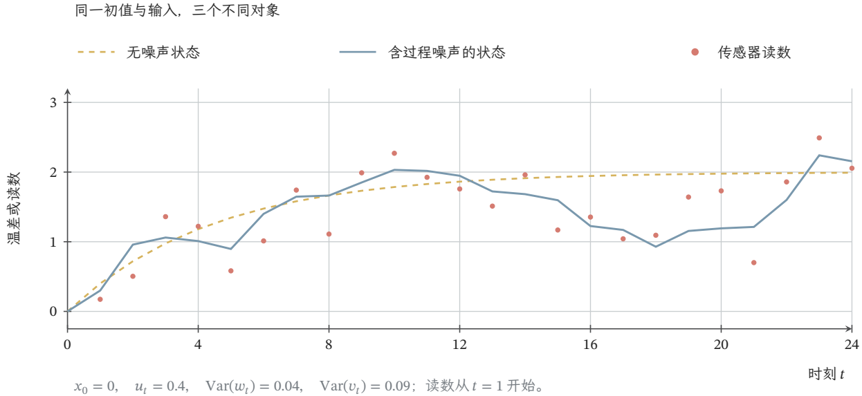
图 13.4 同一温度模型的两个对象。初态 x_0 = 0 , 输入始终为 0.4; 无噪声轨迹趋于 2, 过程噪声改变真实状态, 独立观测噪声又把真实状态变成带噪读数。噪声方差分别为 0.04 和 0.09。图中带噪曲线是固定种子的教学模拟, 不是置信区间, 也没有把读数用于反向校正状态。
