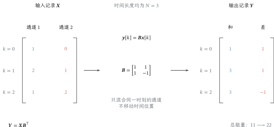
图 12.5 同一双通道三时刻记录的轴与混合。左侧行标记时间、列标记通道; 中间矩阵 \mathbf{B} 对每一行对应的同时读数取和与差, 右侧时间轴长度仍为 3。通道混合不是时间平移, 也不意味着两个输入通道独立; 这里只使用当前时刻的值。
