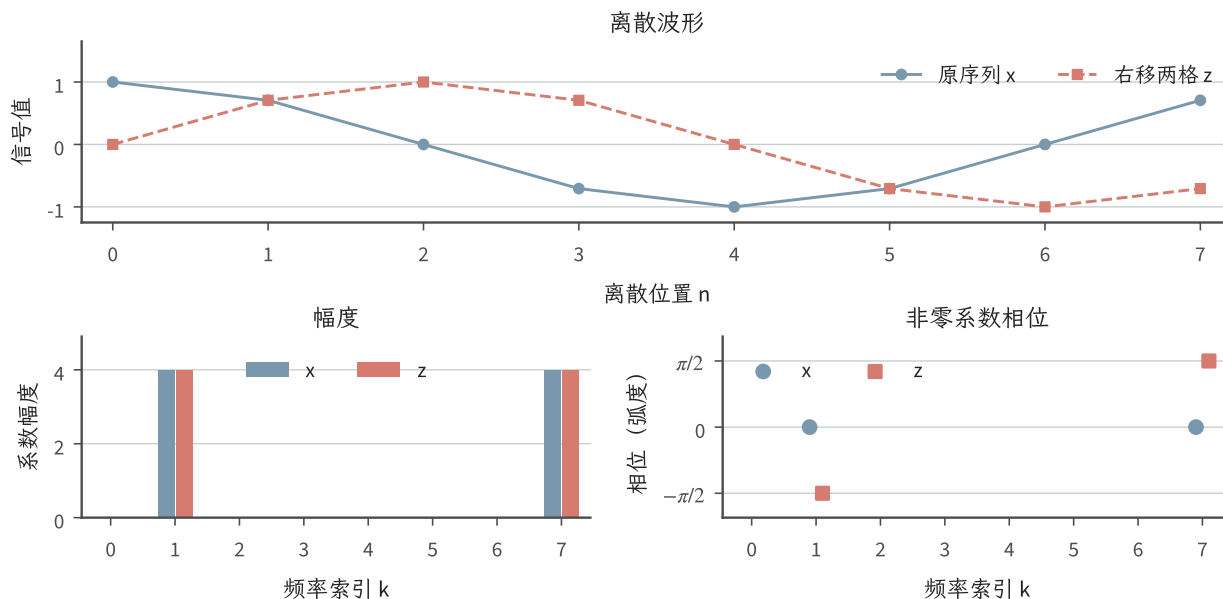
图 12.1 长度 8 的余弦信号 x[n] = \cos(2\pi n/8) 及其循环延迟两格的结果。上方波形的峰值位置不同，下方在 k=1, 7 的幅度均为 4，相位却改变。相位图只画非零系数；波形连线只帮助观察顺序，不表示已选择连续时间插值。
