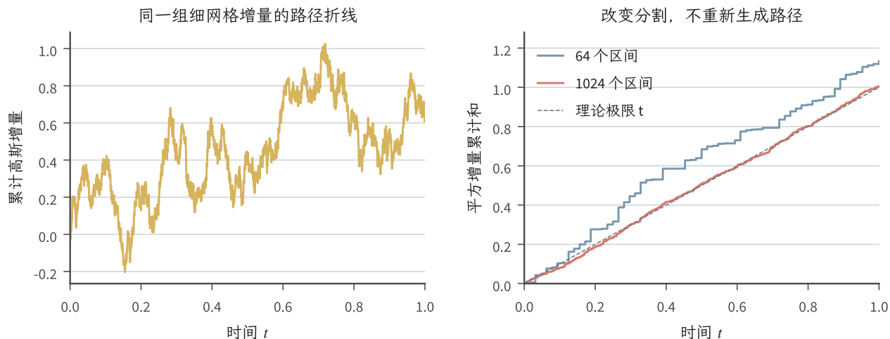
图 8.9 以固定随机种子构造的高斯增量教学例。左图由 4096 个独立增量 \Delta W_i \sim \mathcal{N}(0, 1/4096) 累计成路径折线；右图将同一组增量分别合并为 64 和 1024 个时间区间，再累计各区间增量的平方。蓝、红阶梯线使用不同分割，灰色参考线为理论二次变差 t 。这里只绘制有限网格，不把某一条折线作为连续布朗路径或收敛证明。
