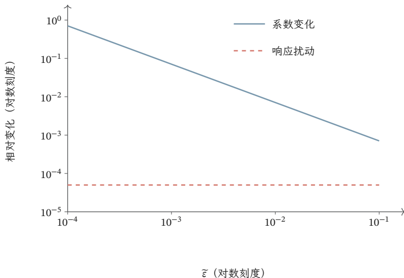
图 6.8 近共线矩阵的精确敏感性。固定 \mathbf{y}_0 = (2, 0)^\top ，扰动为 (0, 10^{-4})^\top ；红线是响应相对扰动 5 \times 10^{-5} ，蓝线是系数相对变化 10^{-4}/(\sqrt{2}\varepsilon) 。双对数坐标显示列越接近，反求系数越敏感；图中没有数值求解误差。
