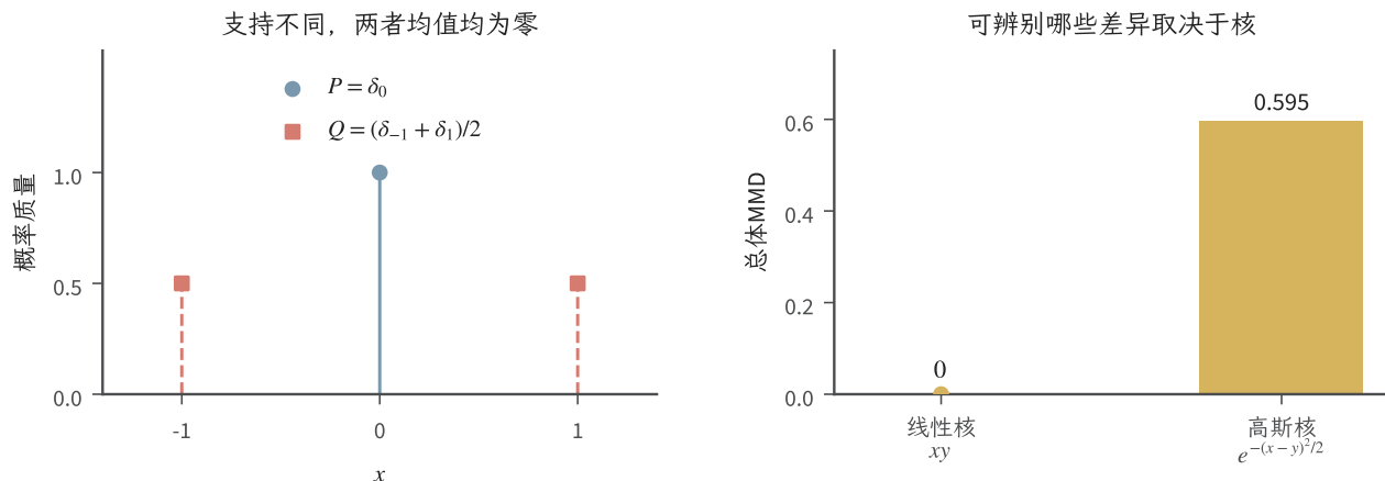
图 9.2 同均值分布在不同核下的 MMD (解析式教学图)。左图为 P = \delta_0 与 Q = (\delta_{-1} + \delta_1)/2 ，右图按精确总体期望计算：线性核给出零，高斯核给出约 0.595。没有使用有限样本估计；差别来自测试函数类。
