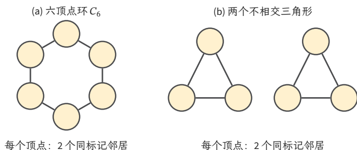
图 11.14 同样的邻居标记计数可以来自不同全局结构。两张六顶点图初始同标记，每轮每点仍见到两个同标记邻居，故 1-WL 计数无法区分一条六环与两个三角形。这不表示连通性难计算，而是说明该细化遗漏了这一差异。浅黄只表示共同标记，不加入唯一编号，以保持无标记图的比较设定。
