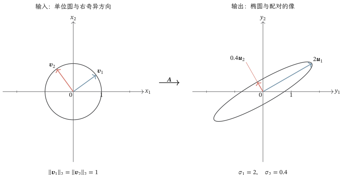
图 6.6 矩阵 A = R(\pi/6)\text{diag}(2, 0.4)R(\pi/5)^T 将单位圆变为椭圆。蓝、红箭头分别标出右奇异方向 \mathbf{v}_i 及其像 \sigma_i \mathbf{u}_i ；两侧坐标比例相同。奇异值决定长度变化，左右方向可以不同，因而这不是沿特征方向的空间缩放。图为教学构造。
