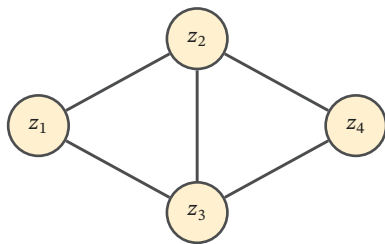
图 11.1 由四变量约束的作用域导出的关系图。边表示两个变量共同出现在至少一个约束中；共享顶点集合 \{2, 3\} 连接左右两侧。图没有记录约束的具体真值表，也没有预先指定边长、容量或相似度。
