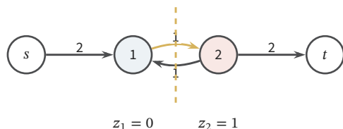
图 11.10 两变量能量的割表示，零容量弧省略。割把 s, 1 与 2, t 分开，因而标签为 z_1 = 0, z_2 = 1 。两个容量为 1 的反向弧中，仅源侧到汇侧的黄弧 1 \rightarrow 2 计费，成本不是 2。终端弧 s \rightarrow 1 的容量 2 = D_1(1) 只在顶点 1 进入汇侧时支付。
