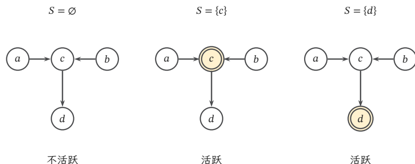
图 11.3 同一底层路径 a-c-b 在三个条件集下的活跃性。箭头及顶点没有改变；空条件集未打开碰撞点，给定碰撞点 c 或其后代 d 都会打开它。双圈表示被给定的顶点，底部文字给出判定。活跃性不是沿箭头从 a 走到 b 的可达性，也不是简单删除条件顶点后的连通性。
