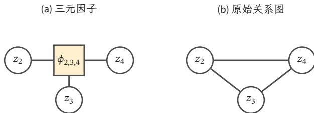
图 11.2 三元因子与原始关系图。左侧方框是同一个依赖 z_2, z_3, z_4 的函数，连线表示作用域归属；右侧只保留变量共同出现的两两关系。右侧三条边不是把三元函数分解成三个二元函数的等价变换，也不能恢复原函数的数值。
