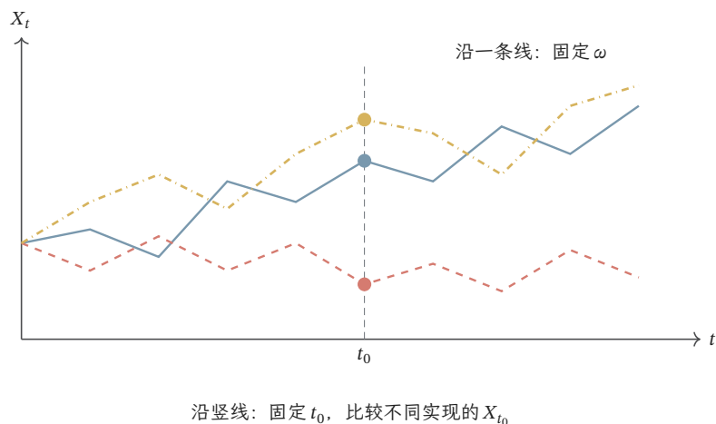
图 8.6 同一过程的路径与时刻截面是不同对象。图为人为给定的三条示意路径，竖虚线固定时刻 t_0 ；交点展示该时刻可能出现的不同值，并非用三条路径估计出的概率密度。
