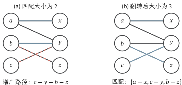
图 11.9 沿交替路径重新安排匹配。两组顶点为 U = \{a, b, c\} 、 W = \{x, y, z\} 。蓝实线是已选边，左图红虚线是增广路径的未选边，灰线是其余候选边。翻转 c - y - b - z 后保留 a - x ，得到三条互不共享端点的边。线条表达候选配对，不表达因果方向。
