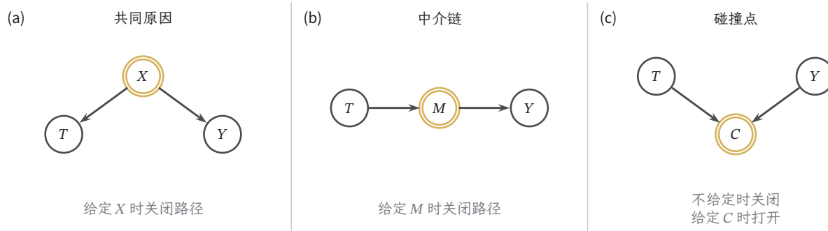
图 10.3 共同原因、中介与碰撞点的局部路径。双边框表示节点已加入条件集。共同原因和中介是非碰撞点, 给定后关闭这条路径; 给定碰撞点则打开原本关闭的路径。路径打开表示图不再保证相应独立性, 并不指定相关的大小或正负。
