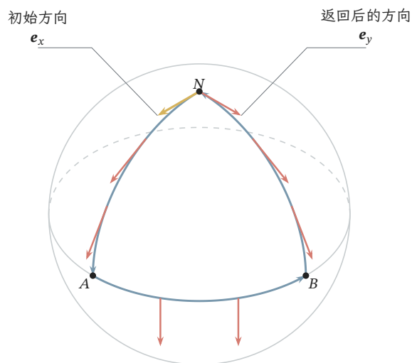
沿路协变导数为零，闭路终值仍可改变
