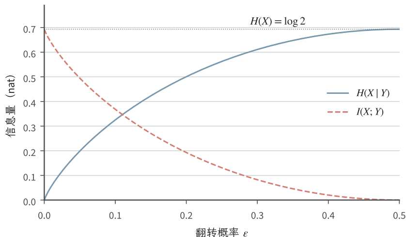
图 9.1 公平二元输入通过独立翻转通道后的信息分配 (解析式教学图)。蓝实线为剩余条件熵 H_b(\epsilon) , 红虚线为互信息 \log 2 - H_b(\epsilon) , 均以 nat 计。输入熵保持不变, 零噪声与公平翻转分别对应完整信息与零信息。
