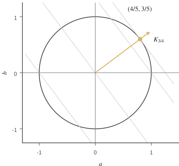
图 5.7 仿射 RKHS 中读取 f(3/4) = a + 3b/4 。灰圆表示 a^2 + b^2 \leq 1 ，黄箭头是核截面 K_{3/4} 对应的系数 (1, 3/4) ；灰平行线为相同点值。黄圆点 (4/5, 3/5) 达到单位范数球上的最大点值 5/4 。这里坐标是函数系数，不是输入位置。图为解析教学示例。
