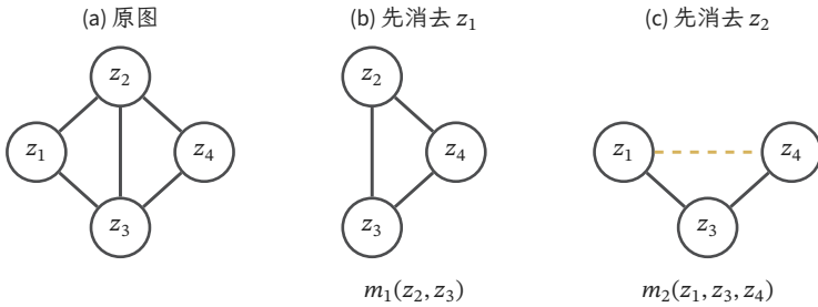
图 11.6 两个首步消元产生不同接口。删去 z_1 后，新表索引 (z_2, z_3) ；删去 z_2 后，通常须索引 (z_1, z_3, z_4) ，黄虚线为填充边 1-4。二值稠密接口表分别有 4 和 8 项，虽然两张余图都只剩三个顶点。特殊函数可能还能分解；图给出的是通用作用域范围。
