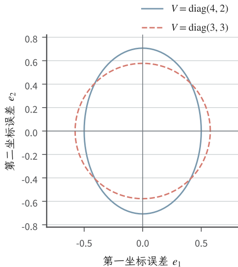
图 8.13 二维设计的归一化误差几何（解析式教学图）。蓝实线为 \mathbf{e}^\top \text{diag}(4, 2)\mathbf{e} = 1 ，红虚线为 \mathbf{e}^\top \text{diag}(3, 3)\mathbf{e} = 1 。它们不是已经具有相同覆盖概率的数值置信区间；真实置信半径由式 (8.62) 另行确定。
