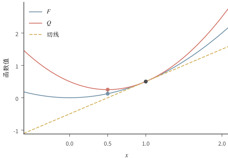
图 4.6 代理上界与切线的区别。蓝线为 F(x) = x^2/2 ，红线为当前点 1 处的主化代理 Q ，黄虚线为同点切线 x - 1/2 。三者在当前点同值同斜率，但切线位于目标下方，最小化它不能使用 MM 的上界链；红点标出代理最小点对应的值。图了解析教学示例。
