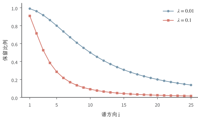
图 5.8 教学谱 \mu_j = j^{-2} 上的收缩比例 \mu_j/(\mu_j + \lambda) 。蓝、红线使用 \lambda = 0.01 和 0.1 ，点标出前 25 个方向；增大正则化后更多方向被抑制。有效维度的定义仍对全部谱方向求和。
