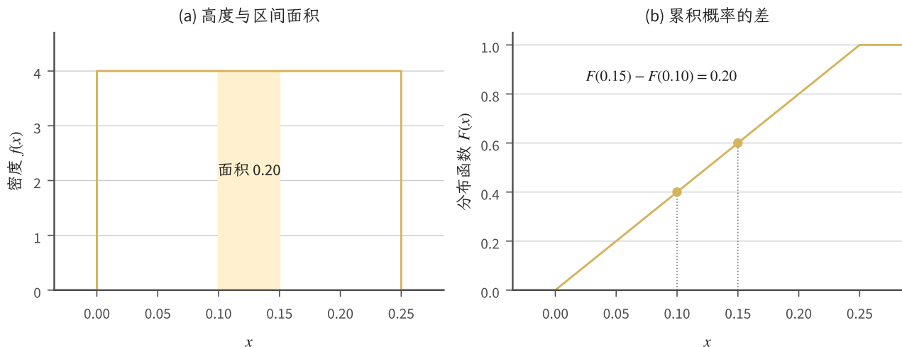
图 8.2 区间 [0, 1/4] 上的均匀分布（解析式教学图）。左图阴影为 [0.10, 0.15] 的概率 0.20，密度高度为 4；右图的概率是 F(0.15) - F(0.10) ，两个端点本身均没有正概率质量。
