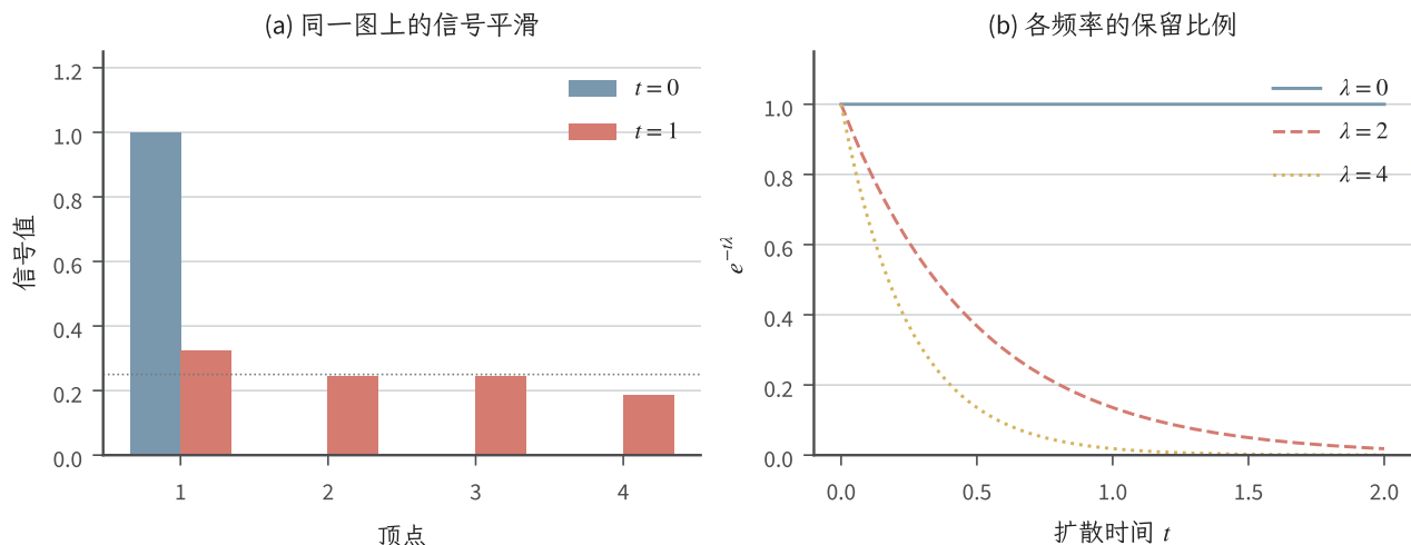
图 11.13 贯穿四顶点图的解析式扩散。左图比较 \mathbf{f}(0) = (1, 0, 0, 0)^T 与 \mathbf{f}(1) = e^{-L}\mathbf{f}(0) , 灰虚线是最终均值 1/4 ; 右图绘制特征值 0, 2, 4 的保留比例, 4 的重数为 2。柱和曲线直接由该图的拉普拉斯计算, 不表示实验均值或误差条。
