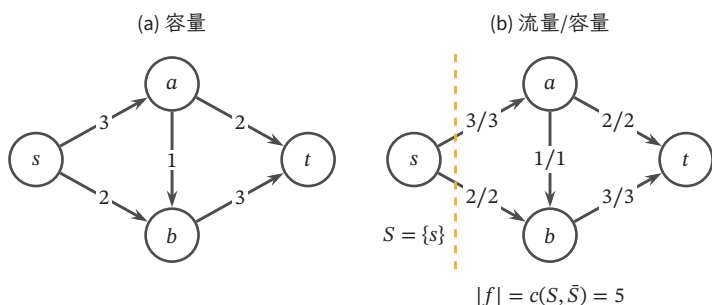
图 11.8 同值流与割构成最优性证书。左图标容量，右图标流量/容量；内部顶点均满足流守恒。黄虚线划出 S = \{s\} ，跨出它的容量为 3 + 2 = 5 ，等于已实现流值。图中画的是原网络弧，未画残量反向弧。
