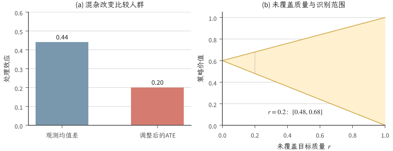
图 10.2 两个独立的教学构造。左图比较风险分层例子的观测均值差 0.44 与调整效应 0.20。右图按式 (10.31) 绘制 [0.6(1-r), 0.6(1-r)+r] 。阴影为总体识别范围，不是抽样置信带；两个面板不表示同一数据集。
