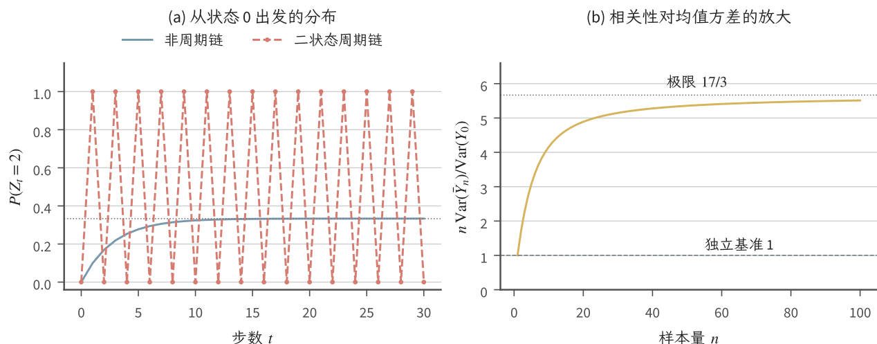
图 8.7 两状态链的解析式教学图。左图蓝线使用例 8.80 的转移矩阵，从 Z_0 = 0 出发绘制 \mathbb{P}(Z_t = 2) = (1 - 0.7^t)/3 ；红线使用确定交替的转移矩阵。右图使用平稳初态和 \rho_k = 0.7^k ，绘制 1 + 2 \sum_{k=1}^{n-1} (1 - k/n) \rho_k ，其极限为 17/3 ，独立观测基准为 1。
