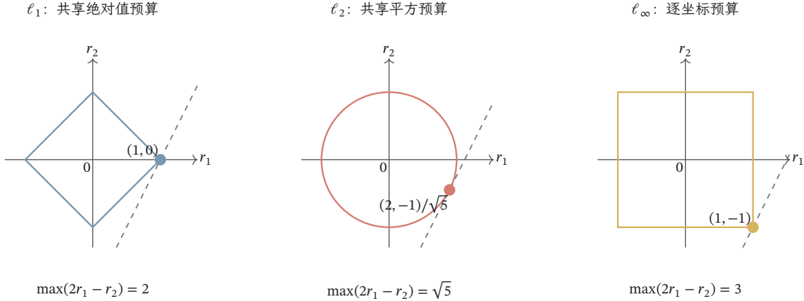
图 6.1 同一线性读取 2r_1 - r_2 在 \ell_1 、 \ell_2 、 \ell_\infty 单位球上的最大值依次为 2、 \sqrt{5} 、3。虚线为最后接触可行集的支撑直线，点为最大化方向。三图坐标尺度相同，均为解析教学例；改变允许误差的形状会改变误差常数。
