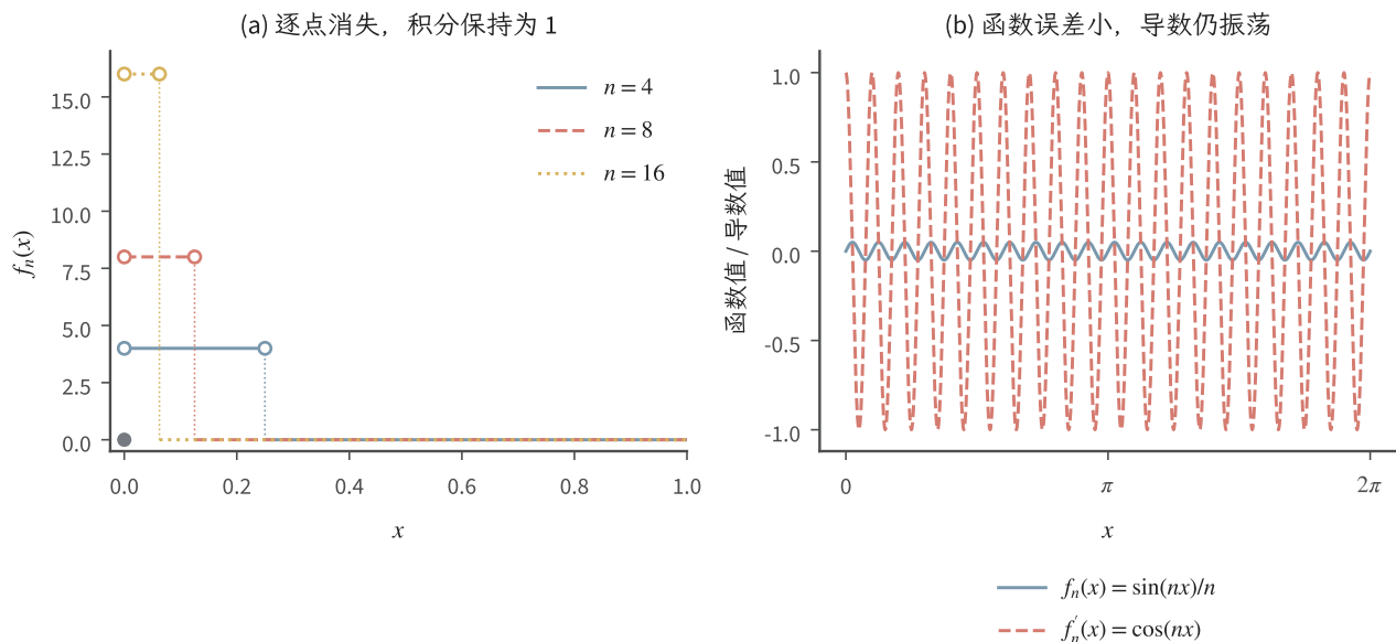
图 3.8 两种交换运算的障碍。左图的尖峰支撑不断收缩，但高度同步增长，每条曲线的积分仍为 1；开圆点标出不取的上端点，竖虚线仅提示跳跃。右图取 n = 20 ， \sin(nx)/n 的函数幅度很小，导数 \cos(nx) 仍有单位幅度。两图均为按给定函数公式构造的教学示例。
