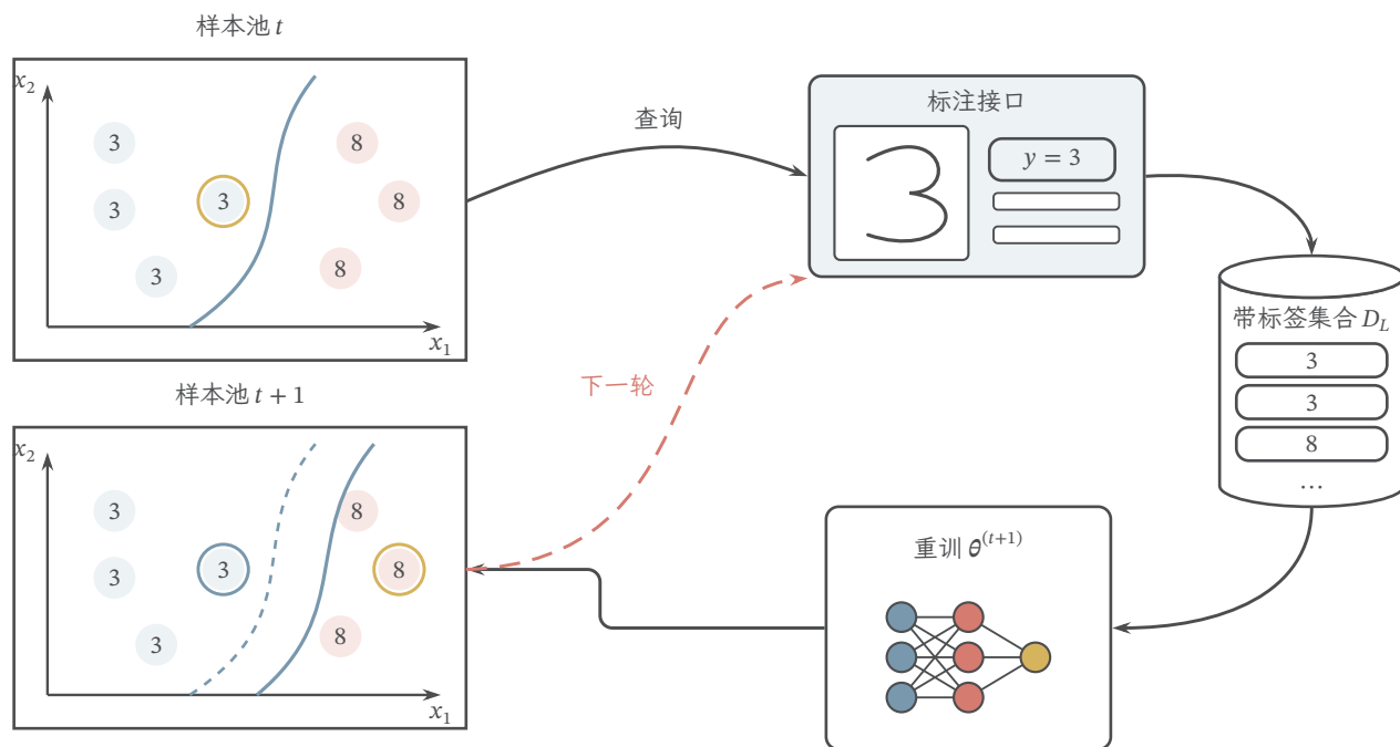
图 3.8 池式主动学习的教学示意。蓝色曲线表示当前模型的决策边界，暖色圆圈标出本轮选择的不确定样本。标注者返回标签后，样本并入带标签集合，用于重训模型。下方的点线保留更新前的边界，实线表示更新后的边界；中央带蓝色圈的数字 3 已获标签，右侧带暖色圈的数字 8 是下一轮查询对象。查询预算限制循环。数字图元、二维位置和边界均为教学构造，不表示实测分布或选择收益。
