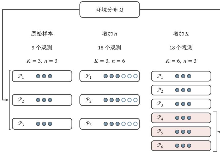
图 9.6 环境数量 K 与环境内样本数 n 对应不同的抽样层。每行边界代表一个环境，圆点代表其中的观测。左侧从同一环境分布 \mathcal{Q} 独立抽取 3 个环境，各取 3 个观测；中间的空心点表示在原有 3 个环境中继续抽取的观测，每个环境增至 6 个；右侧从 \mathcal{Q} 新抽取 3 个独立环境，每个环境仍取 3 个观测。中、右都有 18 个观测，只有右侧增加了独立环境数量。图中数量为教学构造，不对应实测数据。
