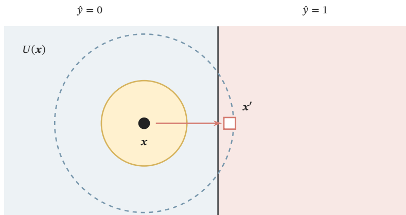
图 12.1 允许变化、认证范围与搜索反例的集合关系示意。虚线圈表示 U(x) ，内圈表示已有认证支持的稳定范围，方点 x' 是跨越决策边界的允许变化。圆的尺寸不是随机平滑的实验结果；搜索没有找到反例时，也不能直接把整个允许集合视为已认证。
