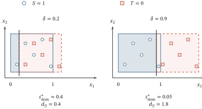
图 9.4 域分类器的错误只对应输入散度项。源输入均匀分布于 [0, 1]^2 ，目标支持沿 x_1 平移 \delta ；圆点、方块的位置为教学构造，错误率由区域概率计算。 \mathcal{H} 含双向阈值与常值假设，域分类器类取 \mathcal{G} = \mathcal{H} \triangle \mathcal{H} 。其中 g = h_0 \oplus h_\delta 在左侧浅色带预测源域， h_a(x) = \mathbb{I}\{x_1 \geq a\} ；两域均等先验时，最小域错误为 (1 - \delta)/2 ， d_g = 2\delta 。任务风险界还包含源风险及 \lambda = \inf_{h \in \mathcal{H}} (R_S(h) + R_T(h)) ，不能只由域错误决定。
