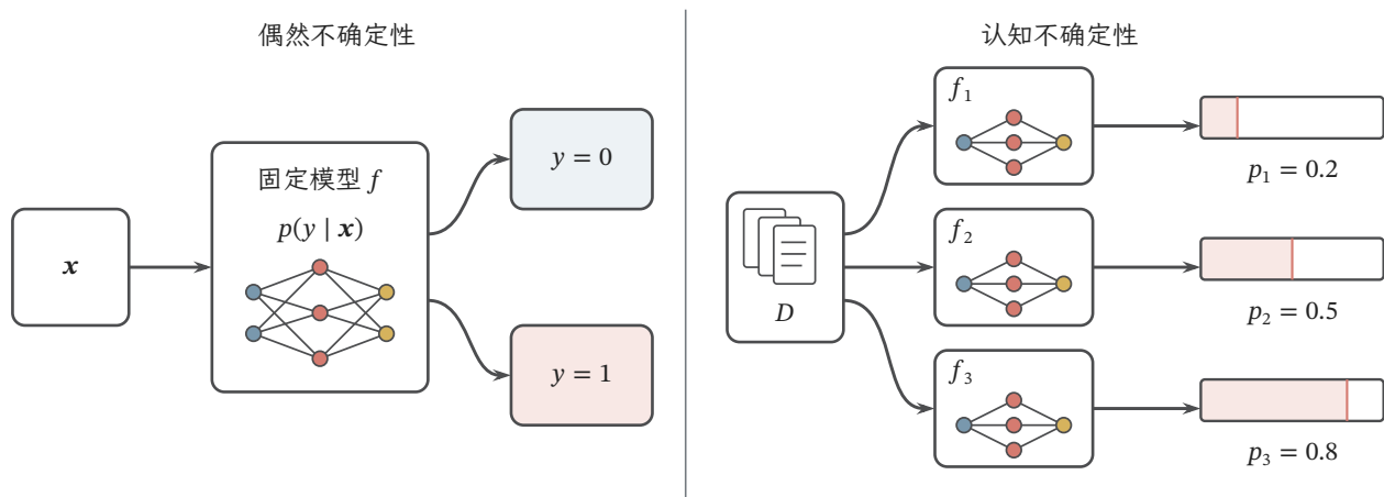
图 11.2 偶然不确定性与认知不确定性的区别。左侧同一可见特征可能对应正常通知或诈骗意图，固定模型也需表达结果分布；右侧相关样本不足，三个候选模型给出不同预测， p_m 简写 p_m(y=1|x) 。概率 0.2、0.5、0.8 为教学构造，条长示意预测分歧，不是实测值或后验抽样。两种来源均相对于当前观测与模型假设而言。
