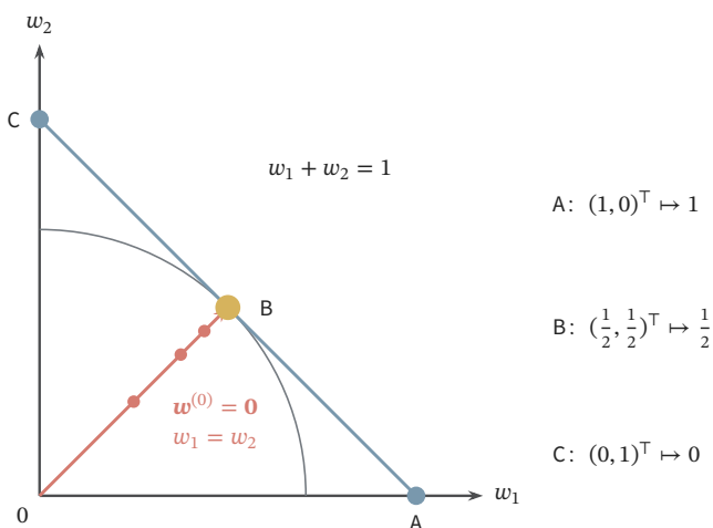
图 8.6 一个训练观测对应多个插值参数。直线上的 A、B、C 都使输入 (1, 1)^\top 的预测为 1, 右侧列出它们对同一新输入 \mathbf{x}_{\text{new}} = (1, 0)^\top 的预测。对半平方损失从零初始化, 图中以步长 1/4 画出前三次更新, 轨迹趋向 B; 细弧表示经过 B 的欧氏范数等值线, 说明 B 是插值直线上距离原点最近的点。这个教学例子解释选解规则, 不给出新输入的真实标签或泛化保证。
