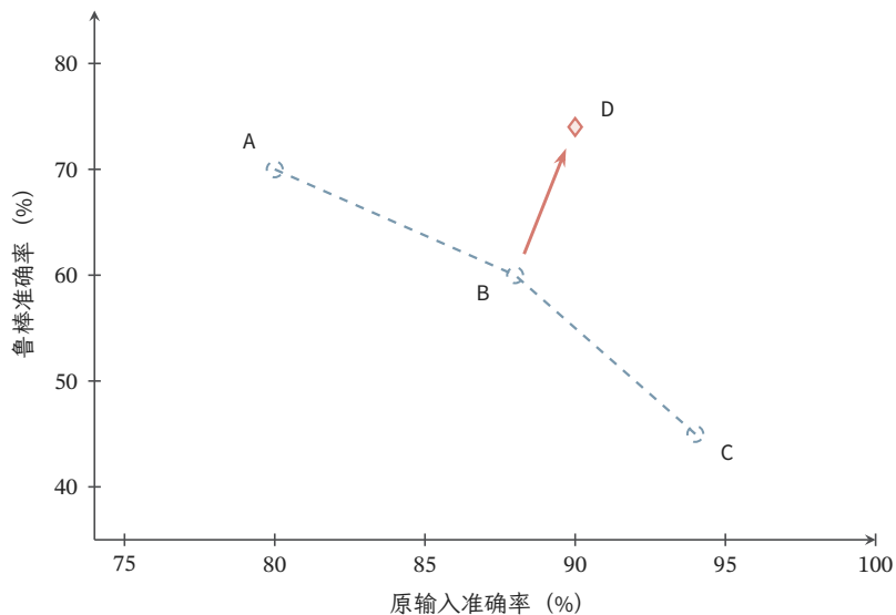
图 12.4 原输入准确率与鲁棒准确率的一种可能取舍。固定 100 个构造样本及同一标签保持扰动范围，A、B、C 的两项正确数分别为 80/70、88/60、94/45；D 为 90/74，同时优于 B。每个候选的鲁棒正确样本都是原输入正确样本的子集。虚线只连接三个教学候选，不是实测曲线或普遍最优边界；评价仍需固定扰动定义与搜索条件。
