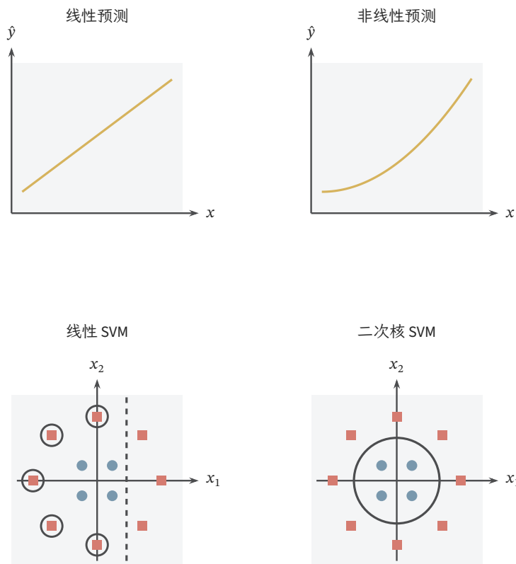
图 2.4 线性与非线性关系的几何示意。上排依次为线性预测与非线性预测，下排用同一组环形样本对照线性 SVM 的限制与二次核 SVM 的表达能力；圆点和方点代表两类。左图虚线只展示一条候选直线，空心圈标出按其左右类别分配时的错分方点，不代表最优 SVM 解。外圈方点的凸包包含内圈圆点，故任何直线都不能完全分离这组样本。右图以圆心为坐标原点，半径 8 的边界可由二次核 \kappa(\mathbf{u}, \mathbf{v}) = (\mathbf{u}^T \mathbf{v})^2 与偏置表示。图为几何构造，非训练结果。
