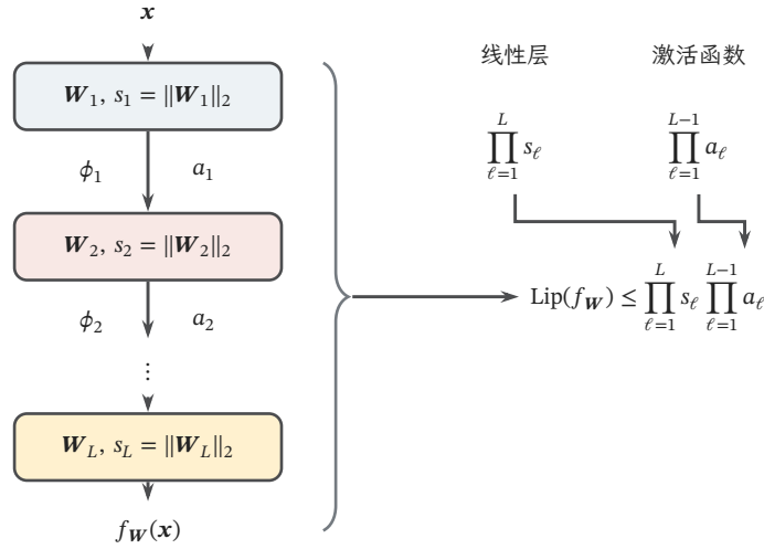
图 8.3 谱范数与激活函数共同控制输入扰动。第 \ell 层线性变换至多放大 s_\ell = \|W_\ell\|_2 倍，层间激活再至多放大 a_\ell 倍；末层为线性输出。右上方两类因子分别连到乘积上界，大括号归并各层作用。当激活均为 1-Lipschitz 时，只剩谱范数乘积；该乘积仍不是完整的泛化复杂度。
