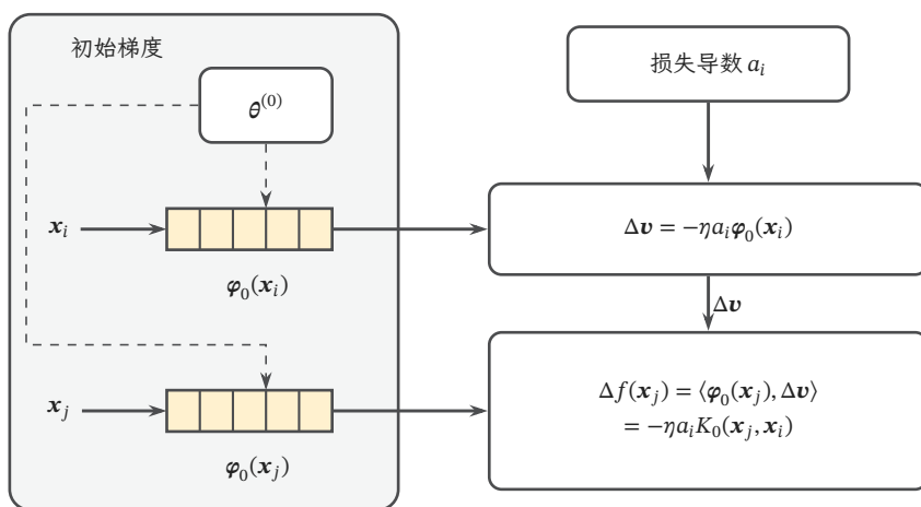
图 8.5 初始梯度特征如何传递一次训练更新。在线性化模型中, 样本 i 的梯度特征与损失对预测的导数 a_i 共同确定参数增量 \Delta \mathbf{v} ; 将同一增量与样本 j 的梯度特征作内积, 得到 \Delta f(\mathbf{x}_j) 。核值 K_0 正是两个初始梯度特征的内积。虚线把两份梯度关联到同一初始化, 特征条仅示意梯度坐标, 不限定参数维数。对真实有限宽网络使用固定特征, 还需控制核变化与线性化误差。
