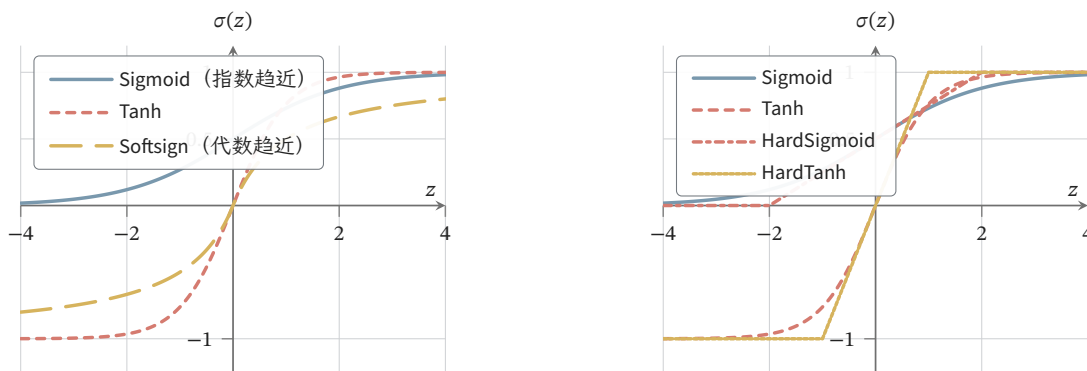
图 8.3 双侧饱和和激活函数。左图比较 Logistic / Sigmoid、Tanh 与 Softsign; Softsign 采用长虚线, 以便在黑白打印中仍能与 Sigmoid 区分, 图例同时指出前者按代数速度、后者按指数速度趋近渐近值。右图将 HardSigmoid 和 HardTanh 与对应平滑函数比较。 HardSigmoid 采用式(8.7)中的斜率 1/4 及截断点 \pm 2 。
