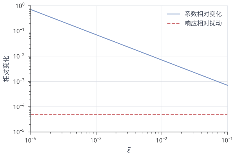
图 6.8 近共线矩阵的精确敏感性。固定 \mathbf{y}_0 = (2, 0)^\top ，扰动为 (0, 10^{-4})^\top ；红线是响应相对扰动 5 \times 10^{-5} ，蓝线是系数相对变化 10^{-4}/(\sqrt{2}\tilde{\varepsilon}) 。双对数坐标显示列越接近，反求系数越敏感；图中没有数值求解误差。
