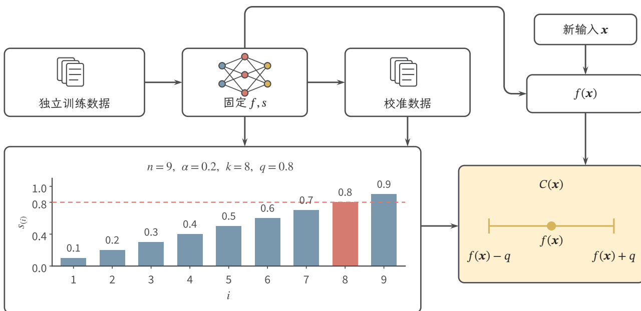
图 11.6 分割共形预测的构造。评分函数先由独立训练数据确定，再用校准分数选择阈值。图中采用教学残差 0.1, 0.2, \dots, 0.9 ，取 n=9, \alpha=0.2 ，故 k=8, q=0.8 ；绝对残差评分产生右侧回归区间。数值说明排序与集合构造，不是覆盖率的实验测量。
