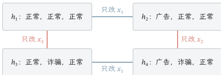
图 6.1 Natarajan 打散的四中预测。每个顶点的三项依次对应 x_1, x_2, x_3 。沿横向只改变第一封邮件的预测, 沿纵向只改变第二封邮件的预测; 第三封邮件始终预测为正常。每个输入的两个标签预先固定, 四个顶点实现全部组合。
