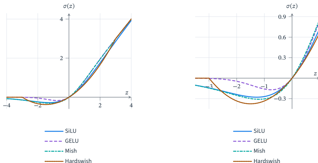
图 8.7 SiLU、GELU、Mish 与 Hardswish。左图展示整体响应，右图放大原点附近的负值和过渡区域；GELU 按标准正态累积分布函数采样。它们在正端接近线性，但负区间的形状和拐点不同。SiLU、GELU 与 Mish 平滑，Hardswish 含有分段边界；两图使用不同坐标范围以显示细节。
