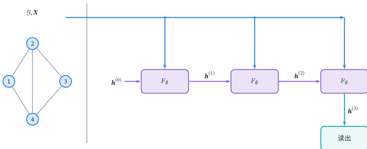
图 11.7 固定图上的循环更新。左侧表示邻接关系，右侧展开三轮共享更新 F_\theta ，每个状态向量包含整张图的节点状态。蓝色路径提供固定的图与输入特征，紫色路径传递状态，青色路径读出任务结果。轮次是内部计算步，不表示图已经发生三个时间点的变化。
