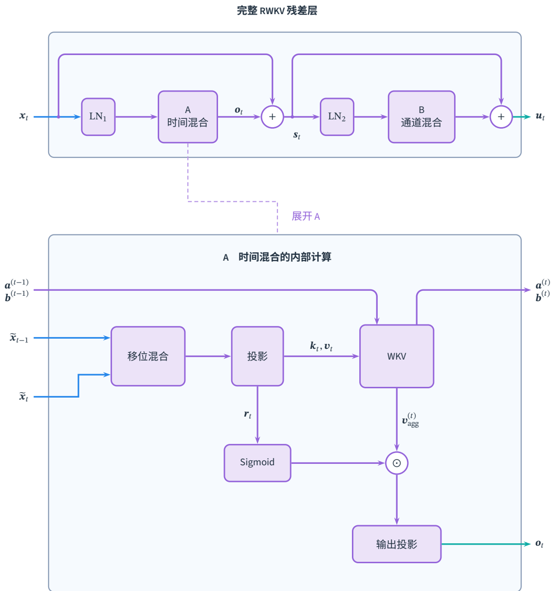
图 10.14 RWKV-4 的完整残差层与时间混合子模块。上方在 A、B 之前分别归一化，并在各子模块之后作残差相加，第一次相加得到 s_t 。下方只展开 A，无箭头虚线表示对应关系； \tilde{x}_t = \text{LN}_1(x_t) 是归一化后的特征。WKV 聚合值向量 v_t 与历史状态，经接收门和输出投影产生 o_t ，回到上方参与第一次残差相加。图中省略数值重缩放状态、移位缓存的保存箭头及 B 的内部计算。
