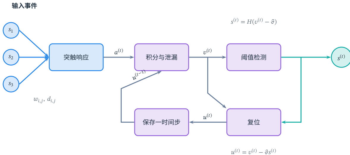
图 13.2 离散脉冲神经元的计算结构。蓝色输入事件经带权突触形成输入增量 a^{(t)} ，紫色模块完成积分、泄漏、阈值检测和复位，青色路径输出 s^{(t)} 。下方反馈保存复位后电位 u^{(t)} ，供下一步使用； v^{(t)} 为复位前电位。图表示本章的更新次序，不表示细胞的解剖结构；突触自身也可保存状态，见式(13.8)。
