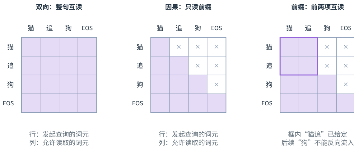
图 12.17 四个位置的读取范围。行表示查询位置 i ，列表示键位置 j ，着色格允许读取，带叉白格禁止读取。左为全部有效输入间的双向读取，中为 j \leq i 的因果读取，右为前两个位置构成条件前缀的读取：前缀内部双向，目标读取全部前缀与截至当前位置的目标输入。目标输入已移位，因此读取当前输入不等于读取当前待预测标签。
