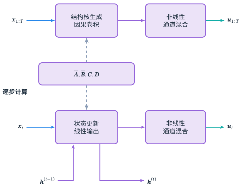
图 10.12 S4 层的整段与逐步计算。两个路径共享同一组离散状态参数及后续通道映射, 虚线表示参数供给。零初态时, 因果卷积与递推得到相同线性序列输出; 非零初态需要补上对应初态响应。图中 \mathbf{u} 是层输出特征, 任务预测还需相应读出。
