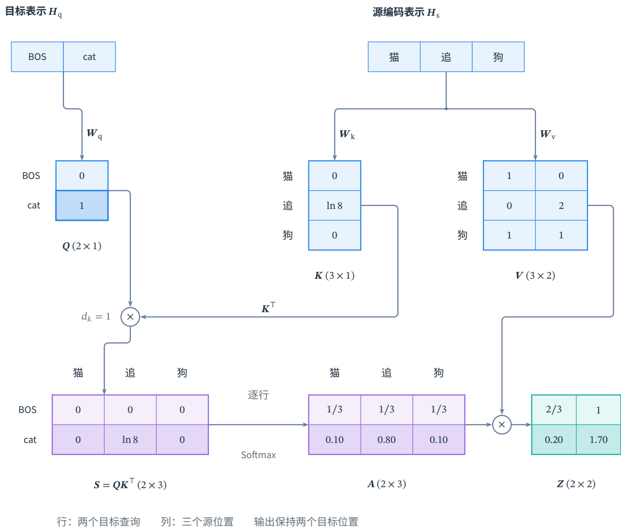
图 12.4 两条不同序列的交叉注意力。目标输入 BOS / cat 的状态投影为两行查询，源输入猫 / 追 / 狗的编码状态分别投影为三行键和值。得分与权重矩阵的行对应目标查询、列对应源词元，因此形状均为 2 \times 3 ；权重矩阵乘以 3 \times 2 的值矩阵后，输出为 2 \times 2 。较深的单元格突出 cat 这一目标位置从查询、评分、归一化到输出的对应关系。 d_k = 1 ，所有投影数值均为教学设定。
