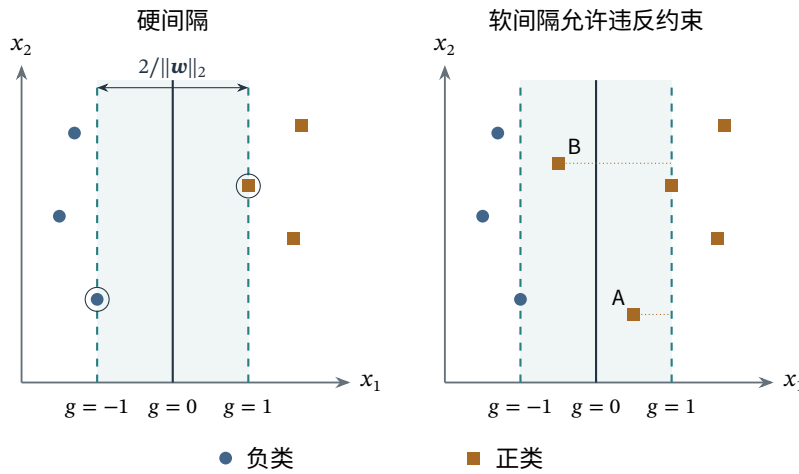
图 3.2 硬间隔与软间隔的教学示意，坐标无量纲。蓝圆为负类，赭方为正类；两个面板都给定 \mathbf{w} = (1, 0)^\top 、 b = -2 ，实线为 g = 0 ，虚线为 g = \pm 1 。单侧规范间隔为 1/\|\mathbf{w}\|_2 = 1 ，两虚线总宽为 2/\|\mathbf{w}\|_2 = 2 ；左图圈出间隔上的样本。右图 A 位于 x_1 = 2.5 ，正确分类但在间隔内， \xi_A = 0.5 ；B 位于 x_1 = 1.5 ，已被错分， \xi_B = 1.5 。右图仅说明给定分界面下的最小松弛量，并非优化后的 SVM 最优解。
