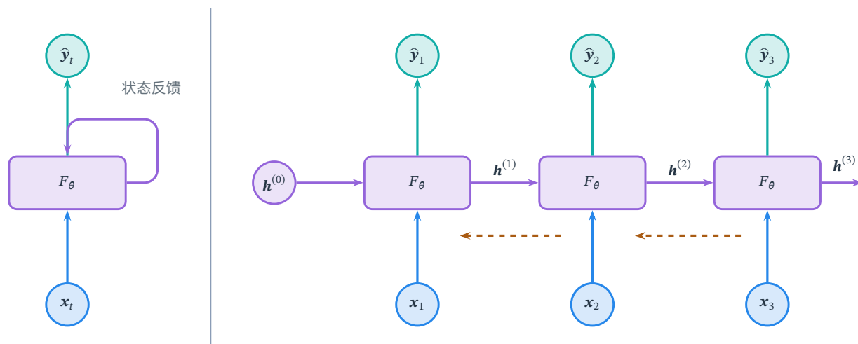
图 10.1 状态递推的紧凑表示与时间展开。蓝色节点提供当前输入，紫色方框计算隐状态，青色节点读出预测。展开图中的 F_\theta 是同一个更新函数的多次调用，参数共享而状态值不同。赭色虚线示意较晚损失沿状态依赖回传梯度；图中只画三个更新步。
