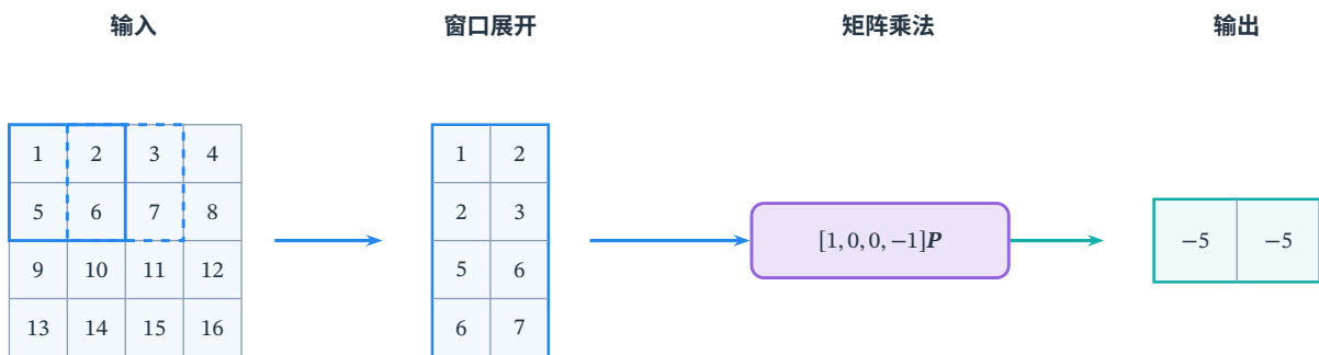
图 9.8 局部点积如何成为矩阵乘法。图中只取前两个相邻窗口，按核行、核列的顺序展平成 \mathbf{P} 的两列；核按相同顺序展平成一行。矩阵乘法同时得到这两个窗口的输出，完整计算包含九列。这里画的是代数上的窗口矩阵，是否实际复制全部数值由工程实现决定。
