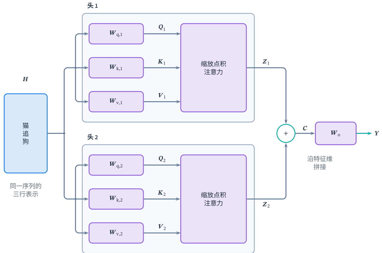
图 12.6 同一输入序列上的两个注意力头。每个头分别学习 W_{q,a} 、 W_{k,a} 和 W_{v,a} ，独立完成评分、归一化和加权聚合，得到 Z_a 。青色圆形 + 表示沿特征维拼接，两路输出的序列位置一一对齐；它不是残差相加。拼接矩阵 C 再经 W_o 投影，得到多头输出 Y 。各头的权重不直接平均，也没有预先指定的语法职责。
