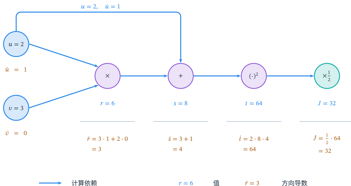
图 8.11 具体算子图上的前向模式。圆形节点表示乘法、加法、平方和缩放，蓝色实线沿原计算依赖传播；节点下方依次列出蓝色计算值和赭色方向导数。输入方向 (1, 0) 给出 \partial J / \partial u = 32 ；加法处的 \dot{s} = 3 + 1 包含了 u 的两条路径。
