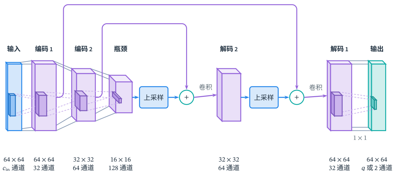
图 9.22 用于分割或着色的三尺度编码器—解码器。长方体表示特征张量，标签给出空间尺寸和通道数。每级解码先上采样到下一尺度，再由圆形 + 沿通道拼接同尺度的编码特征，随后卷积融合；上方旁路均接入拼接节点。图中上采样保持通道数，因此两次拼接分别得到 128 + 64 = 192 和 64 + 32 = 96 个通道，卷积后变为 64 和 32 个。输出头产生 q 个类别得分或两个颜色通道；采用 same 卷积，省略原始 U-Net 的裁剪。
