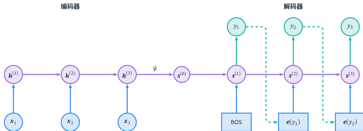
图 10.4 异步序列到序列。编码器读取三个源输入，解码器在初态 s^{(0)} 之后生成三个目标。BOS 启动生成，此前目标经嵌入反馈到下一步，青色虚线示意这一反馈。训练可使用真实目标，预测使用已生成目标；图中省略每步重复读取的固定上下文。
