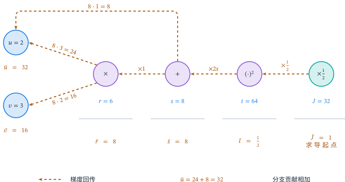
图 8.12 同一算子图上的后向模式。节点位置与前向模式相同，前向数值保持不变，赭色虚线从 \bar{J} = 1 开始回传敏感度；算子之间标出相应的局部导数。输入 u 收到经乘法传来的 24 和直接经加法传来的 8，累加为 32；输入 v 得到 16。一次后向遍历同时得到两个偏导。
