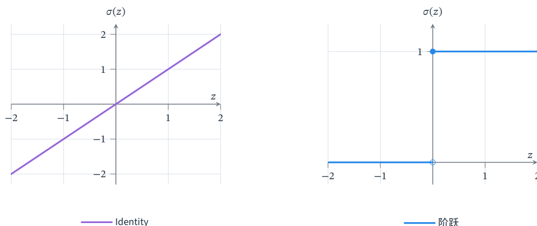
图 8.2 恒等函数与阶跃函数的比较。左图保留输入，斜率恒为 1；右图按零阈值输出 0 或 1，空心点和实心点区分 z = 0 两侧的端点约定。横轴为预激活值 z ，纵轴为输出；阶跃图中的跳跃不能通过普通局部导数传递学习信号。
