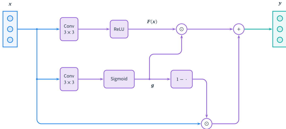
图 9.20 同形状卷积 Highway 模块。上方卷积与 ReLU 产生 F(x) ，门路径经卷积与 Sigmoid 产生 g ，蓝色保留路径传递原输入；两个 \odot 节点分别计算 g \odot F(x) 和 (1 - g) \odot x ，再由 + 节点相加。所有特征与门具有同一空间、通道形状，圆角方框表示各条路径的处理算子。
