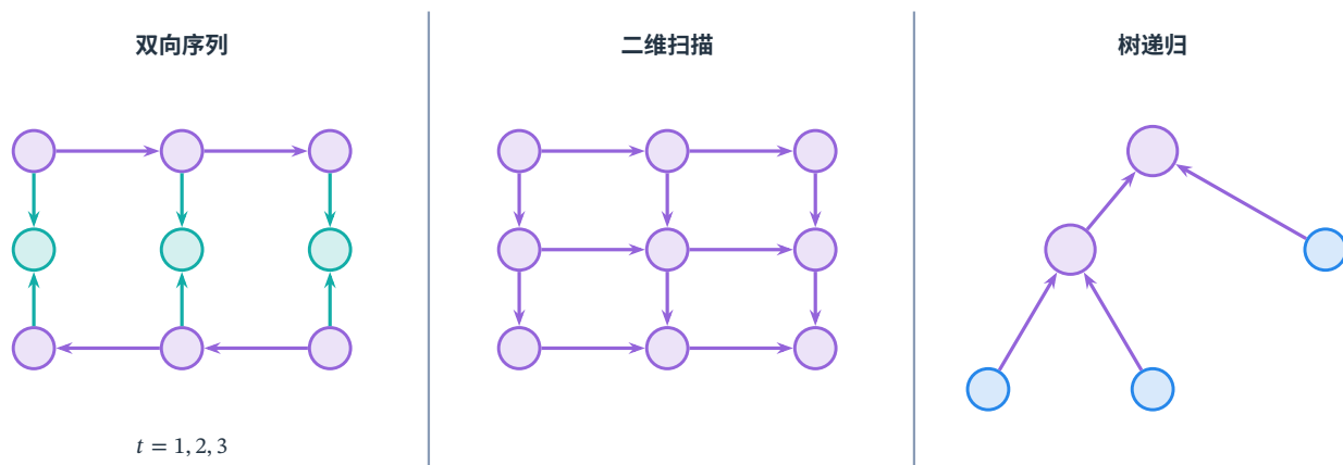
图 10.15 状态依赖拓扑。左图在同一输入位置组合正向与反向状态；中图由上方、左方前驱形成二维状态，箭头给出一个扫描方向；右图由叶节点向父节点组合子结构。紫色表示隐藏计算，青色节点表示组合读出。图中只表达依赖关系；不同方向、位置或孩子组合是否共享参数，需要由具体模型说明。
