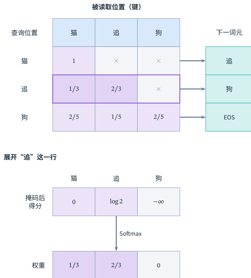
图 12.5 “猫／追／狗”的因果自注意力。行对应查询位置，列对应被读取的键；紫色格为可见位置的示例权重，浅灰叉号表示未来得分被设为 -\infty 、权重为 0。“追”这一行经后续网络计算用于预测右侧的“狗”，却不能读取“狗”的输入，因而预测目标与当前输入错开一步；EOS 为结束符。下方展开框出的这一行：先屏蔽未来得分，再在可见位置间归一化为 (1/3, 2/3, 0)。数值沿用前例，均为教学设定。
