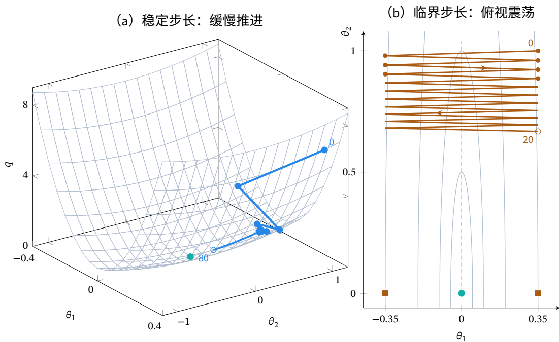
图 14.2 同一病态二次目标在两种步长下的轨迹，起点均为 (0.35, 1)^T ，青色点为极小点。(a) 三维图采用稳定步长 0.015，蓝色实心圆标出第 0–8 步，空心圆标出第 80 步；陡方向收缩快，谷底推进慢。(b) 俯视投影采用临界步长 0.02，橙线连接第 0–20 步，实心圆标出第 0–6 步，空心圆为第 20 步，箭头表示更新方向；灰线为等高线，竖虚线为谷底。左右摆幅保持 0.35，方点为奇、偶步各自趋向的位置，损失趋向 6.125 而无法达到原点处的 0。各轴使用所标范围，曲率比为 a/b = 100 。
