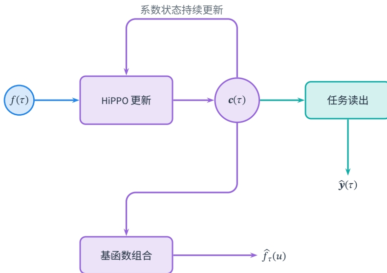
图 10.11 HiPPO 投影记忆与任务网络的一种组合。紫色反馈维护系数状态，青色读出产生任务预测；下方将同一系数与基函数组合，近似重构历史信号。HiPPO 本身规定记忆表示及更新，图中的任务读出与输入特征映射可另行学习，并非唯一的 HiPPO 网络架构。
