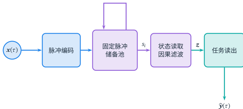
图 10.6 LSM 的输入、动态与读出。输入编码驱动固定的循环脉冲储备池，回路活动形成脉冲列 s_i(\tau) ；因果滤波将这些活动变成当前可读特征 \mathbf{z}(\tau) ，任务读出再映射为预测。紫色反馈表示回路动态，青色表示特征到预测的映射。此处只训练任务读出，脉冲编码、回路参数与滤波核按约定固定。
