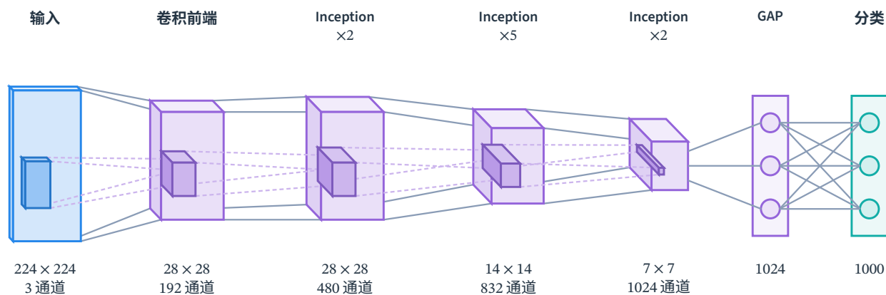
图 9.18 经典 GoogLeNet 的主分类路径。卷积前端把 224 \times 224 输入变成 28 \times 28 \times 192 ；两个、五个、两个 Inception 模块组成三个阶段，阶段间池化改变空间尺度。各阶段末的通道数为 480、832 和 1024，全局平均池化后接 1000 类分类器。辅助分类分支及模块内部细节省略，模块内部结构见图 9.17。
