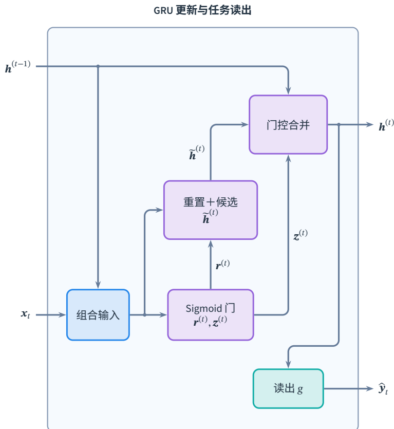
图 10.8 GRU 更新与任务读出。左侧输入为 x_t 和旧状态 h^{(t-1)} ，右侧输出为新状态与预测。组合输入将当前输入与旧状态一并送入门和候选模块。门模块作各自的仿射变换，得到重置门与更新门；候选模块先按重置门调节旧状态，再结合当前输入形成候选。门控合并按式(10.24)使用同一个更新门保留旧状态、写入候选，读出 g 另将新状态映射为任务预测。
