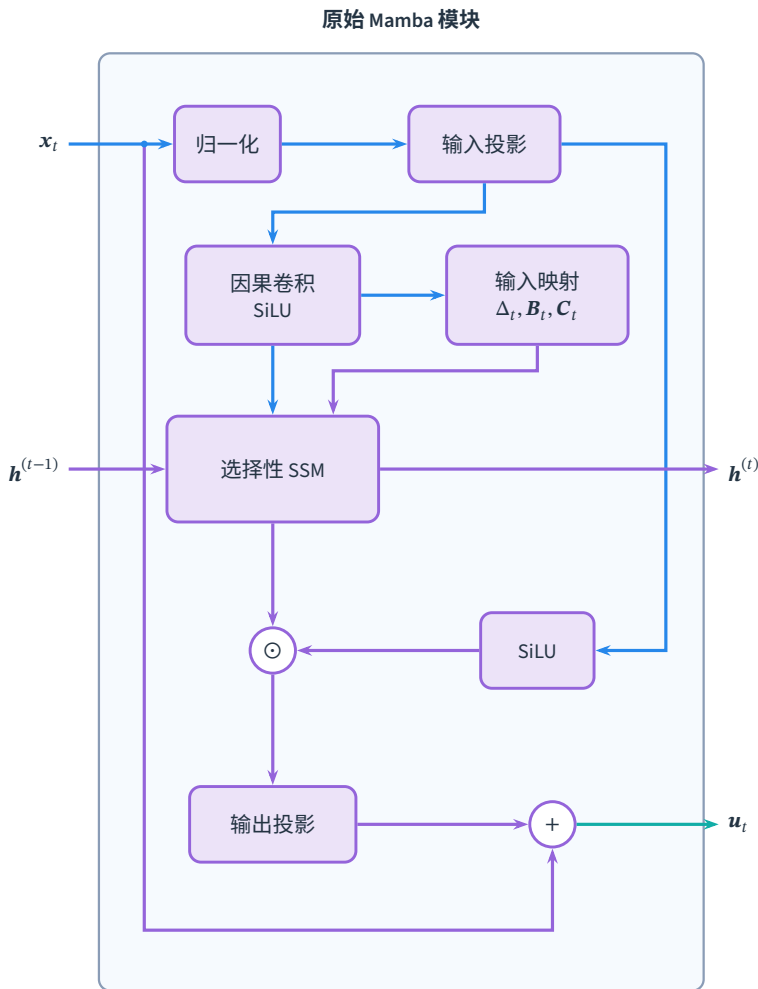
图 10.13 原始 Mamba 模块的主要计算路径。选择系数由短卷积后的输入特征产生，紫色状态从前一步传入并在右侧更新；另一路特征调制 SSM 输出，底部直达线完成跨层残差。 u_t 是模块输出，任务预测由后续网络读出。图中省略短卷积缓存、批次维和跨通道广播细节。
