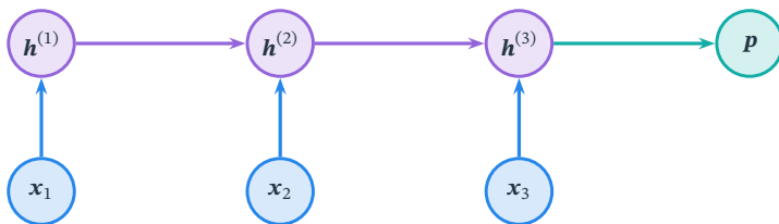
图 10.2 序列到分类。三个输入依次更新同一循环单元，末状态产生类别概率 \mathbf{p} 。蓝色表示输入，紫色表示隐状态，青色表示任务输出；图中只示意长度为 3 的序列。
