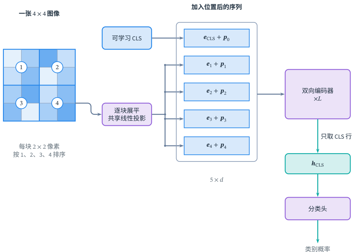
图 12.27 ViT 将图像组织为序列的过程。示意图像有 4 \times 4 个像素，切成四个 2 \times 2 图像块，按从左到右、从上到下的顺序编号；每块展平后通过同一线性投影形成 e_i 。在开头加入可学习 CLS 表示，为五行分别加入位置向量，再送入双向编码器。分类头只读取末层 CLS 行，其他图像块通过注意力参与其形成。图中像素色块仅为结构示意，并非真实识别样本。
