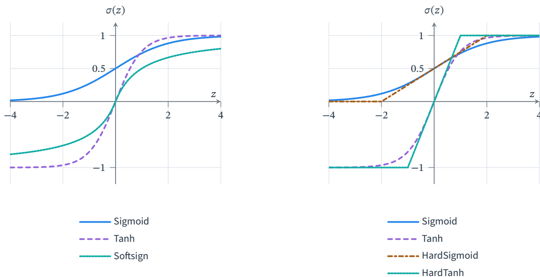
图 8.3 双侧饱和激活函数。左图比较 Logistic / Sigmoid、Tanh 与 Softsign；右图将 HardSigmoid 和 HardTanh 与对应平滑函数比较。HardSigmoid 采用式(8.7)中的斜率 1/4 及截断点 \pm 2 。各函数都限制输出范围，尾部趋近方式与梯度是否严格为零有所不同。
