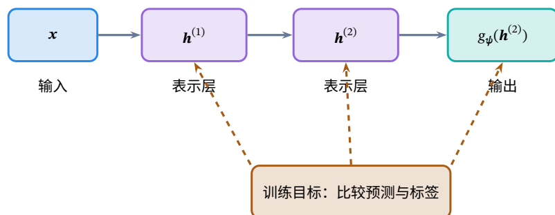
图 7.3 表示学习的一条计算路径。实线表示输入经过两层变换后交给输出映射，虚线表示同一个训练目标约束表示与输出两部分的参数。图只展示层间依赖，不要求隐藏坐标具有预先指定的语义，也不表示参数更新沿虚线完成一次普通前向计算。
