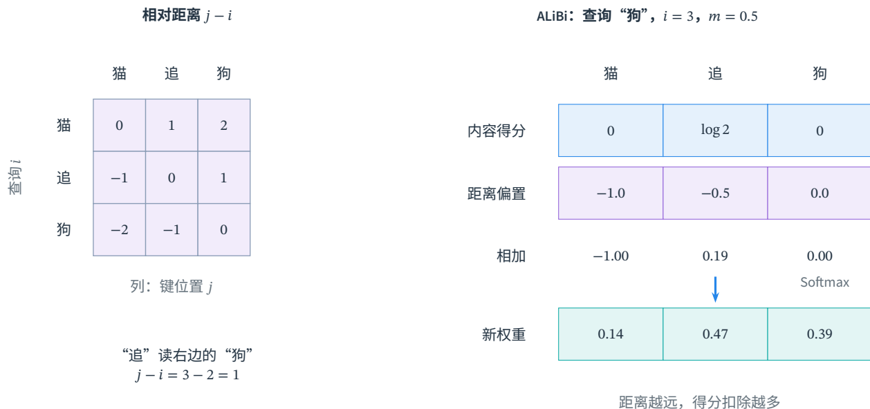
图 12.15 “猫/追/狗”的相对位置。左图行是查询位置 i 、列是键位置 j ，格内为 j - i ，正负号区分左右方向。右图取“狗”为查询、斜率 m = 0.5 ，演示 ALiBi 如何修正教学得分并重新归一化；显示数值保留两位小数，真实计算使用未舍入值。
