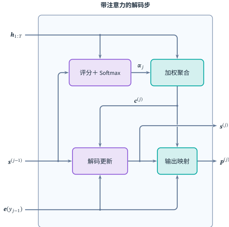
图 10.9 带注意力的一个解码步。左侧为保存的编码状态 h_{1:T} 、旧解码状态和此前目标的嵌入，右侧为新解码状态和输出概率。查询先用旧解码状态产生权重 \alpha_j = (\alpha_{j,1}, \dots, \alpha_{j,T}) ，上下文再进入更新与输出映射；输出映射还可读取目标嵌入。编码状态在各解码步重复读取，图中不重新执行编码器。
