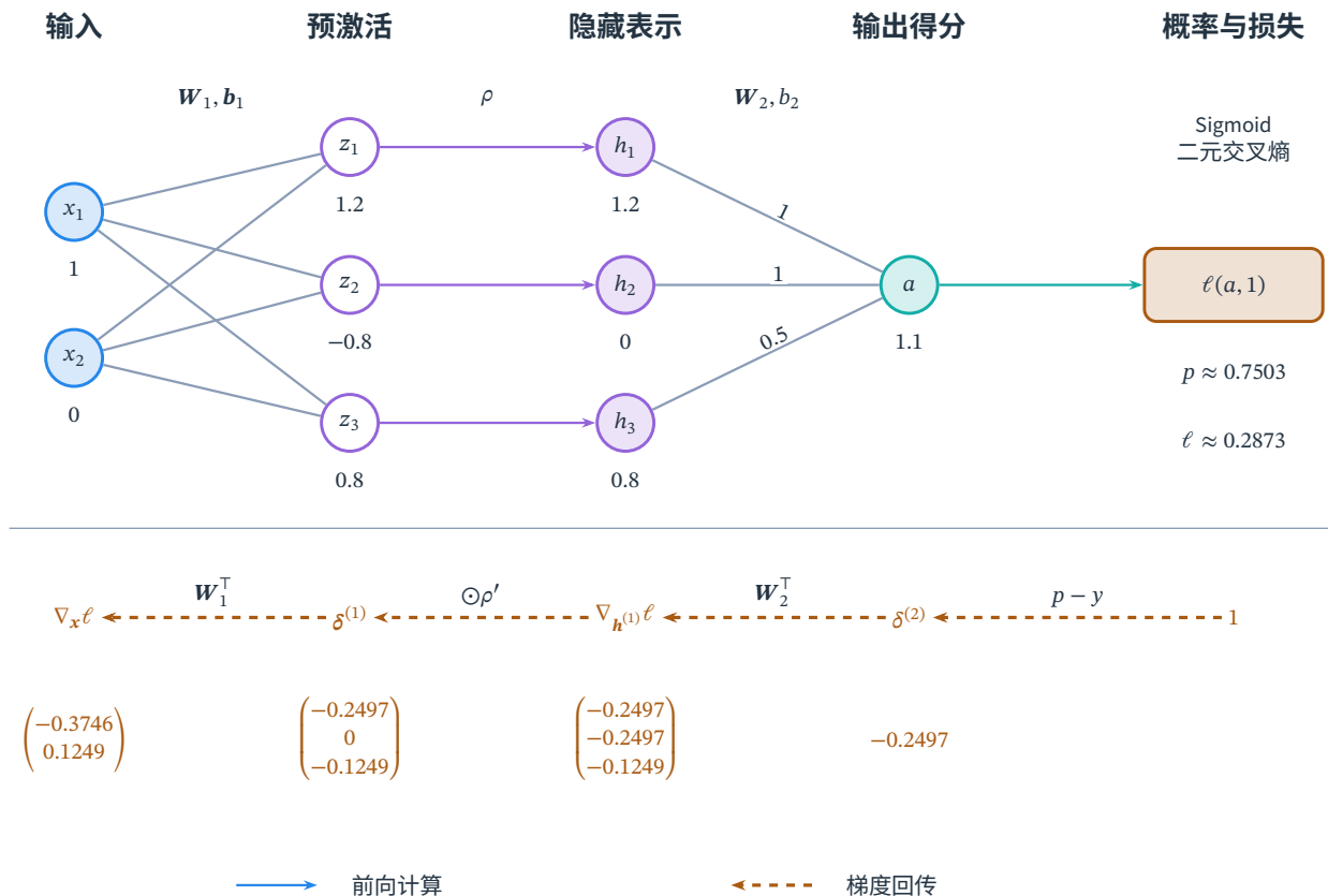
图 8.10 示例 8.1 中 2-3-1 网络的计算图。上方实线从两个输入经过三个 ReLU 单元，到达输出得分及二元交叉熵；预激活与隐藏表示是同一隐藏层的两种数值，不是两个隐藏层。下方赭色虚线反向传播梯度，向量坐标按上方节点从上到下排列。第三个单元通过输出权重 0.5 收到梯度，第二个单元的梯度被负半轴上的 ReLU 截断。数值按更新前参数计算，梯度和概率保留四位小数。
