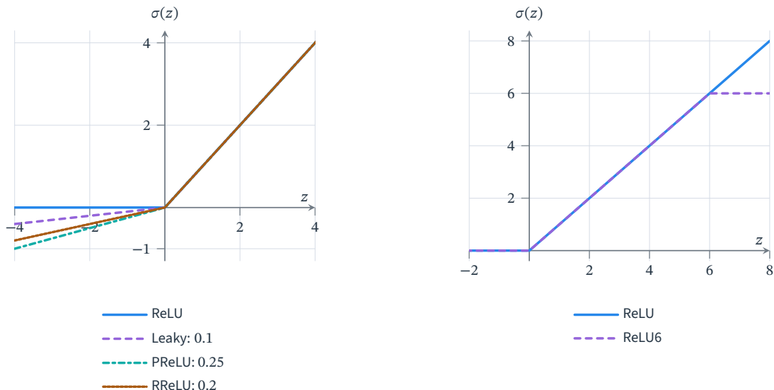
图 8.4 整流函数与负斜率变体。左图固定 Leaky ReLU 的 \alpha = 0.1 、PReLU 的 \alpha_j = 0.25 ，并以 \alpha = 0.2 画出 RReLU 训练阶段的一种可能曲线；三者的形状差异来自斜率选择，PReLU 与 RReLU 的区别主要在参数取得方式。右图比较 ReLU 与 ReLU6，展示 z > 6 时的截断。两图横轴范围不同。
