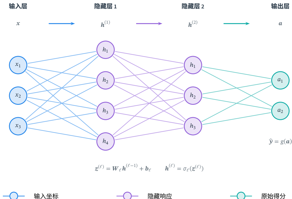
图 8.1 两个隐藏层的全连接前馈网络。蓝色圆点提供输入 x ，紫色圆点计算隐藏表示，青色圆点产生原始得分 a ，之后再使用任务规定的输出变换 g 。细线表示可学习的连接，层间箭头标明前向计算方向；每个目标单元还具有一个未画出的偏置。图中层宽依次为 3, 4, 3, 2，只是结构示例。
