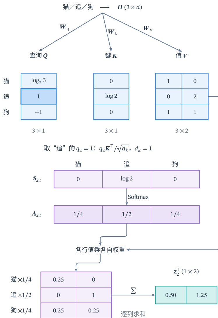
图 12.2 展开“追”的一次缩放点积注意力。输入分别经三组投影产生查询 Q 、键 K 和值 V ，三者各行依次对应猫、追、狗。突出显示的查询为 q_2 = 1 ，与全部键匹配得到三个得分。Softmax 产生权重后，下方三行分别列出各值向量的加权贡献，逐列求和得到 \mathbf{z}_2^T = (0.50, 1.25) 。蓝格表示投影数据，紫格表示中间结果，青格表示输出； d_k = 1 、 d_v = 2 ，数值均为教学设定。
