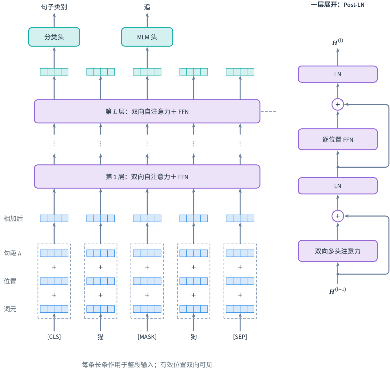
图 12.10 BERT 的双向编码器与预测位置。每列的词元、位置、句段嵌入逐元素相加，本例同属句段 A；向量格条只示意特征维。每个长条是一整层双向自注意力与 FFN 计算，能够在所有有效词元之间交换信息，中间层省略。MLM 头在遮蔽位置恢复“追”，CLS 分类头用于任务适配；两者不要求同时使用。右侧展开一层的 Post-LN 与残差，省略输入归一化、Dropout 与 NSP 头。参考 Bishop 与 Bishop (2024) 图 12.18 的整序列布局重绘，输入与训练目标依据 Devlin 等 (2019)。
