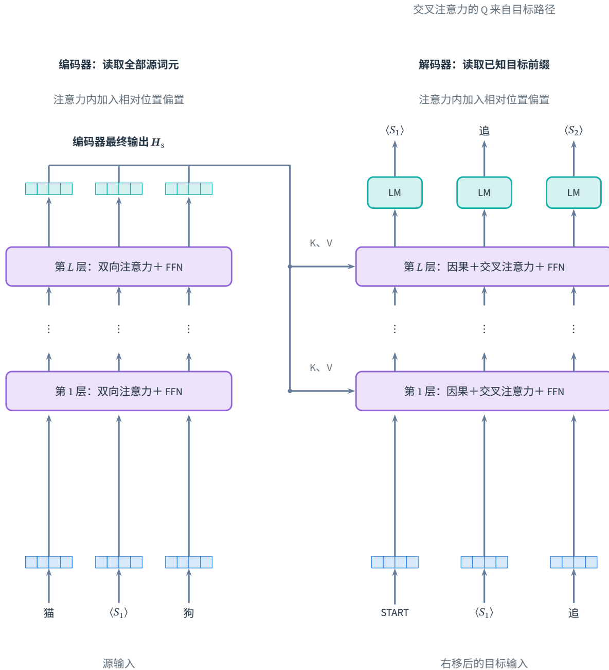
图 12.13 T5 的片段恢复任务与整网结构。 \langle S_1 \rangle 替代源句中被删去的片段，目标中的同名标记引出该片段， \langle S_2 \rangle 标记恢复序列的结束；右侧输入已右移，START 表示解码起始符。每个长条是一整层，编码器最终输出供各解码层的交叉注意力生成 K、V。注意力内部使用相对位置偏置，输入不叠加绝对位置向量。省略层内残差、Pre-LN、Dropout 与末尾 EOS。参考 Bishop 与 Bishop (2024) 图 12.20 的布局重绘，结构与任务依据 Raffel 等 (2020)。
