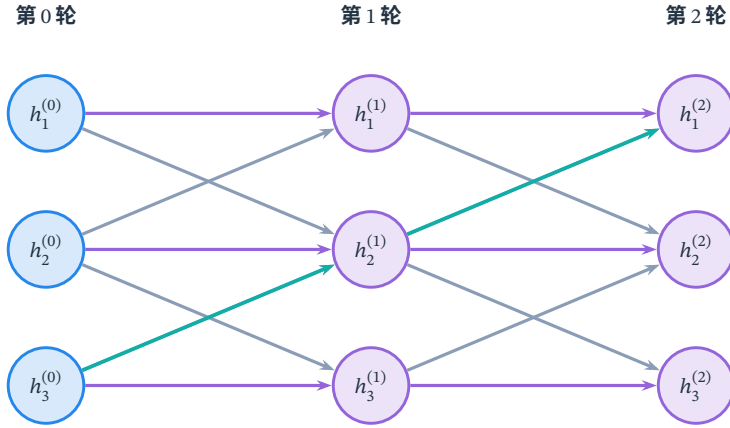
图 11.2 三节点路径上的同步传播。每列是一轮，横向实线传递自身状态，斜线沿原图的相邻关系传递状态。两轮后，节点 3 的初始特征可经节点 2 影响节点 1；同一列内没有即时传播，因此一次更新不能直接读取两跳之外的新信息。
