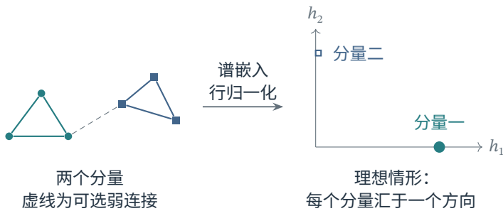
图 4.6 谱聚类的理想情形：圆形与方形分别标识两个互不连接的分量，颜色只作辅助；在归一化谱空间中，两个分量分别落到两个方向。细虚线表示实际数据中可能存在的弱连接；加入这些连接后，谱坐标通常形成近似群组。
