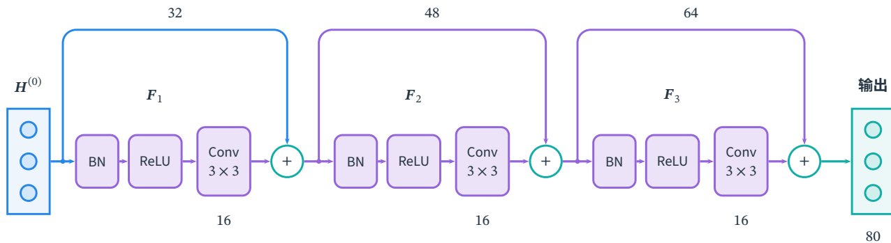
图 9.21 DenseNet 的三层教学密集块。各 F_\ell 依次执行 BN、ReLU 和 3 \times 3 卷积，保持 32 \times 32 空间网格并新增 16 个通道。三次变换分别读取 32、48、64 个通道；上方旁路保留变换前的全部特征，标出的 32、48、64 为累计通道数；卷积下方的 16 为新增通道数。圆形 + 将新旧特征沿通道拼接，最终得到 80 个通道。逐次累积拼接等价于保留并向后传递全部先前层的输出，不作逐元素相加。
