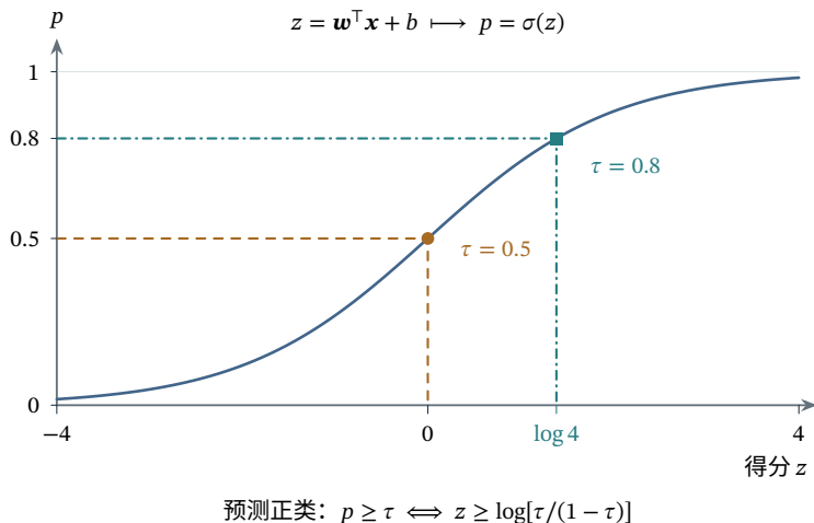
图 3.6 线性得分 z = \mathbf{w}^\top \mathbf{x} + b 经 Logistic 函数转为正类概率 p 。蓝色实线为 p = \sigma(z) ；赭色虚线与圆点标出 (0, 0.5) ，青色点划线与方点标出 (\log 4, 0.8) 。两组辅助线分别连接概率阈值与对应的得分阈值，数值是教学构造，不表示训练或校准结果。
