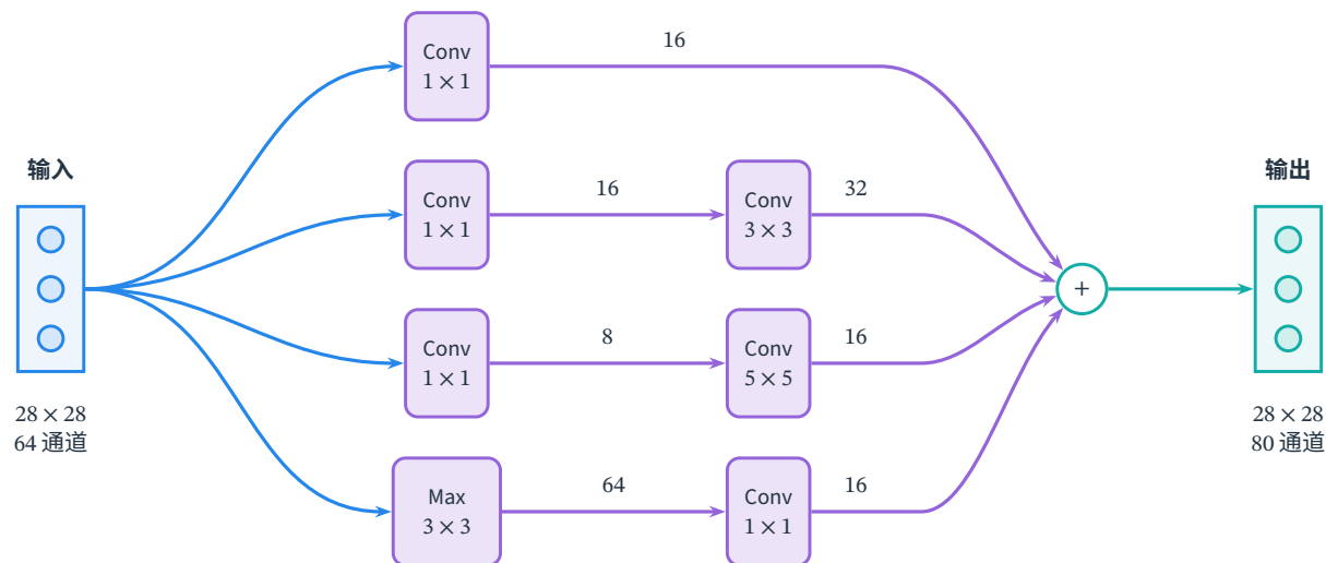
图 9.17 一个 Inception 模块的四分支教学配置。输入为 28 \times 28 \times 64 ；四条分支分别输出 16、32、16、16 个通道，保持同一空间尺度，拼接得到 28 \times 28 \times 80 。中间的逐点卷积先压缩通道，最大池化采用步长一及 same 填充。圆角方框表示处理算子，Max 为最大池化，线路上的数字为通道数；圆形 + 表示沿通道拼接，四条路径实际并行，激活省略。
