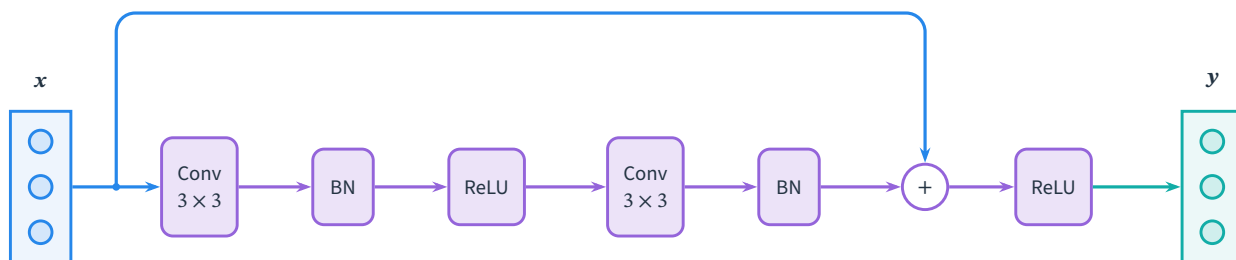
图 9.19 残差基本模块中的逐层变换与恒等旁路。主分支依次经过 3 \times 3 卷积、BN、ReLU 及第二个 3 \times 3 卷积、BN，再与直接传来的输入逐元素相加并激活。两次卷积均保持 32 \times 32 \times 64 形状，上方蓝色旁路跳过主分支的变换。圆角方框表示算子，圆形加号节点表示逐元素相加；改变尺度或通道时，旁路需要投影。
