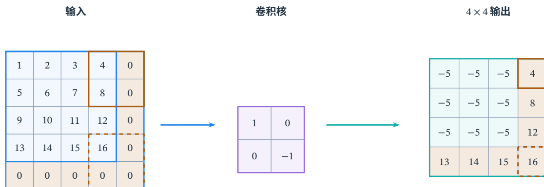
图 9.3 不对称零填充与边界输出。蓝色框内是原 4 \times 4 输入，浅橙色区域是右侧、下侧各新增的一列、一行零。橙色实线窗口产生右上输出 4，虚线窗口产生右下输出 16，输出矩阵中用相同线型标记对应位置。核为 (1, 0; 0, -1) ，步长一、空洞率一，计算采用互相关。
