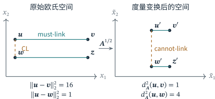
图 4.10 度量如何改变成对关系的几何表达。四点为 \mathbf{u} = (-2, 0.5) 、 \mathbf{v} = (2, 0.5) 、 \mathbf{w} = (-2, -0.5) 、 \mathbf{z} = (2, -0.5) 。实线连接 must-link 对，虚线连接 cannot-link 对（左图简记 CL）。这里人为设定 \mathbf{A} = \text{diag}(1/16, 4) ；右图的距离等于左图的 Mahalanobis 距离，不表示一次真实训练的结果。
