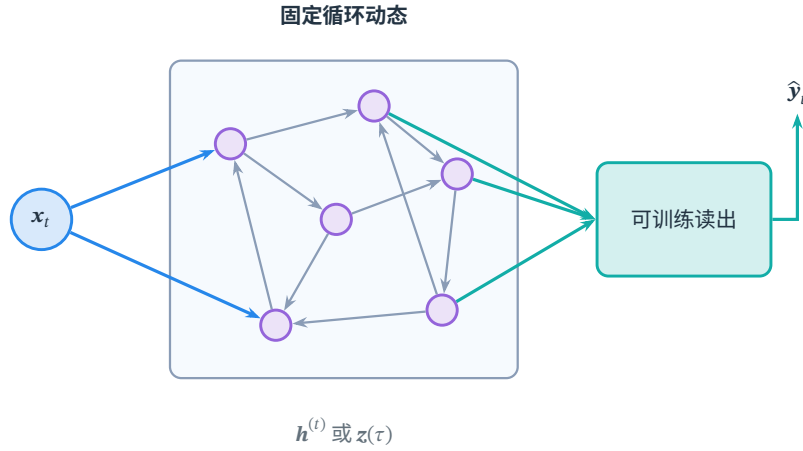
图 10.5 储备池计算的参数分工。输入进入固定的循环动态，多个内部单元共同形成随历史变化的状态，可训练读出将状态映射到目标。灰蓝连线表示固定连接，青色箭头表示参与拟合的读出；内部连接只示意结构，不表示某个随机生成样本。ESN 使用连续值激活，LSM 可由脉冲活动及其滤波响应形成读出特征。
