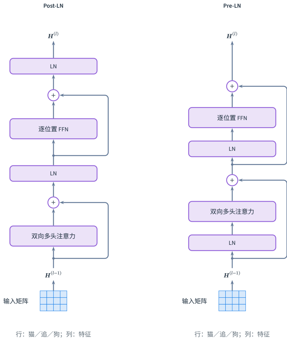
图 12.7 Post-LN 与 Pre-LN 编码器块的计算次序。底部矩阵的三行对应“猫／追／狗”，列示意特征维度，格子数不代表实际宽度。自注意力在行间交换信息，FFN 分别变换各行；圆形 + 表示逐元素残差相加，侧路圆点表示分支。省略 Dropout 与 Pre-LN 堆叠末尾的归一化。参考 Bishop 与 Bishop (2024) 图 12.9 的层内布局重绘，并增加 Pre-LN 对照。
