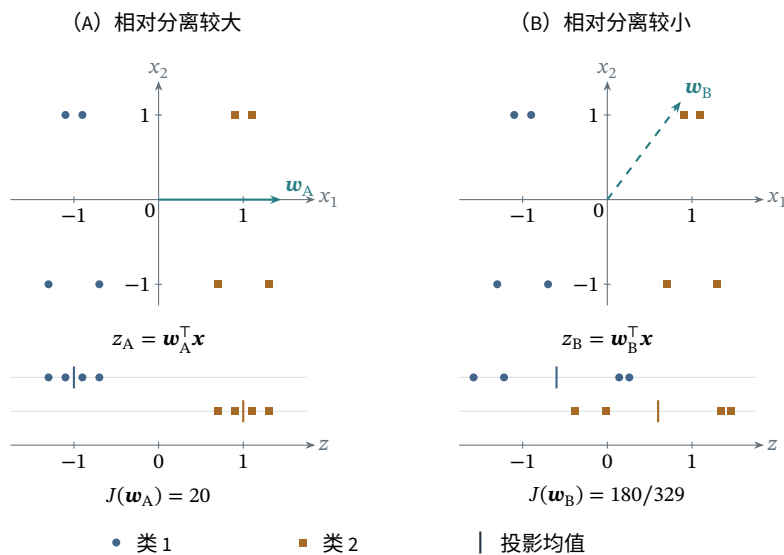
图 3.1 同一点集在两个单位方向上的投影。两类各有 4 点，中心分别为 (-1, 0)^T 、 (1, 0)^T ，都加上偏移 (-0.3, -1)^T 、 (-0.1, 1)^T 、 (0.1, 1)^T 、 (0.3, -1)^T ；这是人为构造，坐标无量纲。蓝圆为类 1，赭方为类 2，青色箭头分别表示 \mathbf{w}_A = (1, 0)^T 与 \mathbf{w}_B = (3/5, 4/5)^T ，并以实线、虚线区分。下方按 z = \mathbf{w}^T \mathbf{x} 计算投影，两类分行显示，纵向位置只为避免遮挡；短竖线标出各类投影均值，两面板共用数轴尺度。
