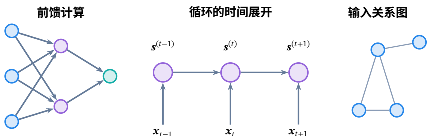
图 7.8 三种不同对象的结构示意。左侧是前馈计算中的单元依赖；中间是循环更新的时间展开，三个更新位置共享同一组状态更新参数；右侧是供图神经网络使用的输入关系图，节点表示数据中的实体，边表示输入中的关系。右图的无向环不等于一次计算中的循环依赖。
