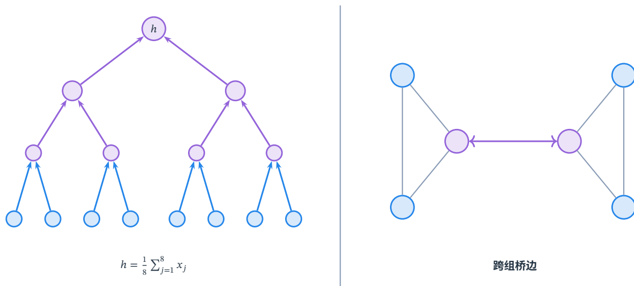
图 11.9 两种信息汇聚瓶颈。左侧八个叶子经三层平均进入一个根状态，每个叶子的影响系数为 1/8 ；右侧两组节点的跨组信息必须经过一条桥边。紫色表示承担汇聚或跨组传递的状态，蓝色表示外围输入。图不要求所有状态相同，强调的是大量信息必须经过较少的表示通路。
