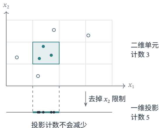
图 4.7 CLIQUE 的投影计数示意。二维高亮单元含三个样本，其在横轴区间上的投影还包含其他纵坐标范围的样本。取共同阈值 \tau = 3 ，二维单元密集必然推出对应一维单元密集，反方向则不成立。
