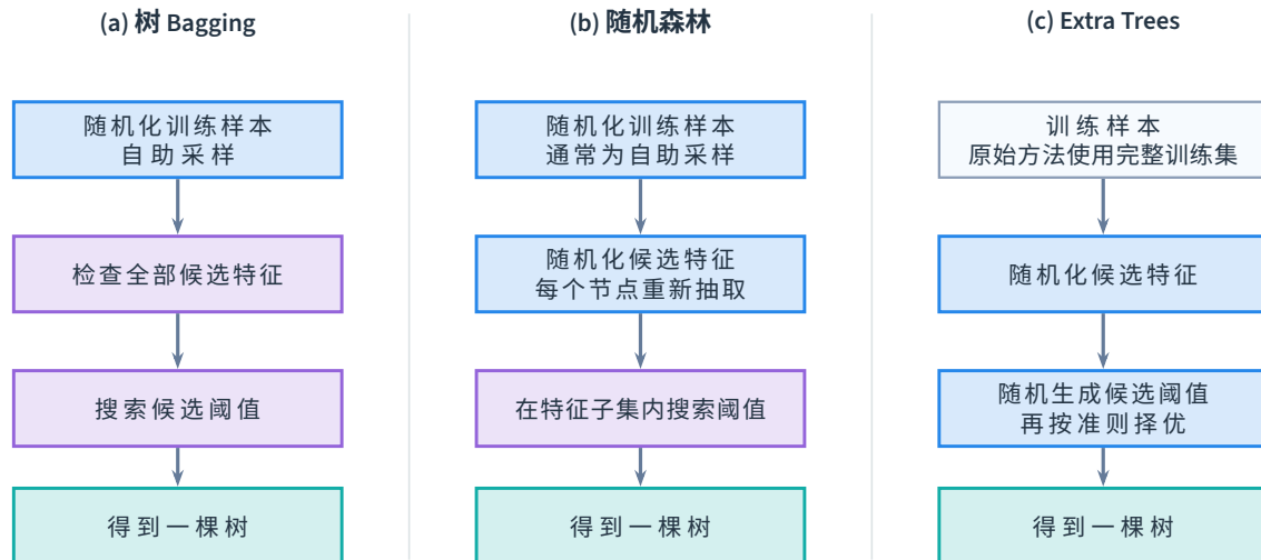
图 6.4 树 Bagging、随机森林与 Extra Trees 的随机化位置。蓝色节点表示引入随机性的环节，紫色节点表示仍按任务准则执行的搜索，青色节点表示得到的成员树。Extra Trees 面板采用原始方法的完整训练集设定；具体实现也可能额外启用自助采样。
