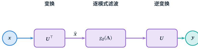
图 11.5 谱滤波的计算路径。节点信号 \mathbf{x} 经 \mathbf{U}^T 分解为图傅里叶系数，每个模式由 g_\theta(\lambda_k) 调整，再经 \mathbf{U} 还原为节点信号。左、右两端使用同一张图和同一节点顺序；中间向量的下标表示频率模式。
