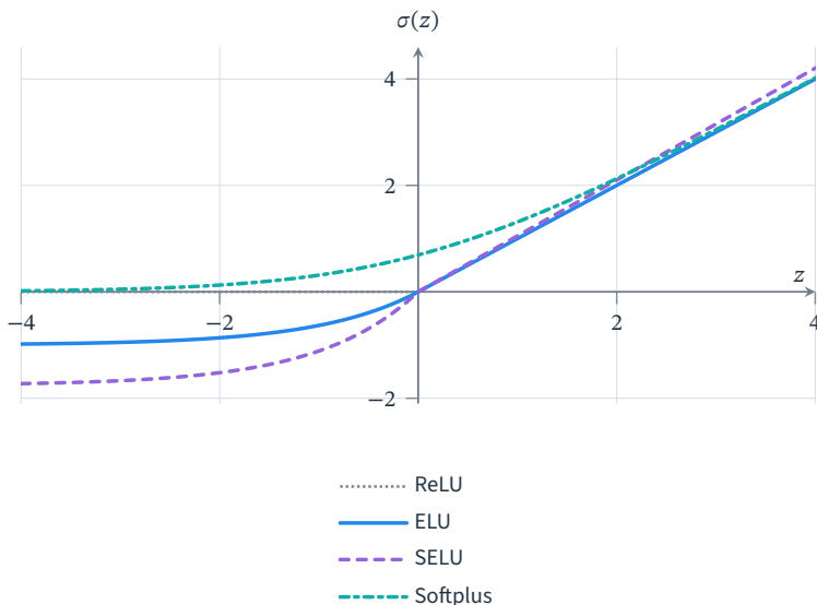
图 8.5 ELU、SELU 与 Softplus 的响应。ELU 使用 \alpha = 1 ，SELU 使用式(8.12)中的常数，ReLU 作为共同参照。ELU 与 SELU 允许负输出并在负端趋向有限下界；Softplus 始终为正，且平滑地趋近正半轴上的线性响应。
