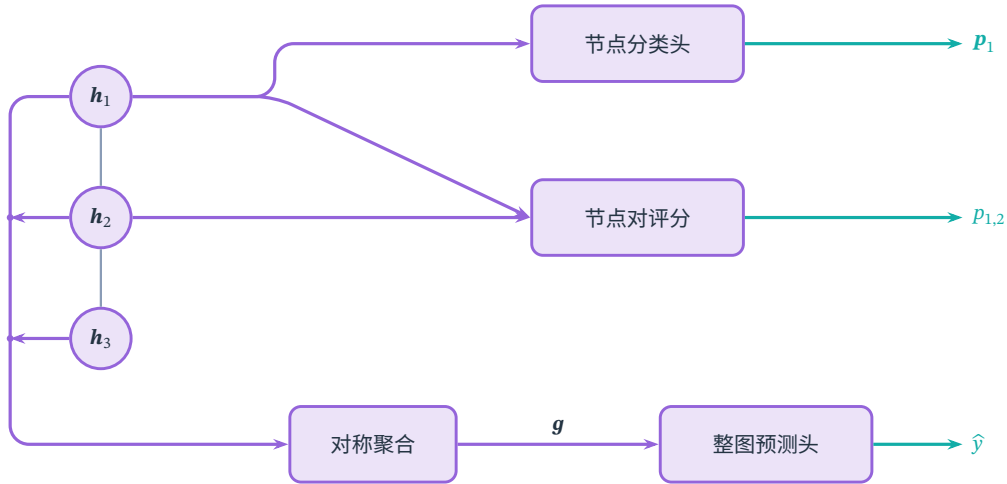
图 11.3 同一组节点表示的三种任务读出。节点预测读取一个节点，边或连接预测读取两个端点及可用的关系属性，整图预测先对全部节点作对称聚合。紫色表示编码后的节点状态，青色表示任务输出；三个分支示意不同任务，不要求一个模型同时使用全部分支。
