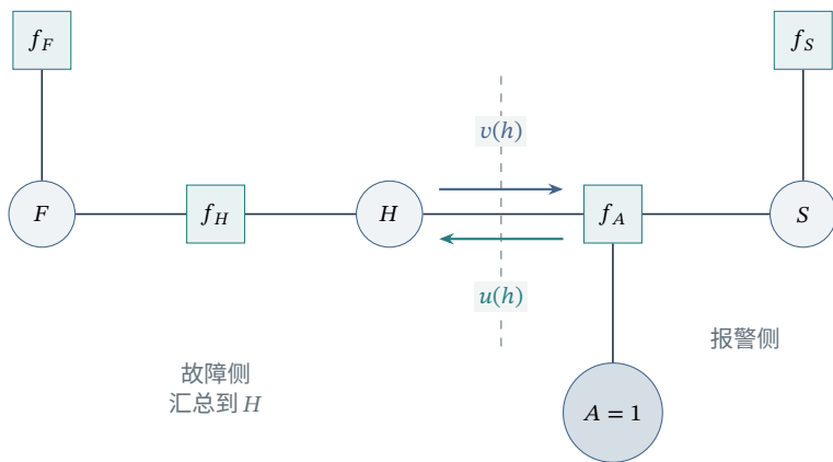
图 21.1 报警模型的树状因子图。圆表示变量，方框表示因子； A = 1 作为变量处的证据。虚线切断 H 与 f_A 之间的边，蓝色与青色箭头分别表示两侧汇总得到的 v(h) 和 u(h) ，不是原有向图的因果箭头。
