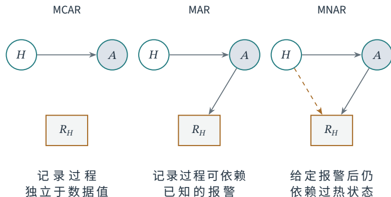
图 24.2 固定已观测的 F, S 后, 温度记录指示量 R_H 的三种示意机制。A 总是观测, H 在 R_H = 0 时不可见。中图的缺失概率只依赖已知报警; 右图在给定报警后仍允许依赖未记录的过热状态。右图需有实际的剩余依赖才属于 MNAR, 单凭箭头存在不能排除参数抵消。
