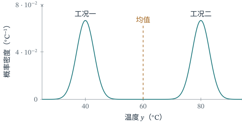
图 16.1 同一个双峰预测分布可以产生均值为 60°C 的点预测。实线为两个等权高斯密度的混合，每个分量的标准差为 3°C；虚线标出均值。点预测没有保留两个高概率区域的位置。
