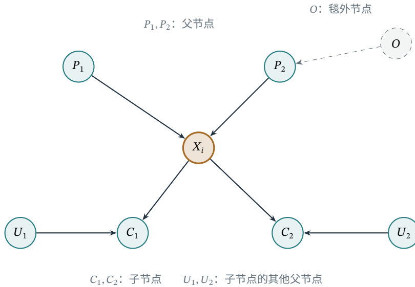
图 17.2 有向图中节点 X_i 的 Markov 毯。青色节点构成 \text{mb}(i) ： P_1, P_2 是父节点， C_1, C_2 是子节点， U_1, U_2 是子节点的其他父节点；虚线节点 O 位于毯外。
