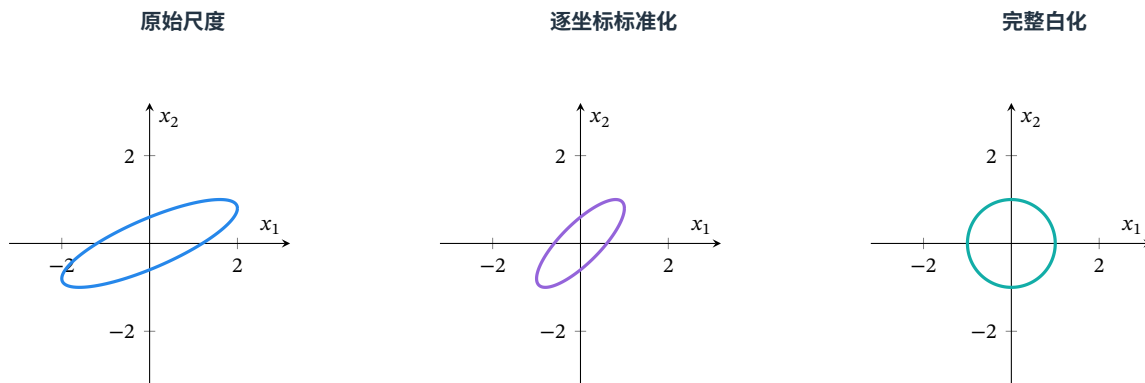
图 14.3 以 \mathbf{C} = \begin{pmatrix} 4 & 1.6 \\ 1.6 & 1 \end{pmatrix} 构造二维协方差椭圆。左图为原尺度，中图分别除以各坐标标准差，边际尺度相同但相关系数仍为 0.8；右图用精确逆平方根白化后成为圆。曲线是解析示意，不是抽样散点或实验结果；忽略稳定项且不加入可学习仿射。
