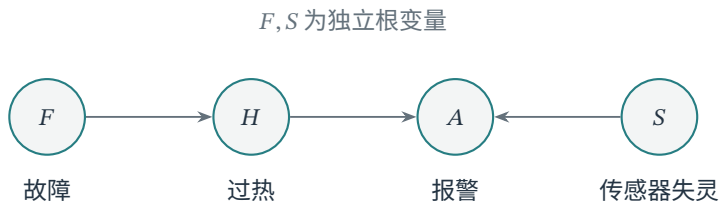
图 16.2 设备诊断模型。节点表示随机变量, 箭头指向局部条件分布所描述的变量, 例如 H \rightarrow A \leftarrow S 对应 p(a | h, s) 。箭头指定概率分解, 不自动具有因果含义。
