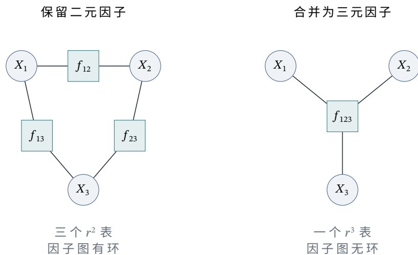
图 19.5 相同联合函数的两种因子图。左图保留三个二元因子，右图用 f_{123} = f_{12}f_{23}f_{13} 将其合并。两图对应的无向变量图都是三角形；因子图的环结构和因子规模却不同。
