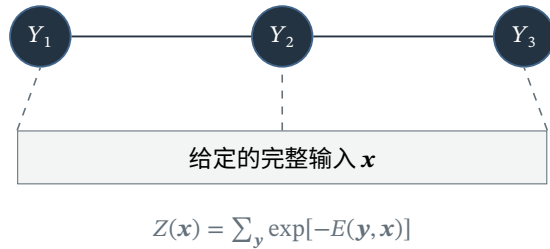
图 27.1 相同的三节点相互作用可以用于联合或条件建模。上图对整组状态求和；下图固定输入 \mathbf{x} ，只对标签 \mathbf{y} 求和。虚线表示输入参与势的计算，不是概率图中的有向生成边。
