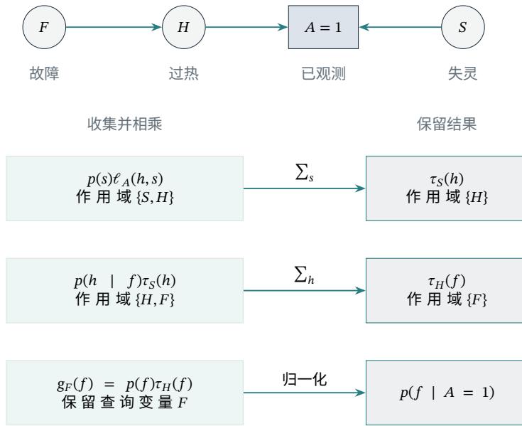
图 20.1 报警查询的局部消元。上部为原有向图，方形节点表示已观测的 A = 1 ；下部按 S, H 的顺序汇总因子。每一行的输出不再包含被消去的变量，查询变量 F 一直保留。
