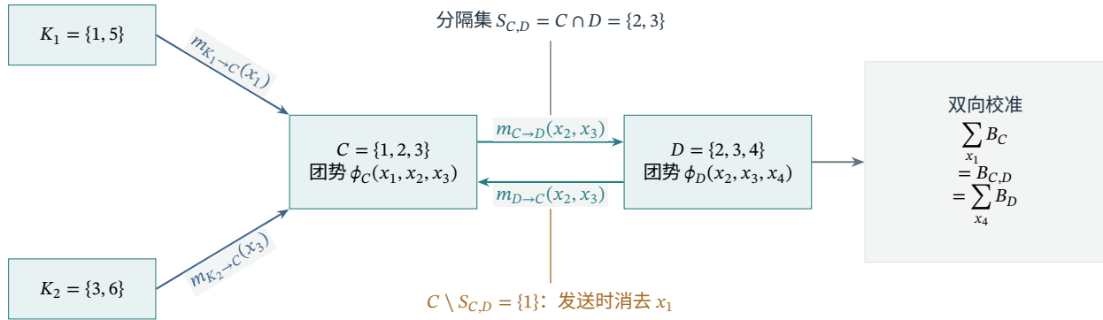
图 21.4 团间消息的组成与双向校准。蓝色箭头是 C 收到的入站消息，团势与这些消息相乘后，对 C \setminus S_{C,D} = \{1\} 中的 x_1 求和，得到定义在分隔集 \{2, 3\} 上的 m_{C \rightarrow D} ；发送时排除接收方 D 的入站消息。青色双向箭头分别汇总树边两侧的贡献，收集与分发都完成后，两个团消去非共享变量所得的表均等于分隔集势 B_{C,D} 。
