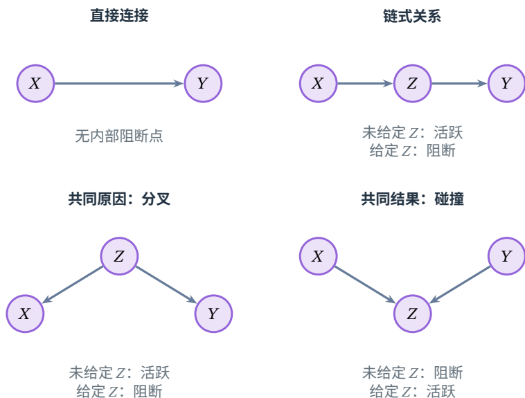
图 17.3 四种基本关系及给定中间节点前后的变化。每个面板只含所画节点和边；链、分叉由活跃变为阻断，碰撞路径则由阻断变为活跃。活跃表示这条路径不再保证两端独立，并不保证任意参数下都实际相关。在更大的图中，碰撞节点的后代被给定也能打开该碰撞位置。直接连接没有内部节点，不能靠给定其他节点阻断这条边。
