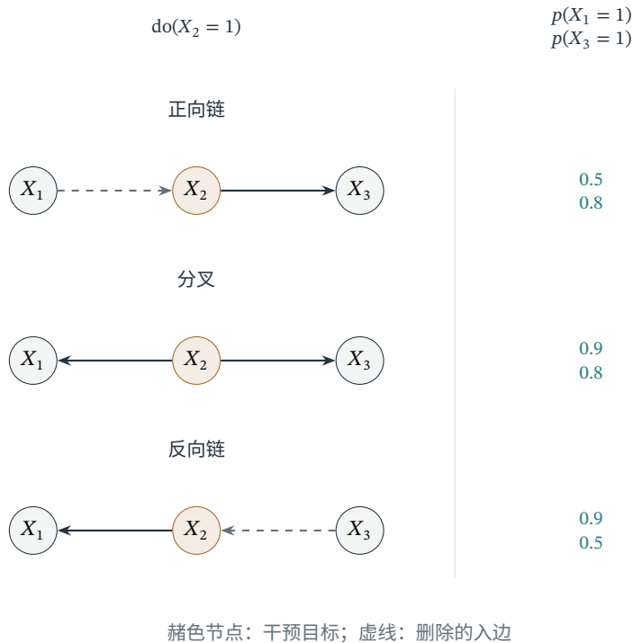
图 25.3 同一观测 MEC 在干预 X_2 后产生不同预测。实线箭头为干预后的保留边，虚线边被切断；右侧给出外部固定 X_2 = 1 时的两端边缘概率。在该三节点例子及给定假设下，这些预测足以区分三个方向。
