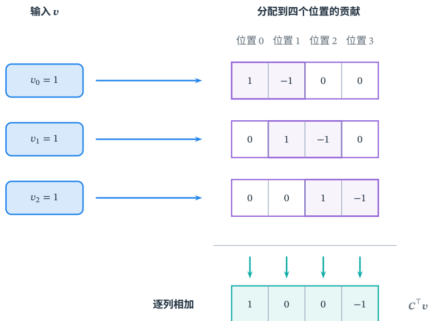
图 9.7 转置卷积的分配与累加。输入为 \mathbf{v} = (1, 1, 1)^T , 核为 (1, -1) , 步长一、无填充。每行分别表示一个输入值对四个输出位置的贡献, 紫框圈出两个可能非零的位置; 没有贡献的格子记为零。逐列相加得到 (1, 0, 0, -1)^T , 中间两格均包含来自不同输入的重叠贡献。
