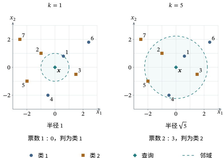
图 3.4 同一查询下的近邻范围与投票变化。教学构造取 n = 7 、 d = 2 、无量纲坐标和欧氏距离，查询为 \mathbf{x} = (0, 0) ；两图的样本、编号及坐标尺度完全相同，具体坐标见正文。蓝色圆点表示类 1，赭色方点表示类 2，青色菱形表示查询，青色虚线圆表示包含边界的近邻范围。左图 k = 1 、半径 1，类 1 与类 2 票数为 1 : 0；右图 k = 5 、半径 \sqrt{5} ，票数为 2 : 3。各邻居等权投票，距离和票数均无并列；点的位置、标签与参数均为人为设定，不代表真实数据实验。
