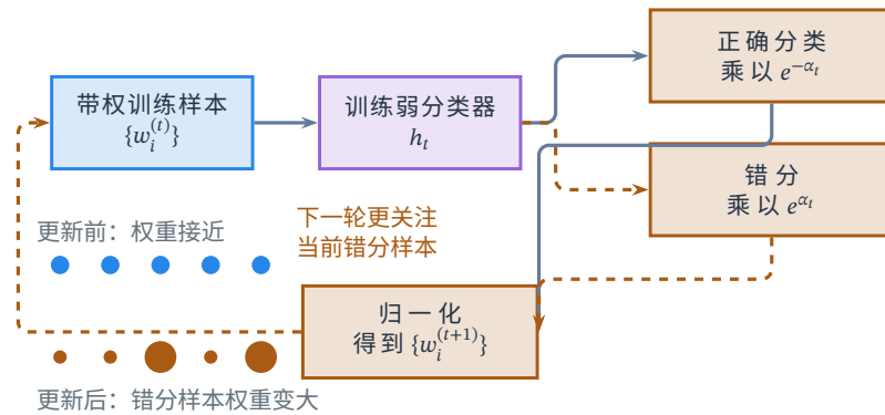
图 6.5 AdaBoost 的样本权重更新。实线表示常规训练与正确分类样本的更新路径，深橙色虚线强调错分样本被放大的反馈路径。圆点大小仅示意相对权重变化，不表示具体样本数或实测权重。
