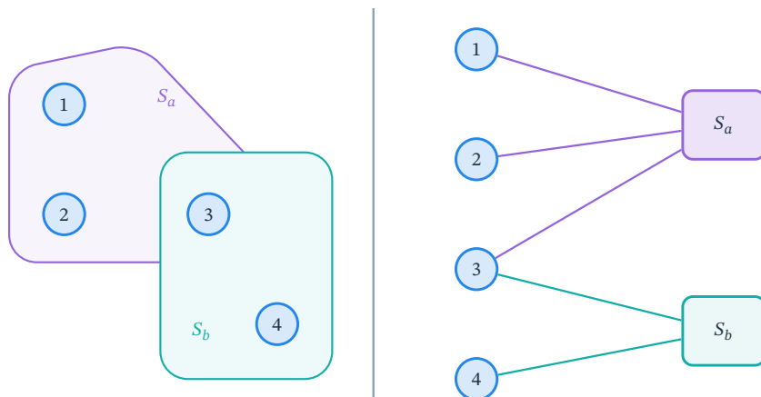
图 11.8 超边及其关联表示。左侧一条超边 S_a 连接节点 1、2、3，另一条超边 S_b 连接节点 3、4。右侧将超边画成方框，以连线表示参与关系；节点 3 向两个关系对象提供信息，并从二者读取聚合结果。方框是关系状态，不是新增的原始参与者。
