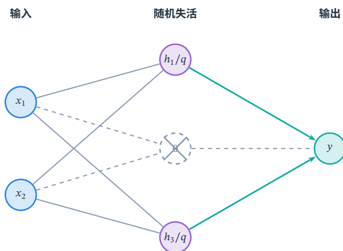
图 15.3 一个三单元隐藏层的构造性 Dropout 示意。中间单元被屏蔽，灰色虚线为本次不参与前向计算的路径，其余实线仍传递信息。此图只展示一个掩码样本；实际保留概率不由图中剩余单元比例决定，训练时按式(15.7)缩放。
