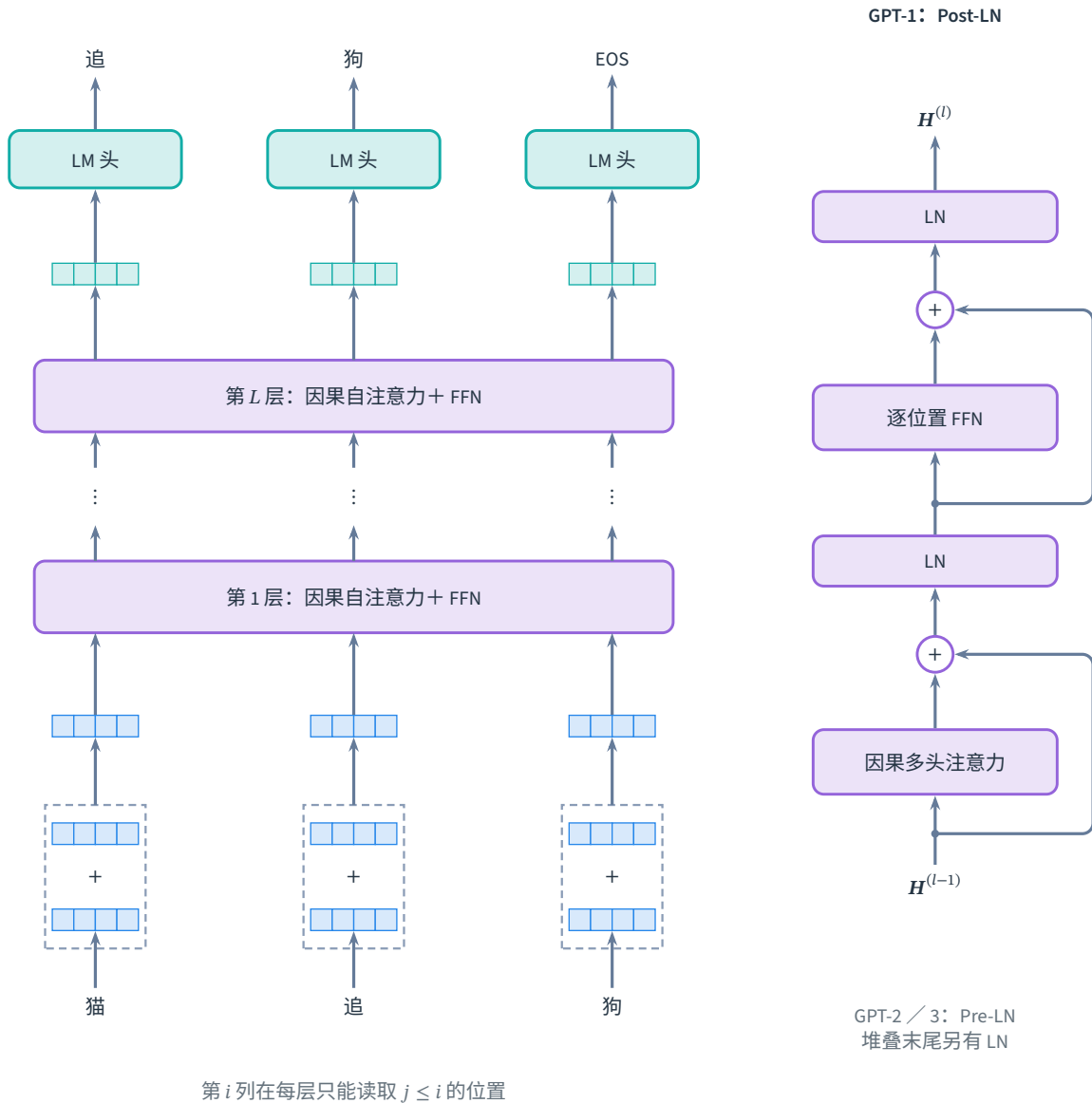
图 12.12 GPT 的因果网络与下一词元监督。每列的词元与位置嵌入相加后，经过整序列网络层，再由 LM 头预测下一词元；“追”所在列只能读取“猫、追”，对应标签为“狗”。每条长条在内部应用因果掩码，中间层省略，LM 头含词表投影与 Softmax。右侧展开 GPT-1 的 Post-LN 层；GPT-2 与 GPT-3 改用 Pre-LN 并在堆叠末尾归一化。格条只示意特征维，省略 Dropout 与 KV 缓存，推理仍逐步生成。参考 Bishop 与 Bishop（2024）图 12.15 的布局重绘。
