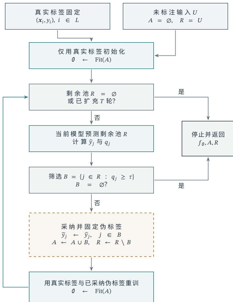
图 3.8 固定阈值、固定已采纳伪标签的自训练流程，对应算法 3.6。真实标签保持不变，虚线框中的伪标签始终是模型预测。每次采纳后先重训，再用更新后的模型处理剩余候选；空池、无样本通过筛选或达到轮数上限时停止。这个模型反馈回路也可能产生确认偏差：错误预测被当作后续监督，使模型进一步强化原有误判。
