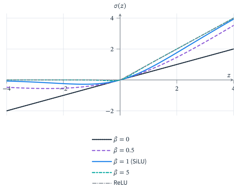
图 8.6 Swish 在不同 \beta 下的函数图像。 \beta = 0 给出线性函数 z/2 , \beta = 1 就是 SiLU, 较大的 \beta 逐渐形成接近 ReLU 的响应。图中参数固定为 0, 0.5, 1, 5, ReLU 用作极限参照; 它不展示可学习 \beta 在某次训练中的实际轨迹。
