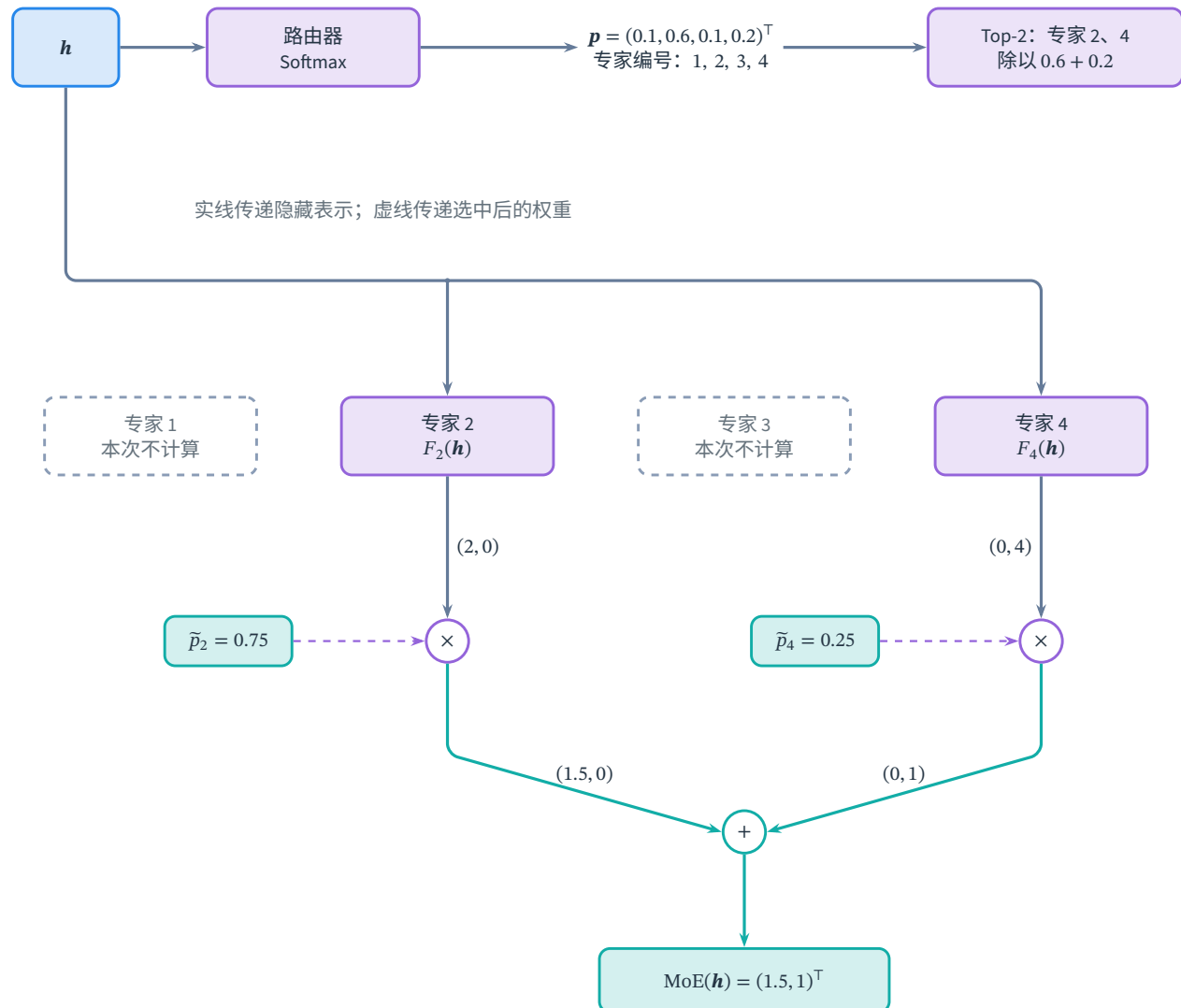
图 12.24 Top-2 混合专家的一次完整计算，概率与二维专家输出均为教学设定。上方路由器选出专家 2、4 并给出重新归一化的权重；下方实线传递隐藏表示及专家结果，虚线向乘法节点提供标量权重。专家输入始终是同一个 h ，加权发生在专家输出之后，最终 0.75(2, 0)^T + 0.25(0, 4)^T = (1.5, 1)^T 。灰色专家 1、3 本次不计算；图省略容量限制、辅助训练目标及块外残差。
