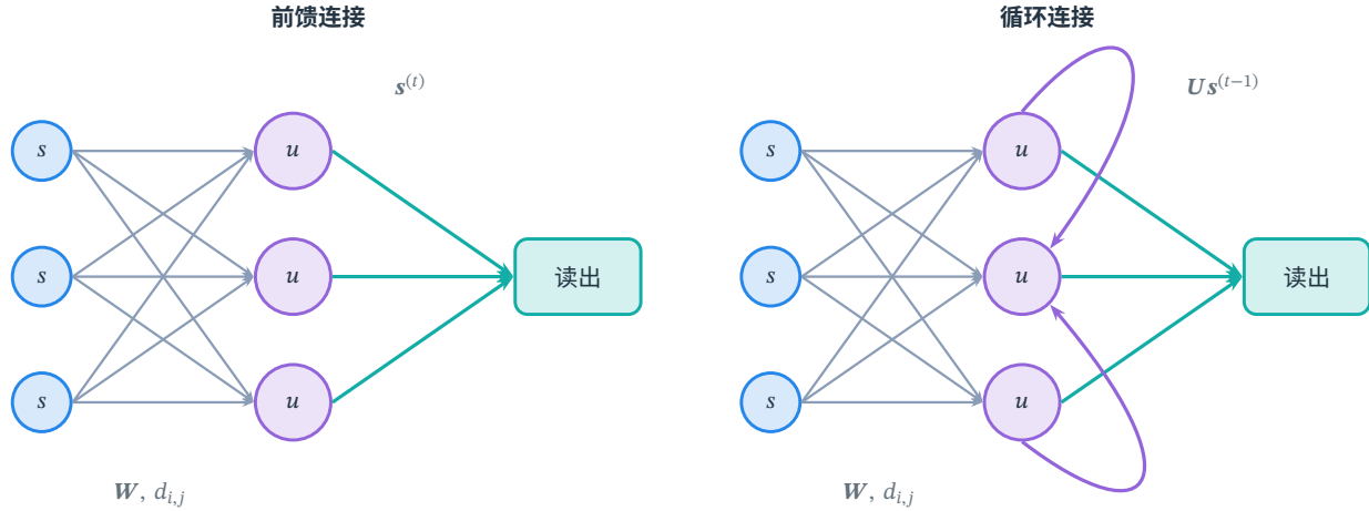
图 13.4 脉冲前馈网络与循环网络的构造性比较。圆内 u 表示各单元保存膜电位，箭头传递离散发放，青色方框为输出读出。左图只保留层间前馈连接；右图增加使用上一时间步脉冲的循环边 U 。边还可带权重与传播延迟，图中只标出一条代表连接。神经元数和连边用于说明结构，不对应训练模型。
