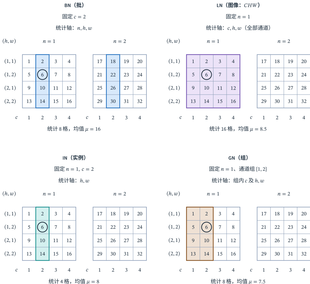
图 14.5 在 N = 2, C = 4, H = W = 2 的图像张量上, 对同一元素 X_{1,2,1,2} = 6 比较统计伙伴。按样本、空间行、通道的展示顺序填入教学数值 1 至 32, 每行标出 (h, w) ; 并非按张量存储顺序编号。蓝、紫、青、橙分别标出 BN、LN、IN、GN 的统计集合, 边界轮廓与固定/统计索引提供颜色之外的读法, 深色圈为目标元素。GN 取通道组 \{1, 2\} ; LN 统计整幅图像的 CHW, 不是 Transformer 逐词元的特征维 LN。均值用于核对范围, 未加入仿射变换。
