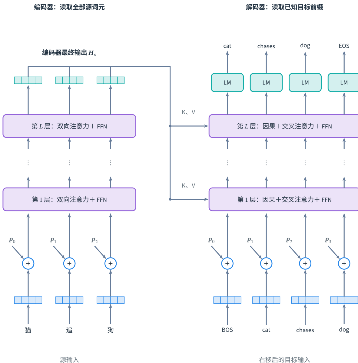
图 12.8 将“猫／追／狗”翻译为“cat / chases / dog”的整网结构。每个长条表示作用于整段序列的一层，中间省略的层数由网络配置决定；词元列保持位置对应。训练时右移的目标输入分别预测 cat、chases、dog、EOS。左侧最终源表示经同一条侧路供每个解码器层的交叉注意力生成 K、V，Q 来自该层目标路径；不会把某个中间编码层与同编号解码层一一配对。省略层内残差、归一化与 Dropout。参考 Bishop 与 Bishop (2024) 图 12.20 的布局重绘。
