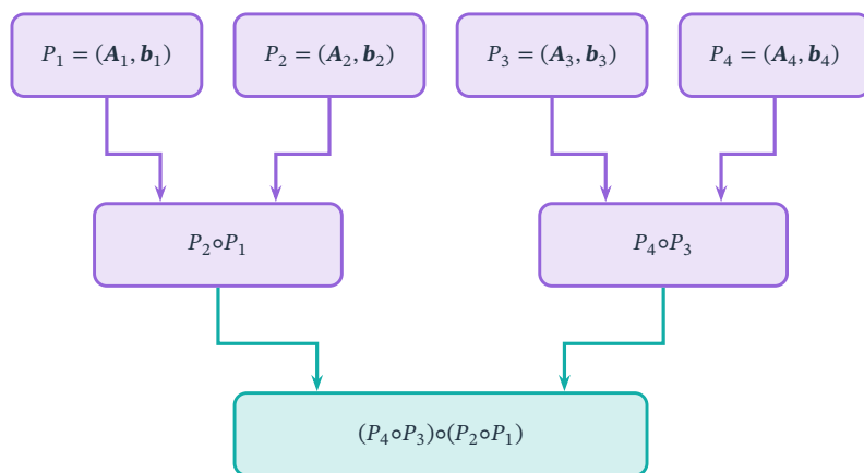
图 10.10 仿射状态更新的有序组合。四个单步变换先组成两个连续片段，再组成整段； Q \circ P 表示先执行 P 再执行 Q 。平衡组合树展示的是扫描中的汇总阶段，完整前缀扫描还要把此前片段的結果传给各位置，才能得到每步状态。树形计算可缩短依赖深度，但不改变输入顺序。
