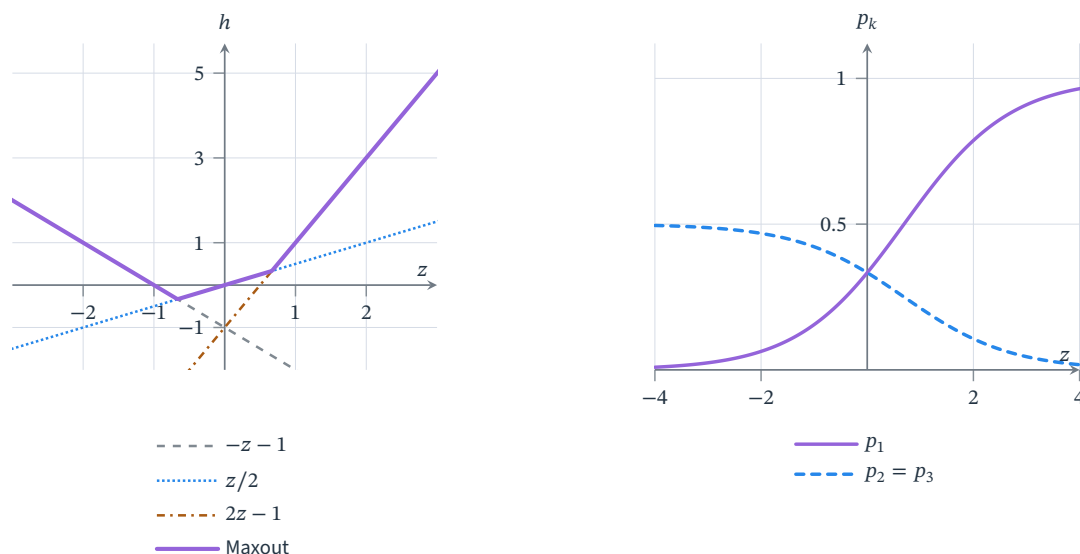
图 8.8 Maxout 和 Softmax 的一维观察方式。左图取三个仿射候选 -z-1 、 0.5z 和 2z-1 ，粗实线是它们的最大值包络；它展示固定参数后沿一维输入的 Maxout 响应。右图固定三类得分为 (z, 0, 0) ，绘出三项 Softmax 概率，其中 p_2 = p_3 ，用同一条曲线标注。这些切片不能代表所有输入与参数下的唯一函数图像。
