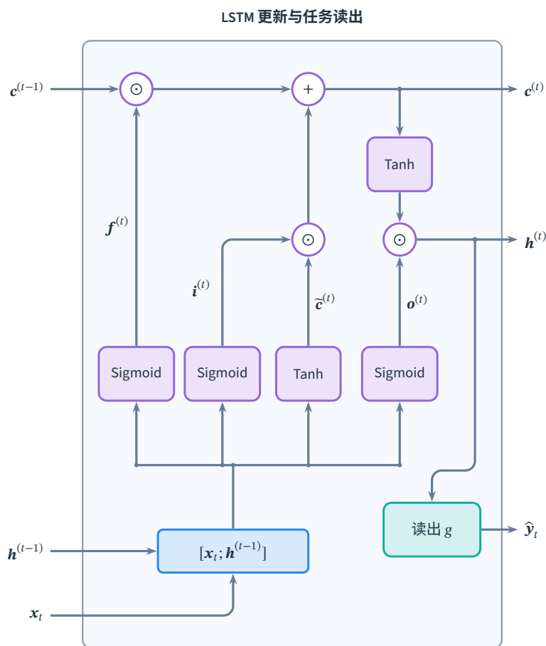
图 10.7 LSTM 更新与任务读出。框外左侧为当前输入 x_t 和旧状态 h^{(t-1)}, c^{(t-1)} ，右侧为新状态和预测 \hat{y}_t = g(Vh^{(t)} + c) 。四个门/候选模块各自包含仿射映射；圆形 \odot 与 + 分别表示逐元素乘法和相加。灰色箭头表示数据流，蓝框为组合输入，紫框为状态计算，青框为任务读出。
