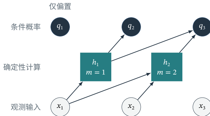
图 26.2 MADE 的合法计算路径。方框表示确定性隐藏计算, 圆框表示输入或条件分布输出; 输出 q_i 代表 p(X_i = 1 | \mathbf{x}_{<i}) 。隐藏单元的次序号限定可读前缀, 任何输出 q_i 都不能通过路径访问 x_i 或更后的输入。
