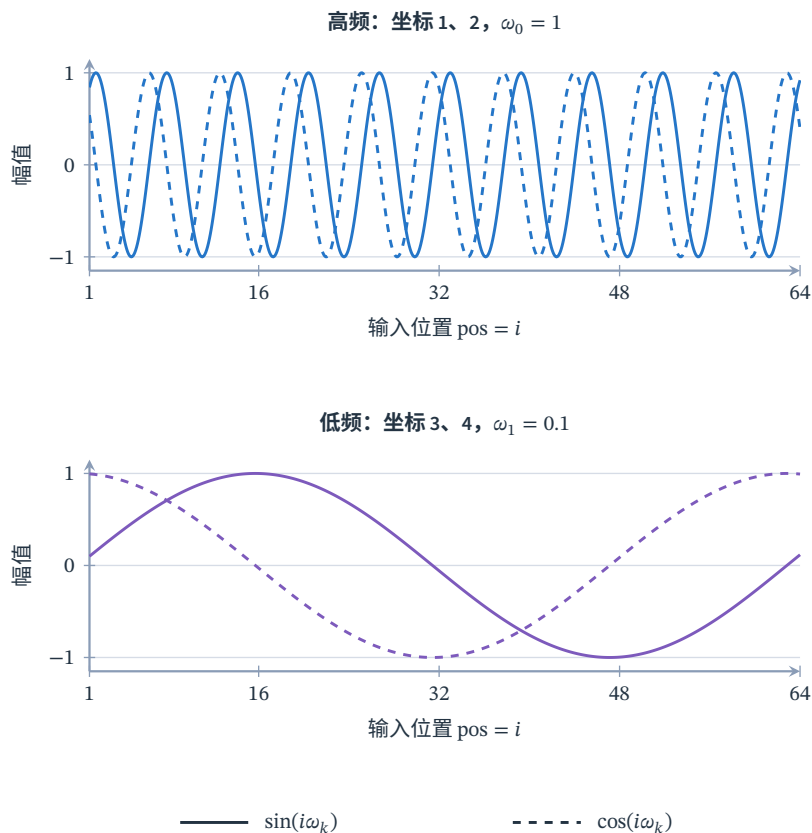
图 12.14 固定正弦编码中选定坐标随输入位置的变化。取 d = 8 ，上图为坐标 1、2 ( k = 0 )，下图为坐标 3、4 ( k = 1 )；两图横轴范围相同，幅值无量纲。实线为正弦，虚线为同频余弦，周期分别约为 6.28 和 62.83 个位置。连续曲线帮助观察波形，实际序列只在整数位置取值；本图仅示意选定维度，不是完整八维编码或训练结果。
