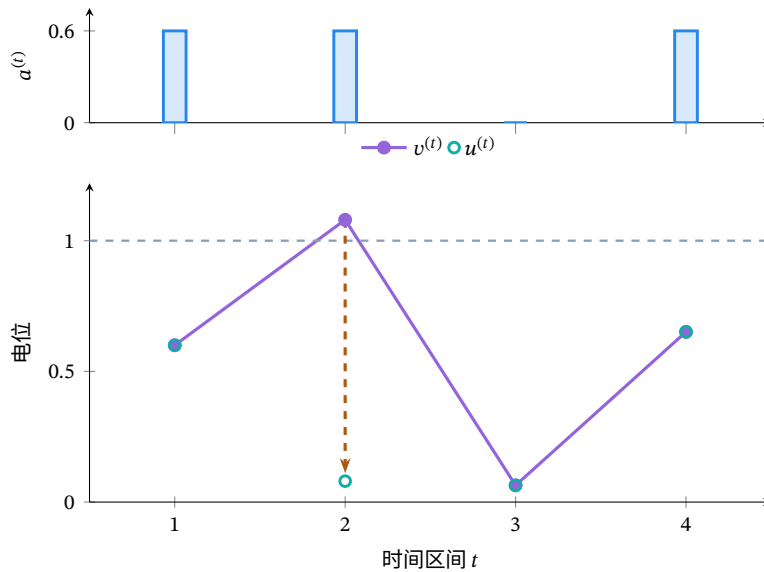
图 13.3 示例 13.1 的离散 LIF 计算。蓝色竖线表示输入增量，紫色实线连接检测前电位 v^{(t)} ，青色空心圆为复位后电位 u^{(t)} ，虚线为阈值；第二步检测后发放并减去 1。连线帮助比较离散状态，不表示步间的连续电位轨迹。
