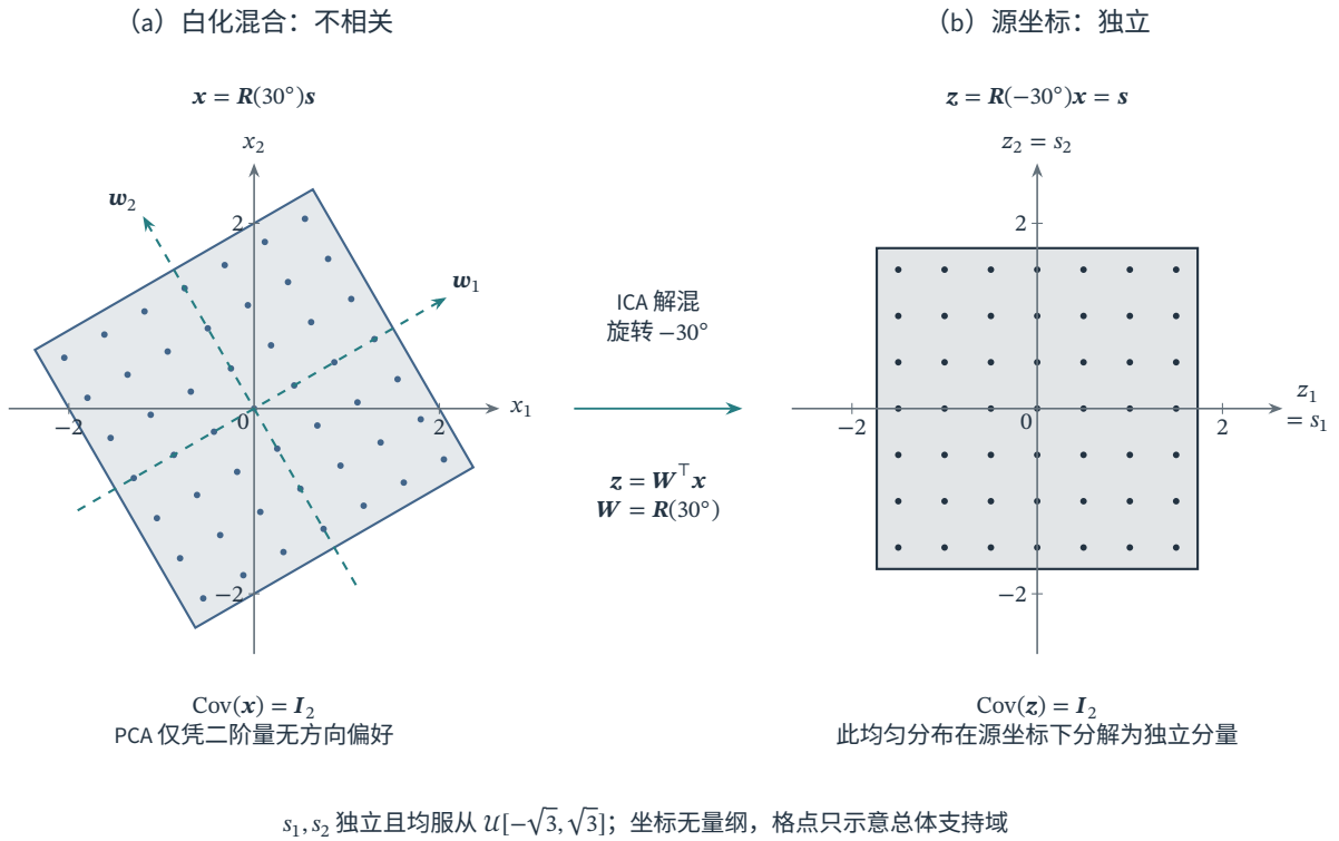
图 5.3 白化与独立源恢复的区别。设 s_1, s_2 独立且均服从 \mathcal{U}[-\sqrt{3}, \sqrt{3}] , \mathbf{R}(\theta) 为逆时针旋转矩阵。左图为 \mathbf{x} = \mathbf{R}(30^\circ)\mathbf{s} , 右图为逆旋转恢复的 \mathbf{s} ; 两者协方差均为 \mathbf{I}_2 , 只有右侧所示坐标对应独立源。实线轮廓为总体支持域, 圆点为确定性格点, 虚线箭头为解混方向。图为无量纲构造示意, 未运行 ICA 优化; 该方形解混本身不减少维数。
