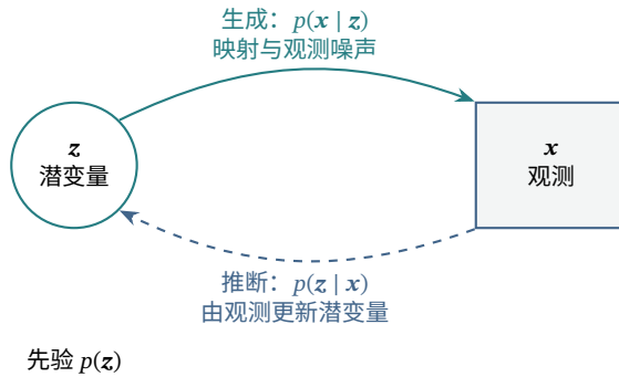
图 5.10 概率生成与后验推断的结构示意。实线表示 \mathbf{z} \rightarrow \mathbf{x} 的生成方向; 虚线表示 \mathbf{x} \rightarrow \mathbf{z} 的后验推断, 不是额外的生成依赖。图中节点与箭头只说明变量角色和条件关系, 不表示实测数据、网络层数或计算流程; 噪声描述观测对信号的偏离, 不是新增的潜变量维数。
