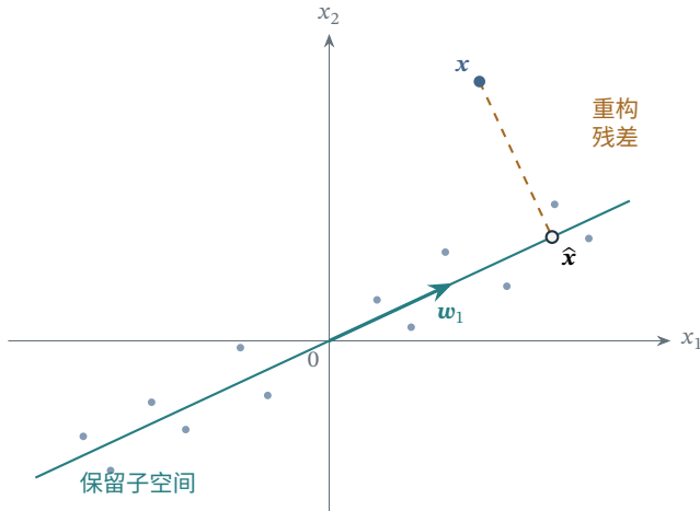
图 5.1 二维到一维的正交投影示意。实线方向 w_1 张成保留子空间，点 x 投到 \hat{x} ，虚线为与子空间垂直的重构残差。图中散点为示意位置，未表示真实实验。
