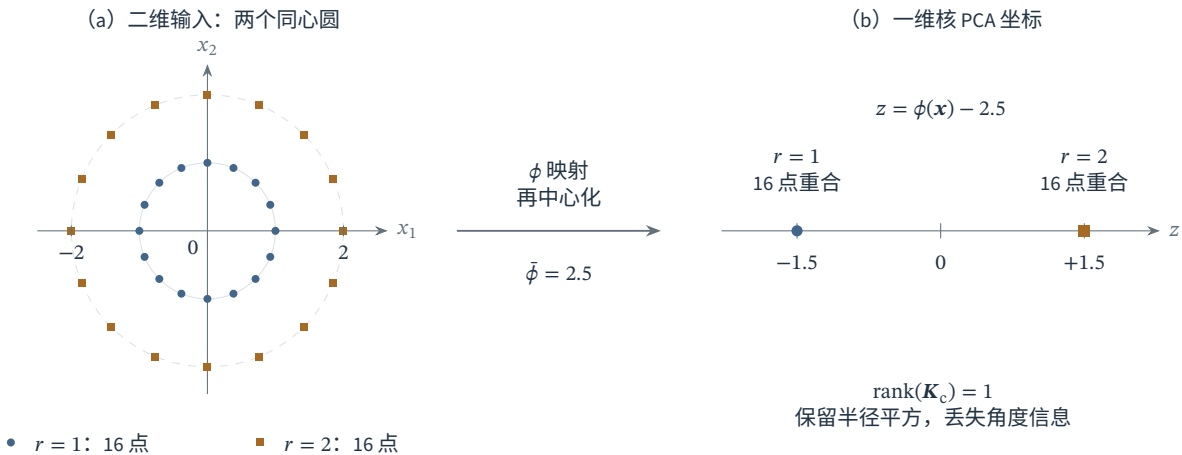
图 5.5 由核选择保留量的构造例子。左图在半径为 1, 2 的圆上各取 16 个等角度样本, 圆点与方点区分两圈。所示特制核对应标量特征 \phi(\mathbf{x}) = \|\mathbf{x}\|_2^2 , 中心化核矩阵秩为 1; 选择图示主轴方向, 核 PCA 坐标为 \pm 1.5 。右侧每个标记表示 16 点重合, 坐标无量纲。此结果依赖所选核, 不能推广为任意高斯核或多项式核的输出。
