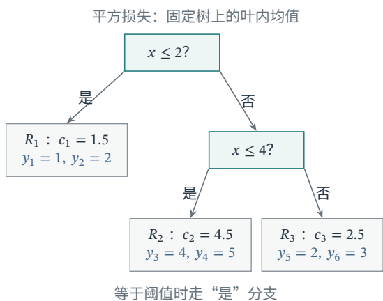
图 2.4 给定阈值树与分段常数预测。六个无量纲教学样本按 x 递增排列；按 x \leq 2 及右分支上的 x \leq 4 划分后，三组响应分别为 (1, 2) 、 (4, 5) 、 (2, 3) ，叶均值为 1.5、4.5、2.5。蓝色点表示样本，墨色虚线表示预测，青色竖线表示阈值；阈值处实心、空心端点区分取与不取该值。右图只显示 0 \leq x \leq 6 ，树结构预先给定。
