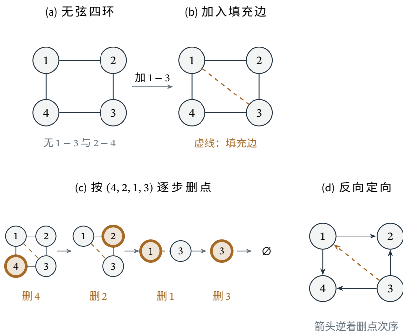
图 19.2 从无弦四环到完美有向图。先加入虚线填充边 1-3 完成弦化，再按完美消除序 (4, 2, 1, 3) 逐步删点；每幅删点快照用双圈和“删”字同时标出当前节点。最终从序中较晚节点指向较早节点，得到 3 \rightarrow 1 、 1 \rightarrow 2 、 3 \rightarrow 2 、 1 \rightarrow 4 和 3 \rightarrow 4 ；实线箭头来自原四环，虚线箭头来自填充边。
