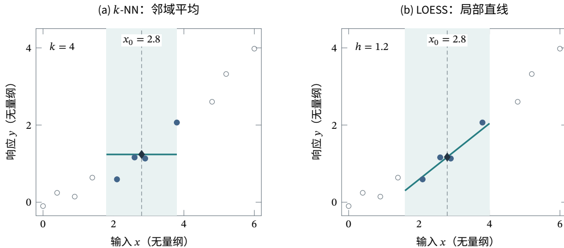
图 2.3 同一查询点上的邻域平均与局部线性拟合。横、纵轴均无量纲，所有点均为构造样本；空心点为未使用样本，蓝色实心点为本次使用的四个样本，菱形为 x_0 = 2.8 处的预测。左图取 k = 4 、等权平均，预测约为 1.238；右图取 h = 1.2 与三立方距离权重，不做残差重加权，局部线性预测约为 1.171。浅色带标出各自的邻域，两图同时改变了局部函数形式和权重，不据此断言某种方法总是更准。
