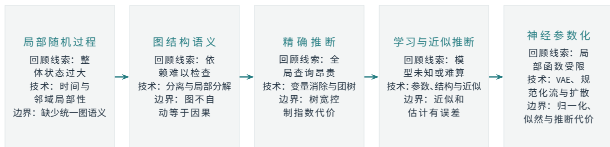
图 16.3 按本书问题线索组织的概率图模型现代回顾。图中的“回顾线索”联系问题、技术与边界；箭头表示讨论的问题逐步扩展，不表示后出现的技术取代了此前方法。
