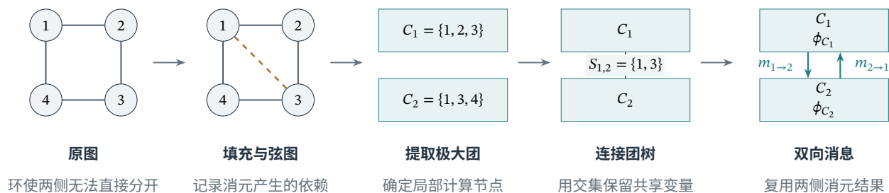
图 21.2 团树编译与传播总览。四环先通过填充边 1-3 变为弦图，再提取极大团 C_1 = \{1, 2, 3\} 与 C_2 = \{1, 3, 4\} ；以分隔集 S_{1,2} = \{1, 3\} 连接两个团后，原始因子被唯一分配到团势，双向消息分别汇总树边两侧的贡献。团树的节点和边属于计算结构，不是把原变量图改画成树。
