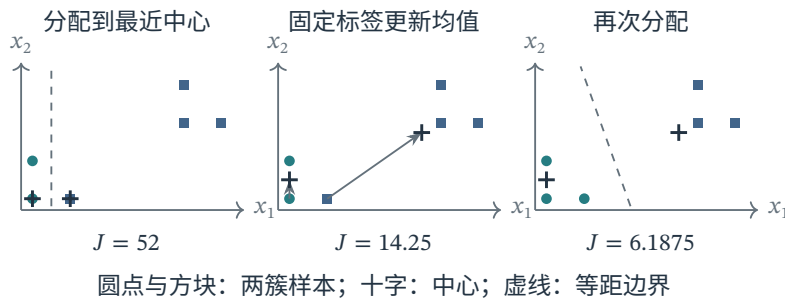
图 4.1 Lloyd 迭代的教学例，六个样本为 (0,0)、(0,1)、(1,0)、(4,2)、(4,3)、(5,2)，初始中心为 (0,0) 和 (1,0)。首次更新后中心为 (0,0.5) 和 (3.5,1.75)；图中依次展示分配、均值更新与再次分配。
