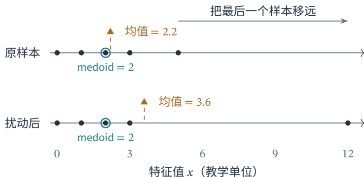
图 4.2 中心样本与均值对极端值的不同反应。固定 K = 1 , 上方样本为 \{0, 1, 2, 3, 5\} , 下方只把 5 改为 12; 黑点为观测, 圆圈标出绝对距离下的 medoid, 三角形标出平方距离下的最优均值。
