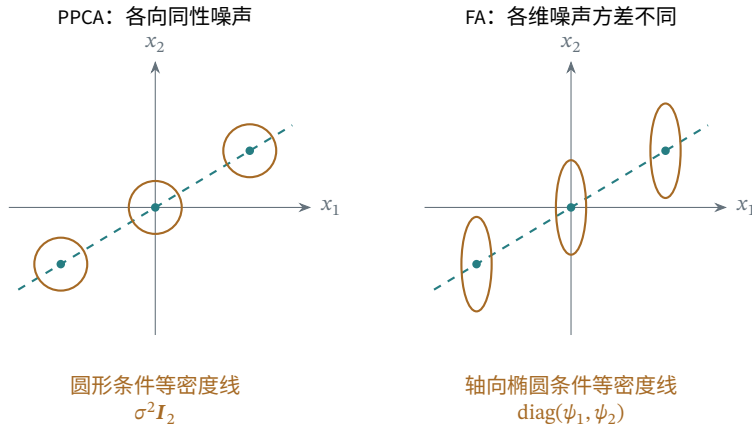
图 5.11 PPCA 与 FA 的条件噪声示意。设 d = 2 、 k = 1 、 \boldsymbol{\mu} = \mathbf{0} 、 \mathbf{W} = (1, 0.6)^\top , 三个实心点对应 z = -1, 0, 1 的条件均值。左图取 \sigma = 0.28 , 右图取 \Psi = \text{diag}(0.16^2, 0.50^2) ; 每条轮廓到其中心的平方 Mahalanobis 距离均为 1。坐标为无量纲构造值, 轮廓是条件等密度线, 不是总体数据云或置信区域。
