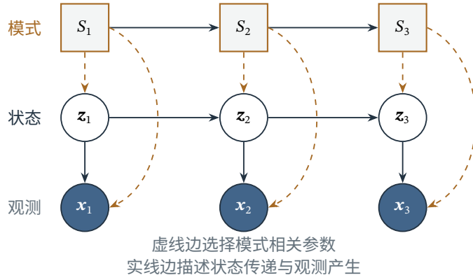
图 28.3 切换线性动态系统的三层展开。方形节点为离散模式，空心圆为连续状态，填充圆为观测。给定完整模式路径后，连续部分可用 Kalman 递推；只给定当前模式不足以合并具有不同历史的所有高斯分量。
