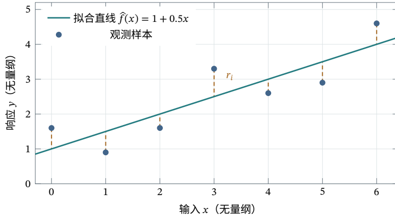
图 2.1 一维 OLS 与响应残差。七个构造样本的最小二乘直线为 \hat{f}(x) = 1 + 0.5x ；蓝色实心点表示观测，青色实线表示预测，赭色竖虚线表示 r_i = y_i - \hat{f}(x_i) 。横、纵轴均为无量纲教学变量。
