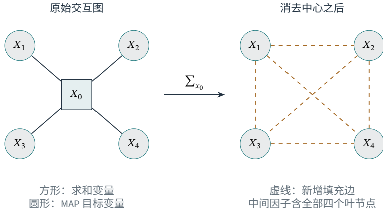
图 20.2 边缘 MAP 引起的填充，图中 k = 4 。左侧中心 X_0 要求和，四个叶节点要共同最大化；右侧消去中心后，叶节点由虚线填充边连成团。若是 MPE，则可以先消叶节点，此时不产生这些填充边。
