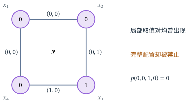
图 18.6 零概率破坏逆向分解的反例。节点给出被禁止配置 \mathbf{y} = (0, 0, 1, 0) 的取值，边旁的局部取值对按变量下标递增排列；每一对都出现于表 18.2 的某个正概率配置。若存在非负边势分解，这四个边势值就必须都为正，其乘积也为正，与 p(\mathbf{y}) = 0 矛盾。这里不否定“因子分解推出 Markov 性质”的方向。
