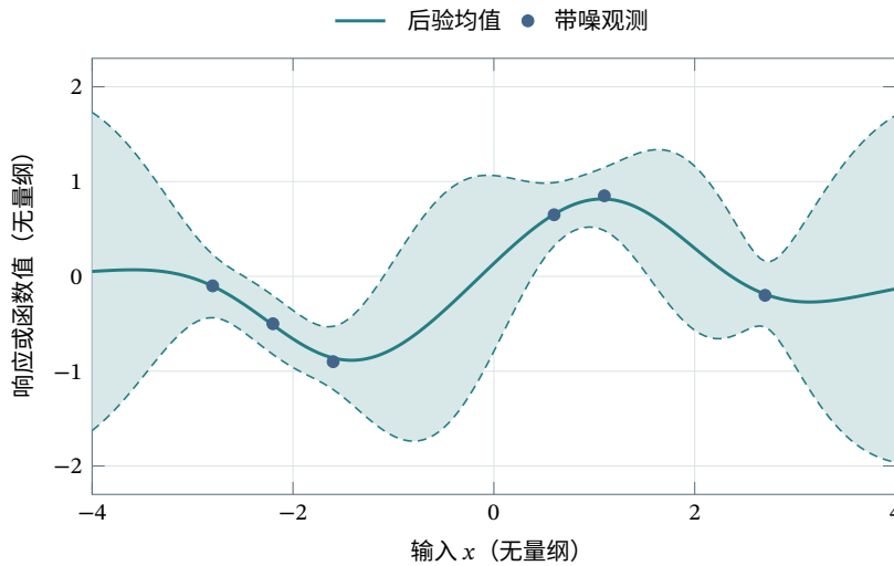
图 2.5 高斯过程的后验均值与函数不确定性。六个点为构造观测; 先验均值为零, 平方指数核取 \ell = 0.9 、 \sigma_f = 1 , 观测噪声标准差为 \sigma = 0.18 。实线为 \mu_\star , 浅色带及虚线边界为 \mu_\star \pm 1.96\sqrt{\mathbf{v}_\star} , 表示潜在函数值的逐点约 95% 后验可信区间。它不是整条函数的同时可信带; 预测未来带噪声响应时, 方差还须加 \sigma^2 。
