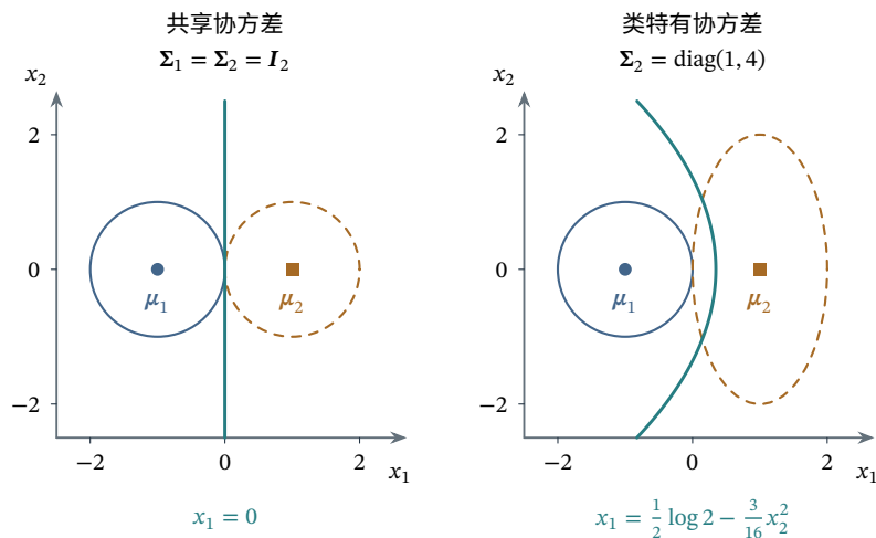
图 3.7 两图均取 \pi_1 = \pi_2 = 1/2 、 \mu_1 = (-1, 0)^T 、 \mu_2 = (1, 0)^T 和 \Sigma_1 = I_2 , 仅第 2 类协方差变化。蓝色圆点和赭色方点为均值, 蓝色实线与赭色虚线分别为 \Delta_1 = 1 和 \Delta_2 = 1 的等密度轮廓; 不同类的这些轮廓不保证密度值相同。青色粗线按 g_1 = g_2 的解析式绘制, 左为直线, 右为抛物线。参数均为教学构造, 不是采样或拟合结果。
