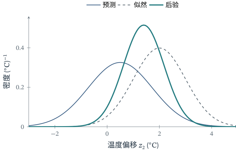
图 28.2 标量 Kalman 更新的可复算密度。蓝色实线为预测 \mathcal{N}(0.5, 1.5) ，灰色虚线为对状态归一化后的似然 \mathcal{N}(2, 1) ，青色粗线为后验 \mathcal{N}(1.4, 0.6) 。横轴是温度偏移，纵轴是密度；本例观测矩阵为 1，似然才可直接画成同一坐标下的归一化密度。
