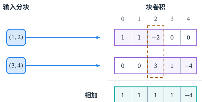
图 9.11 重叠相加的数值例子。输入在原位置零和二分别开始两个长度二的块，块内补零后计算与 (1, -1) 的完整卷积，恢复到图上的五个全局输出位置。紫色区域表示该块可能产生贡献的位置，区域外记为零。虚线框内的两项贡献相加为一，最终结果与不分块的线性卷积相同。
