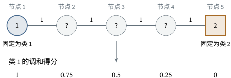
图 3.9 五节点等权无向路径上的硬钳制标签传播。每条边权重为 1，左端圆形节点固定为类 1，右端方形节点固定为类 2，问号表示未知标签。下方列出精确调和解的类 1 得分，类 2 得分为其补数；内点得分等于两侧邻居的平均。中间节点两类并列，按最小类别编号规则判为类 1。这是教学构造，不是实测结果。
