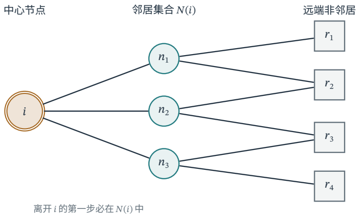
图 18.2 无向图中节点 i 的结构性 Markov 毯。双边框大圆表示中心节点 i ，单边框小圆表示邻居 n_1, n_2, n_3 ，方形表示远端非邻居。图中所有线段都是现存的无向边，统一使用实线；由于 i 不与方形节点直接相连，从 i 通向远端节点的路径都先经过 N(i) 。
