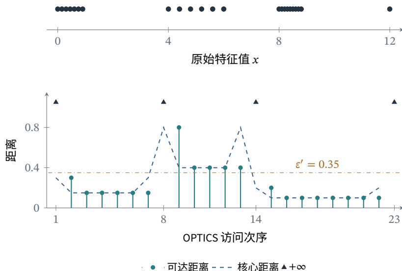
图 4.4 固定一维教学数据上的 OPTICS 排序，取 \text{MinPts} = 3 (含自身)、 \epsilon_{\max} = 1.1 。三组样本的间距分别为 0.15、0.4、0.1，另有 x = 12 的孤立点。实线竖棒为可达距离，蓝色虚线为核心距离；无穷可达距离用顶部三角形表示，不能按其显示高度作数值比较。
