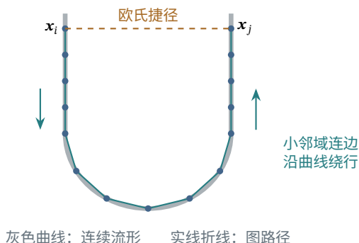
图 5.6 一维弯曲曲线上的距离示意。曲线表示嵌入观测空间的一维流形，曲线上的点表示离散样本；连接两个目标点的直线表示欧氏距离，沿相邻样本连接的折线表示邻域图路径，其各段长度之和用于近似沿曲线的测地距离。直线穿过曲线之外的区域，不能视为沿流形行走；若将这样的连接误纳入邻域图，就会形成低估测地距离的短路。图为几何示意，不是算法输出或实验结果，未给出数值误差。
