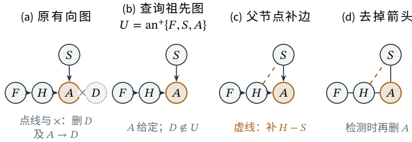
图 19.1 查询祖先图的道德化过程。原有向图在报警节点 A 后接一个后代 D ；对查询 F \perp S \mid A ，祖先闭包 U = \{F, H, A, S\} 依赖端点和条件集，因而先删去不在 U 中的 D 及其关联边 A \rightarrow D 。点线轮廓、点线有向边与 × 共同标识这些待删元素；随后在共同子节点 A 的父节点 H, S 之间加入的虚线专门编码补边，并用“补 H-S ”直接标注。最后去掉原边的箭头得到查询祖先图的道德图；检测该查询时还要删除条件节点 A 。橙色填充并配合“给定”文字标识条件节点。
