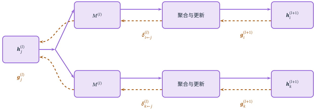
图 11.4 一份节点状态的梯度来自多条读取路径。节点 j 分别向 i, k 发送消息，实线表示前向计算，深橙虚线表示从下一轮状态回到消息及发送端的导数。两份贡献在 \mathbf{h}_j^{(l)} 处相加；图省略其他邻居的消息、接收节点自身的更新分支和任务输出头。反向依赖由前向读取决定，不要求原图存在反向边。
