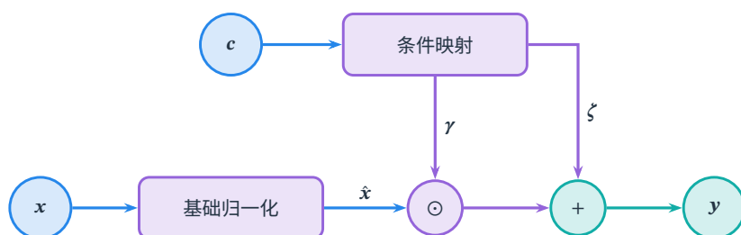
图 14.4 条件归一化的共同计算图。蓝色内容路径产生 \hat{x} , 紫色条件映射产生缩放 \gamma 与偏移 \zeta , 圆形节点分别表示逐元素乘法与加法。条件既可以是风格统计, 也可以是类别、文本或时间等输入; 空间调制还让仿射参数随位置变化。
