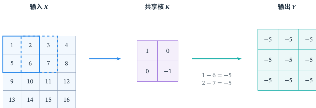
图 9.2 共享核在二维矩阵上滑动的教学例子。蓝色实线和虚线分别框出相邻的两个 2 \times 2 输入窗口，紫色矩阵为不翻转的核，青色矩阵为互相关输出。每个输出计算窗口左上数值减去右下数值，因此均为 -5；两个位置使用同一组权重。
