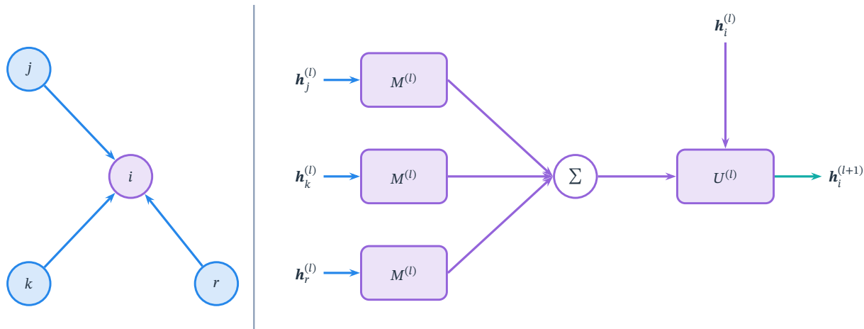
图 11.1 节点 i 的一轮消息传递。左侧蓝色节点 j, k, r 与紫色节点 i 相连, 右侧分别计算三条消息, 再求和并更新 i 。上方路径把 i 的旧表示送入更新函数。图中省略消息函数对接收节点和边属性的额外输入, 所有节点使用相同的消息与更新规则。
