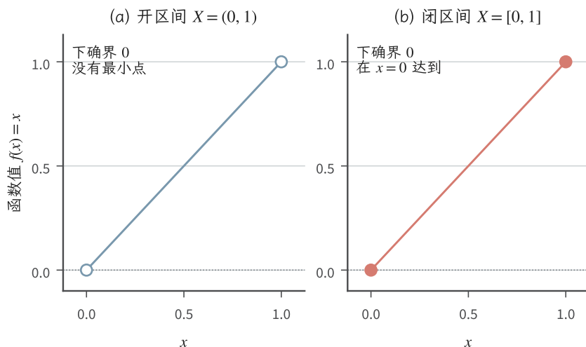
图 1.2 同一函数 f(x) = x 的边界对照。左图定义域为 (0, 1) , 空心端点不属于图像, 函数值可任意接近 0, 却不能取到; 右图定义域为 [0, 1] , 实心端点 (0, 0) 达到下确界。两图的下确界相同, 最小点是否存在取决于可行端点是否保留。图为解析教学示例。
