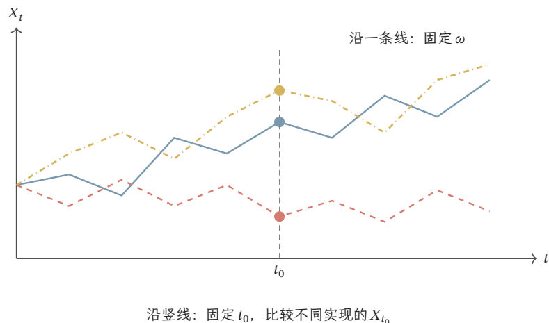
图 10.6 同一过程的路径与时刻截面是不同对象。图为人为给定的三条示意路径, 竖虚线固定时刻 t_0 ; 交点展示该时刻可能出现的不同值, 并非用三条路径估计出的概率密度。
