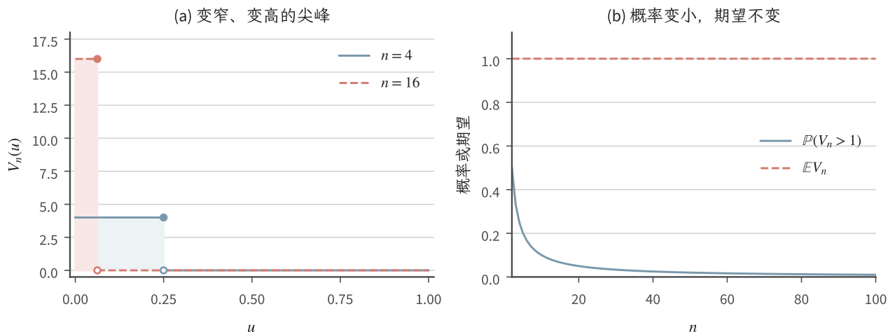
图 10.5 小概率尖峰对期望的贡献 (解析式教学图)。左图为 V_n(u) = nI\{u \leq 1/n\} 在 n = 4, 16 时的取值, 均以面积 1 贡献期望; 右图对 n \geq 2 显示 P(V_n > 1) = 1/n 趋于零, 而 EV_n = 1 不变。基础变量为 U \sim \text{Unif}(0, 1) 。
