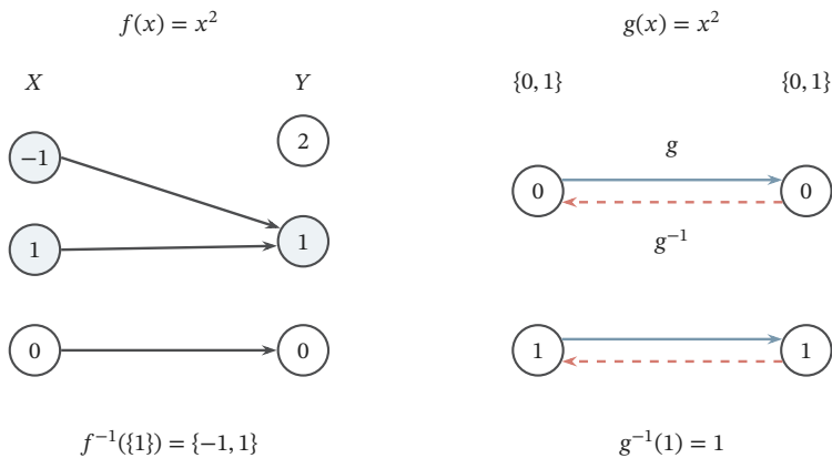
图 1.1 原像与逆映射回答不同问题。左侧 f : \{-1, 0, 1\} \rightarrow \{0, 1, 2\} 按平方取值，标出的 1 有两个原输入，2 没有原输入；原像 f^{-1}(\{1\}) = \{-1, 1\} 仍有定义。右侧将定义域与陪域都限制为 \{0, 1\} 得到双射 g ，实线表示正向求值，虚线表示逆映射，因而 g^{-1}(\{1\}) = \{1\} 是一个元素。两侧均为精确的有限映射。
