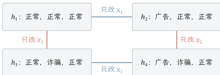
图 2.6 Natarajan 打散的四种预测。每个框中的三项依次对应 x_1, x_2, x_3 ；横向只改变 x_1 ，纵向只改变 x_2 ，而 x_3 始终预测为正常。每个输入处的两个标签预先固定，四个函数实现全部二选一组合。
