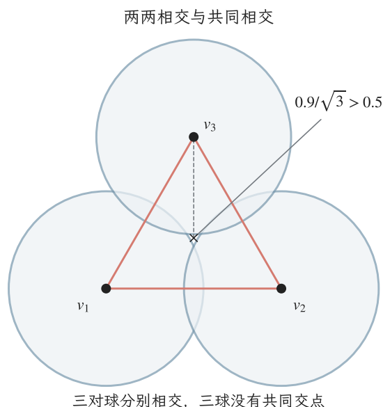
图 7.1 固定同组三点比较共同交集与成对条件。正三角形边长 0.9, \varepsilon = 1 , 蓝色开球半径 0.5; 红色边满足两种构造的连边条件。三球无共同交集, Čech 不含二维面, Rips 含二维面。中心到各顶点的距离为 0.9/\sqrt{3} > 0.5 。圆周只标开球边界, 图为解析教学构造。
