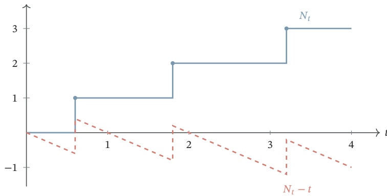
跳跃量同为 1；补偿只加入斜率 -1 的连续漂移
