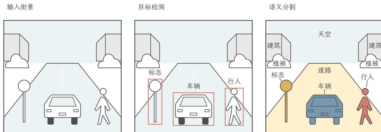
图 1.3 同一构造街景的三种表示。三幅图共用对象与位置；中间用带类别的边界框定位车辆、行人和标志，右侧用不同颜色标识语义区域，细轮廓只辅助辨认对象。图为教学示意，用来比较三种表示所保留的信息。
