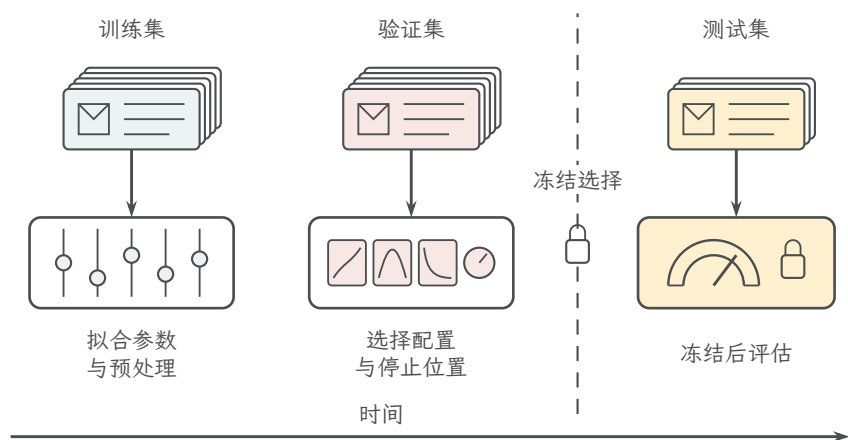
图 1.4 训练集、验证集和测试集的用途。时间箭头表示一种面向未来预测的划分方式；记录数量仅作示意，不代表划分比例。训练集用于参数学习与预处理拟合，验证集用于配置和停止位置的选择，测试集在这些选择冻结后才用于最终评估。
