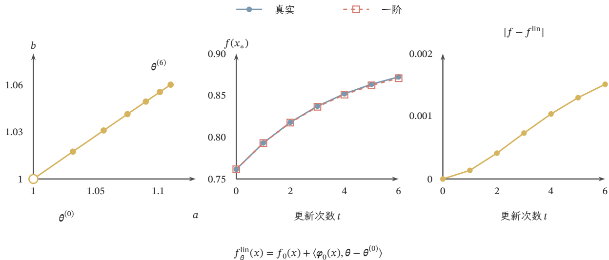
图 8.4 初始化附近的参数轨迹与输出线性化。教学网络为 f_{(a,b)}(x) = a \tanh(bx) ，初值为 (1, 1)^\top ；用单个样本 (x, y) = (1, 0.9) 的半平方损失、步长 0.3 执行六次梯度下降，连同初值共七个检查点。中间的真实输出和一阶输出均在左侧同一参数轨迹上计算；三面板绘图区大小相同，参数、输出和绝对余项各用所标坐标范围，不能按纸面高度直接比较数值。右侧余项末次约为 0.00152。近初始化时二者接近，但余项非零。参数增量经初始雅可比映射到输出/函数空间的切空间；NTK 是初始梯度在不同输入上的内积。此有限网络示例展示近似对象，不证明训练中核恒定或新输入上的误差受控。
