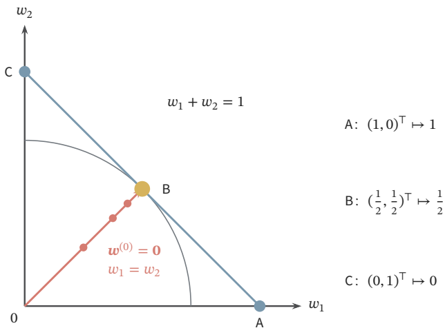
图 8.6 一个训练观测对应多个插值参数。直线上的 A、B、C 都使输入 (1,1)^T 的预测为 1，右侧列出它们对同一新输入 \mathbf{x}_{\text{new}} = (1,0)^T 的预测。对半平方损失从零初始化，图中以步长 1/4 画出前三次更新，轨迹趋向 B；细弧表示经过 B 的欧氏范数等值线，说明 B 是插值直线上距离原点最近的点。这个教学例子解释选解规则，不给出新输入的真实标签或泛化保证。
