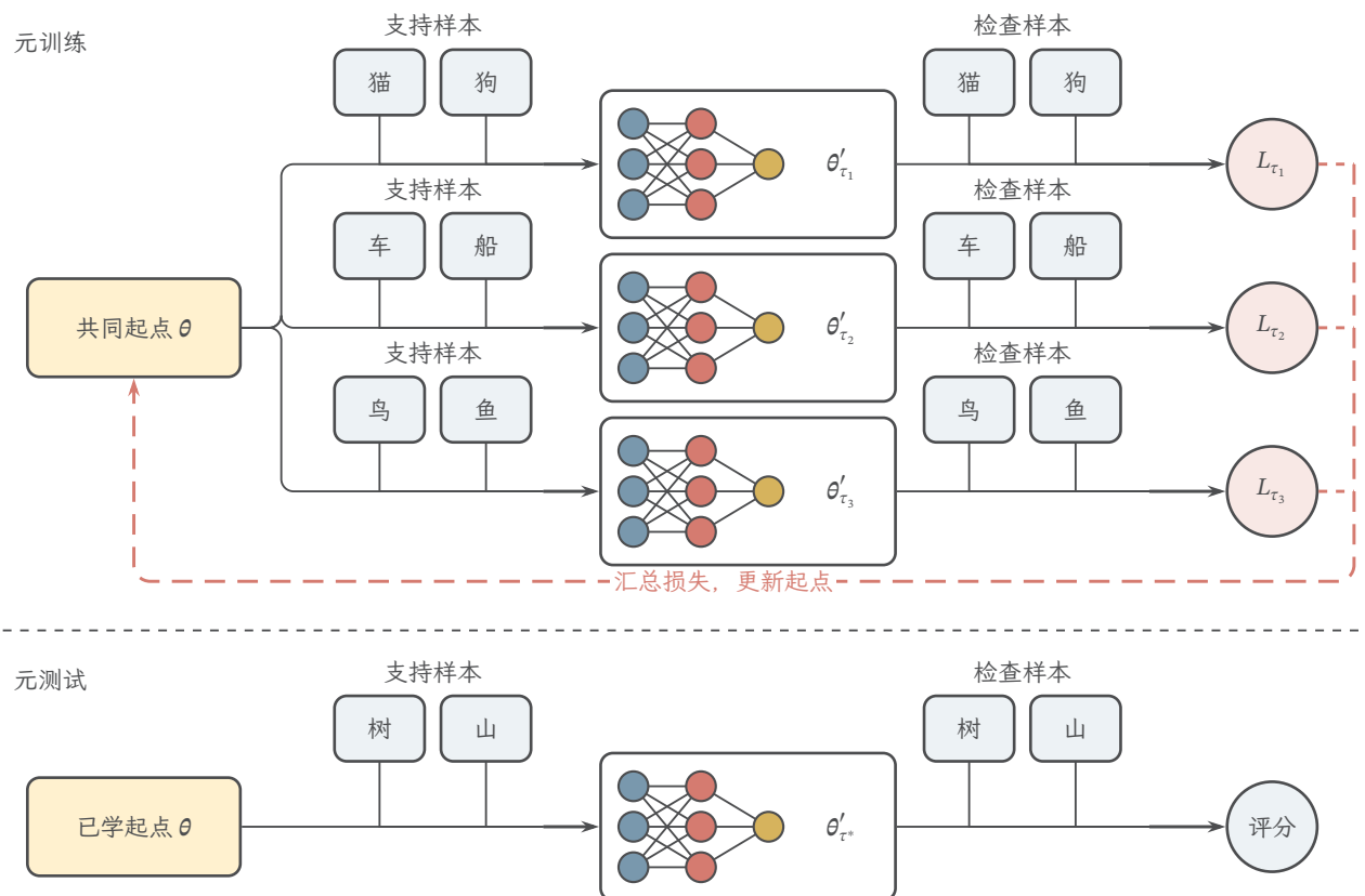
图 3.12 任务内适应与跨任务更新。元训练任务从共同起点 \theta 出发，用支持样本得到适应参数 \theta'_\tau ，再汇总检查损失 L_\tau 更新起点；两批样本都参与元训练。元测试的新任务只用支持样本适应，检查评分不回传共同起点。任务与类别名为教学构造，同名卡片代表同一类别的不同记录，不是 Omniglot 原始样本。
