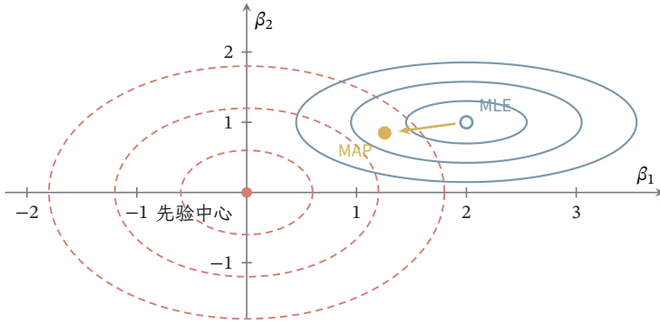
图 2.6 MLE 与 MAP 的参数几何。蓝色实线是以 (2, 1)^T 为中心、两坐标尺度分别为 1 和 0.55 的高斯似然等高线；红色虚线是以原点为中心、尺度为 1.3 的各向同性高斯先验等高线。空心点为 MLE，黄色实心点为两项相加后的 MAP (1.256, 0.848)^T 。该构造用于显示先验如何改变点估计，不代表 MAP 总在两中心的连线上。
