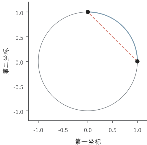
(a) 圆上允许的路径与环境弦
