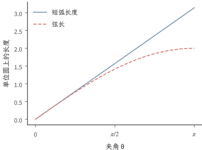
(b) 同一对端点的两种距离
