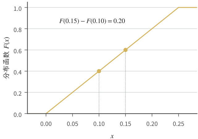
(b) 累积概率的差
