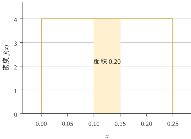
(a) 高度与区间面积
