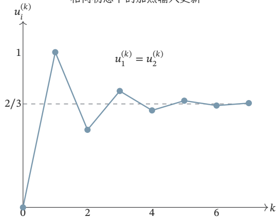
相同初态下的加热输入更新
