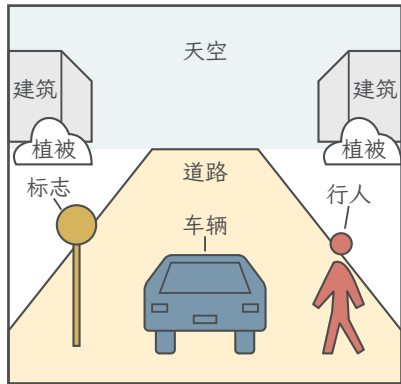
语义分割
