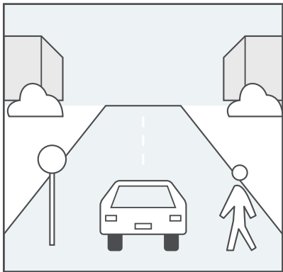
输入街景
