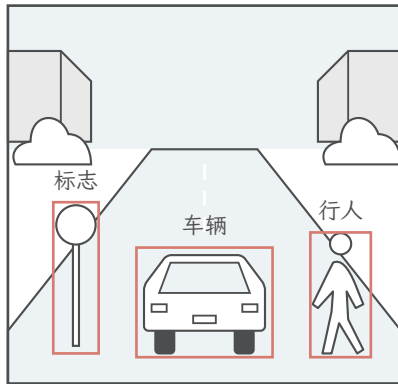
目标检测
