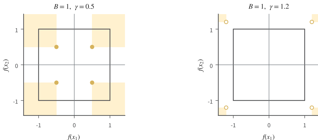
图 2.9 两个分块、 B = 1 与固定阈值 r_1 = r_2 = 0 的输出几何。灰框是函数类允许的 (f(x_1), f(x_2)) \in [-1, 1]^2 ; 浅黄区域要求两坐标分别离阈值至少 \gamma 。左图 \gamma = 0.5 的四种符号可由实心点实现; 右图 \gamma = 1.2 的空心点只标出要求的边界, 全部落在允许框之外, 因而不是类中的函数输出。图为解析教学构造。
