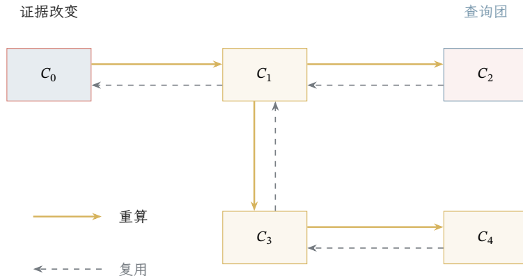
图 21.5 仅 C_0 的局部势改变时的更新方向。实线箭头沿远离 C_0 的方向传播新贡献，反向虚线箭头表示仍可复用的消息；团节点只画名称，具体变量集合须满足运行交集。查询 C_2 时只需更新路径 C_0 - C_1 - C_2 ，其他团的旧边缘不因路径更新而自动全部有效。
