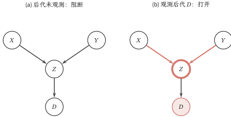
图 17.4 观测碰撞节点的后代也会打开路径。左图中 Z 及其后代都未给定， X \rightarrow Z \leftarrow Y 被阻断；右图只把后代 D 填色为观测， Z 仍空心但用双圈标出已激活的碰撞位置，红色路径因 Z \in \text{an}^+(S) 而打开。图结构只给出是否保证独立，不给出实际依赖强度。
