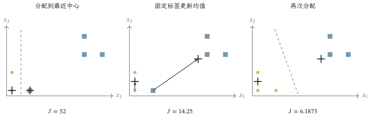
图 4.1 Lloyd 迭代的教學例，六个样本为 (0,0)、(0,1)、(1,0)、(4,2)、(4,3)、(5,2)，初始中心为 (0,0) 和 (1,0)。圆点与方块表示两个簇，十字表示中心，虚线表示等距边界。首次更新后中心为 (0,0.5) 和 (3.5,1.75)；图中依次展示分配、均值更新与再次分配。
