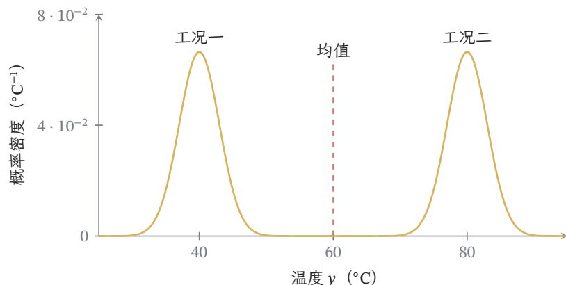
图 16.1 同一个双峰预测分布可以产生均值为 60^{\circ}\text{C} 的点预测。实线为两个等权高斯密度的混合，每个分量的标准差为 3^{\circ}\text{C} ；虚线标出均值。点预测没有保留两个高概率区域的位置。
