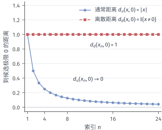
(a) 同一数列 x_n = 1/n
