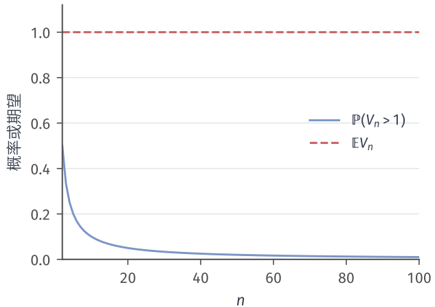
(b) 概率变小，期望不变
