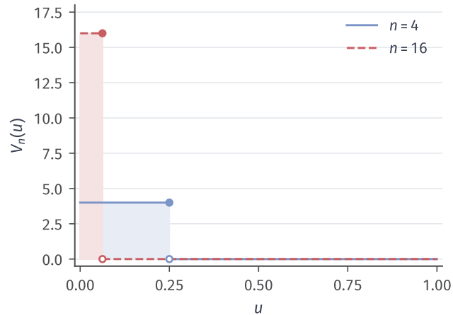
(a) 变窄、变高的尖峰
