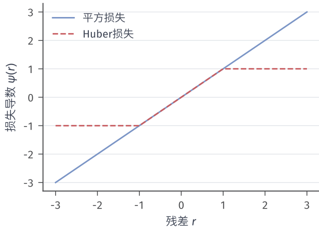
(b) 单个残差的得分贡献
