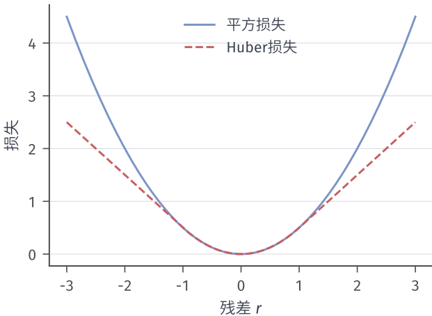
(a) 对大残差的惩罚
