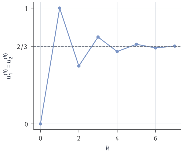
相同初态下的加热输入更新
