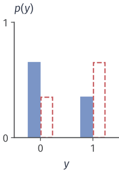
标签偏移
