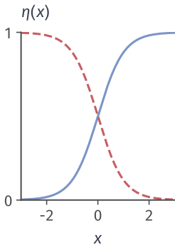
概念偏移
