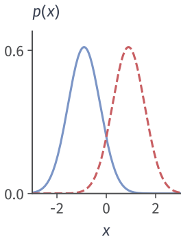
协变量偏移
