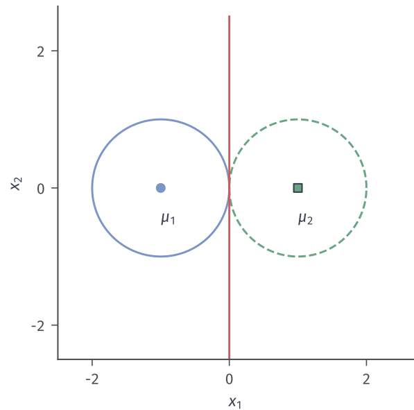
LDA: 共享协方差
