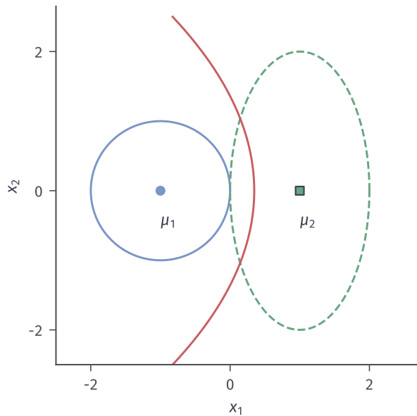
QDA: 类特有协方差
