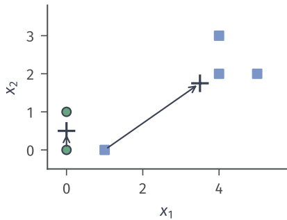
固定标签更新均值
